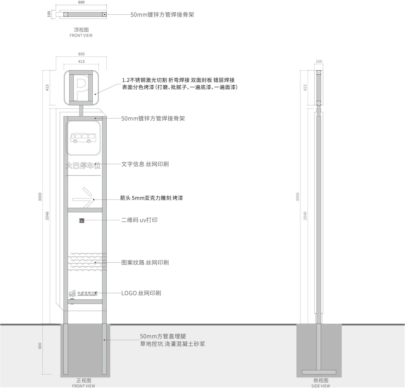
结构图
