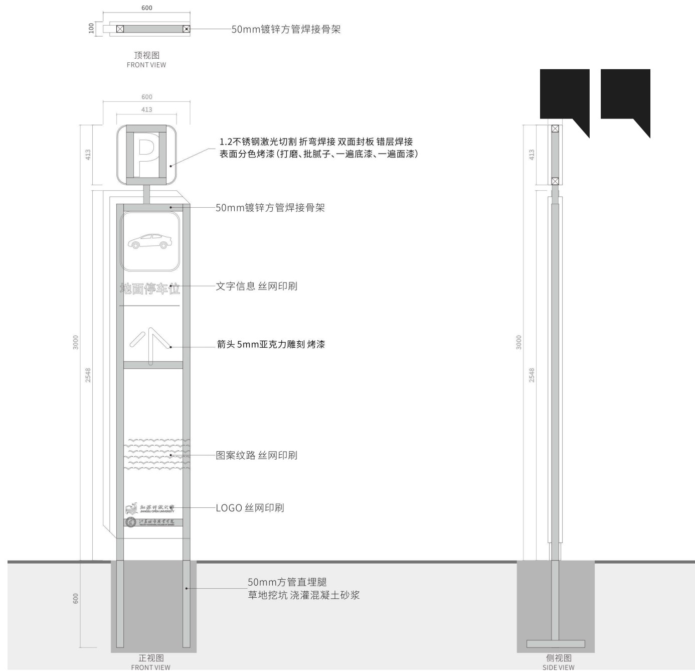
结构图
