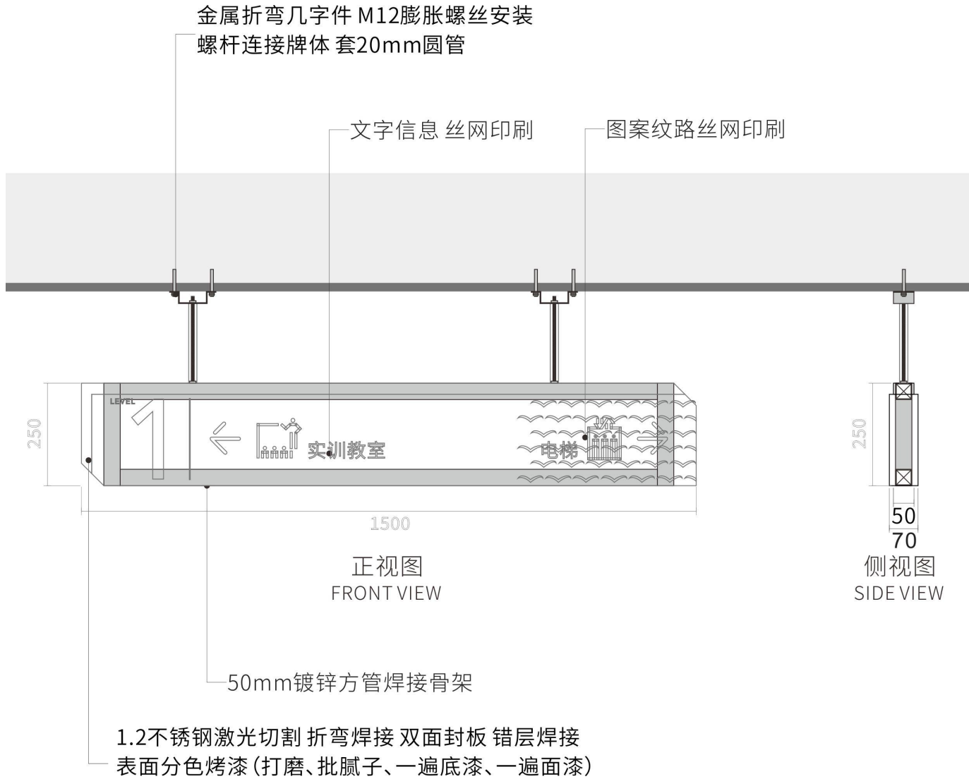
结构图
