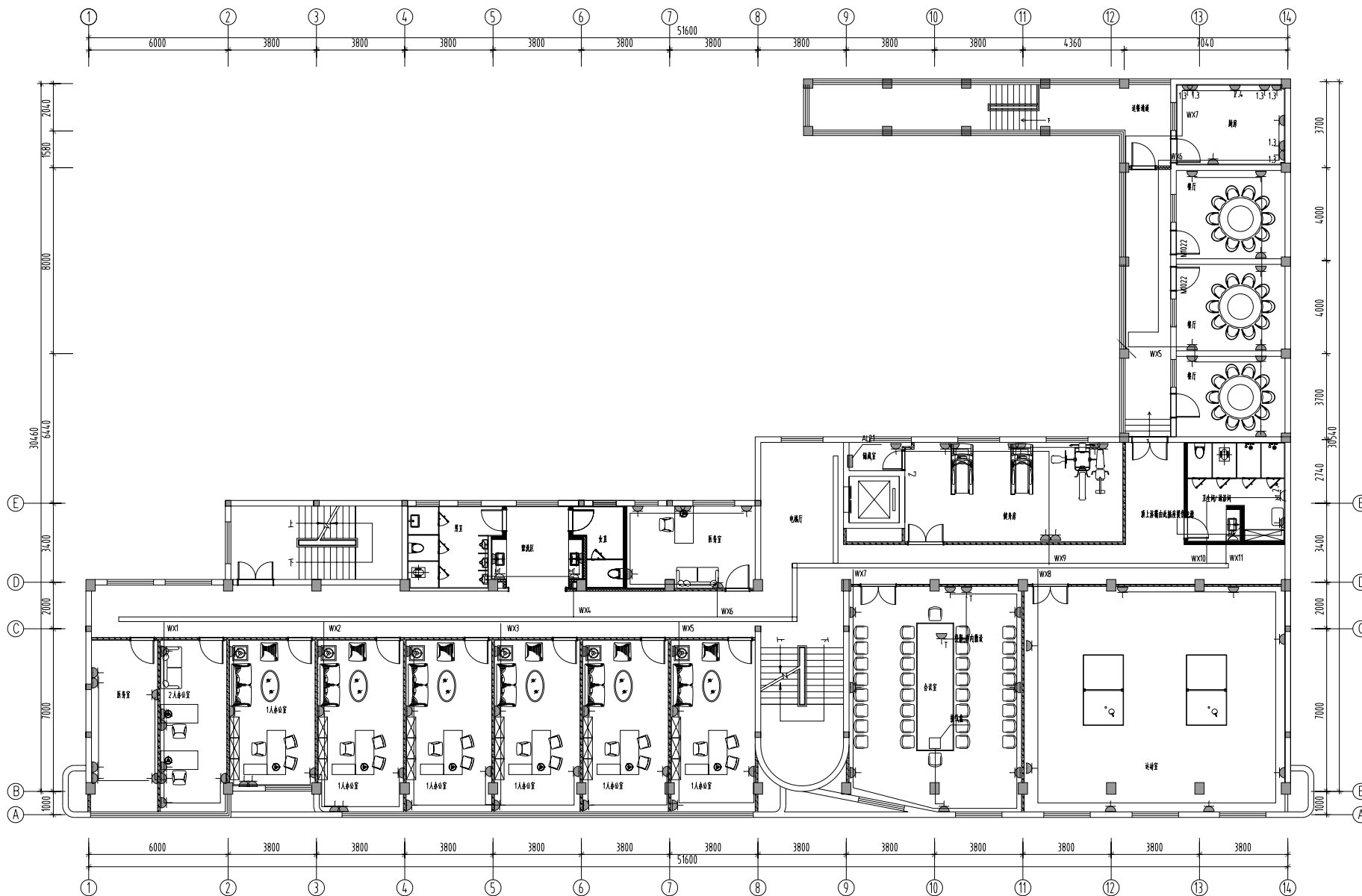
二层插座平面图
