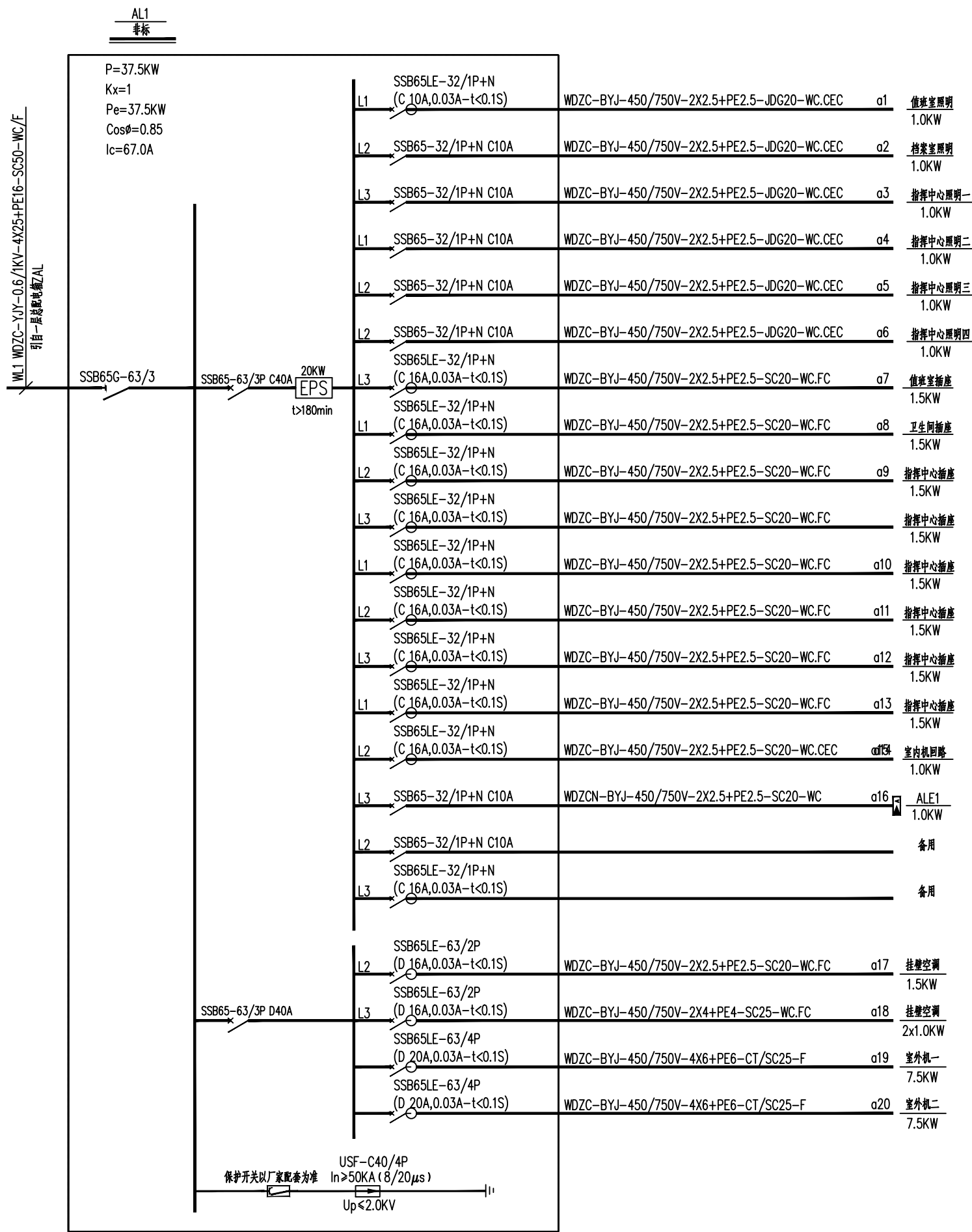
一层照明配电箱AL1 配电系统图
