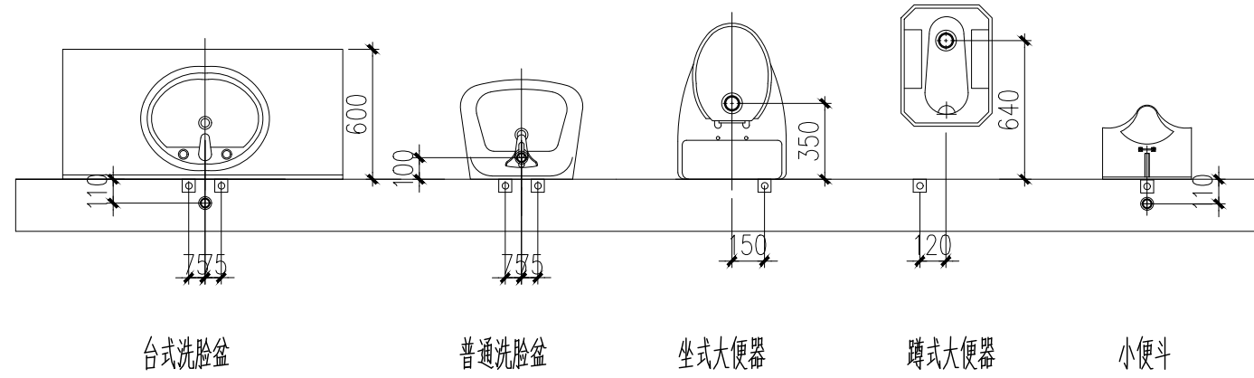
卫生设备楼板洞平面位置
