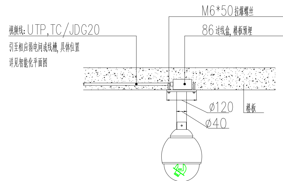
室内全球摄像机楼板安装大样图
