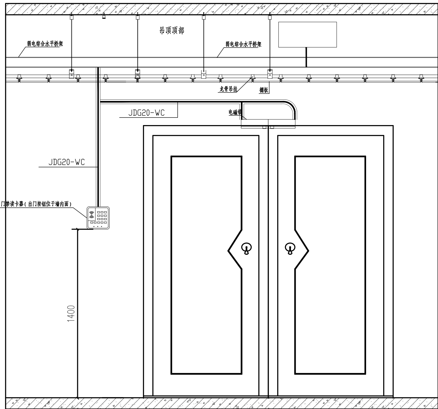
门禁安装大样图 (双门正面)
