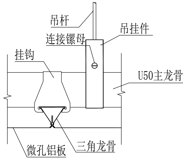
顶部龙骨接点图
