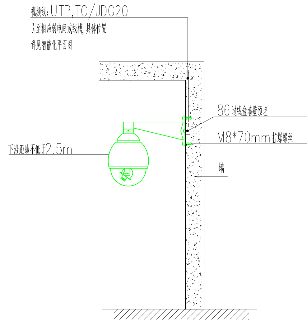
室内全球摄像机壁挂安装大样图
