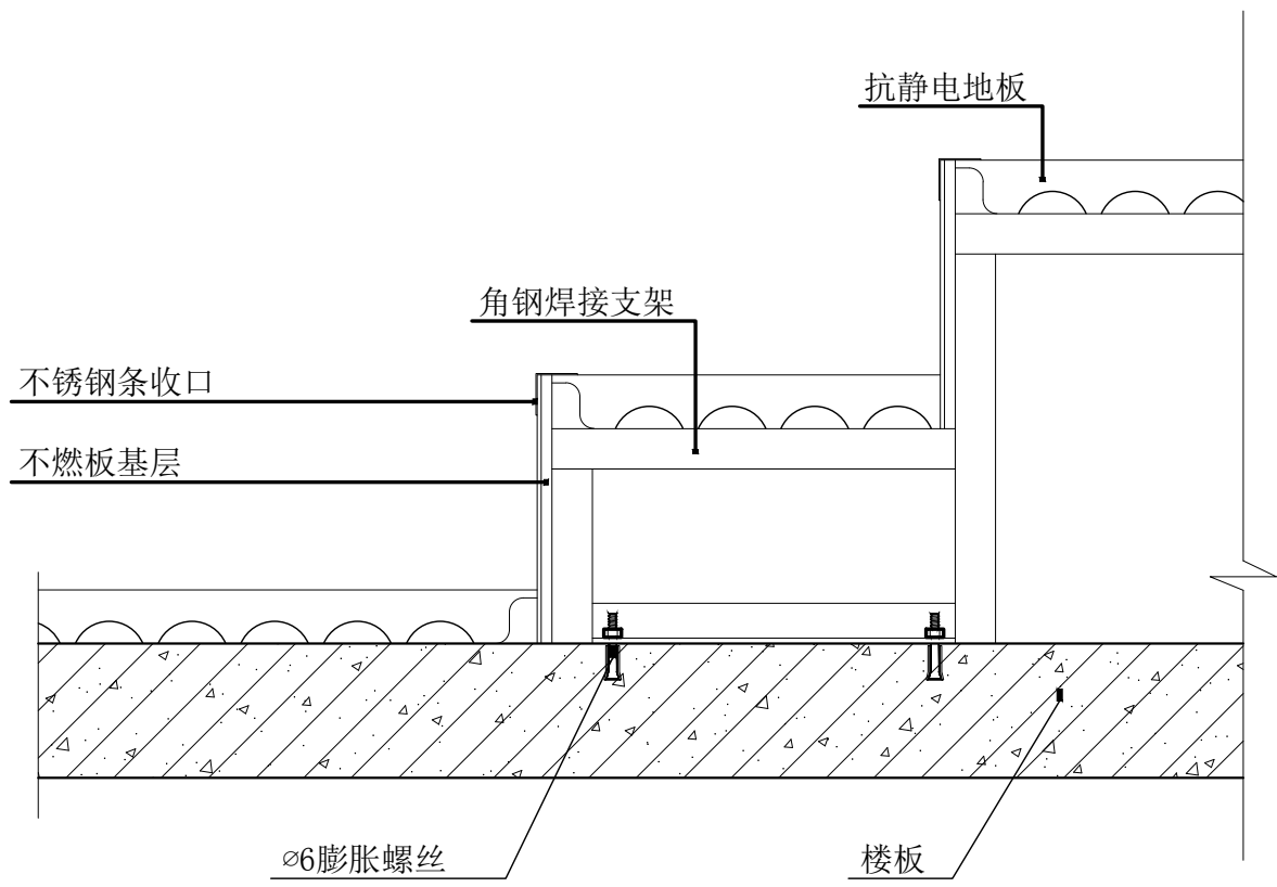
地板台阶剖面图
