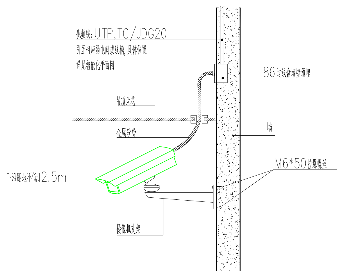
室内固定式摄像机壁挂安装大样图
