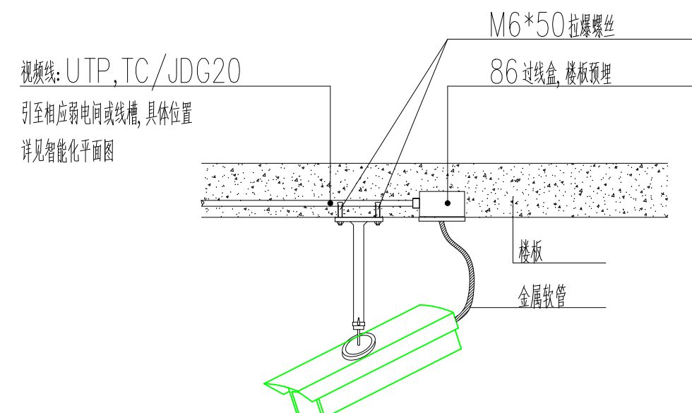
室内固定式摄像机楼板安装大样图
