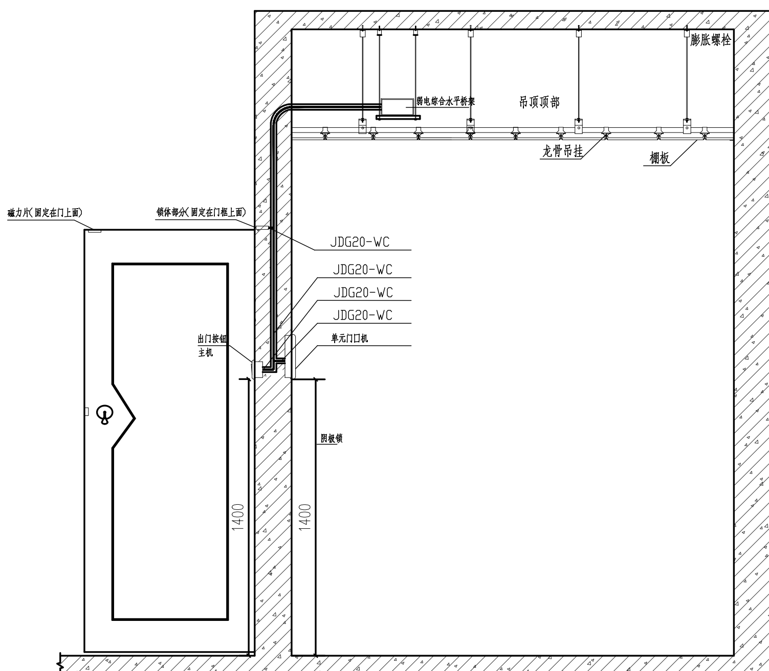
门禁安装大样图 (双门侧面)
