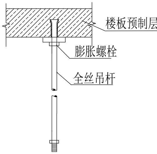
吊杆大样图
