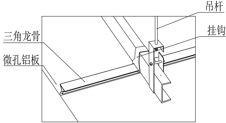
顶部龙骨接点透视图
