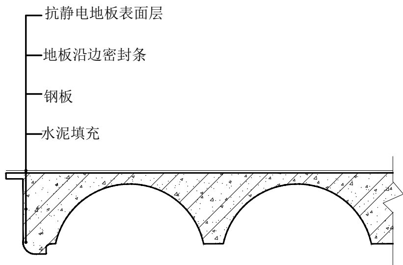
防静电地板剖面
