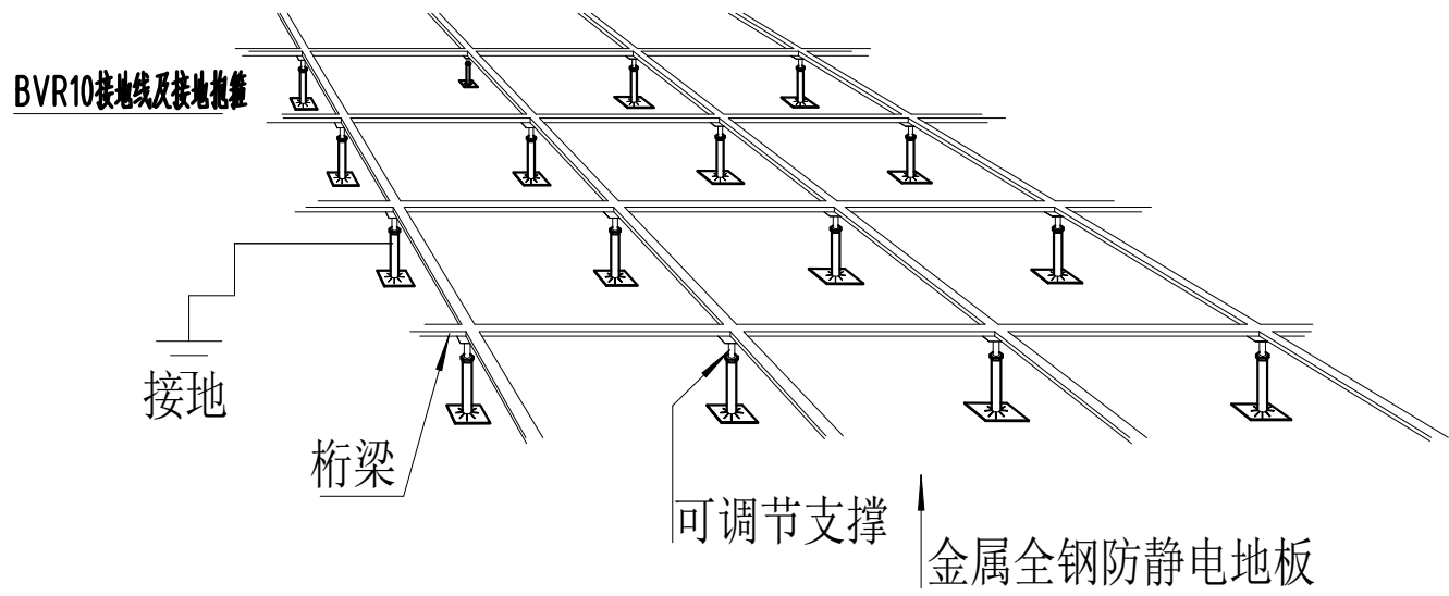
机房设备布局图
