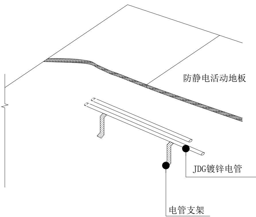
地板下走线剖面图
