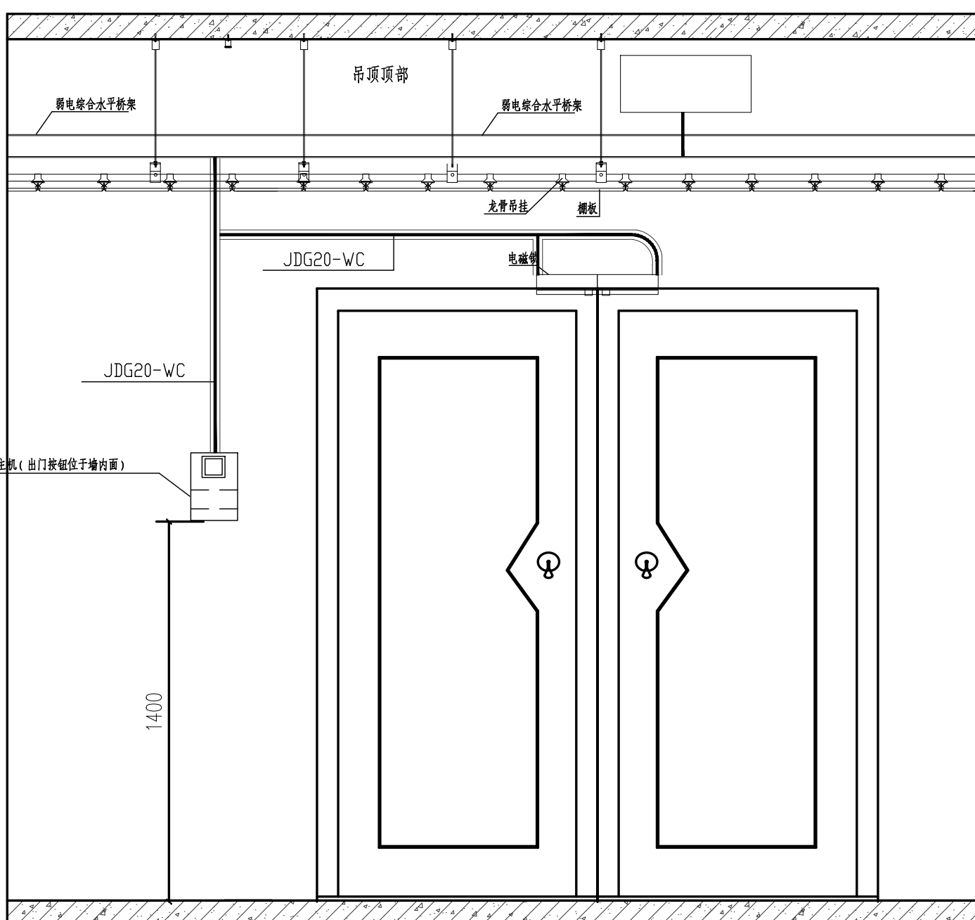
单元门口机安装大样图 (双门正面)
