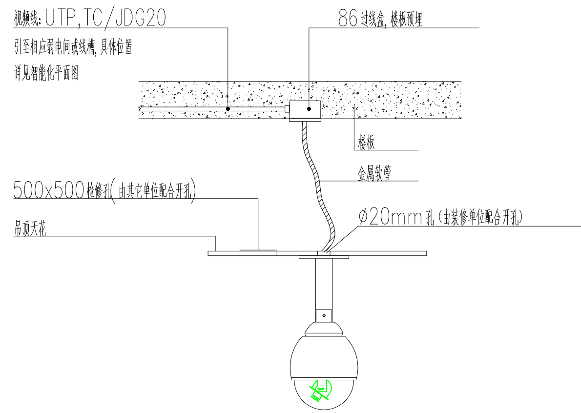
室内全球摄像机吊顶安装大样图
