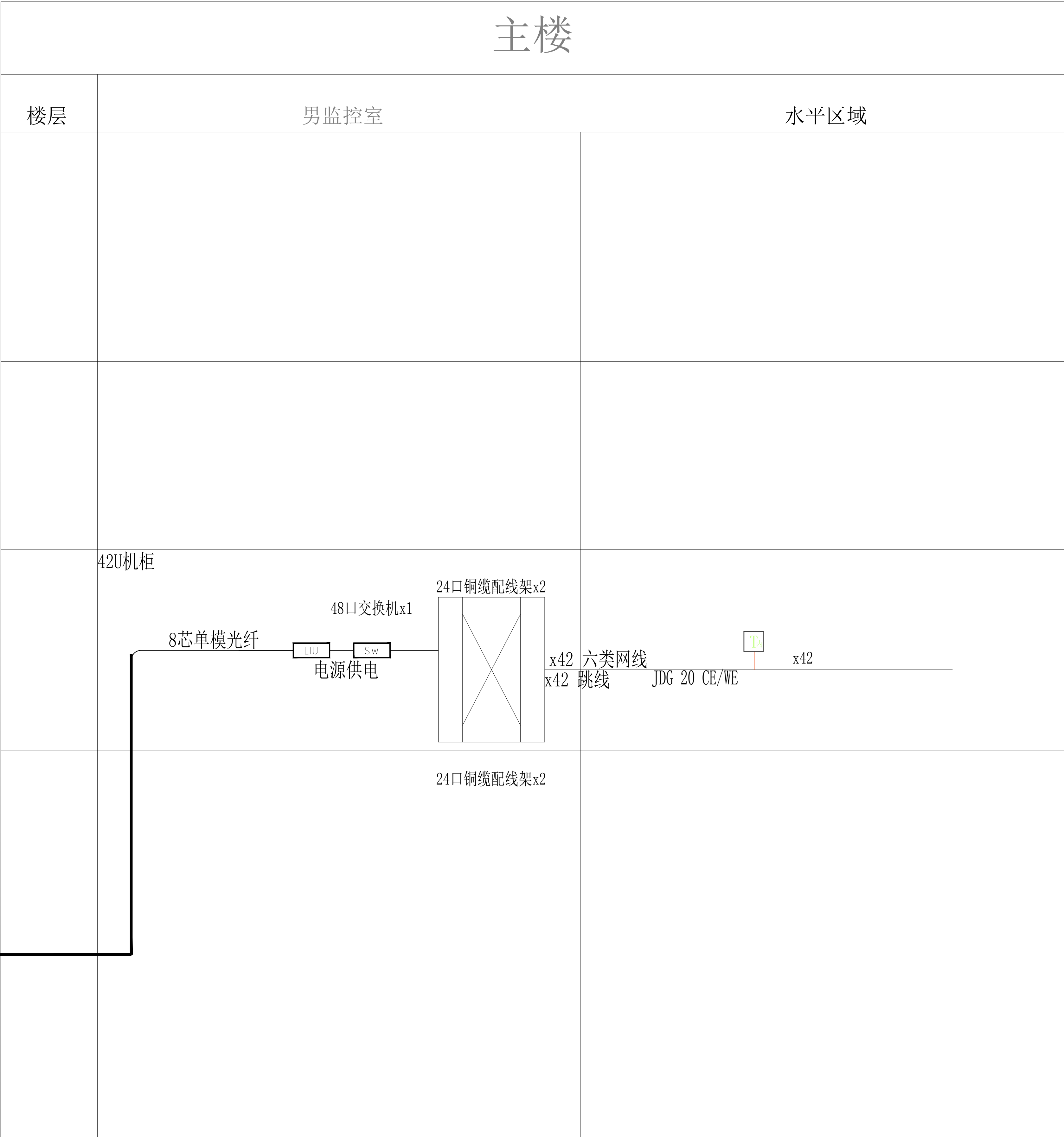
内网系统图
