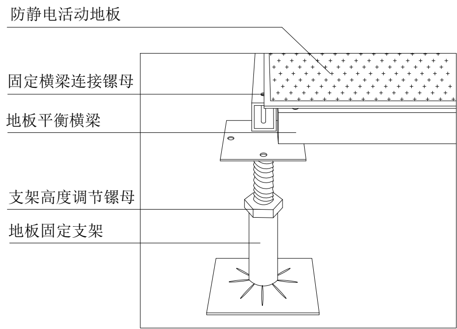
地板与支架透视图
