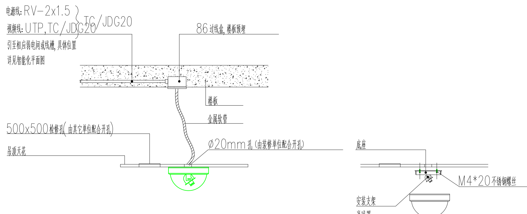
室内半球摄像机吊顶安装大样图
