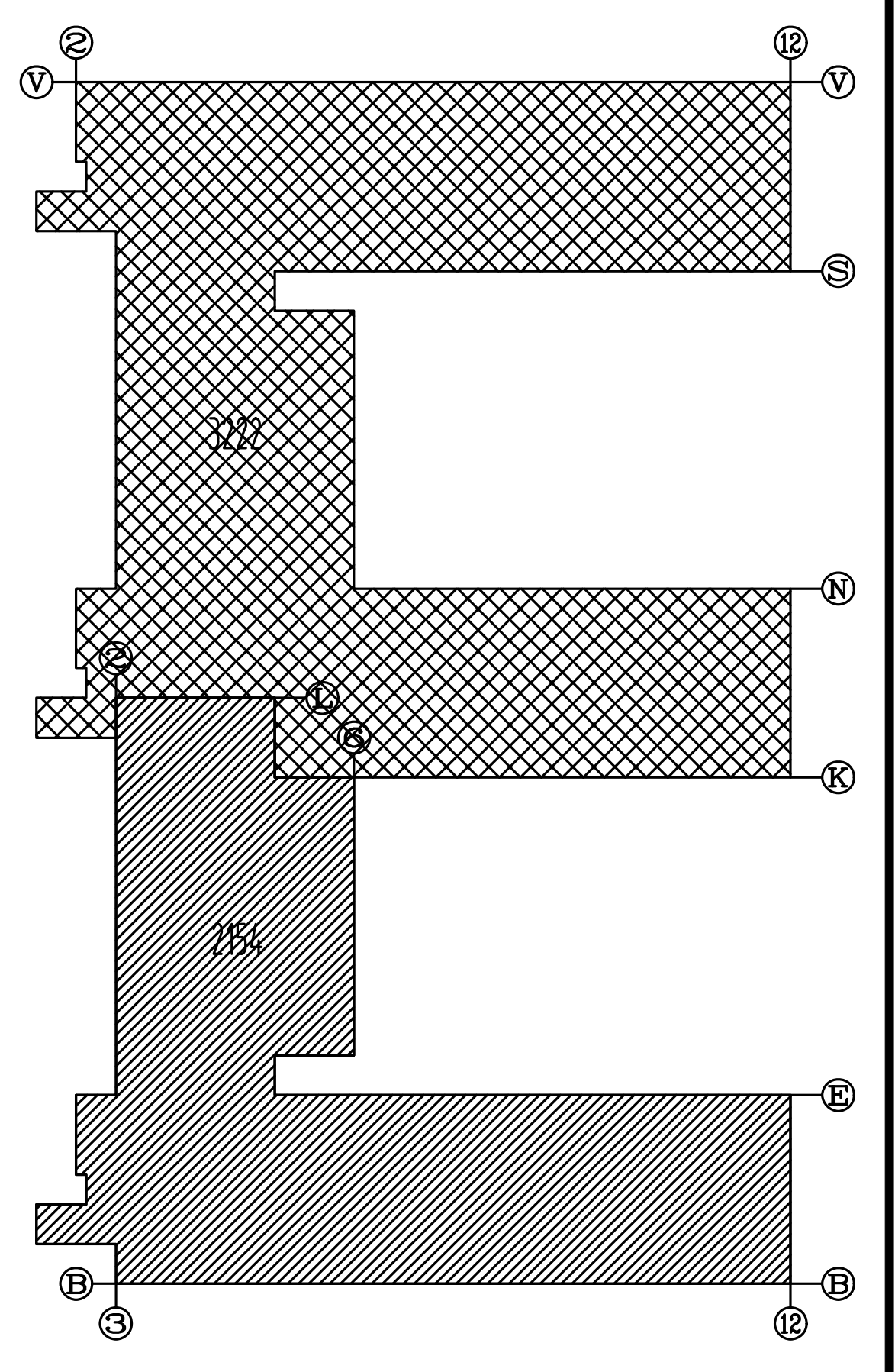
五层防火分区示意图
