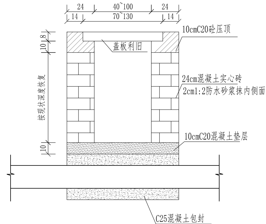
B-B剖面图
