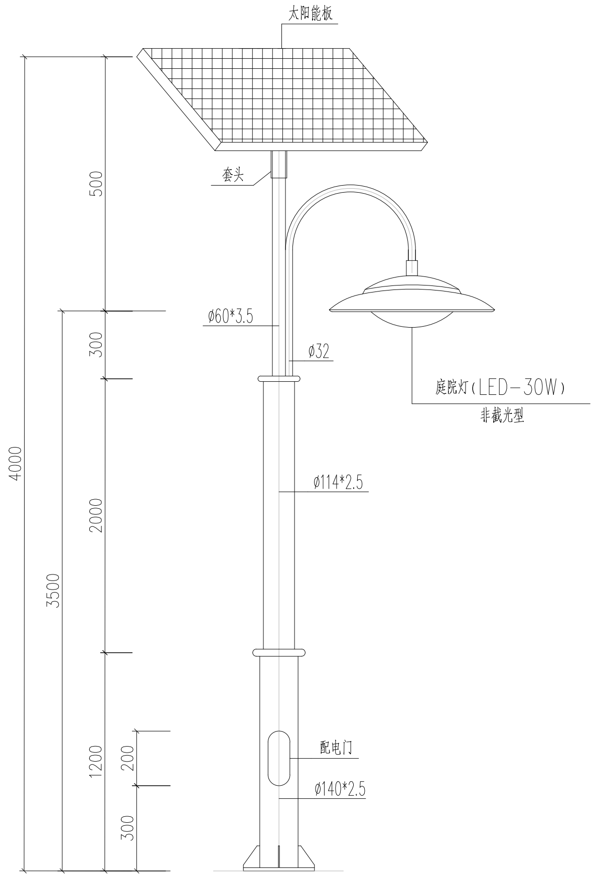
4m 太阳能庭院灯灯杆大样图
