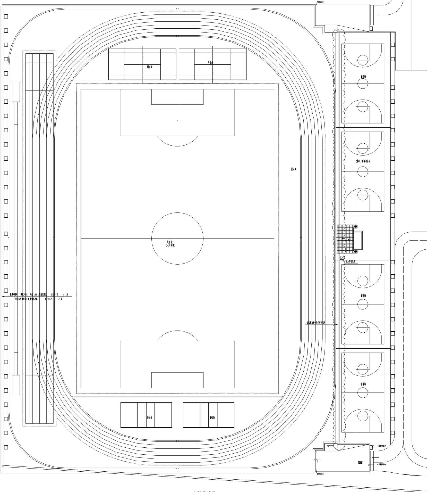
新建电缆沟平面图 1:250
