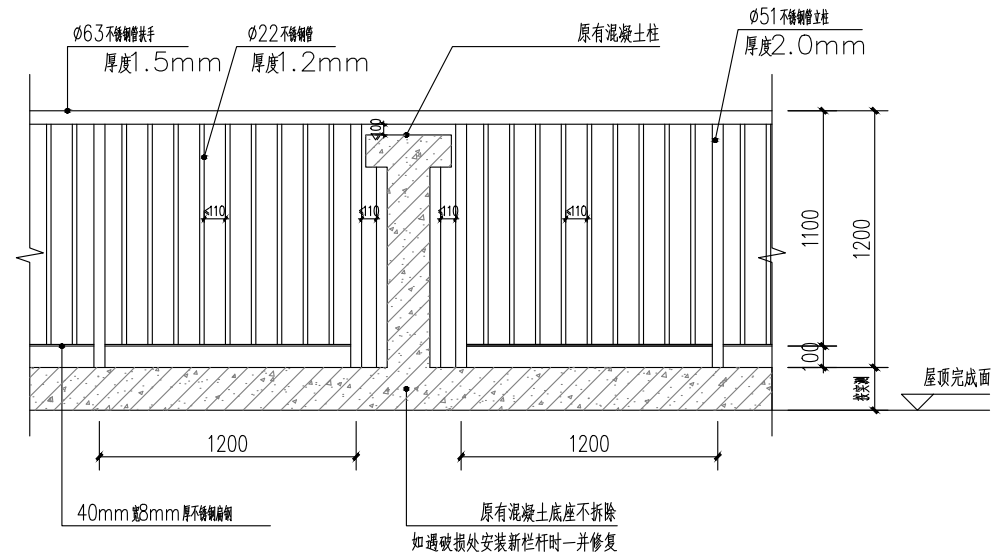
栏杆立面详图一 1:25
