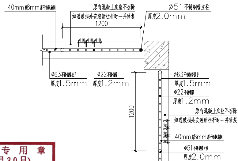
栏杆平面详图三 1:25
