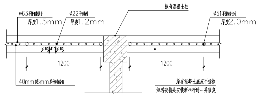
栏杆平面详图一 1:25
