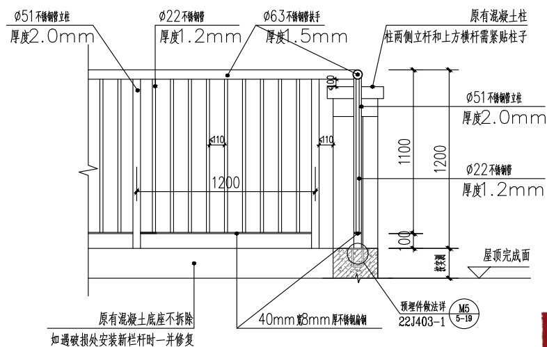
栏杆立面详图三 1:25
