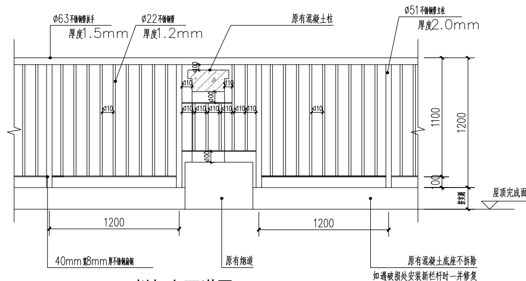
栏杆立面详图二 1:25
