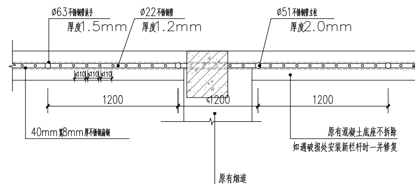
栏杆平面详图二 1:25
