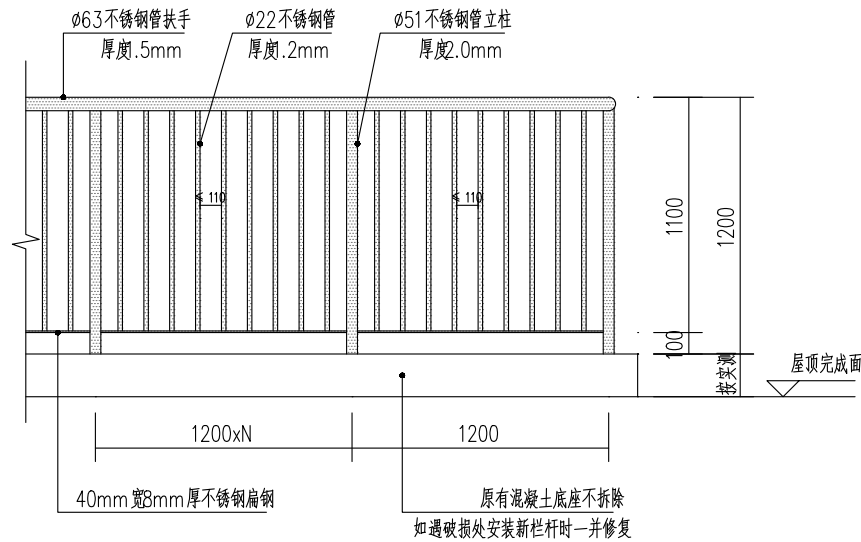
栏杆立面详图 1:25
