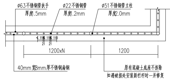
栏杆平面详图 1:25
