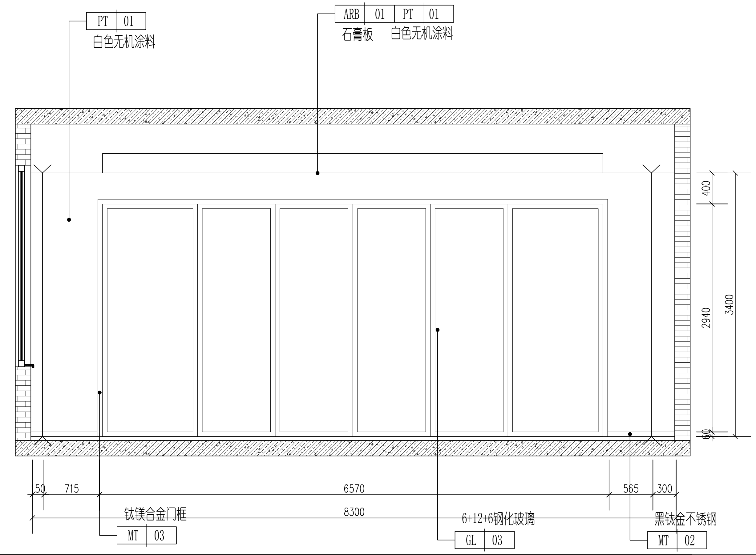
4 喷丝实验室D立面图 1:30
