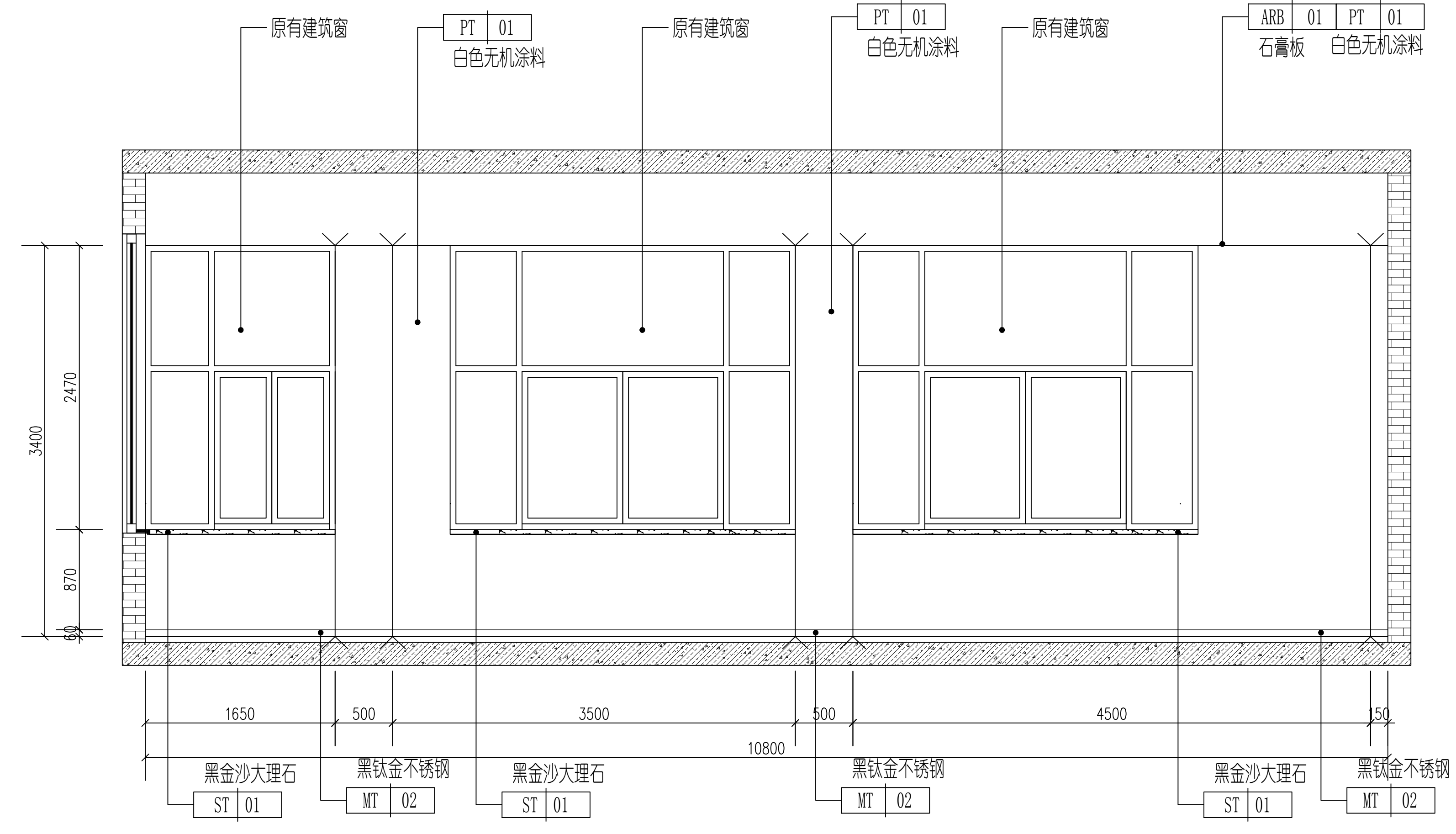
3 备用室C立面图 1:30
