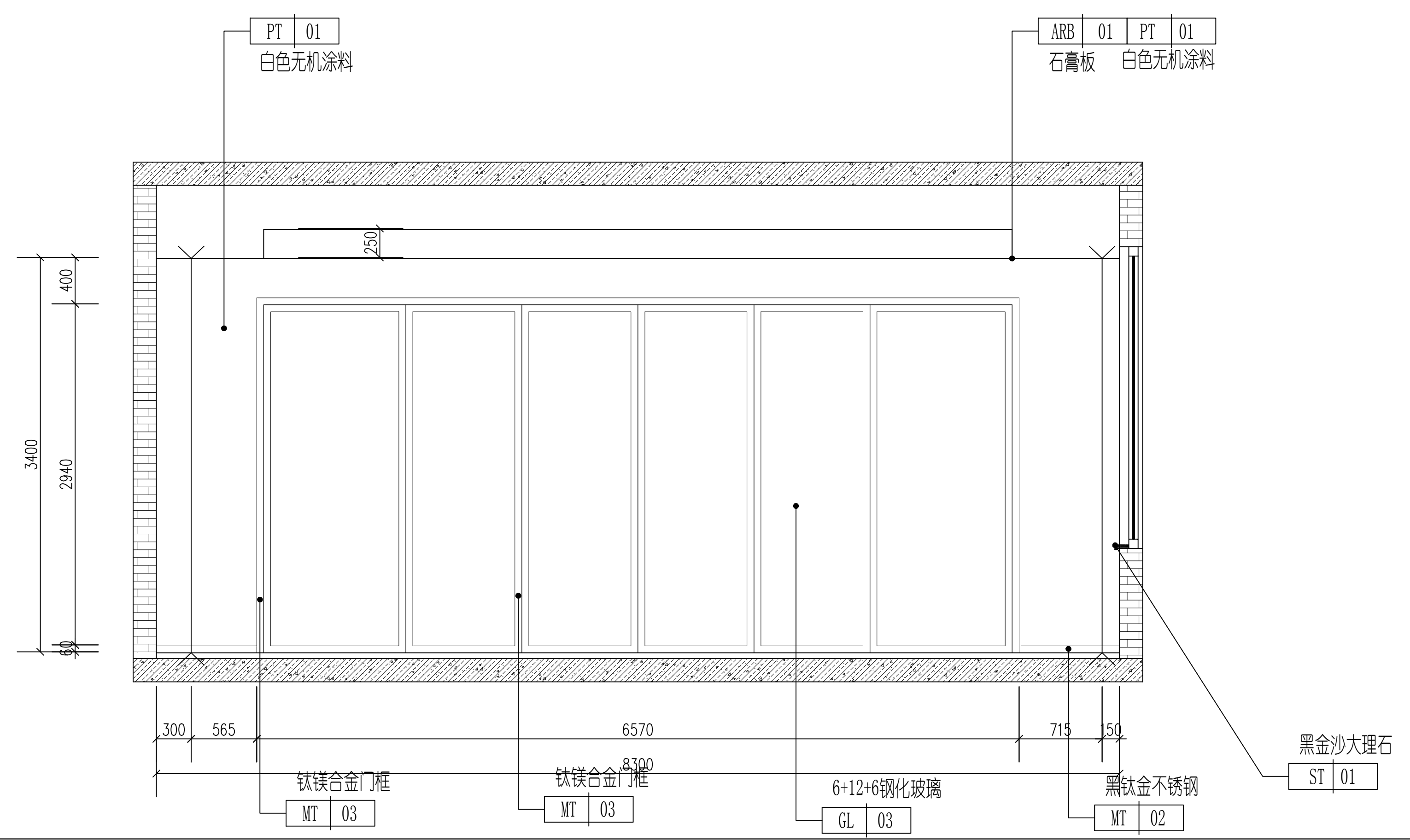
2 共混实验室B立面图 1:30
