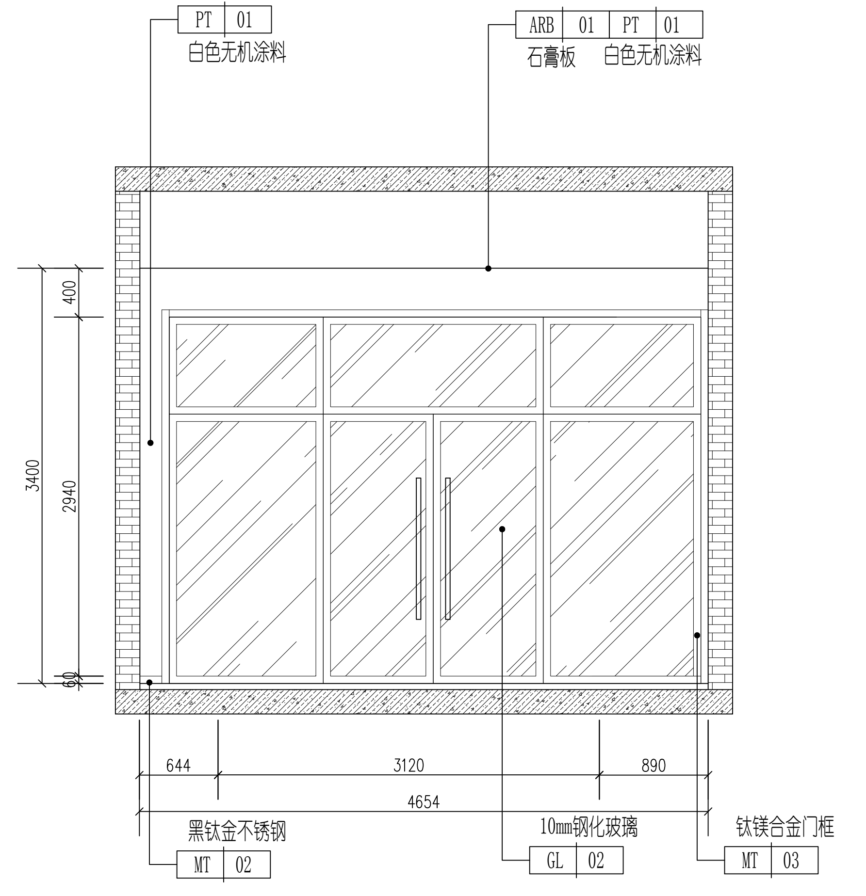
3 南门厅B立面图 1:30
