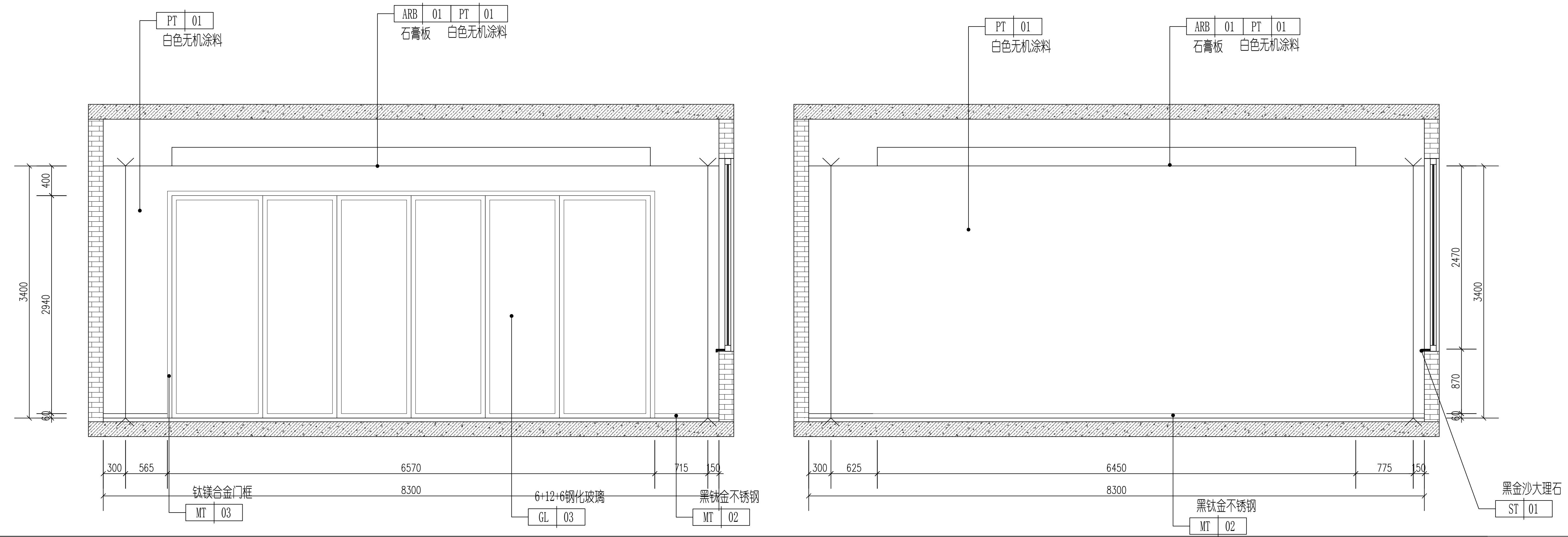
4 检测实验室D立面图 1:30
