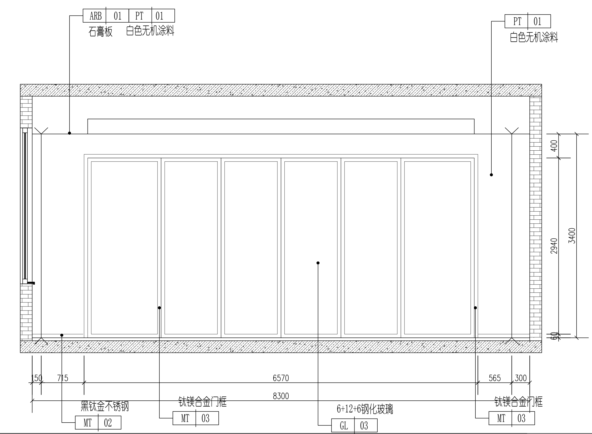
4 拉膜实验室D立面图 1:30
