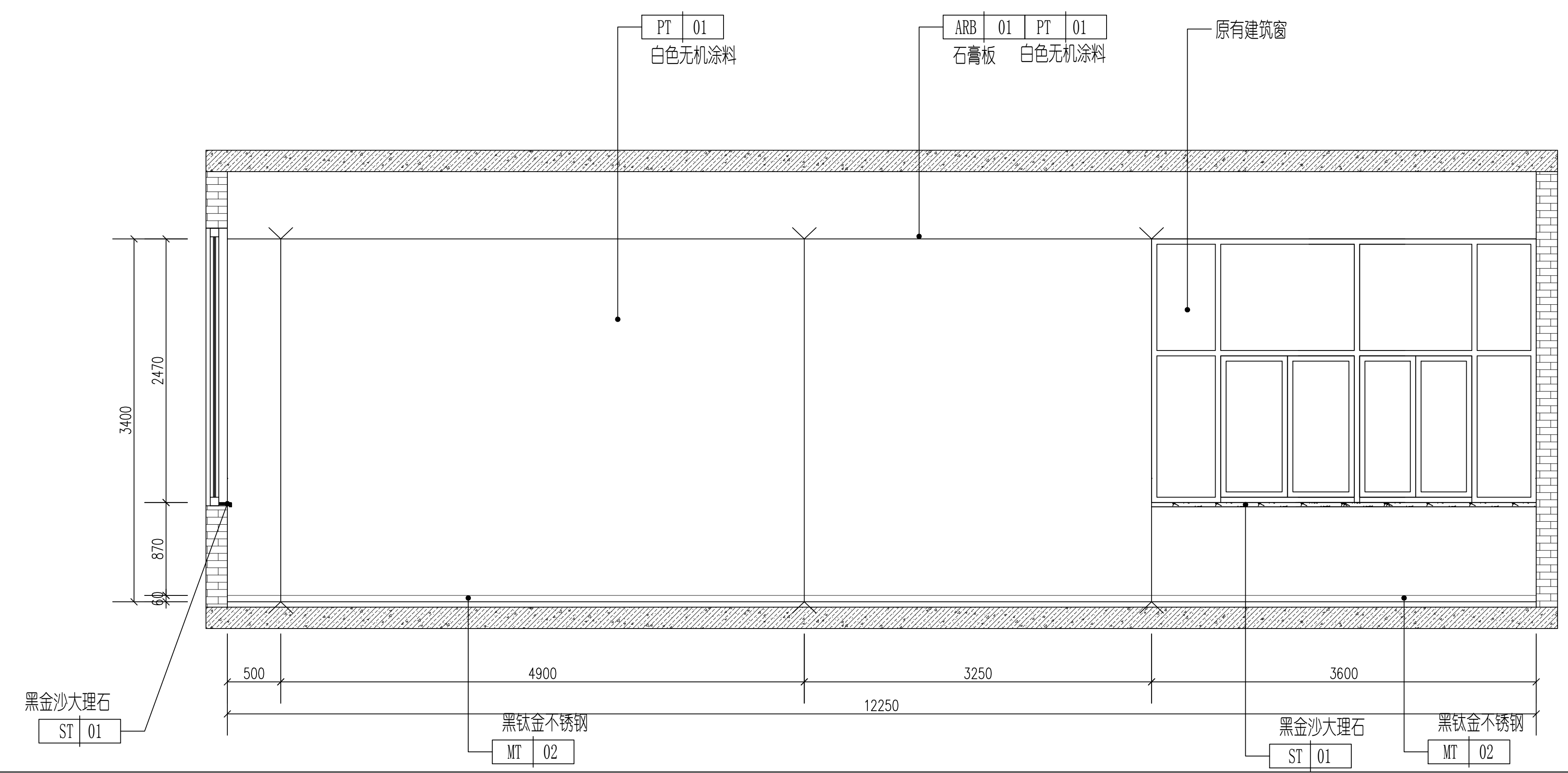
2 高分子材料展厅B立面图 1:30
