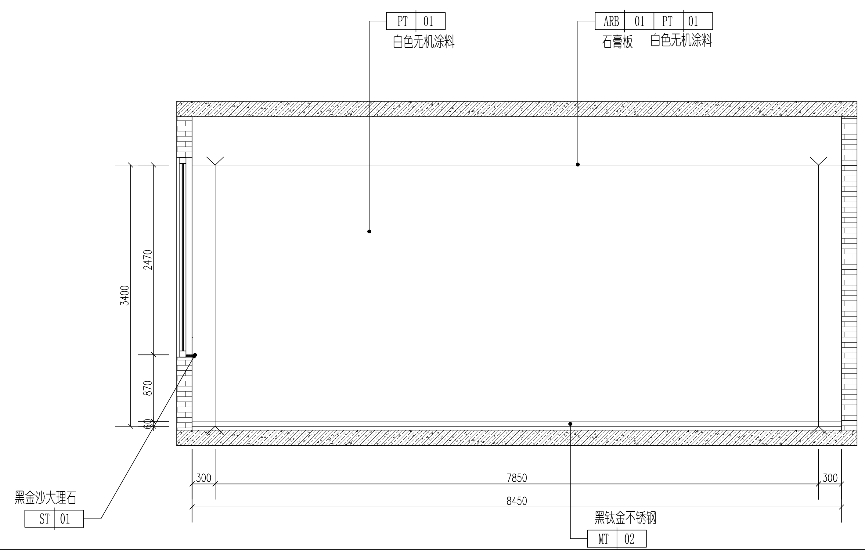
4 仓库D立面图 1:30
