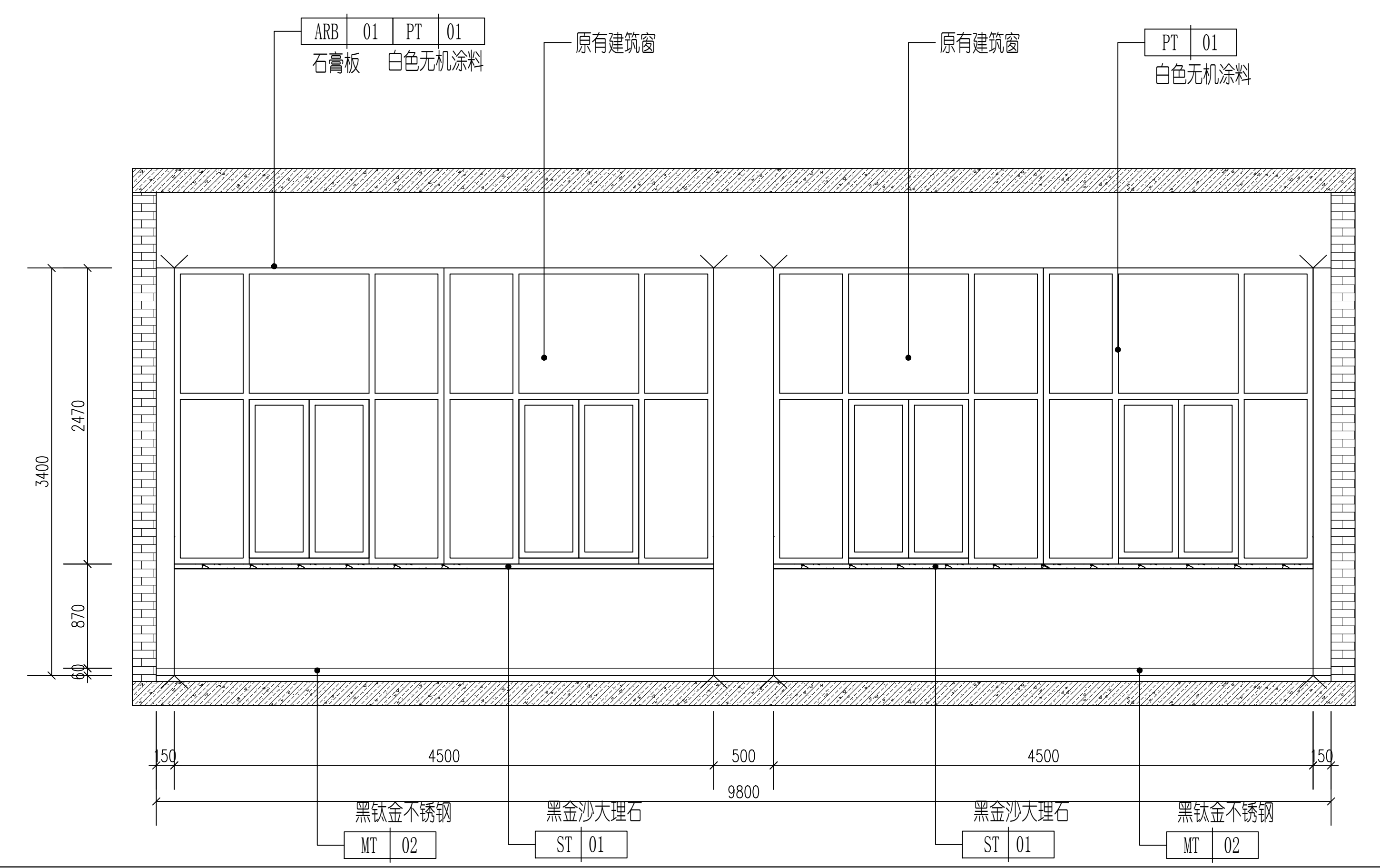
3 拉膜实验室C立面图 1:30
