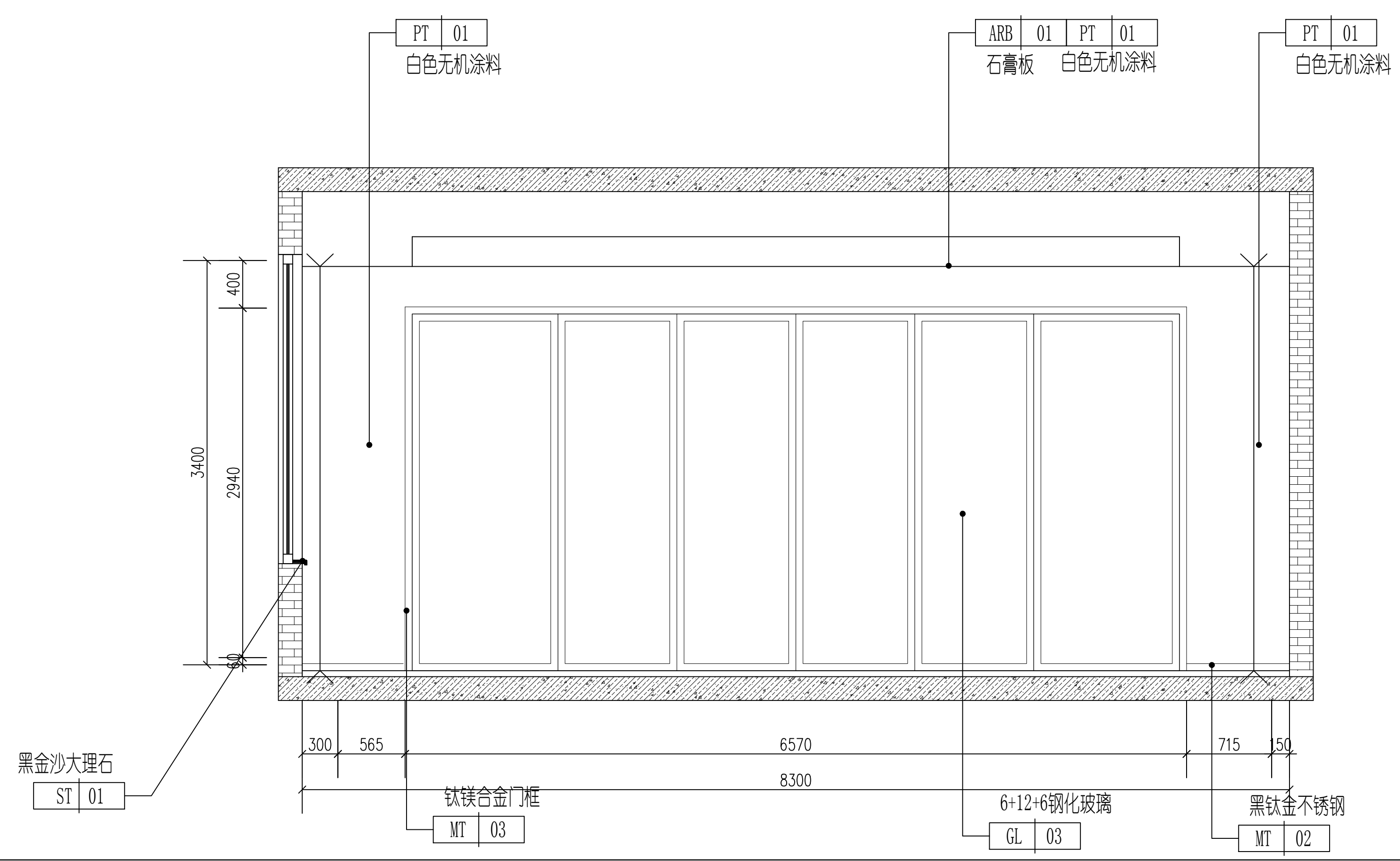
4 注塑实验室D立面图 1:30
