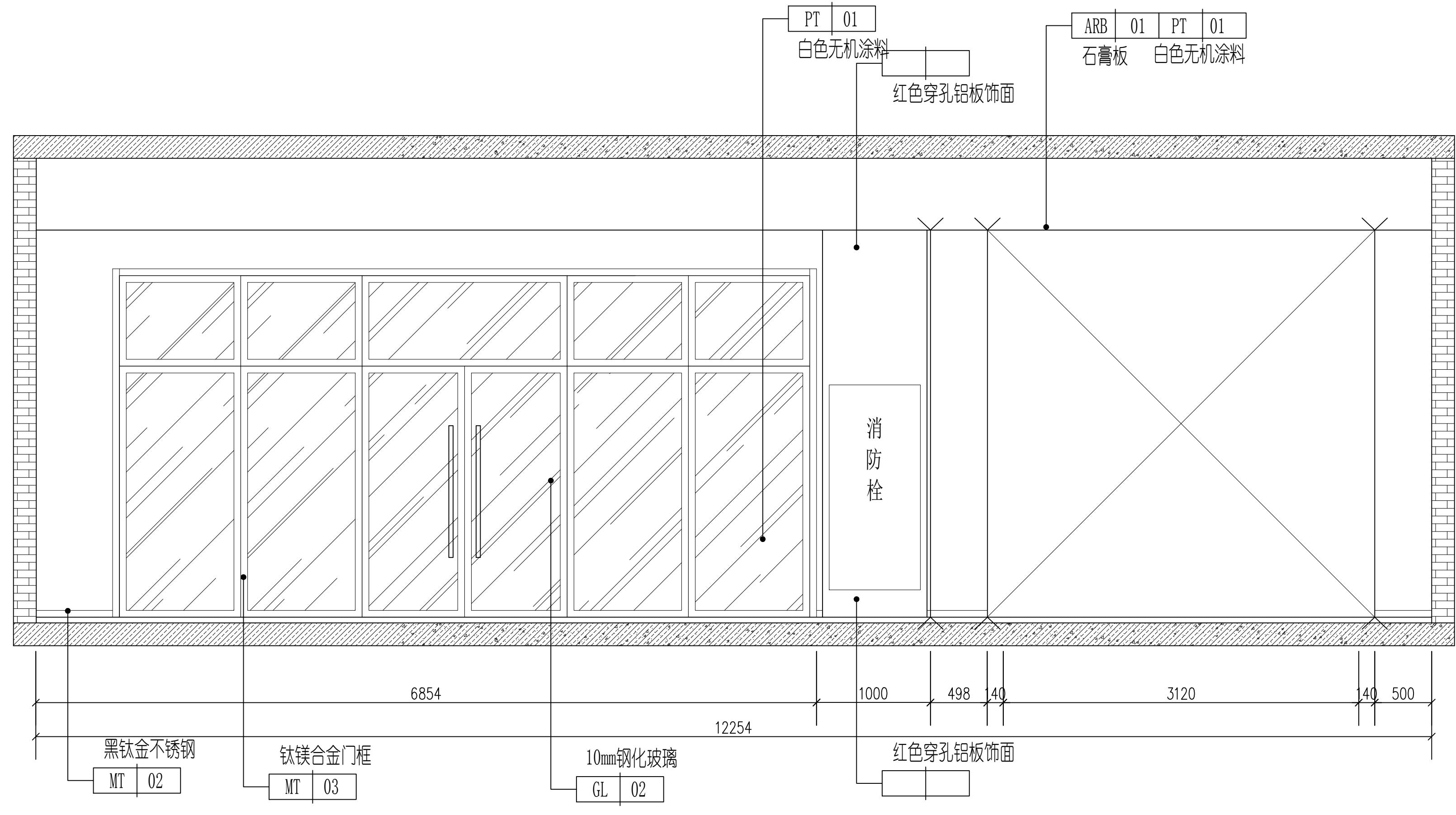
3 过道2B/D立面图 1:30
