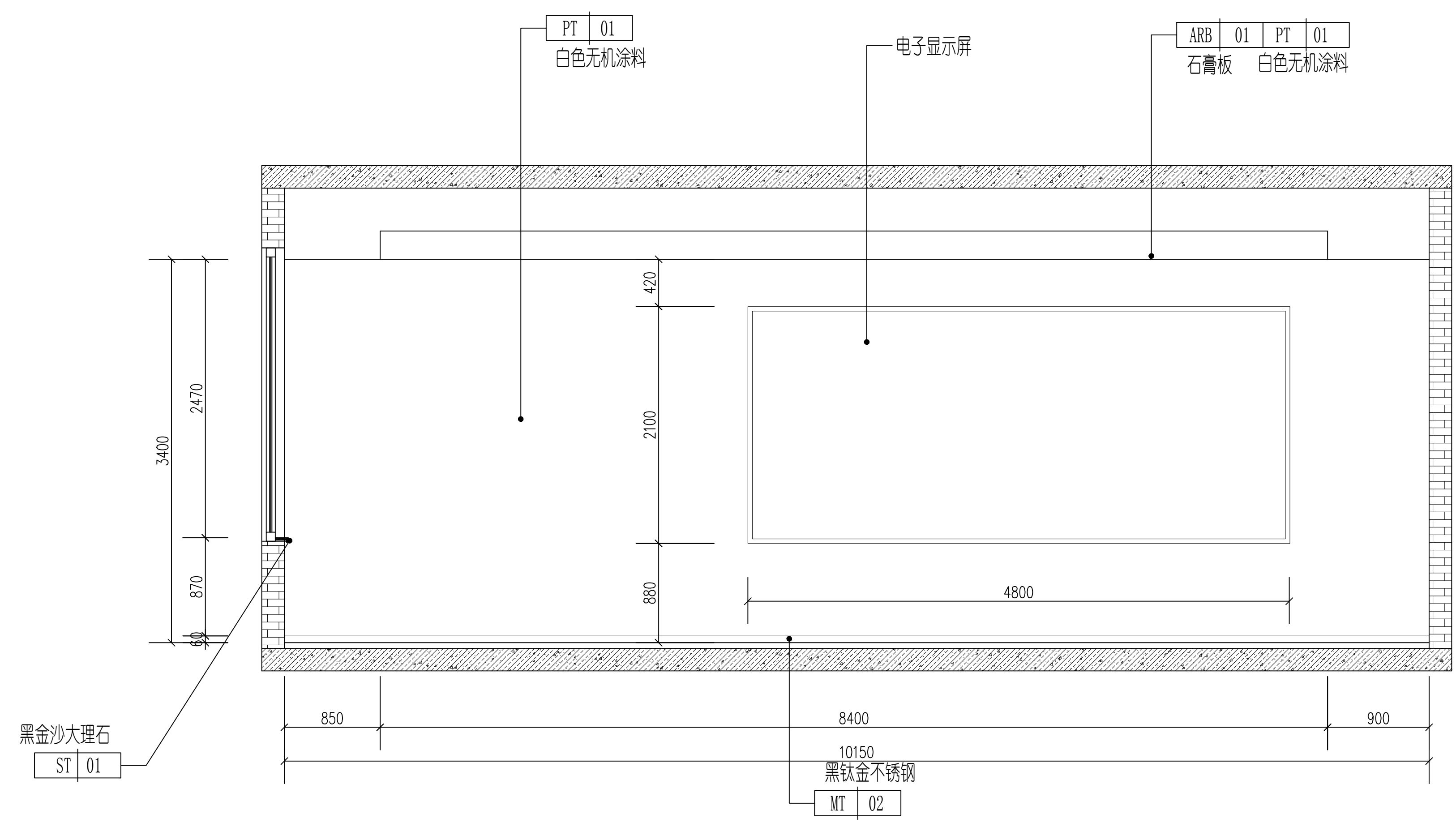
4 合成室D立面图 1:30
