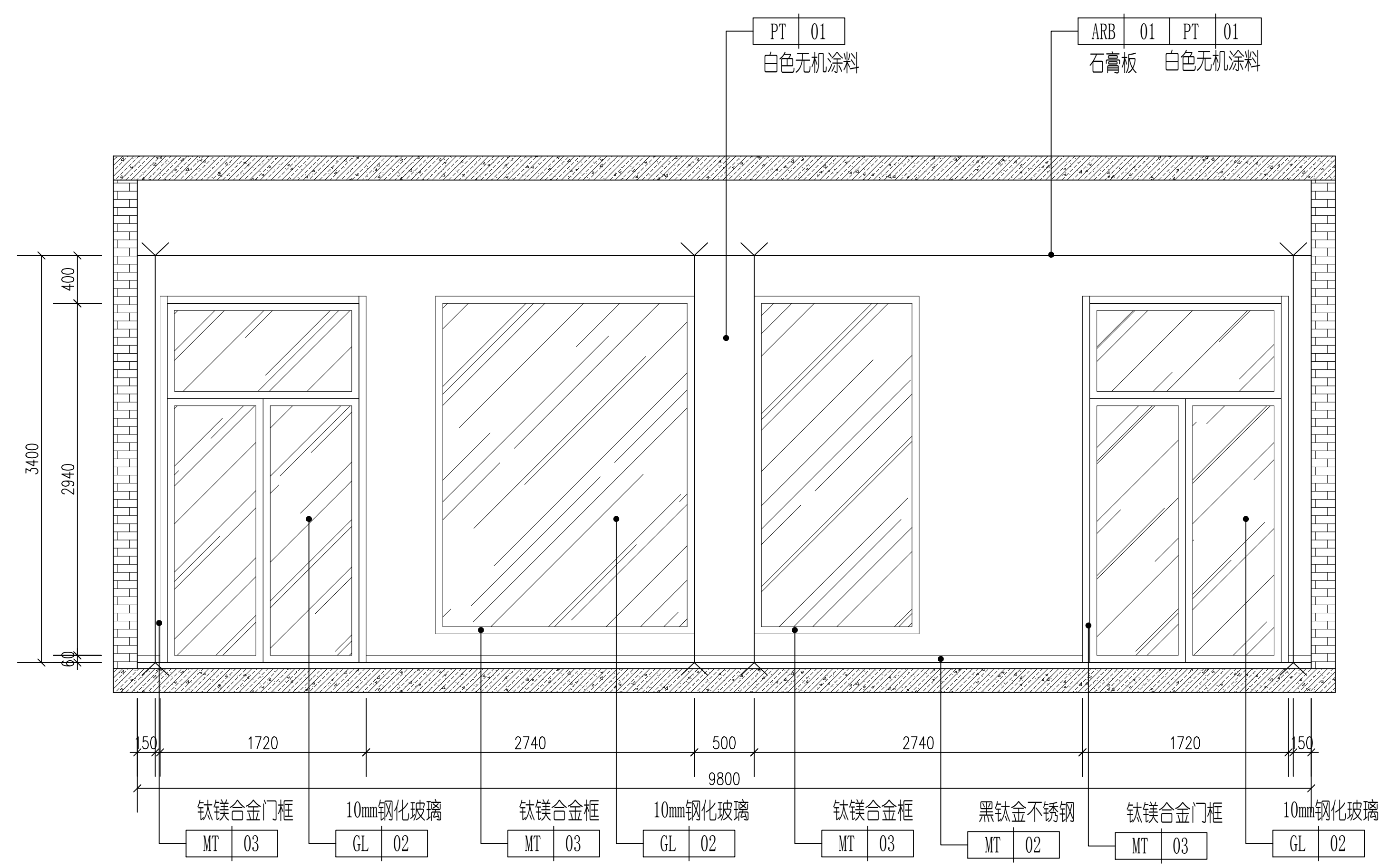
1 喷丝实验室A立面图 1:30
