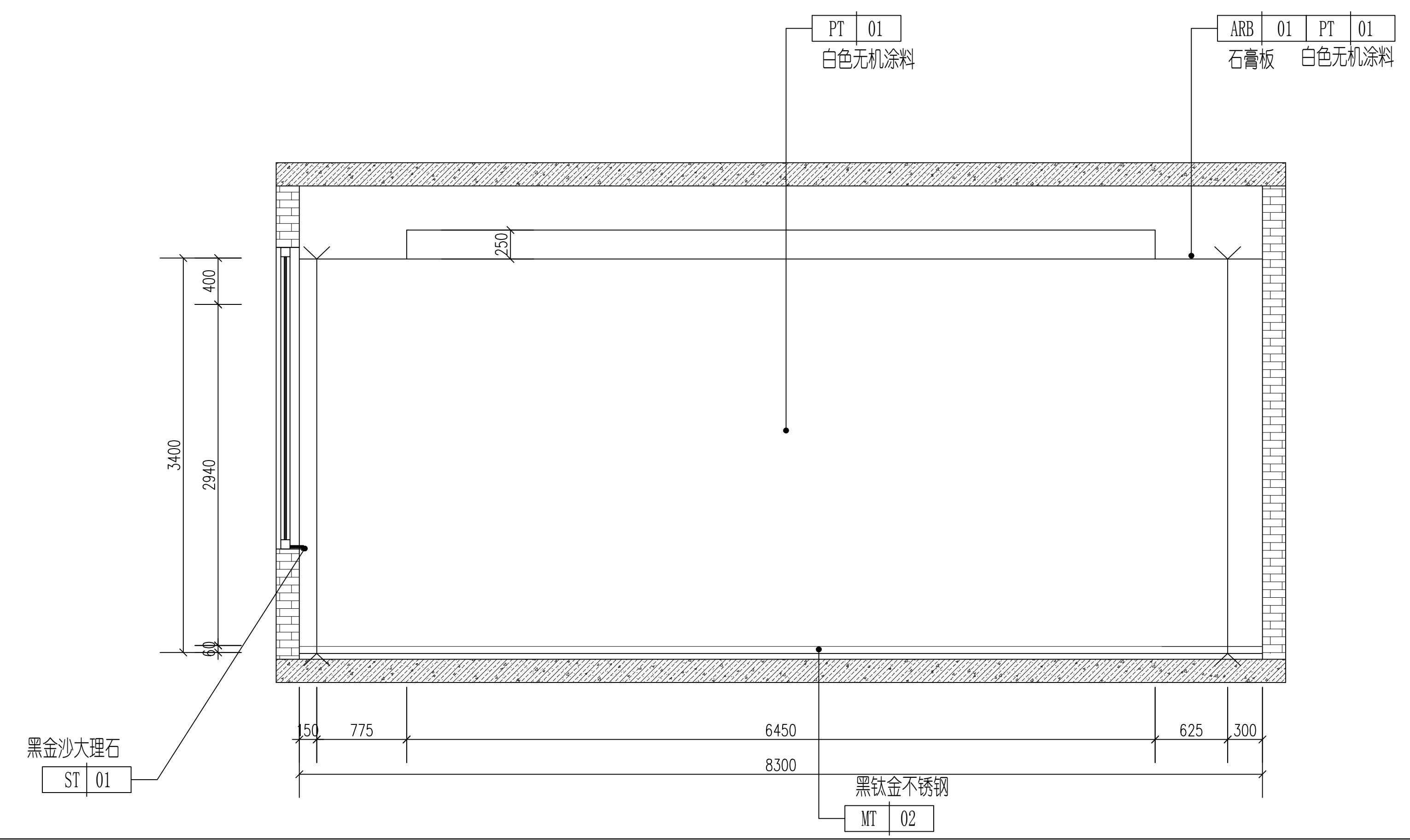
4 共混实验室D立面图 1:30
