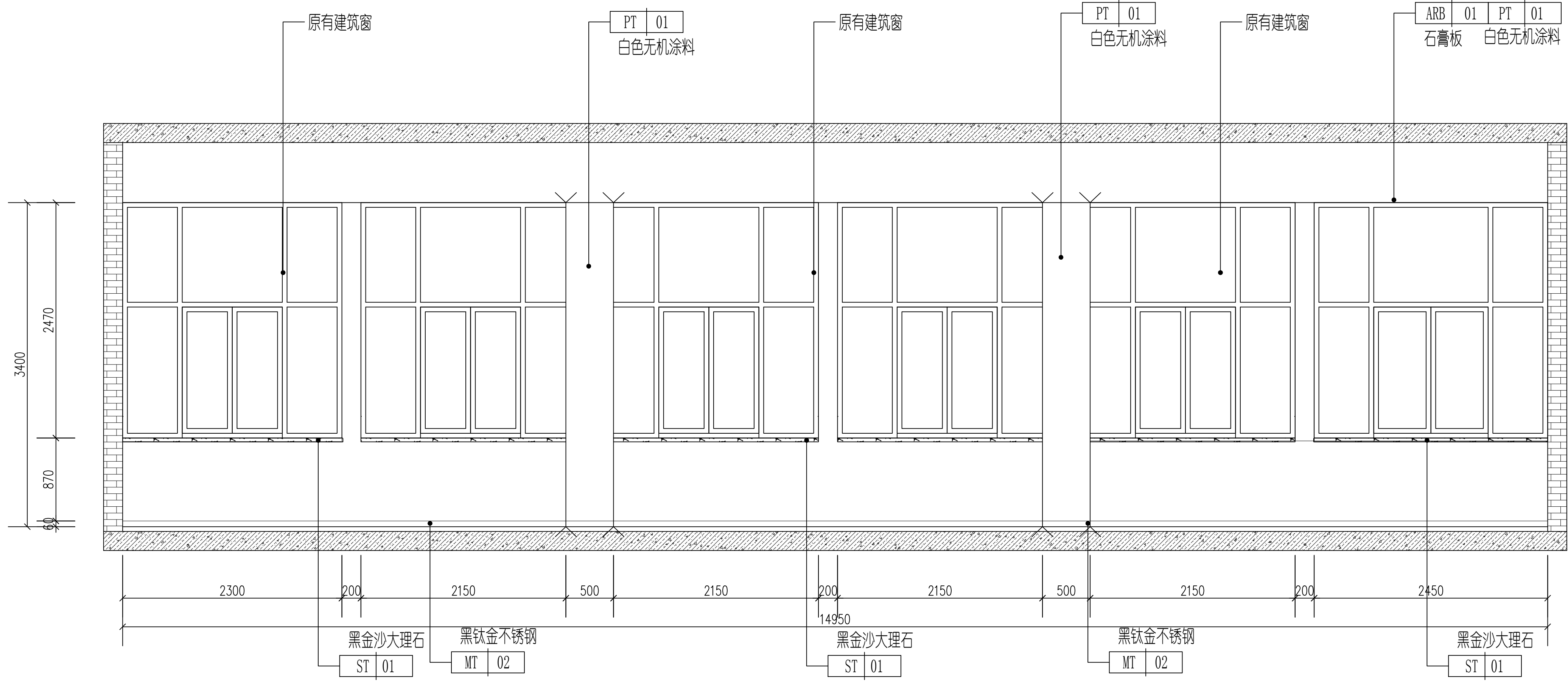
3 合成室C立面图 1:30
