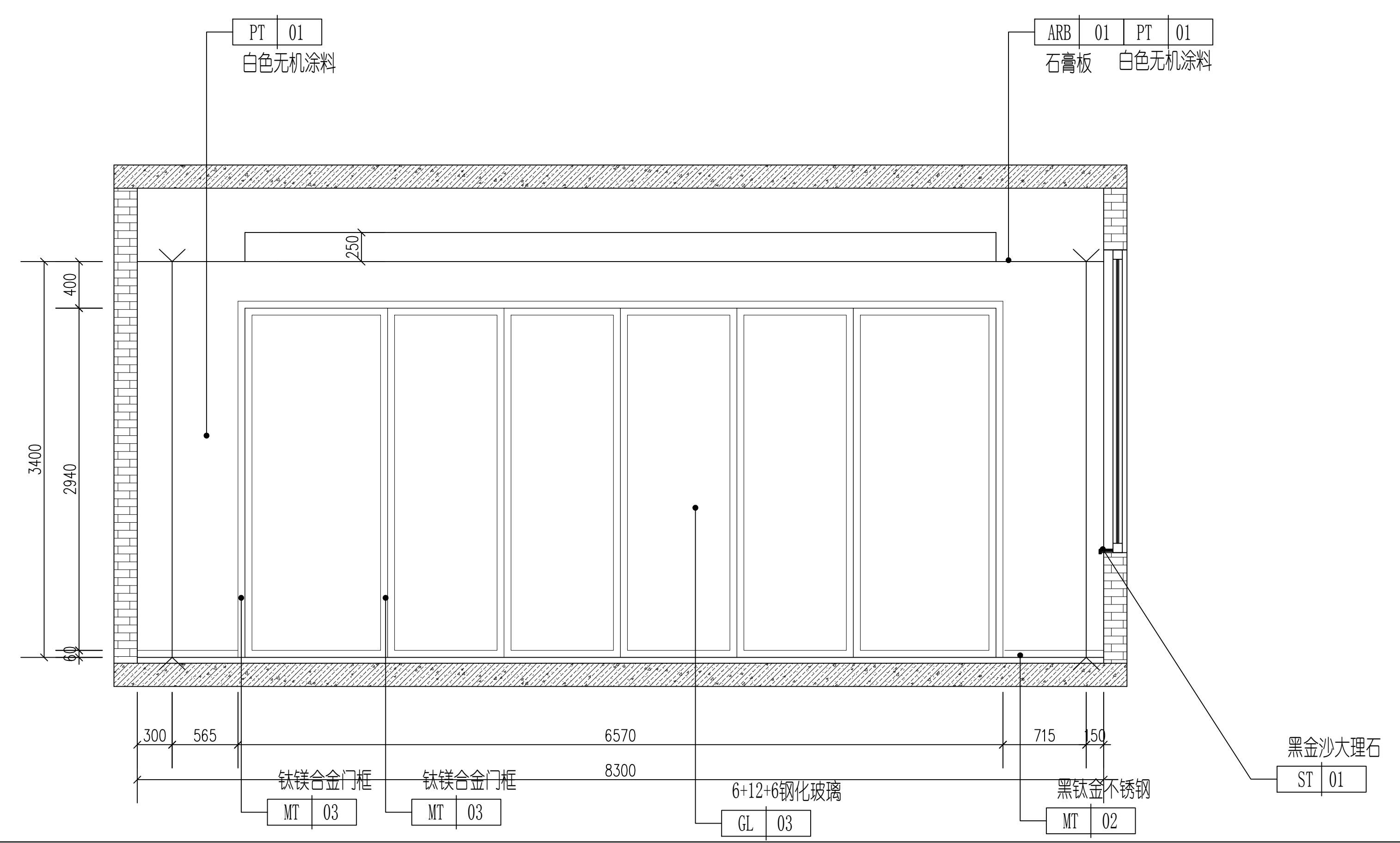
2 注塑实验室B立面图 1:30
