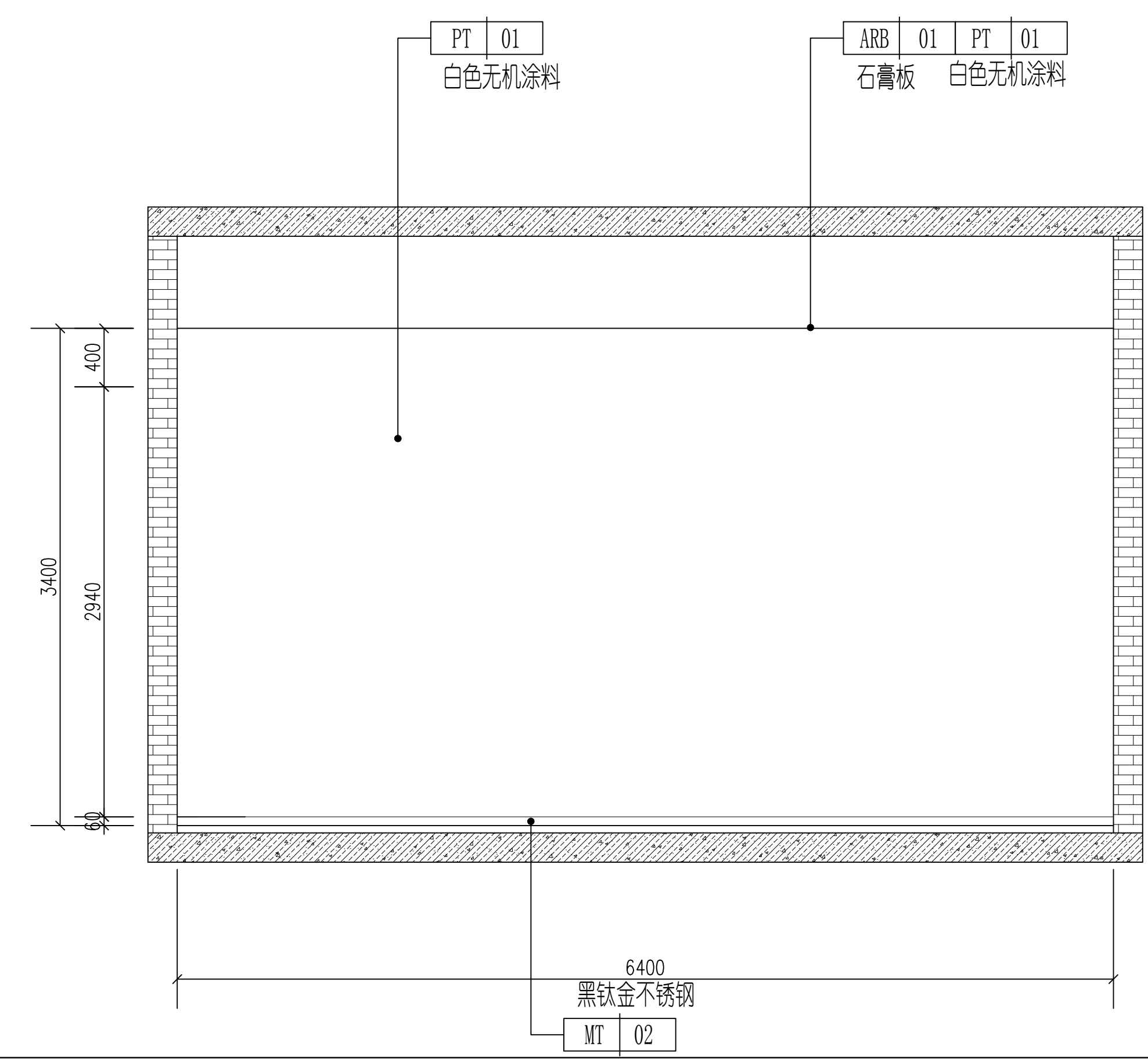
2 北门厅B立面图 1:30
