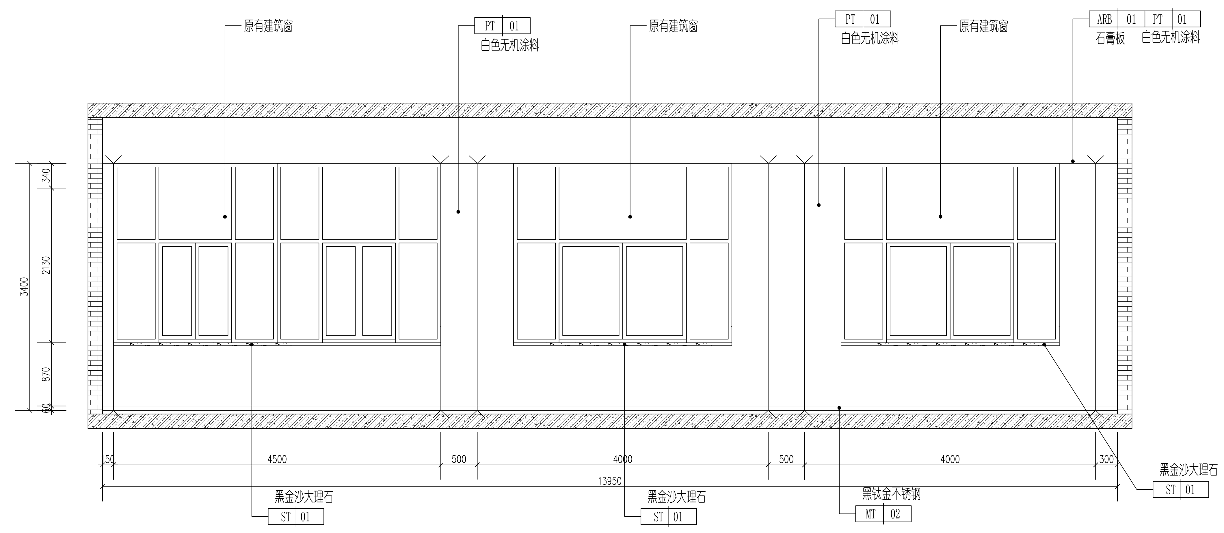
3 共混实验室C立面图 1:30
