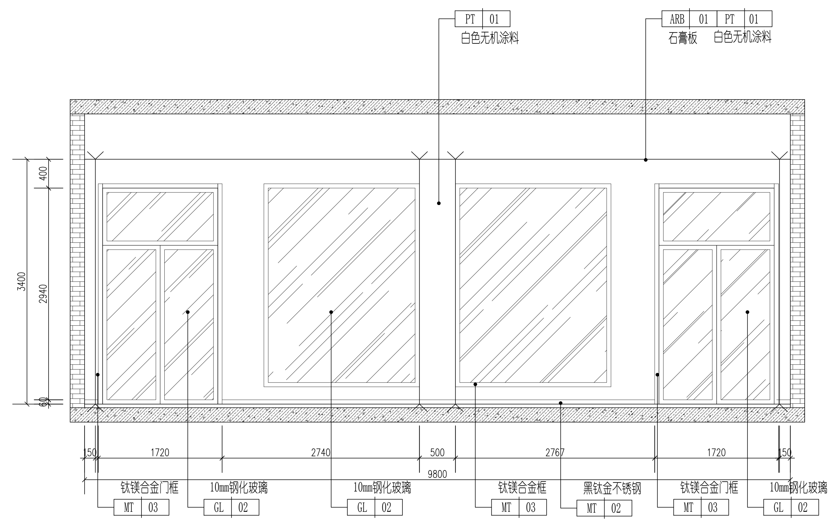
1 拉膜实验室A立面图 1:30
