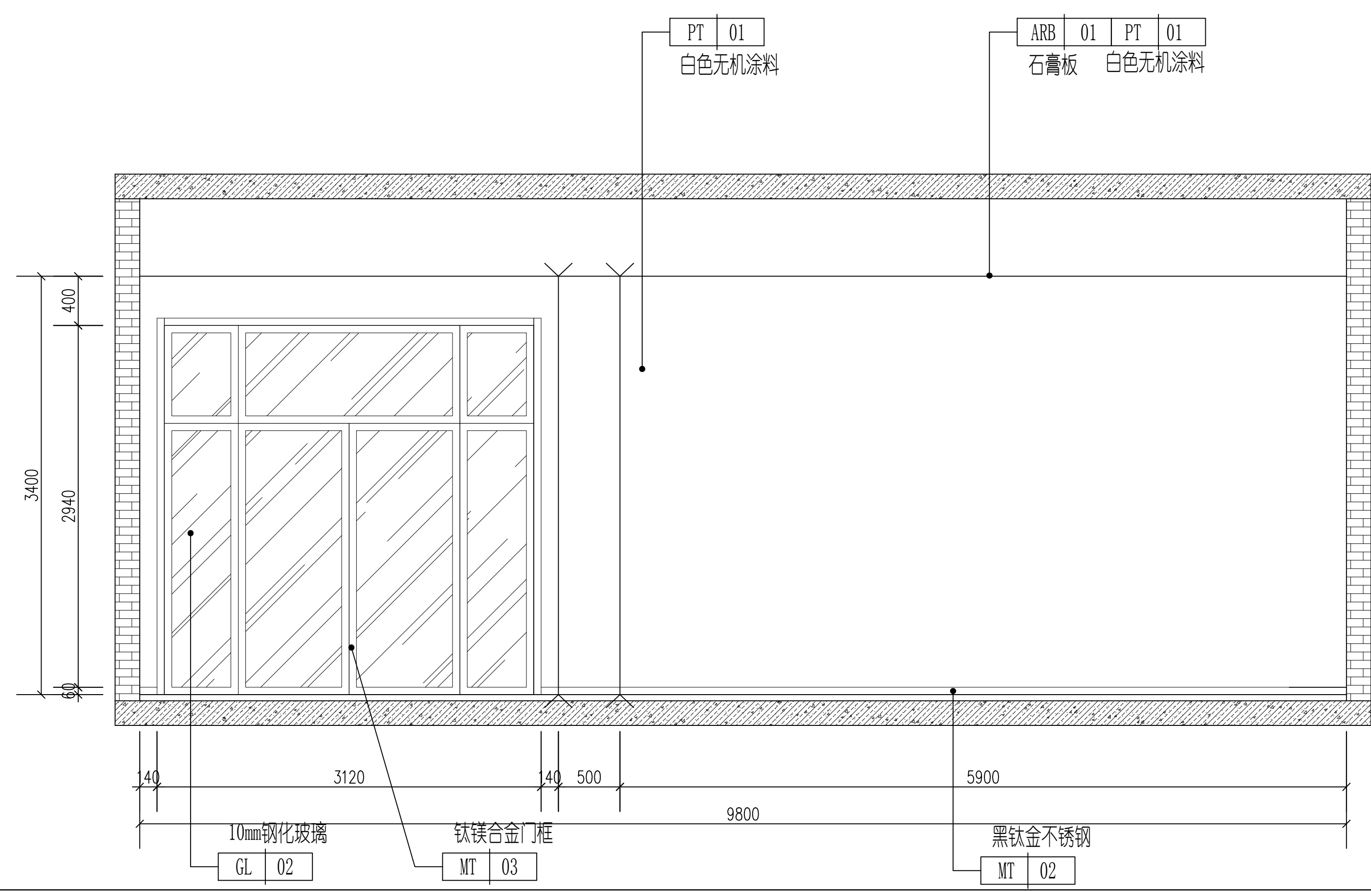
3 北门厅D立面图 1:30
