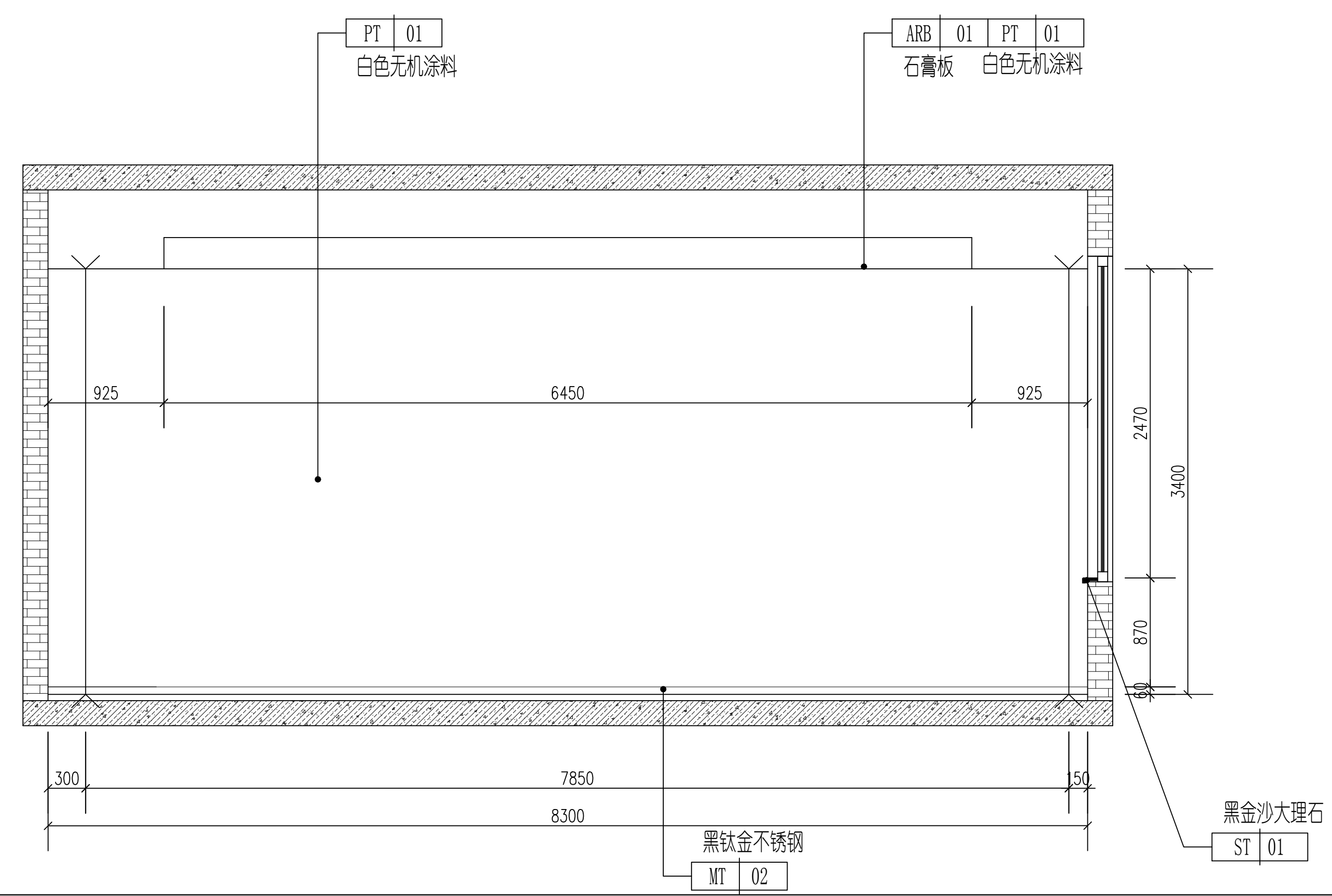
4 微反应器实训中心D立面图 1:30
