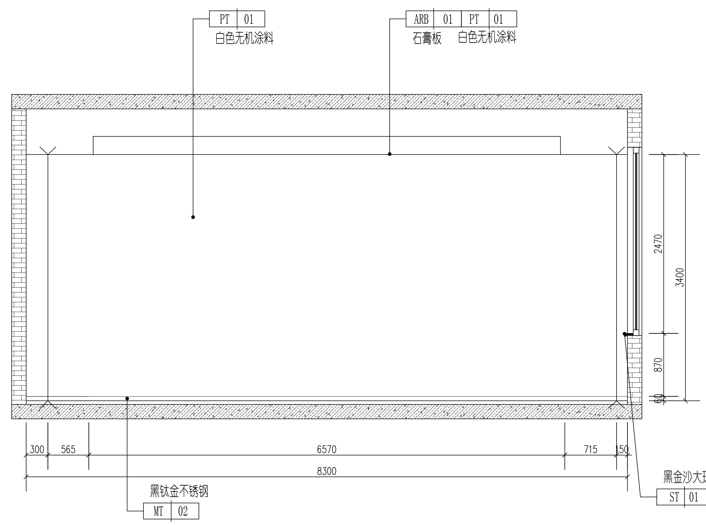
2 喷丝实验室B立面图 1:30
