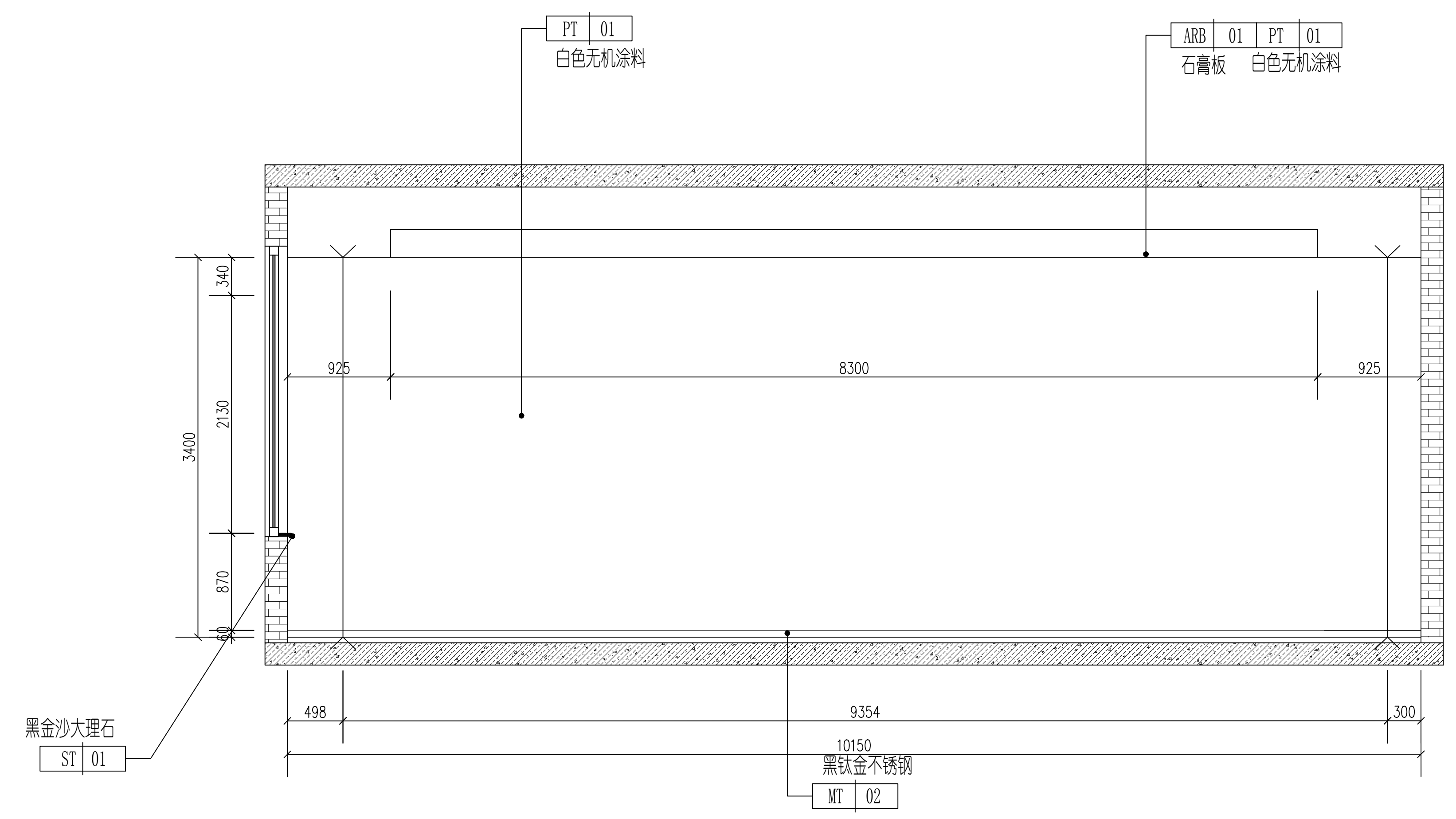
2 备用室B立面图 1:30
