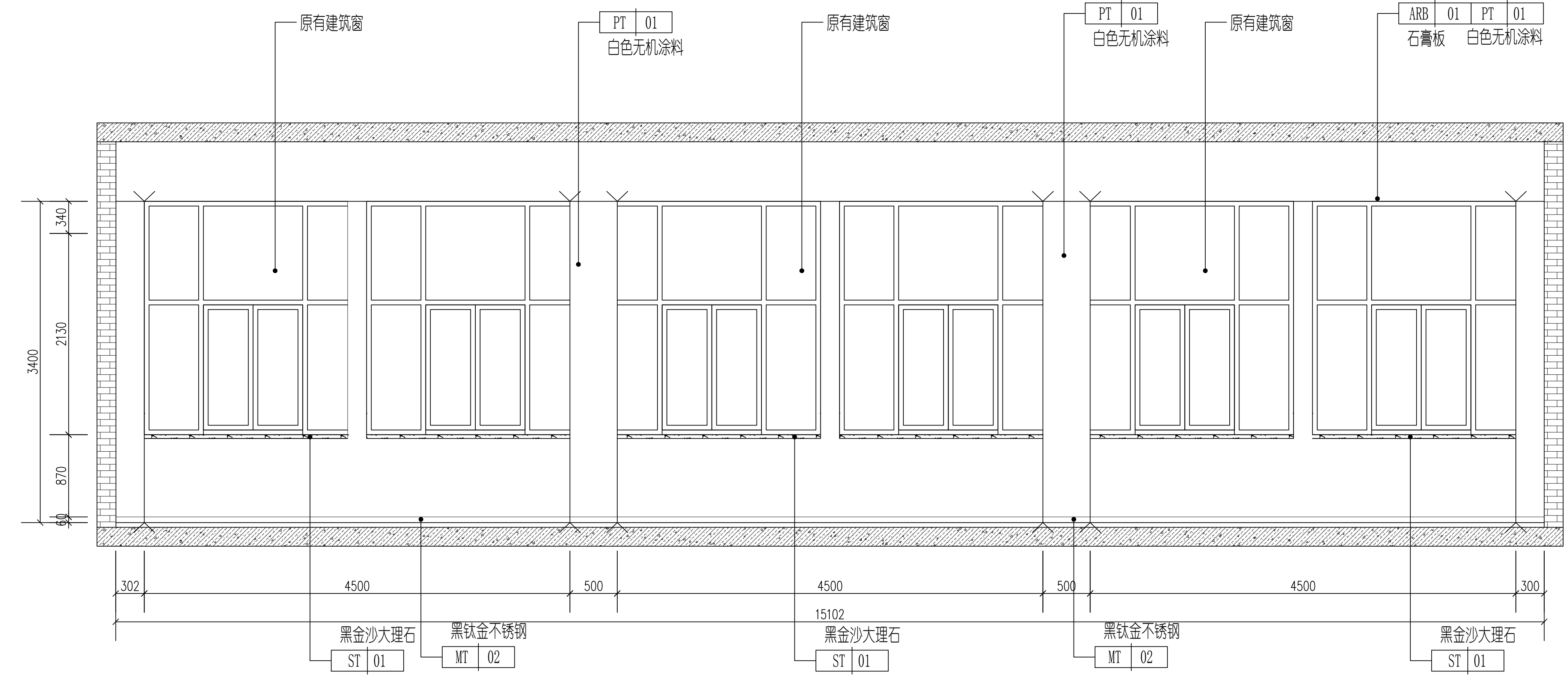
1 备用室A立面图 1:30
