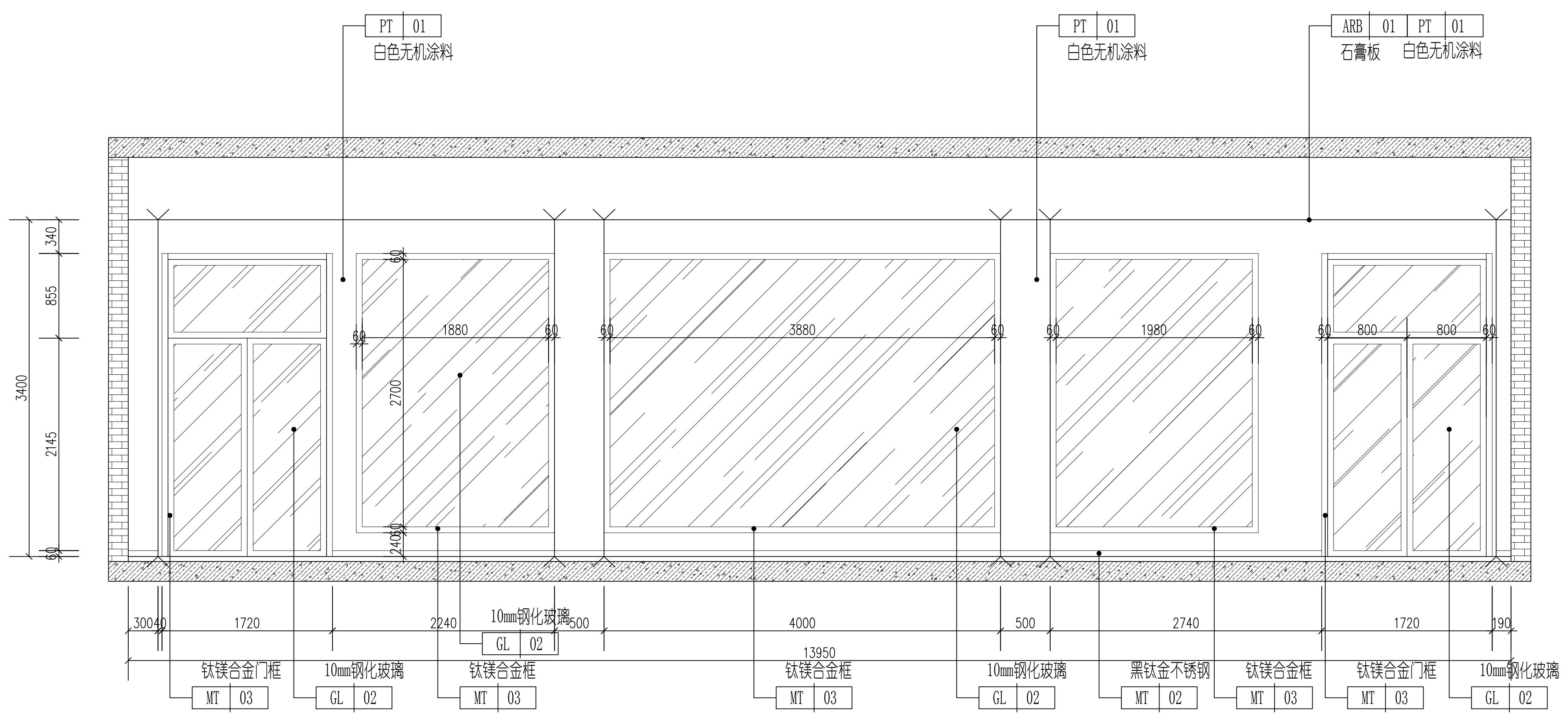
1 共混实验室A立面图 1:30
