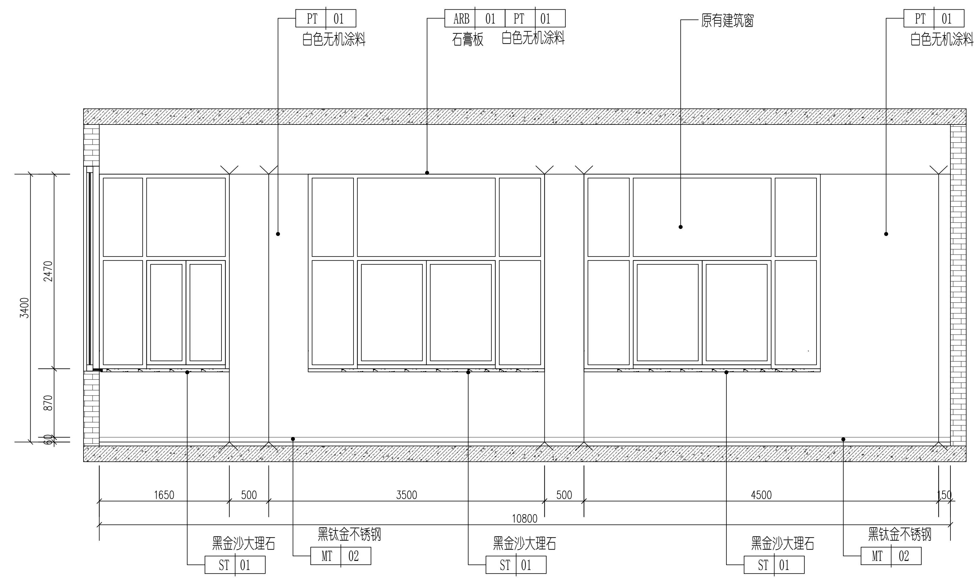
3 仓库C立面图 1:30
