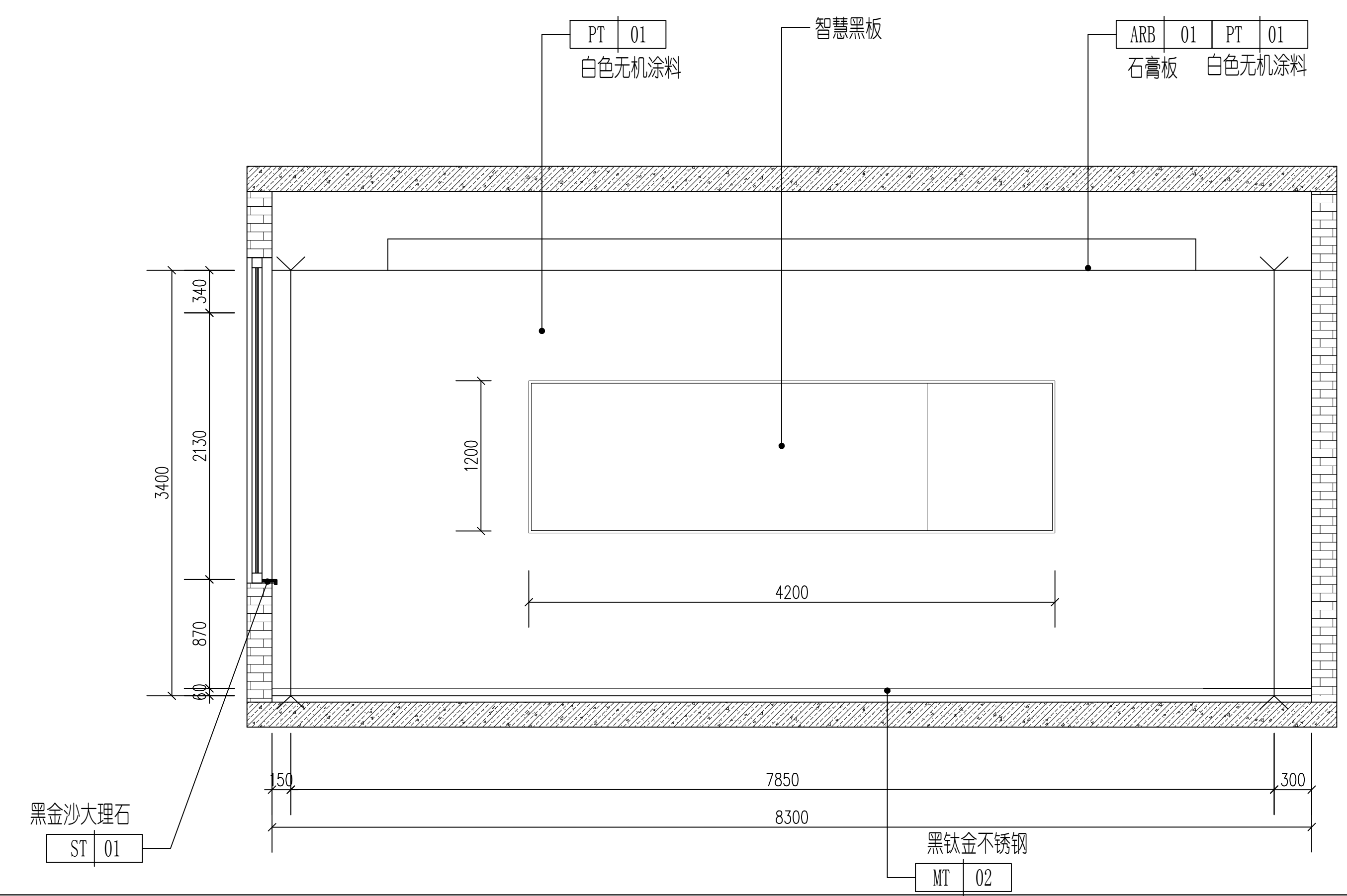
2 微反应器实训中心B立面图 1:30
