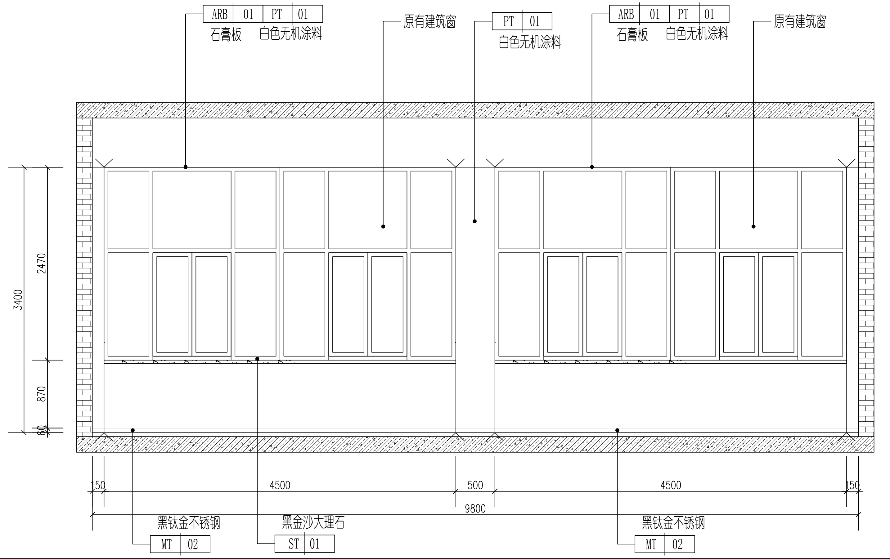
3 吹塑实验室C立面图 1:30
