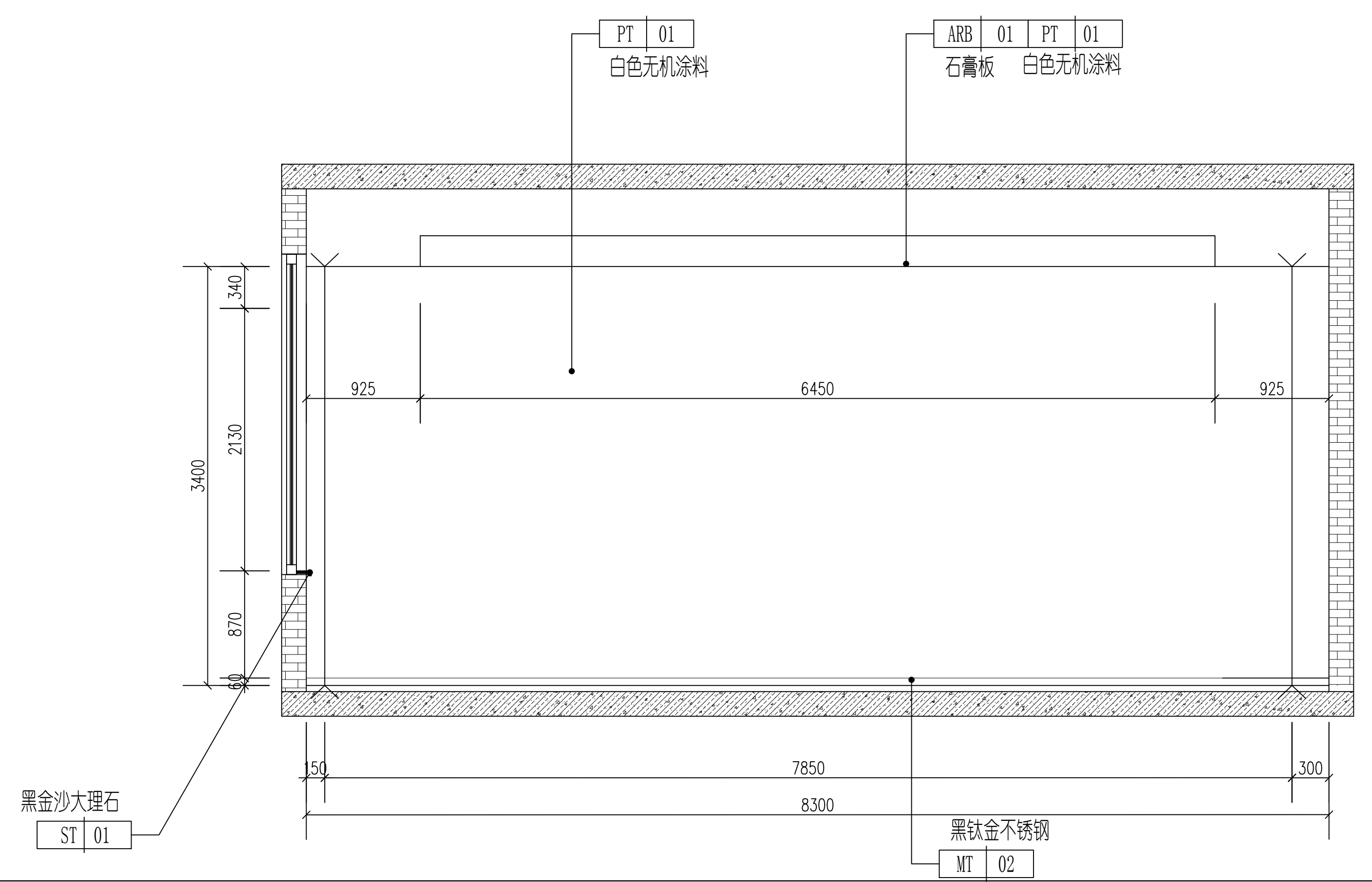
2 检测实验室B立面图 1:30
