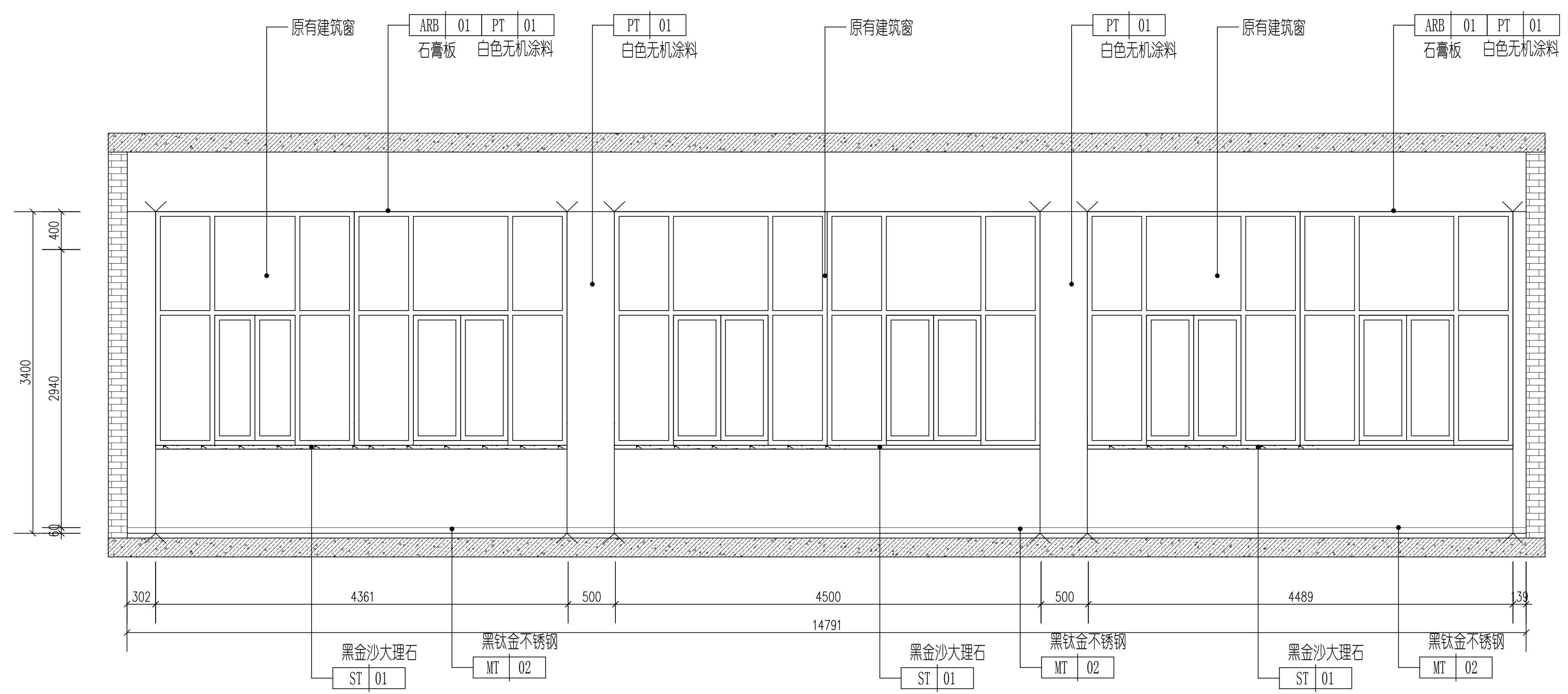
1 微反应器实训中心A立面图 1:30
