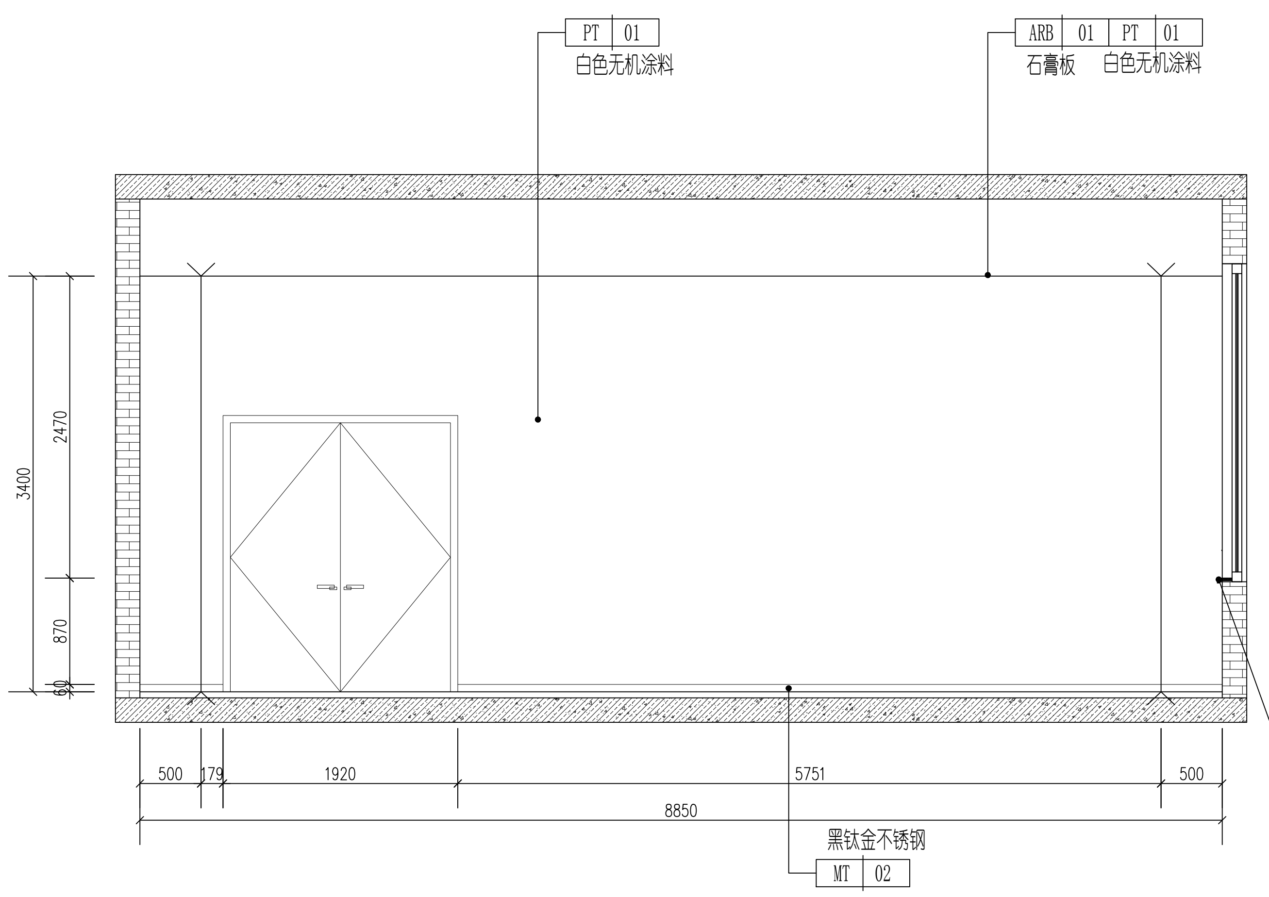
3 高分子材料展厅D立面图 1:30
