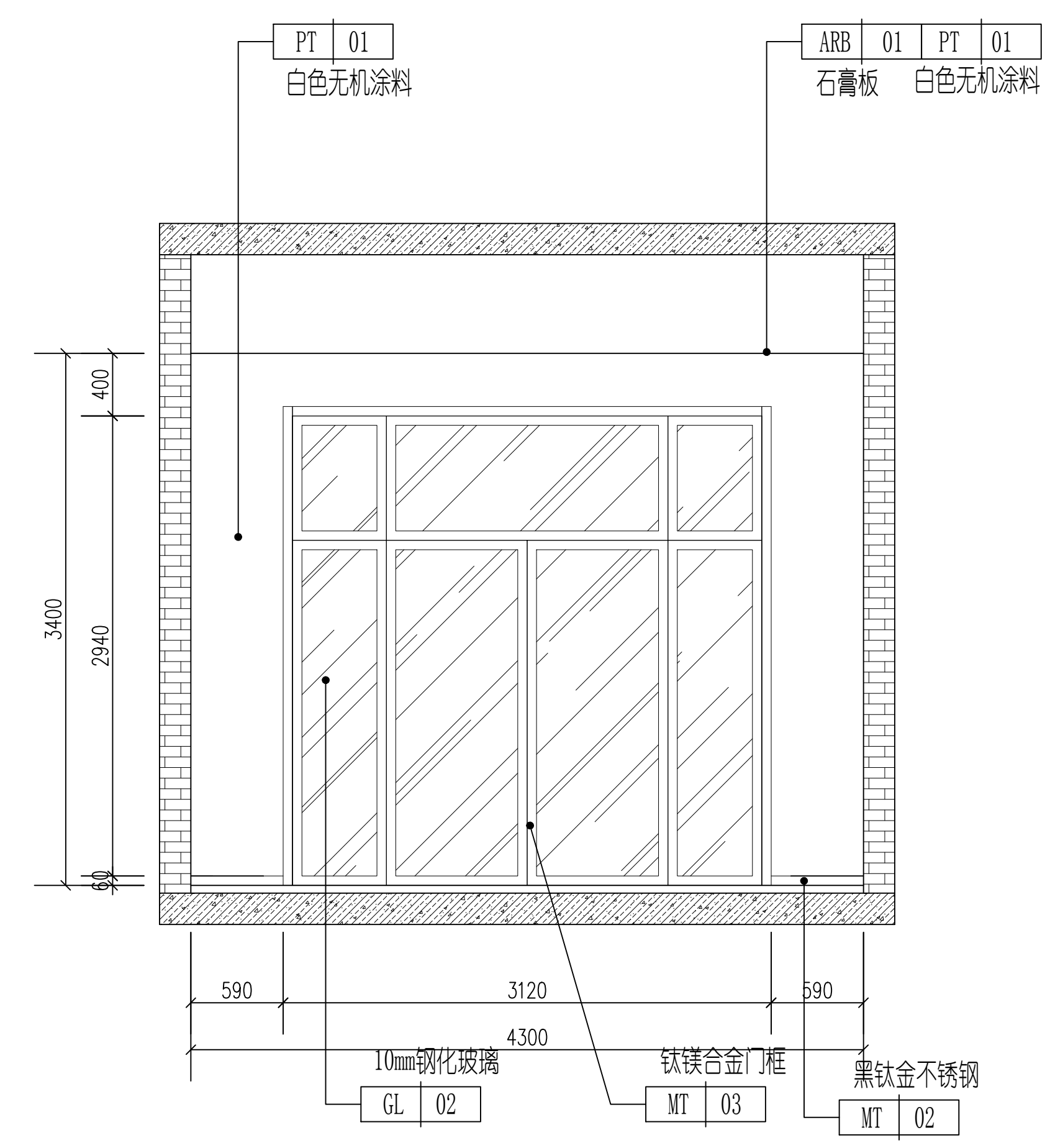
1 北门厅A立面图 1:30
