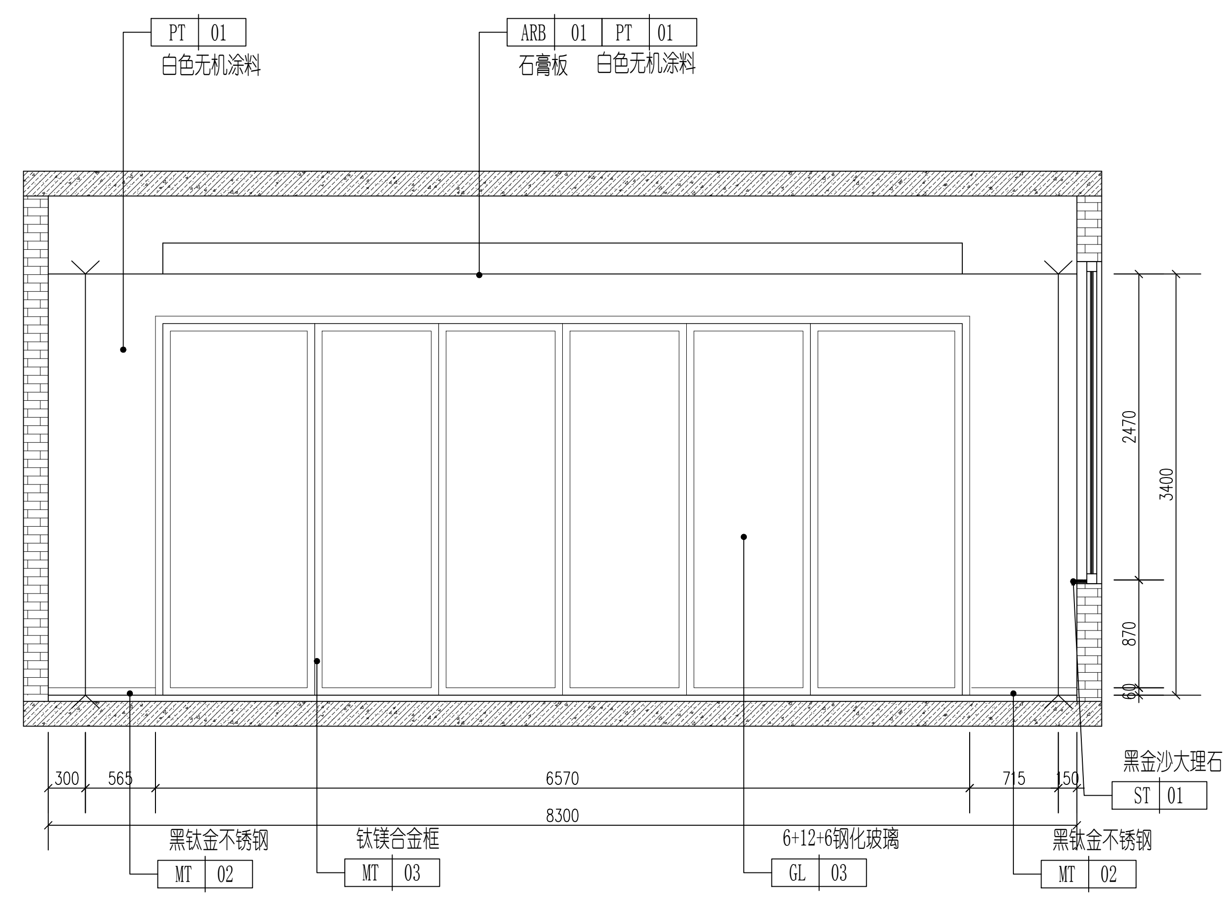
2 拉膜实验室B立面图 1:30
