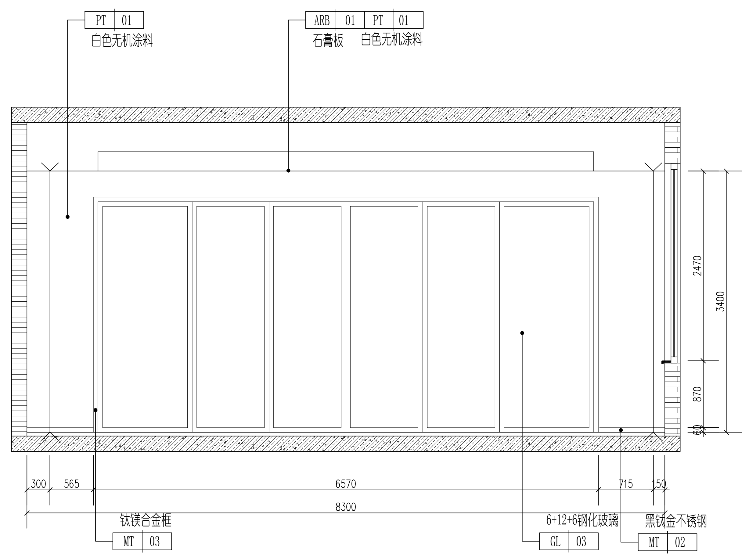
2 吹塑实验室C立面图 1:30
