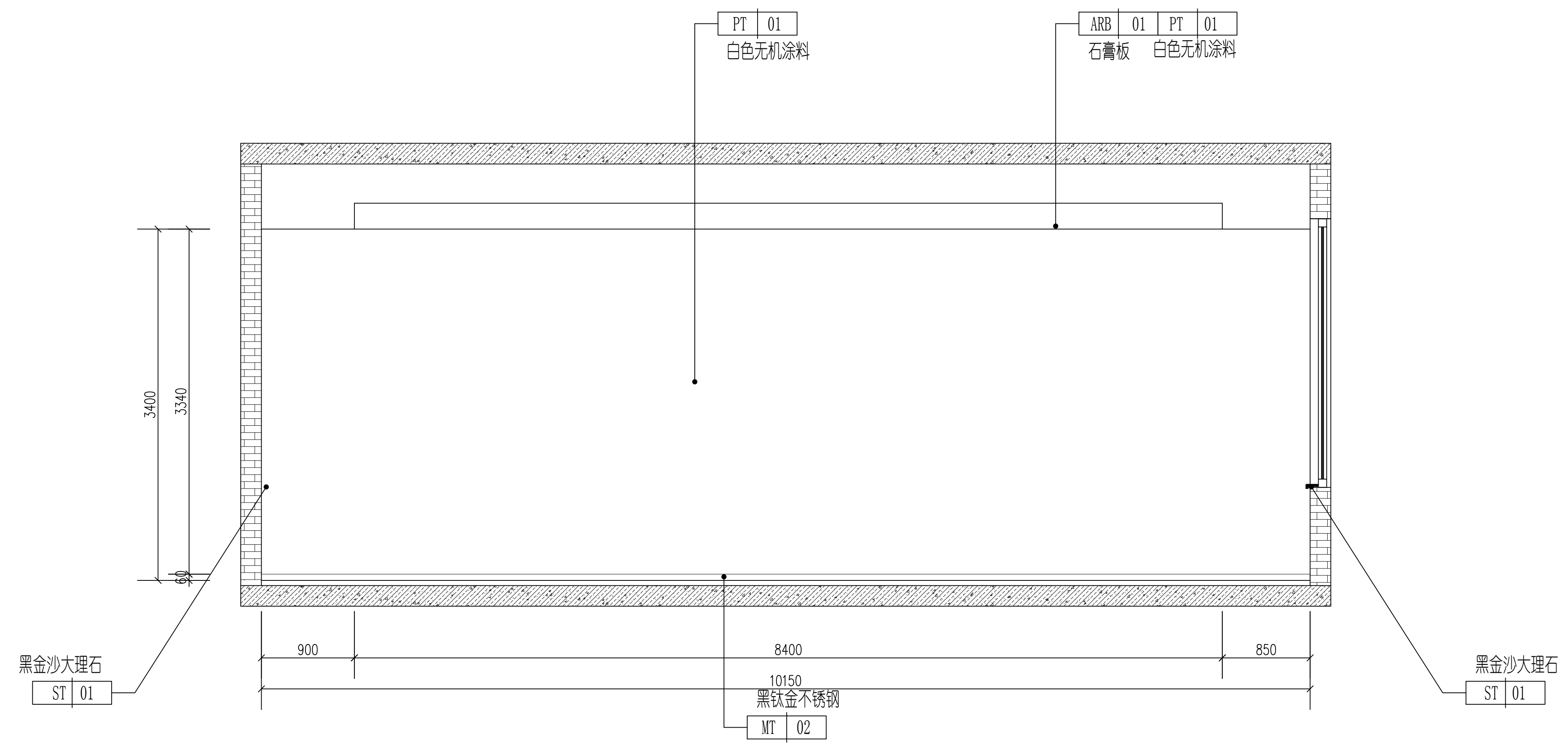
2 合成室B立面图 1:30
