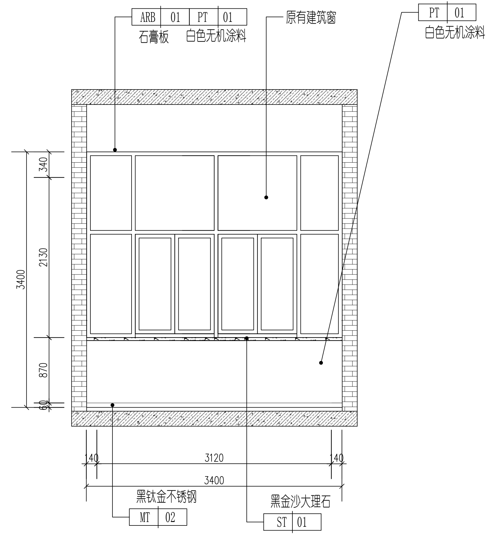
1 南门厅C立面图 1:30
