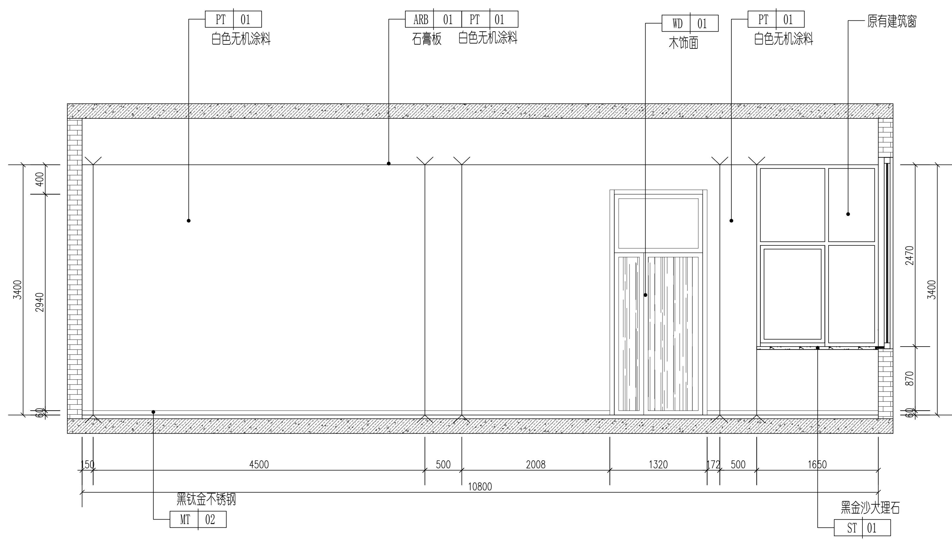
1 仓库A立面图 1:30
