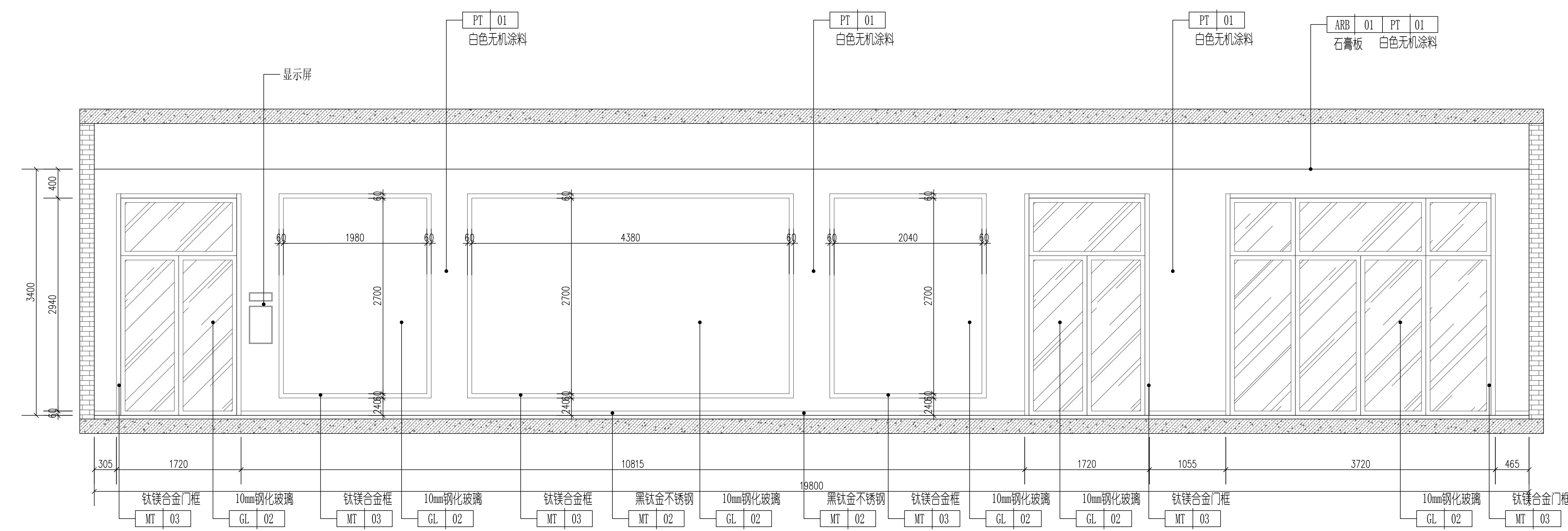
2 过道2C立面图 1:30
