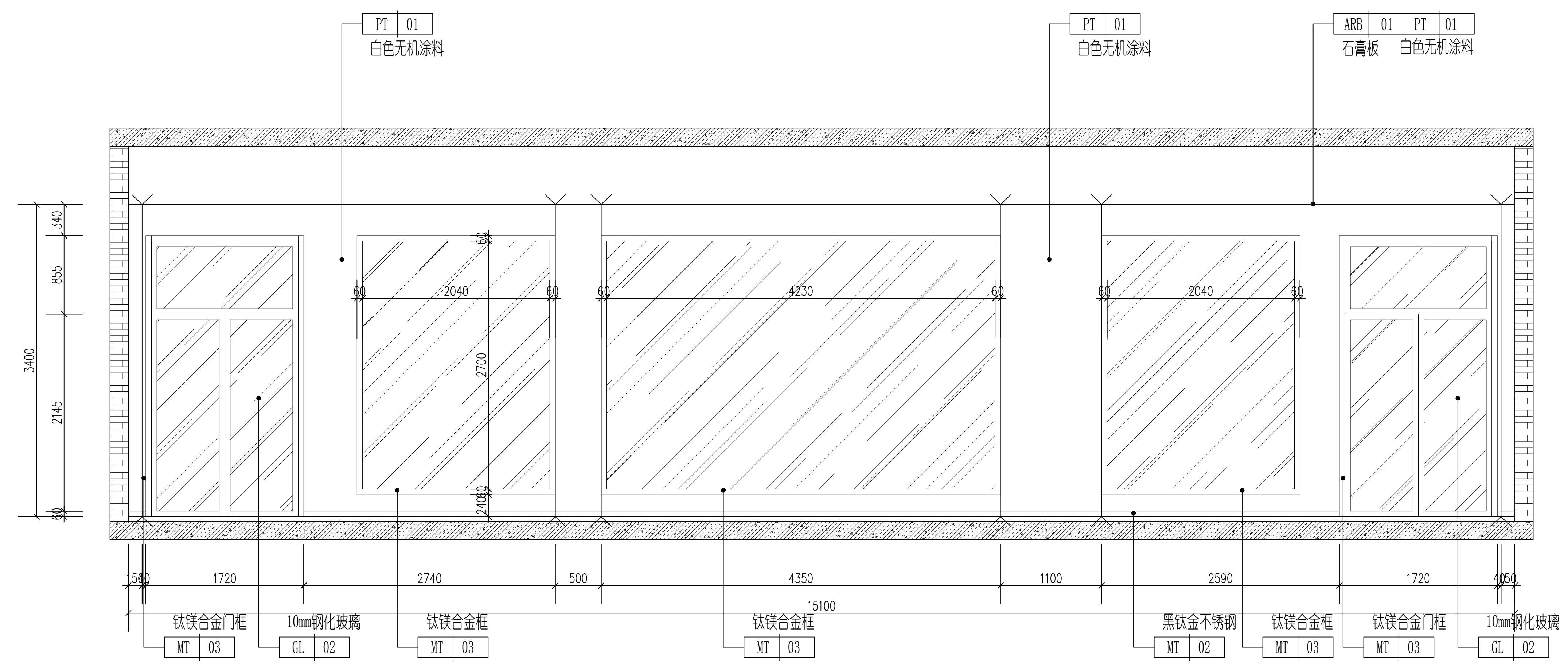
1 注塑实验室A立面图 1:30
