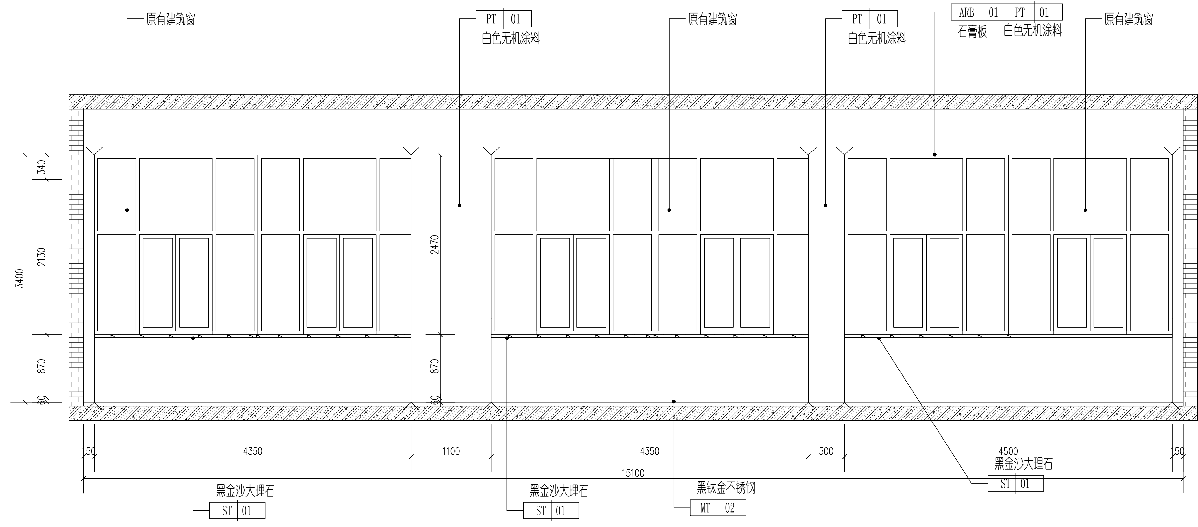
3 注塑实验室C立面图 1:30
