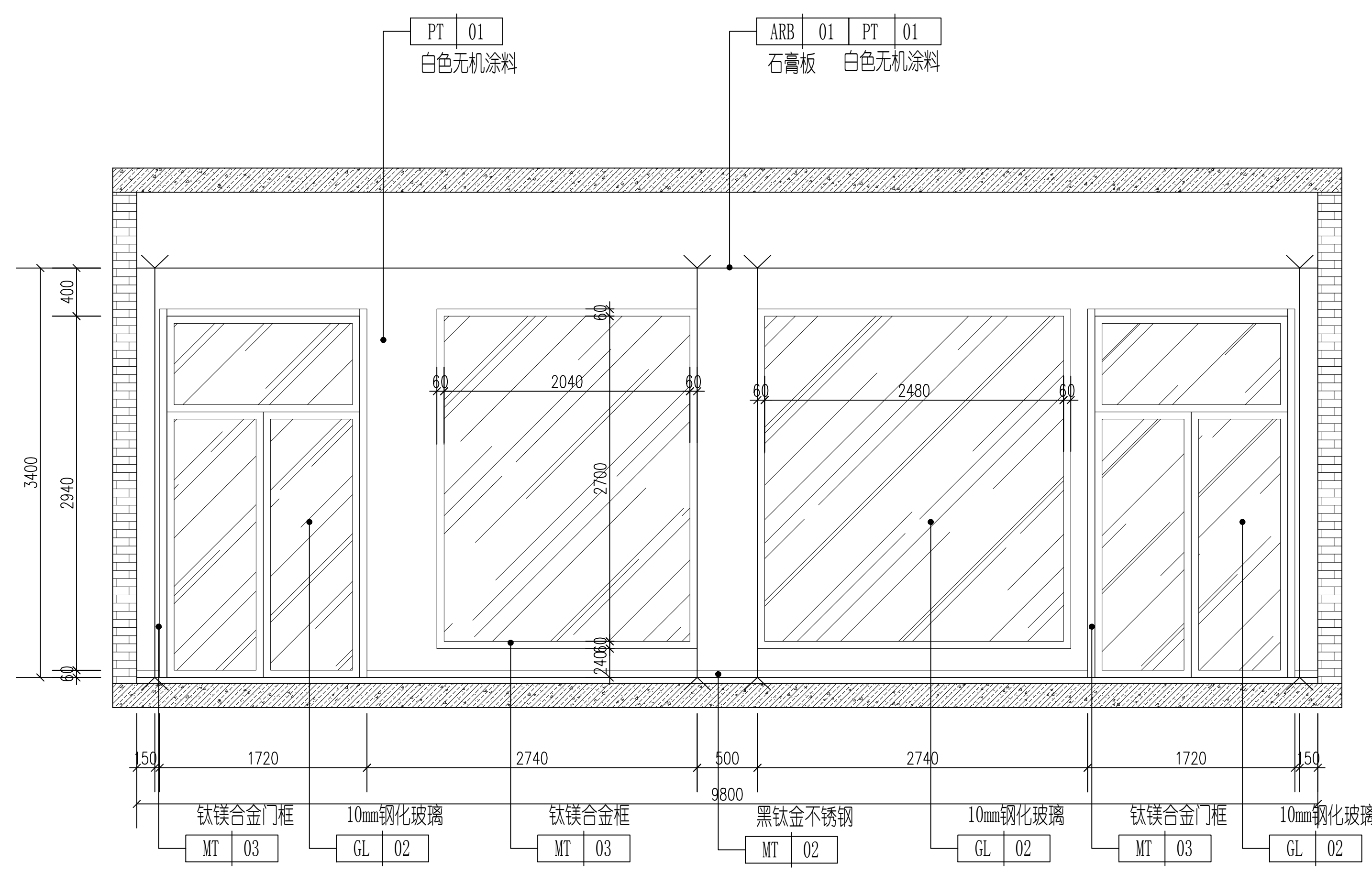
1 吹塑实验室A立面图 1:30
