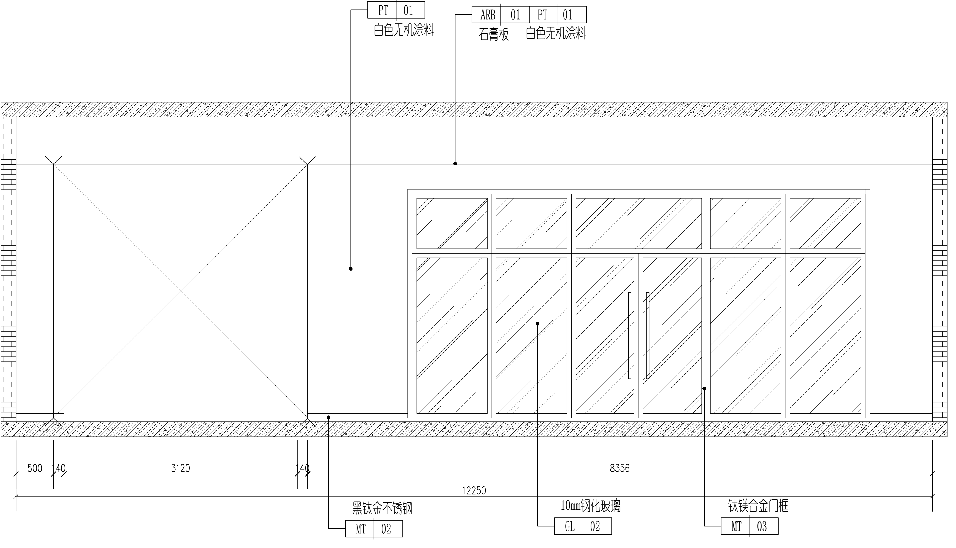
2 南门厅D立面图 1:30
