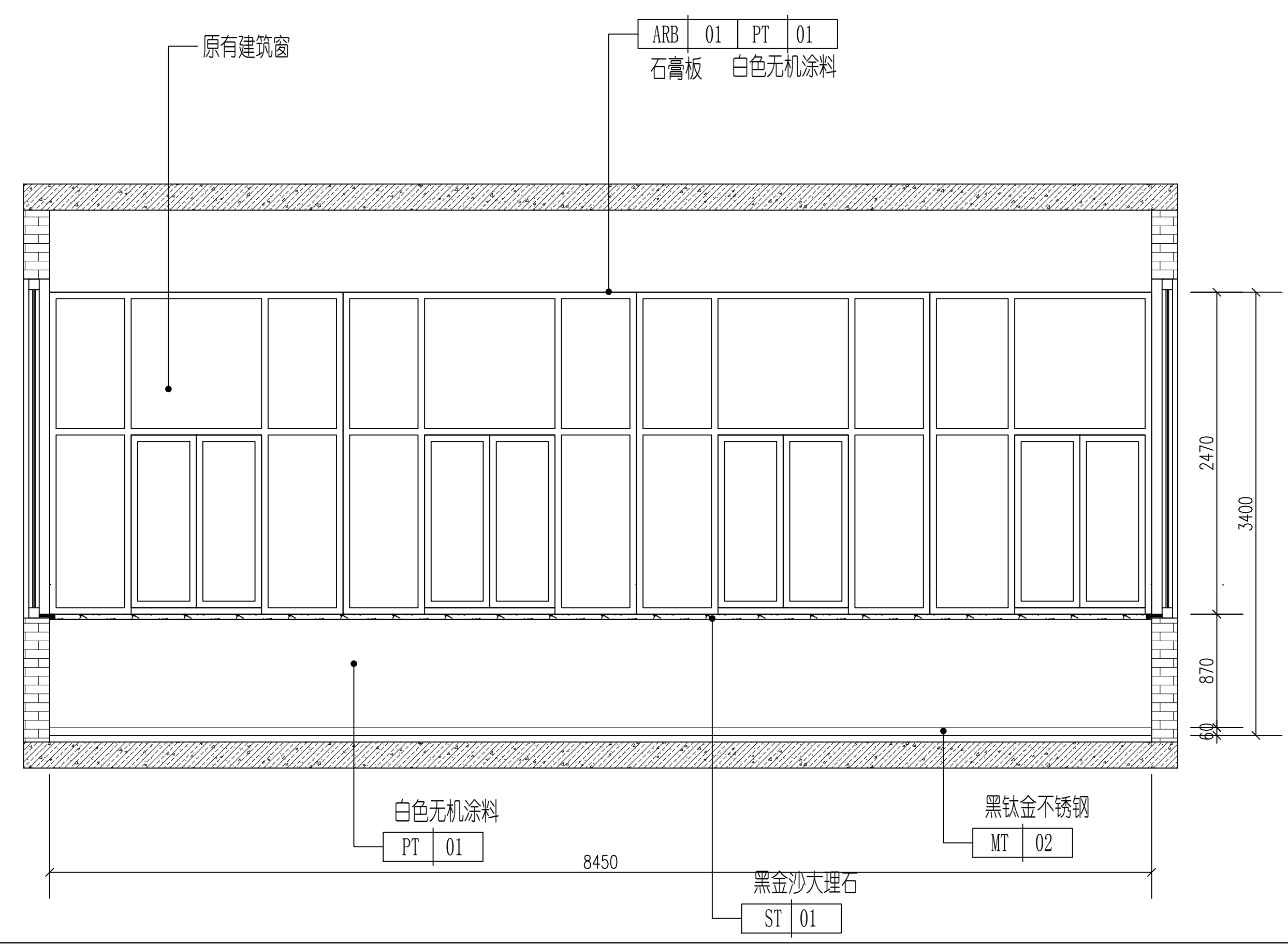
2 仓库B立面图 1:30
