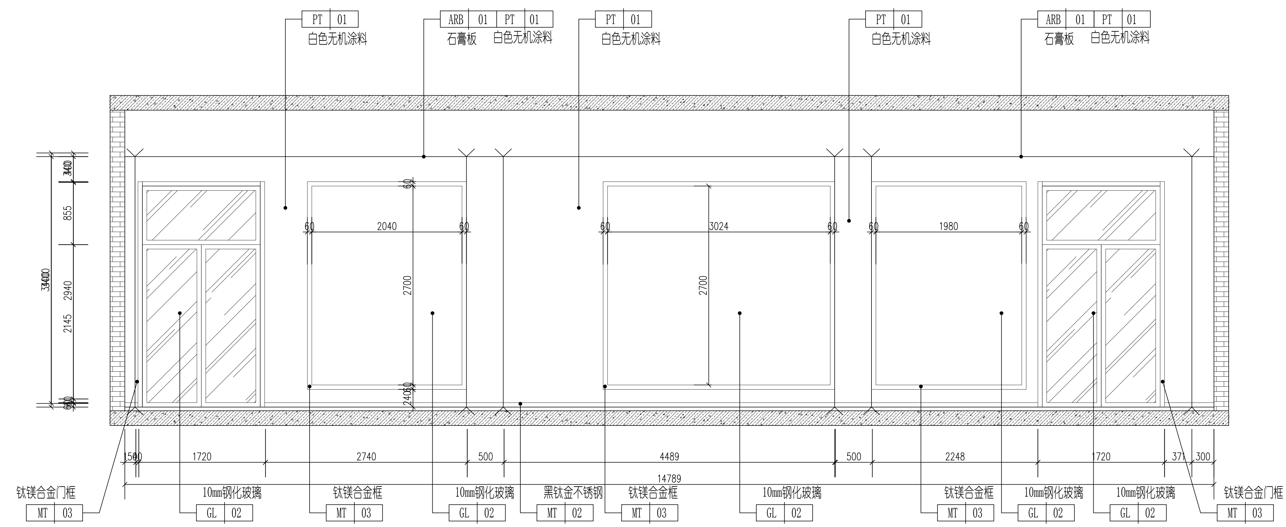
3 微反应器实训中心C立面图 1:30
