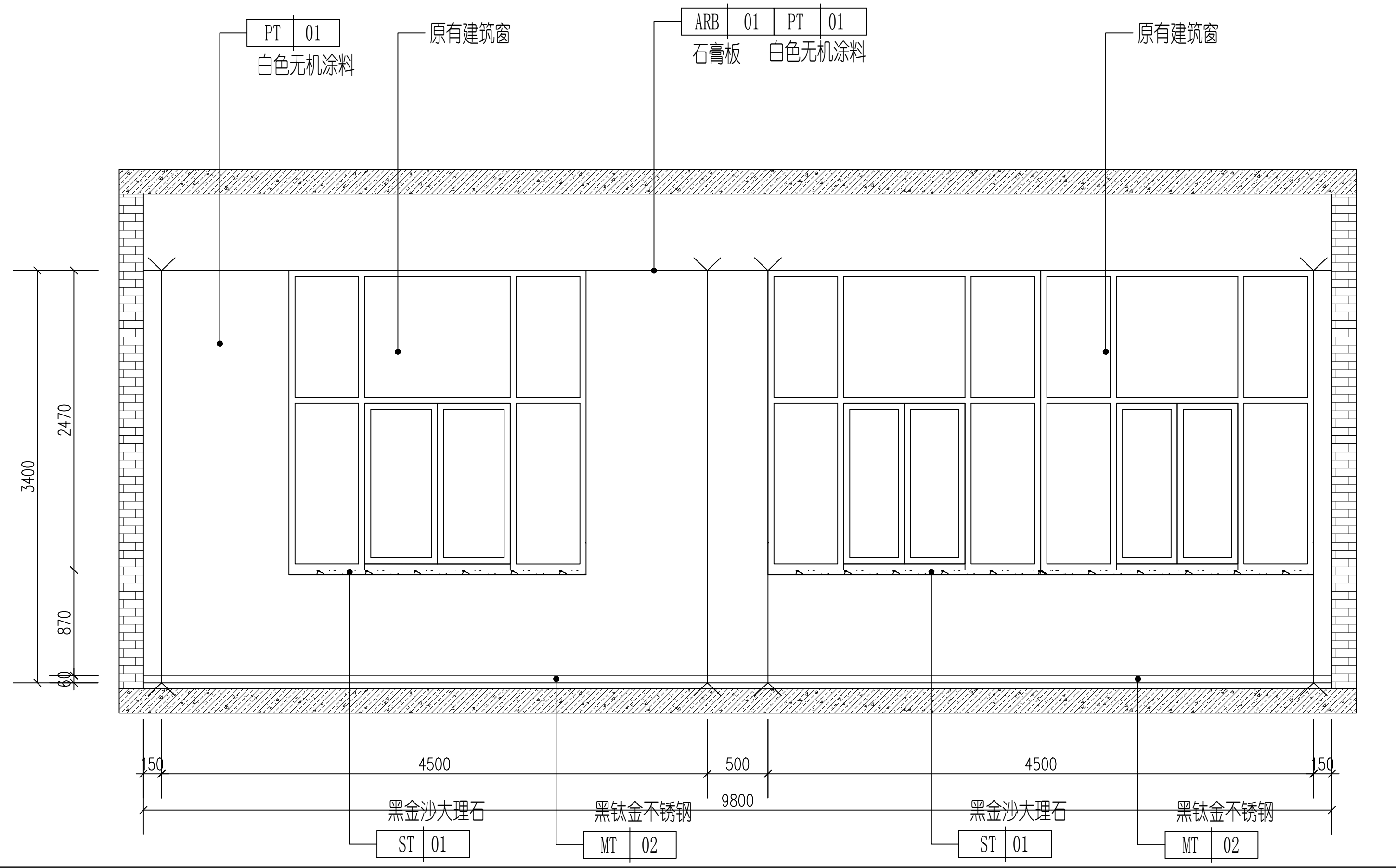
3 喷丝实验室C立面图 1:30
