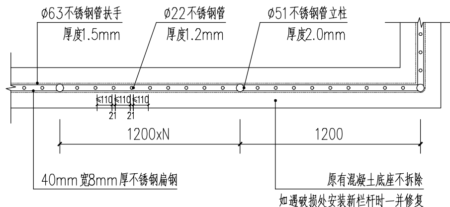
栏杆平面详图 1:25
