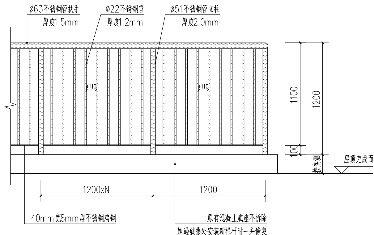
栏杆立面详图 1:25
