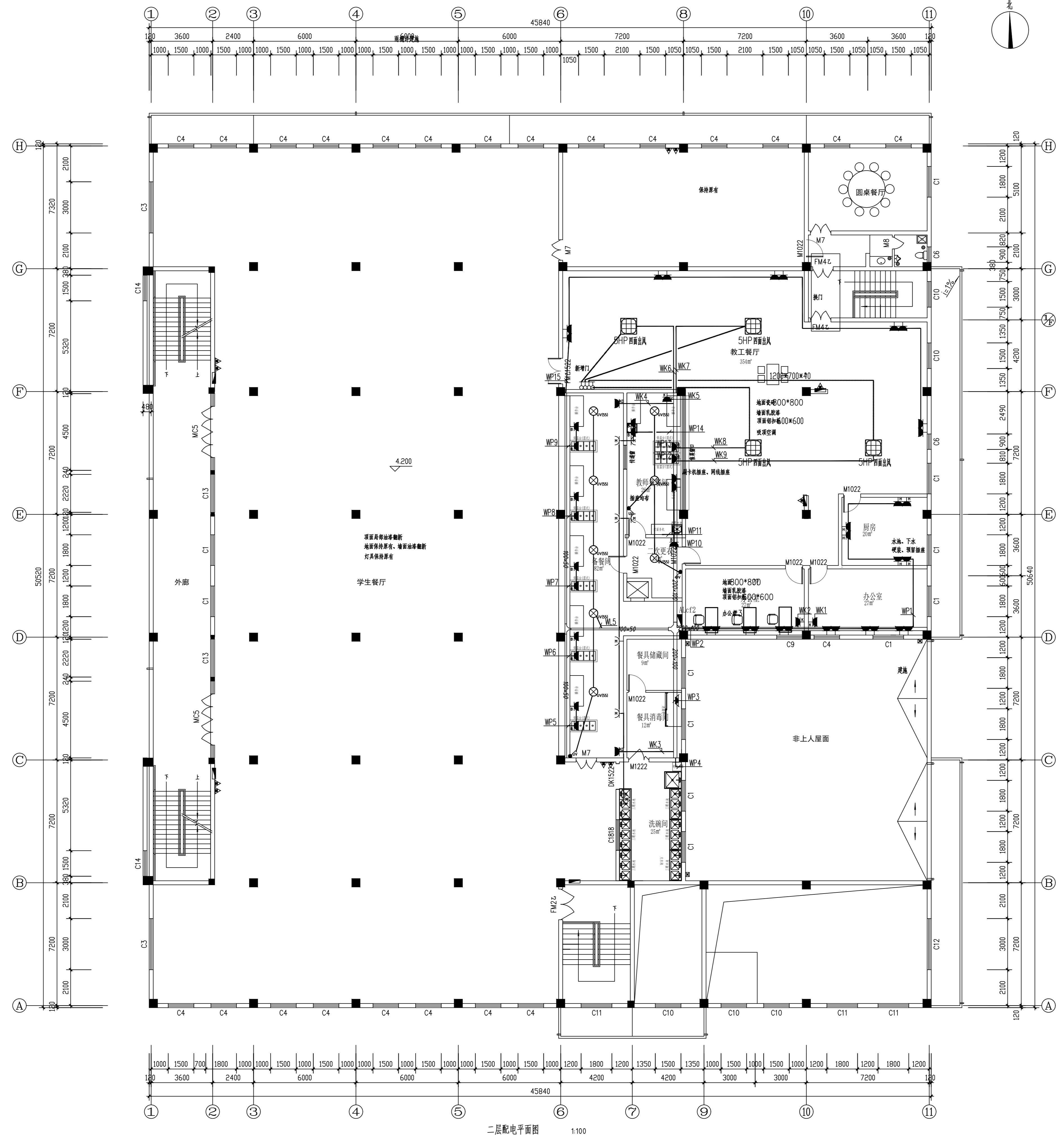
二层配电平面图 1:100
