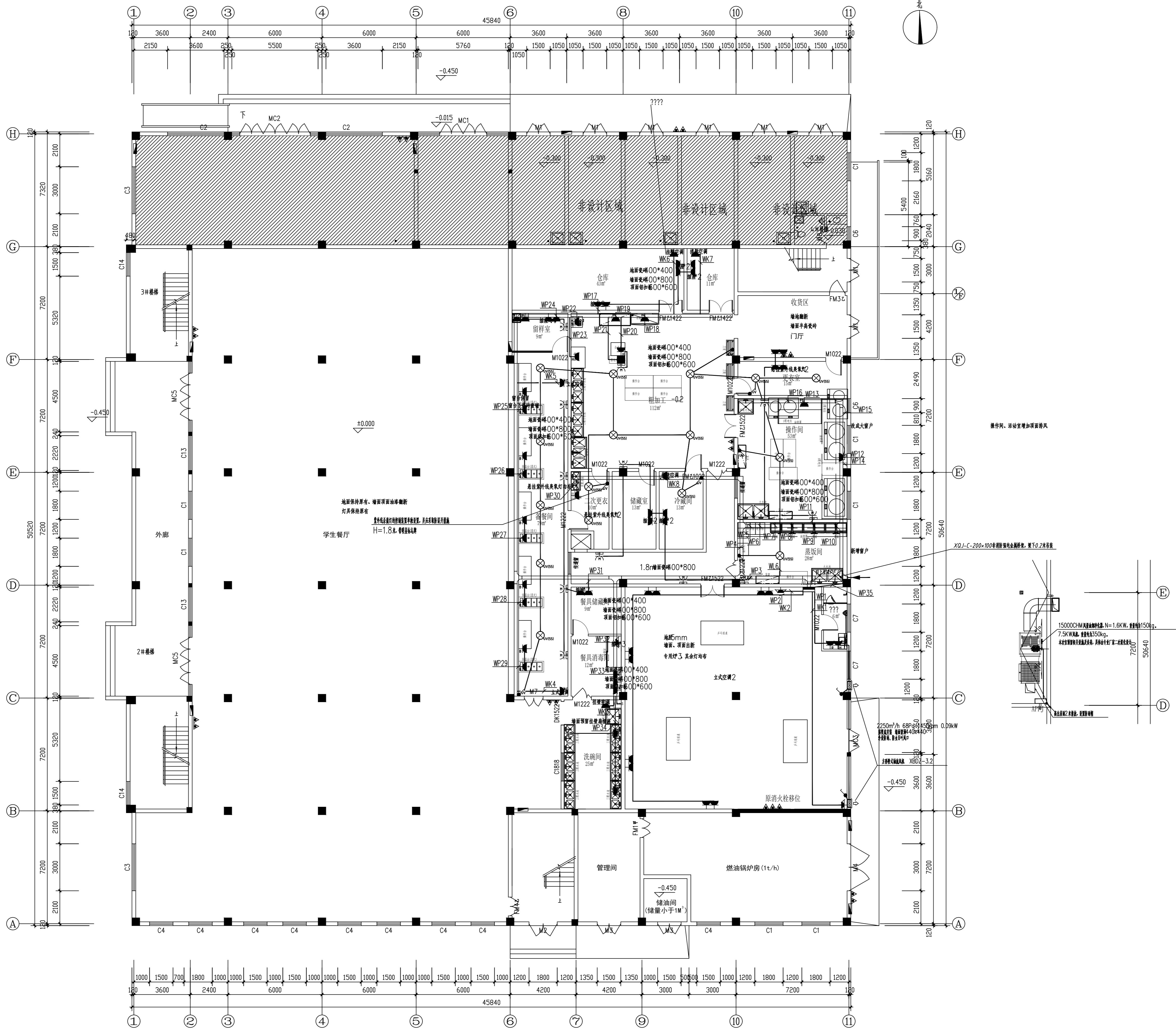
一层配电平面图 1:100
