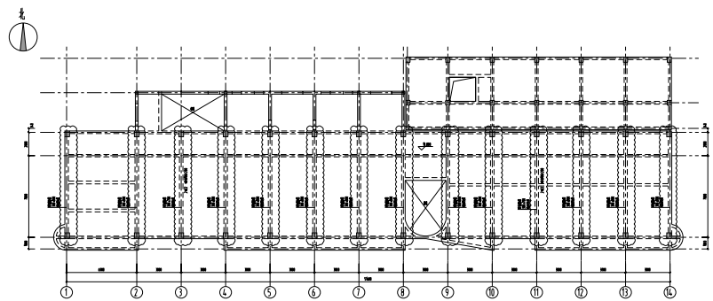
四层楼面结构加固平面示意图
