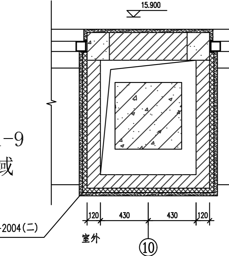
① 墙身详图 1:20
