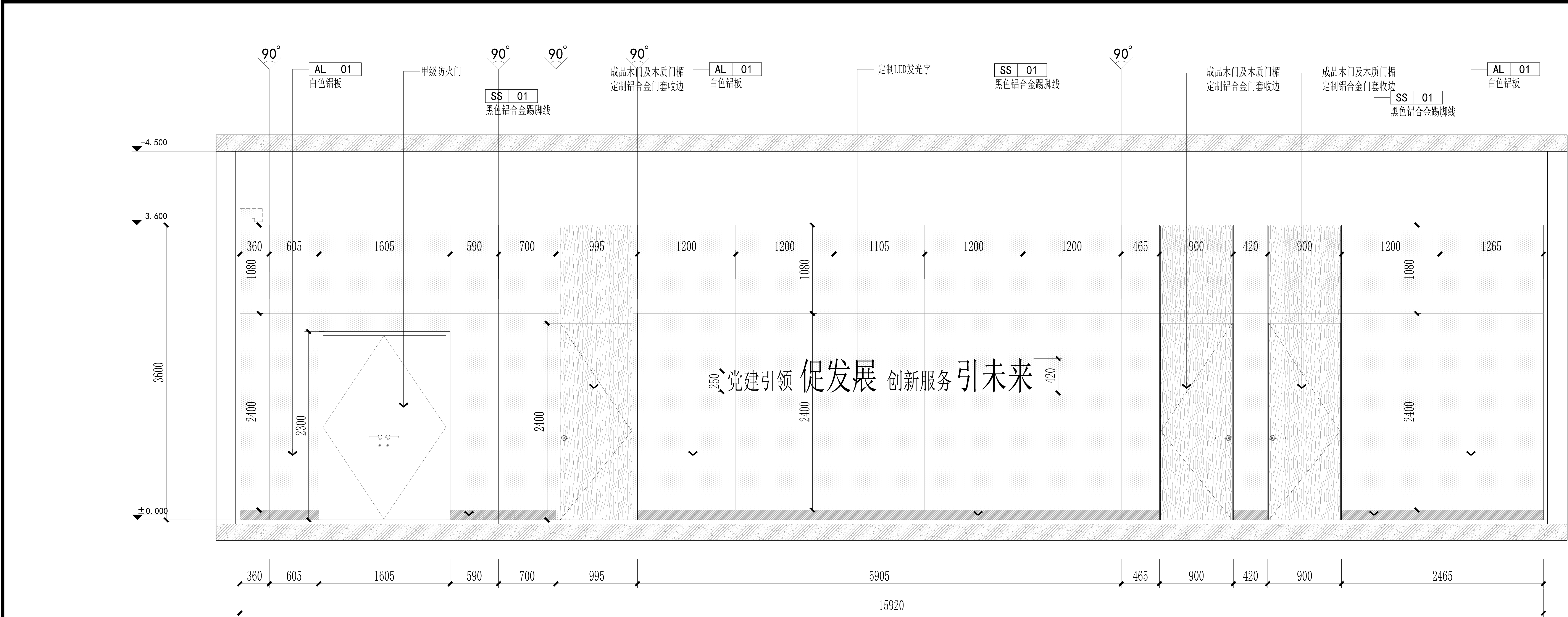
E3 ELEVATION 立面图
