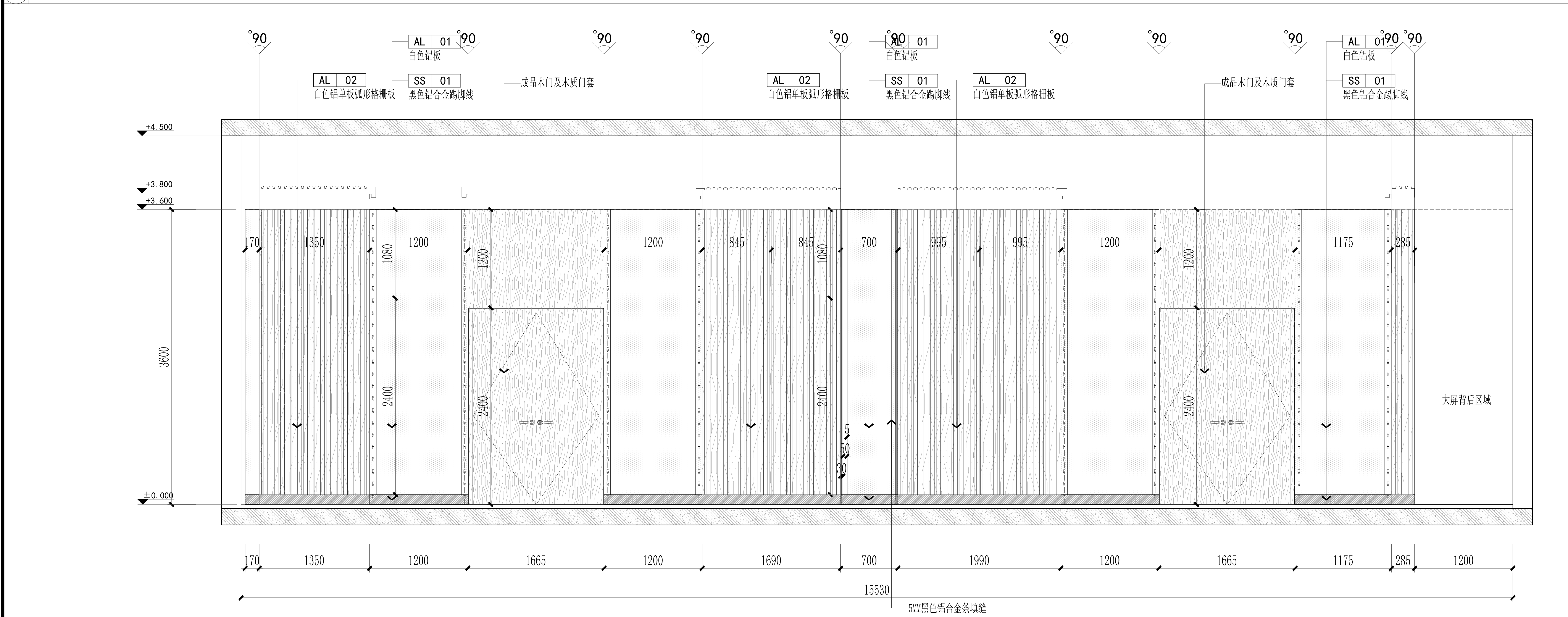
E4 ELEVATION 立面图
