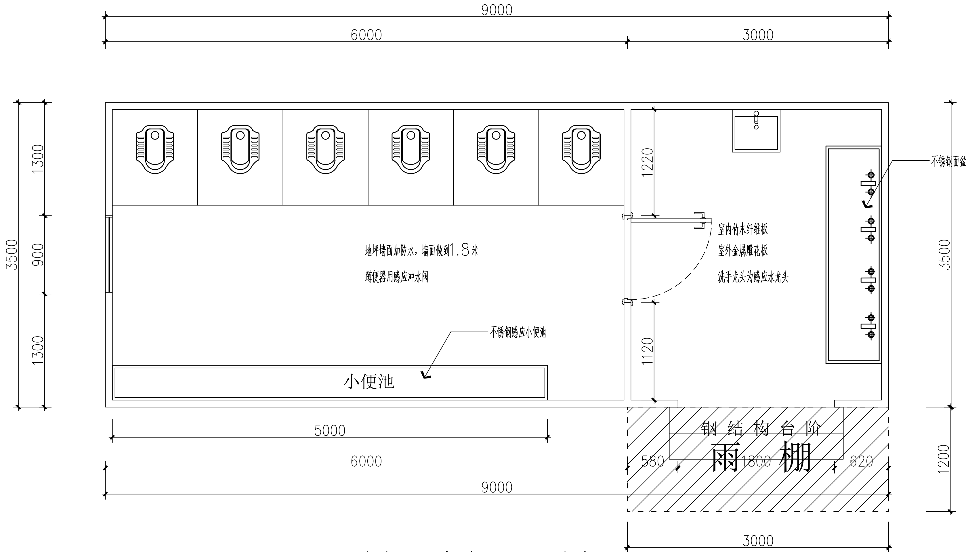
男卫生间平面布局
