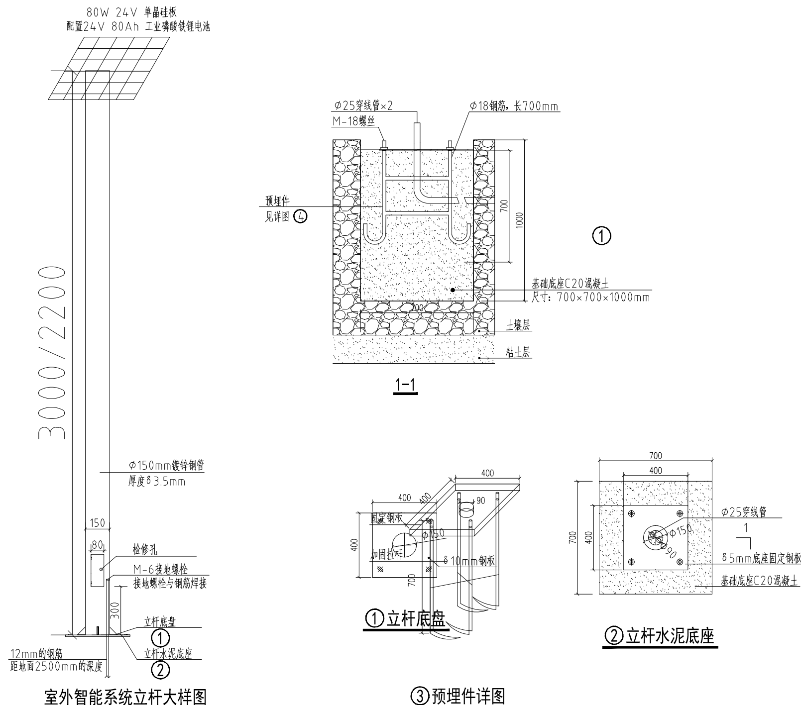
室外智能系统立杆大样图 太阳能板供电 内置：锂电池、MPPT 控制器、空开、防雷模块
