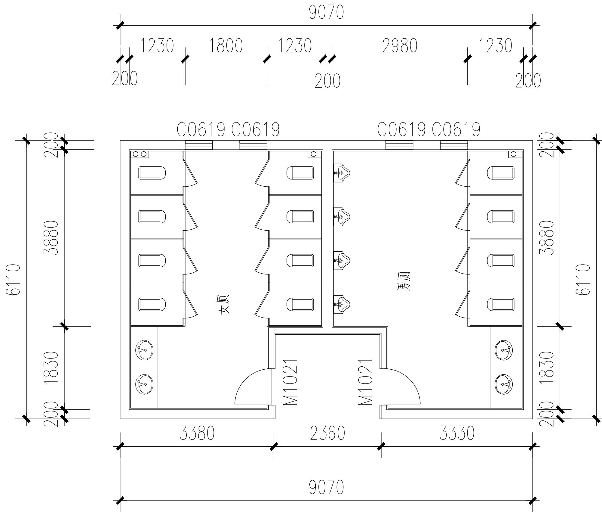
拆除平面图
