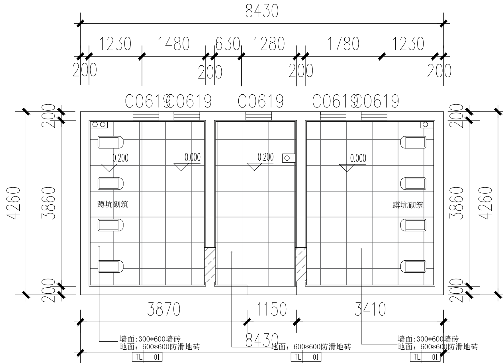
地面铺装图
