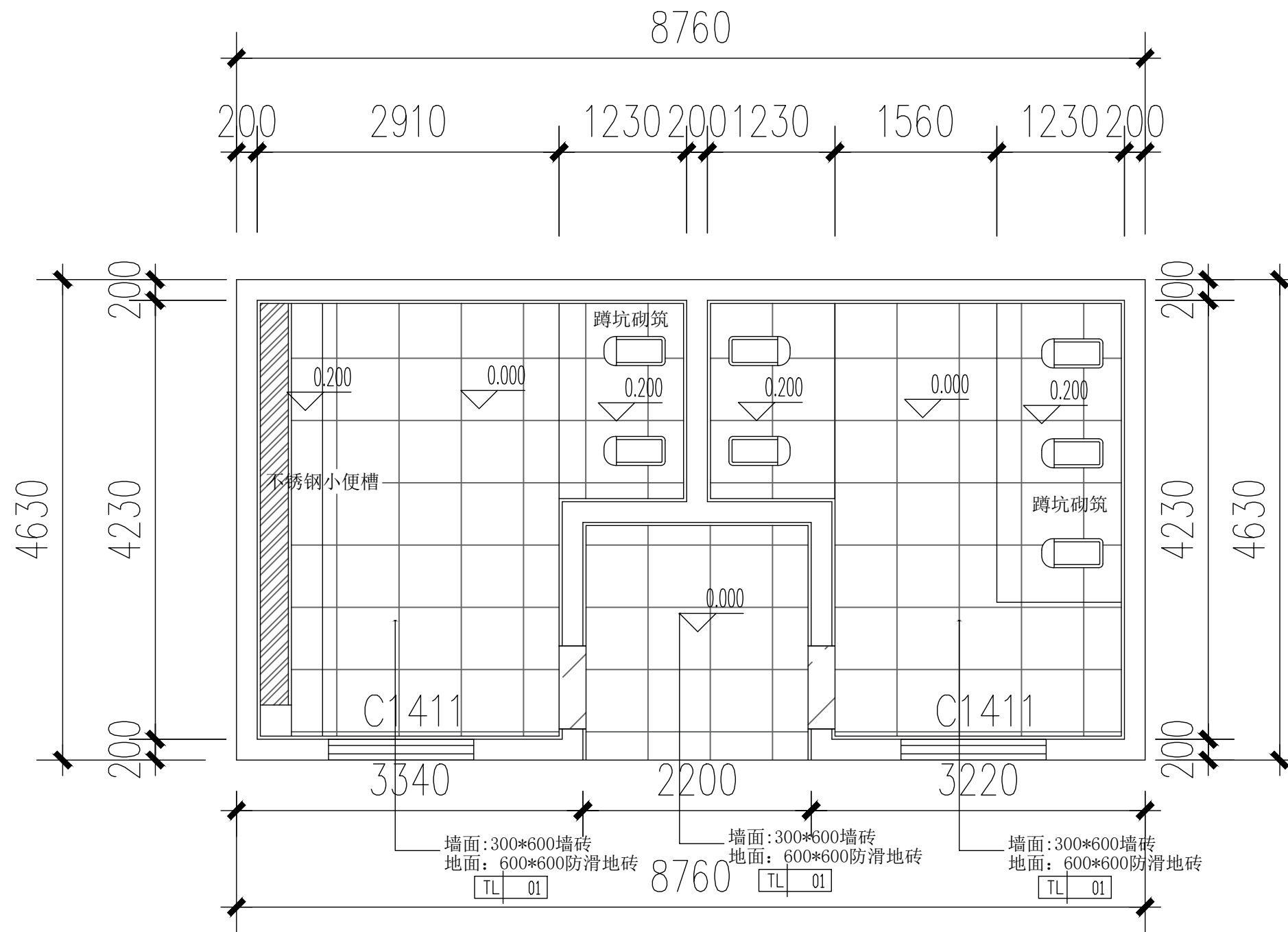
地面铺装图
