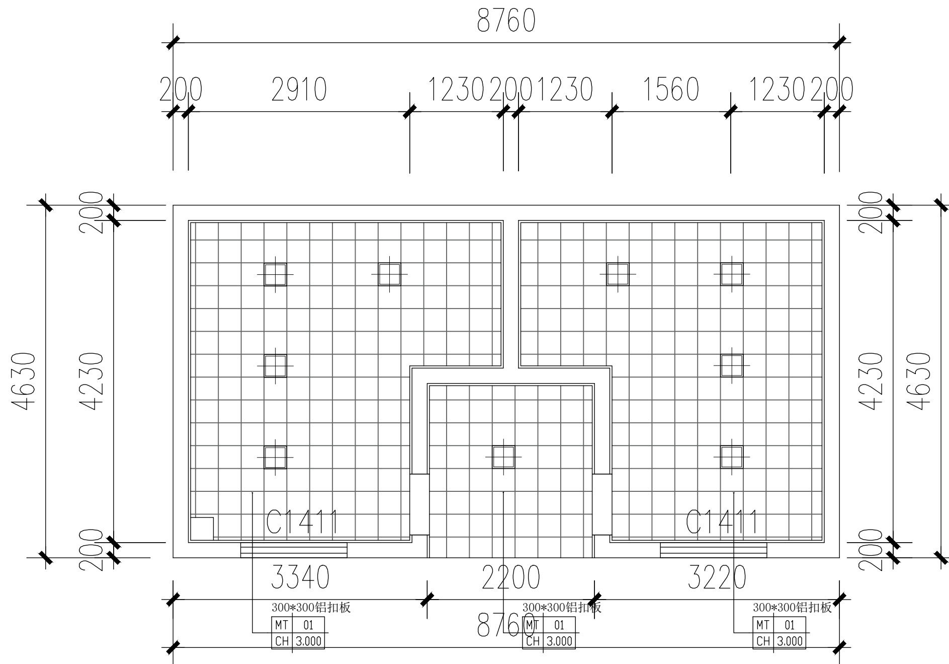
天花布置图
