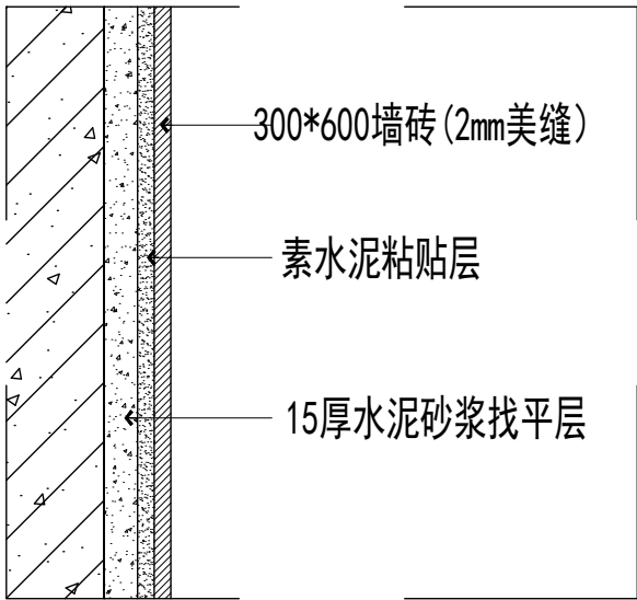
SECTION DETAIL 通用 墙砖做法 SCALE 1:3
