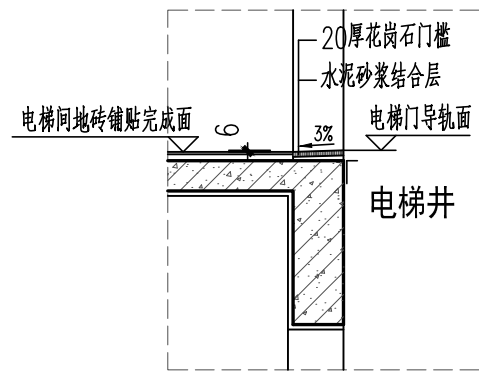
电梯厅及电梯井挡水示意图
