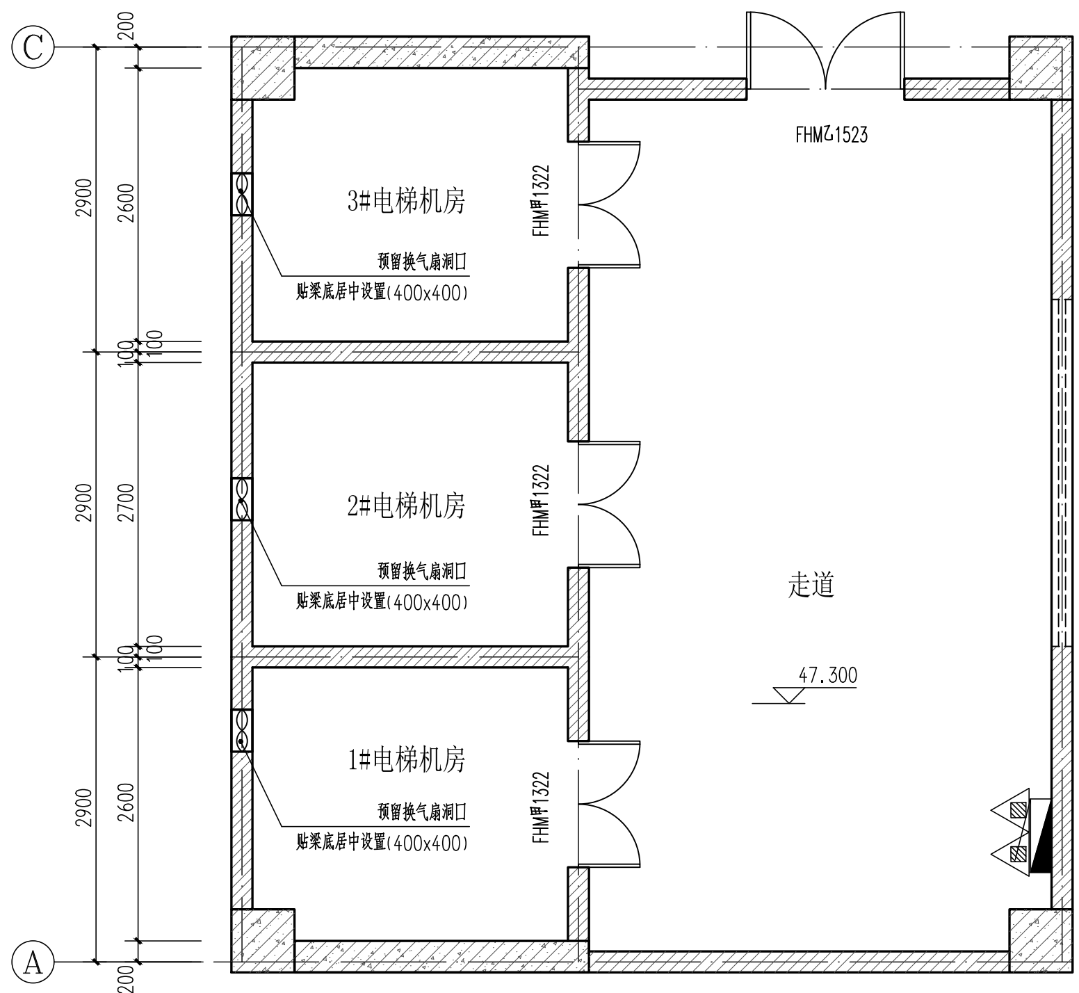
电梯机房平面放大图 1:50
