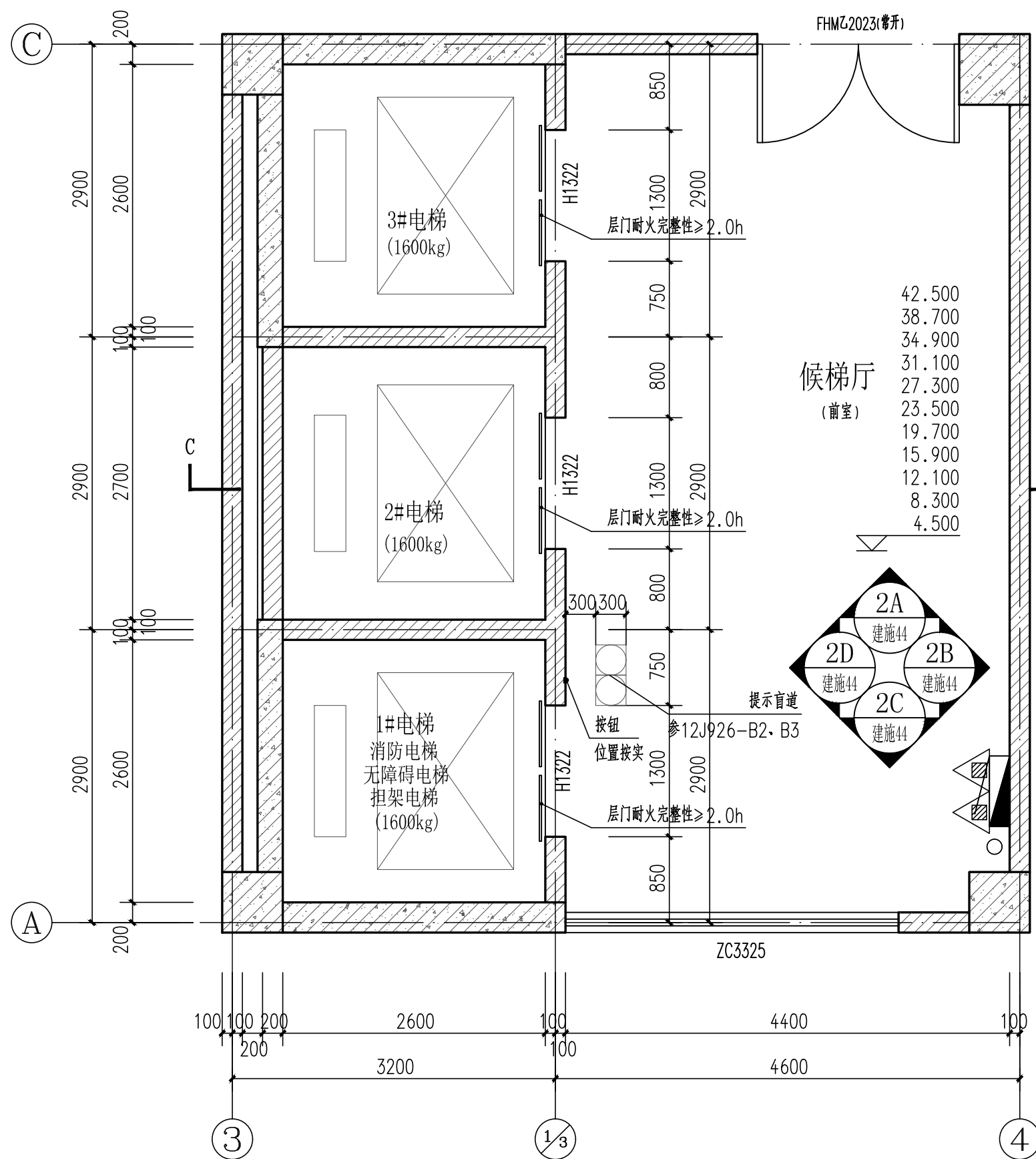
电梯平面放大图 1:50
