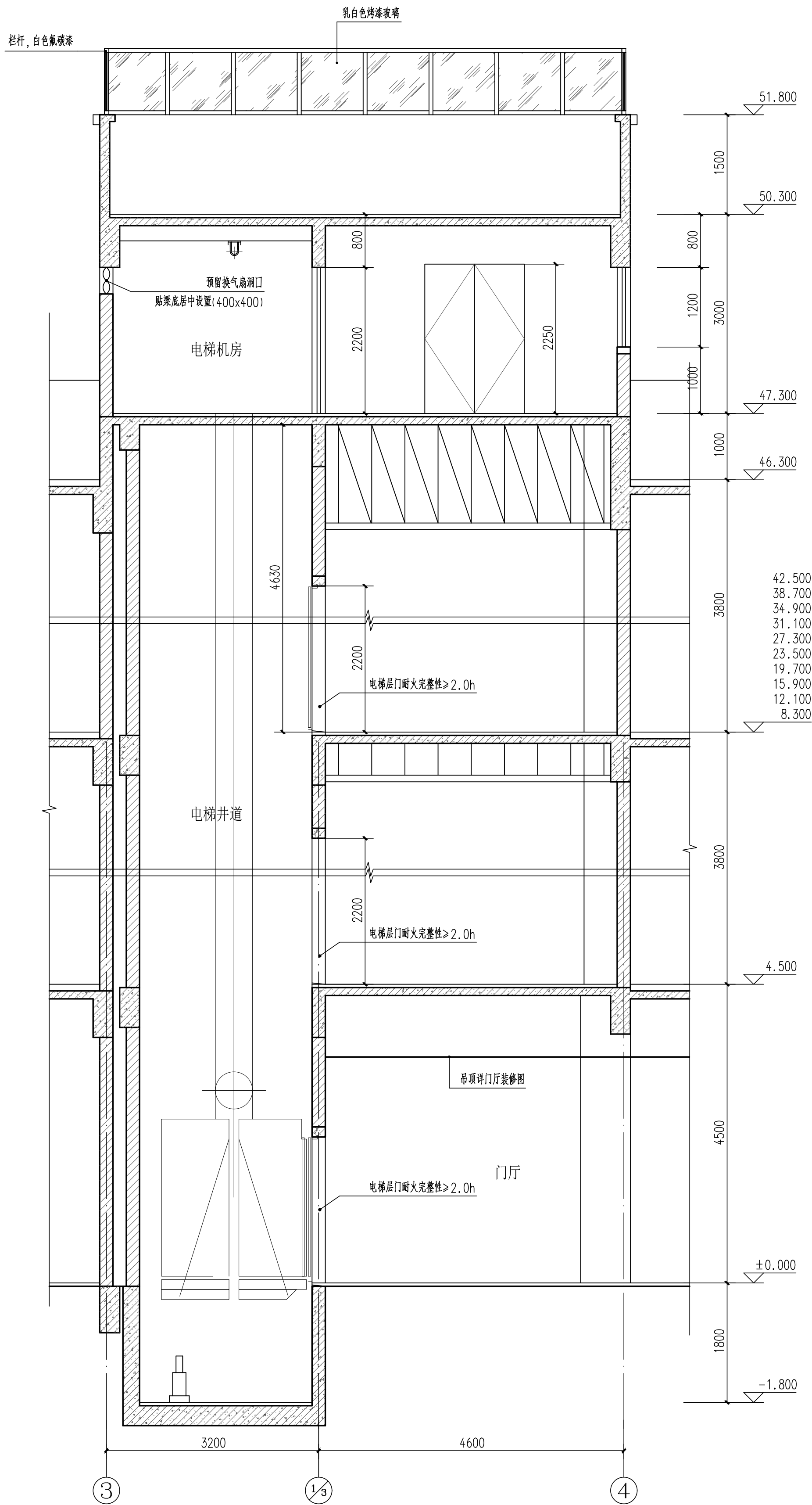
电梯C-C剖面图 1:50
