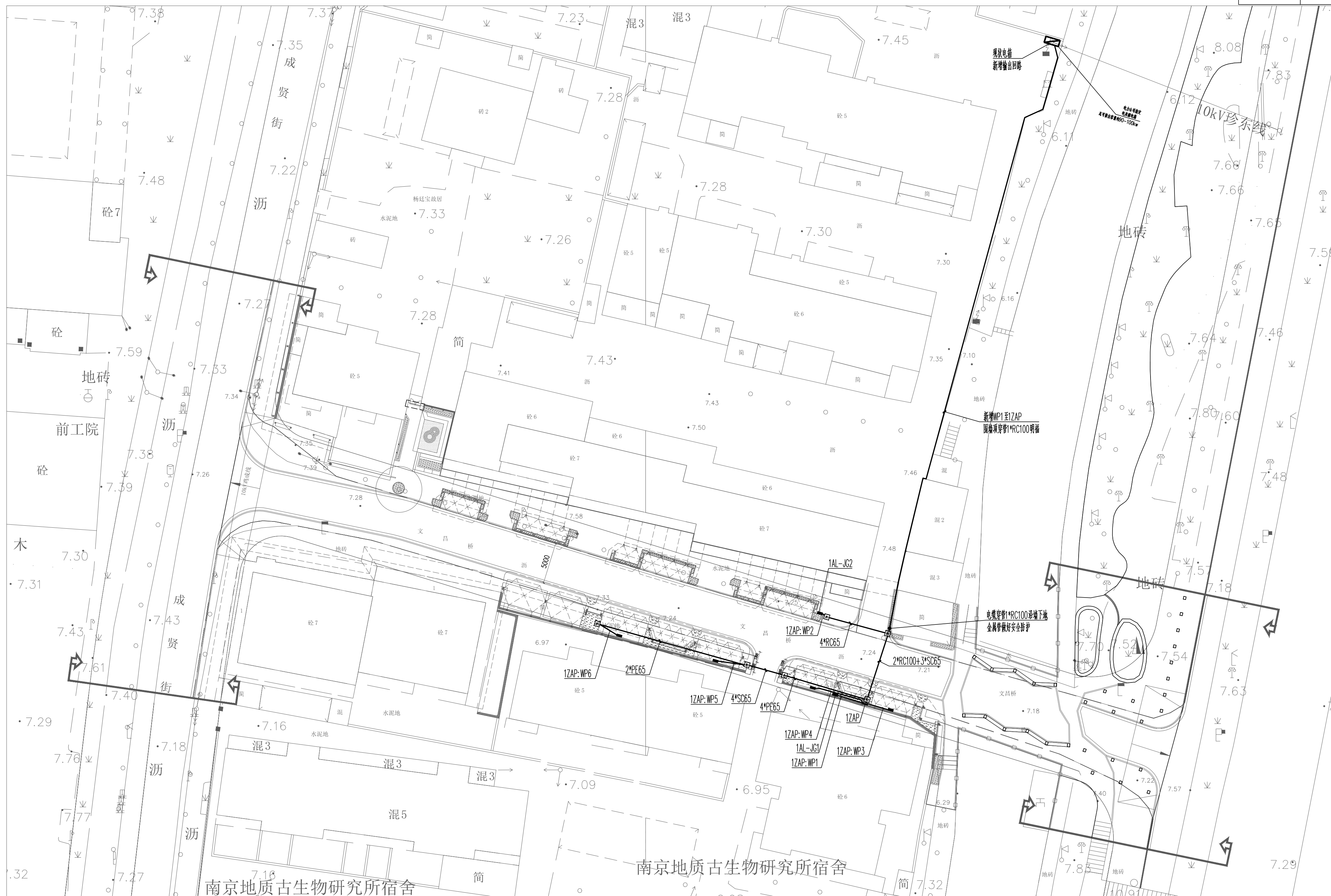
苏邑设计集团有限公司 SUYI DESIGN GROUP CO.,LTD 建设单位 南京市玄武区人民政府新街口街道办事处 图 名 景观配电平面图 项目负责人 审 定 校 核 专 业 电 气 版 次 01 项目名称 南京市玄武区文昌桥特色街巷改造工程 项目编号 260159901 设计阶段 施工图 专业负责人 审 核 设 计 图 号 DS-05 日 期 2026.07
