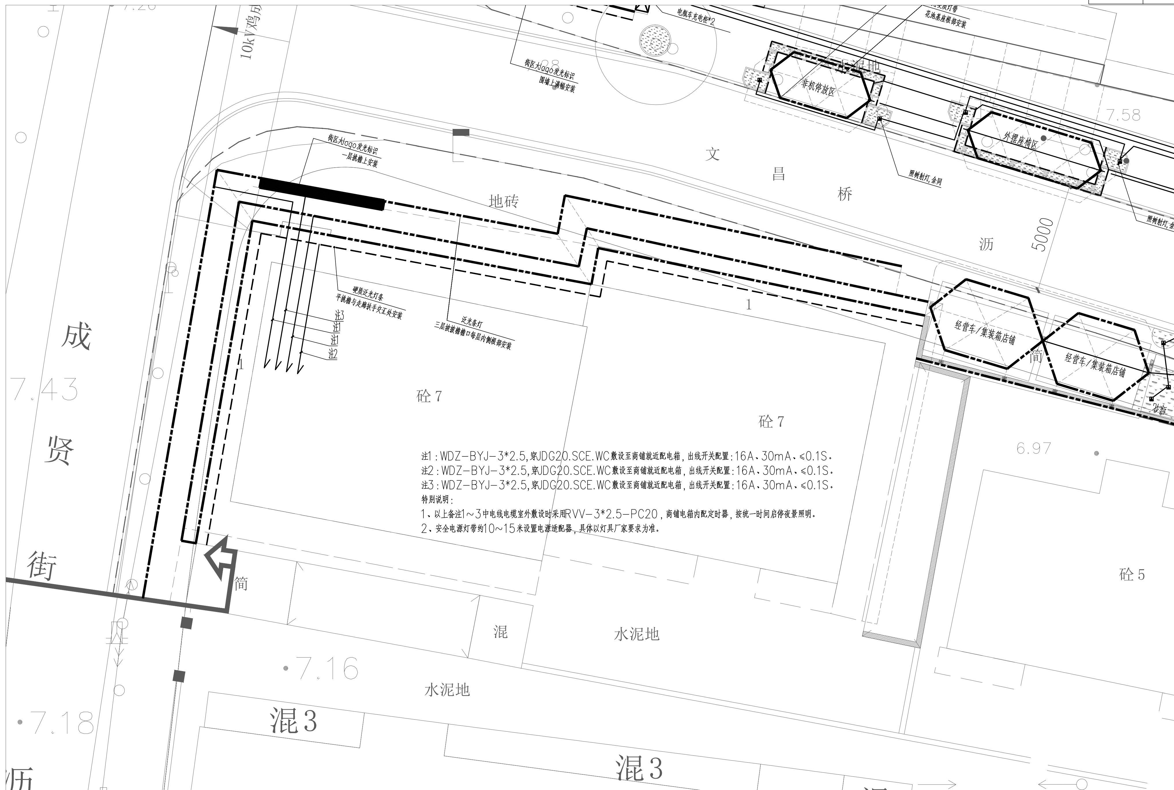
区域二景观照明平面图 1:100
