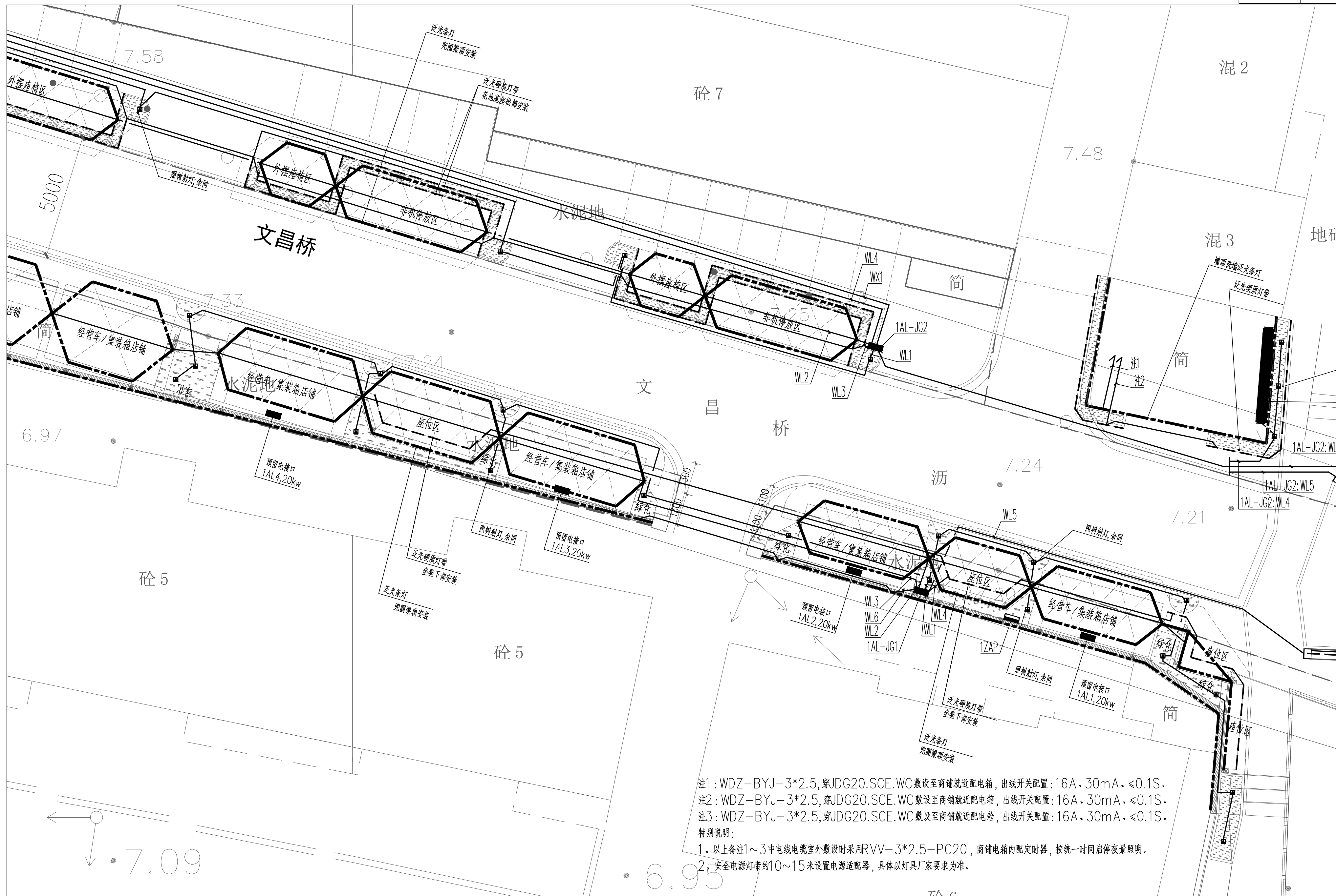
区域三景观照明平面图 1:100
