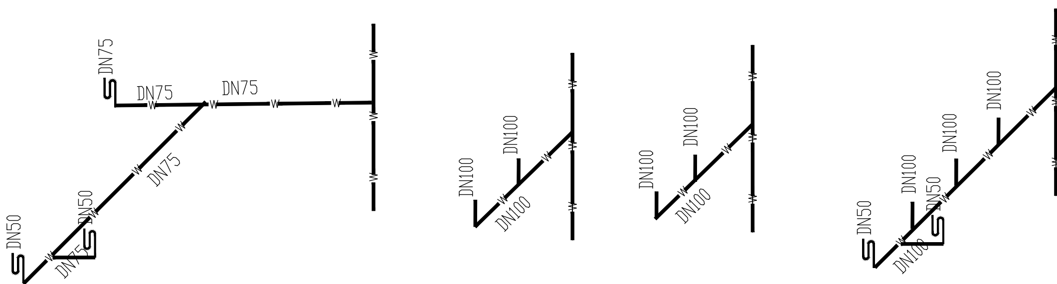
体育馆看台排水系统图
