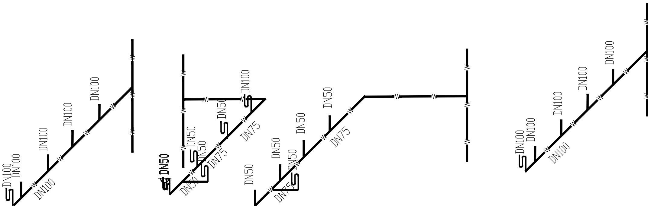
篮球馆1-2层排水系统图
