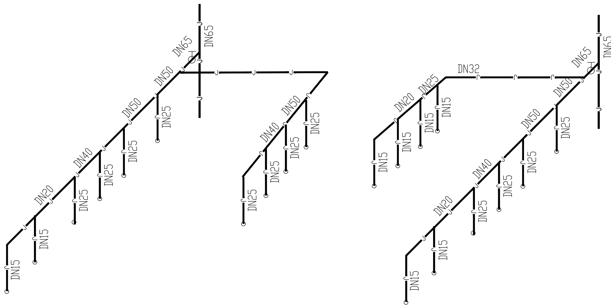
羽毛球馆1-3层给水系统图
