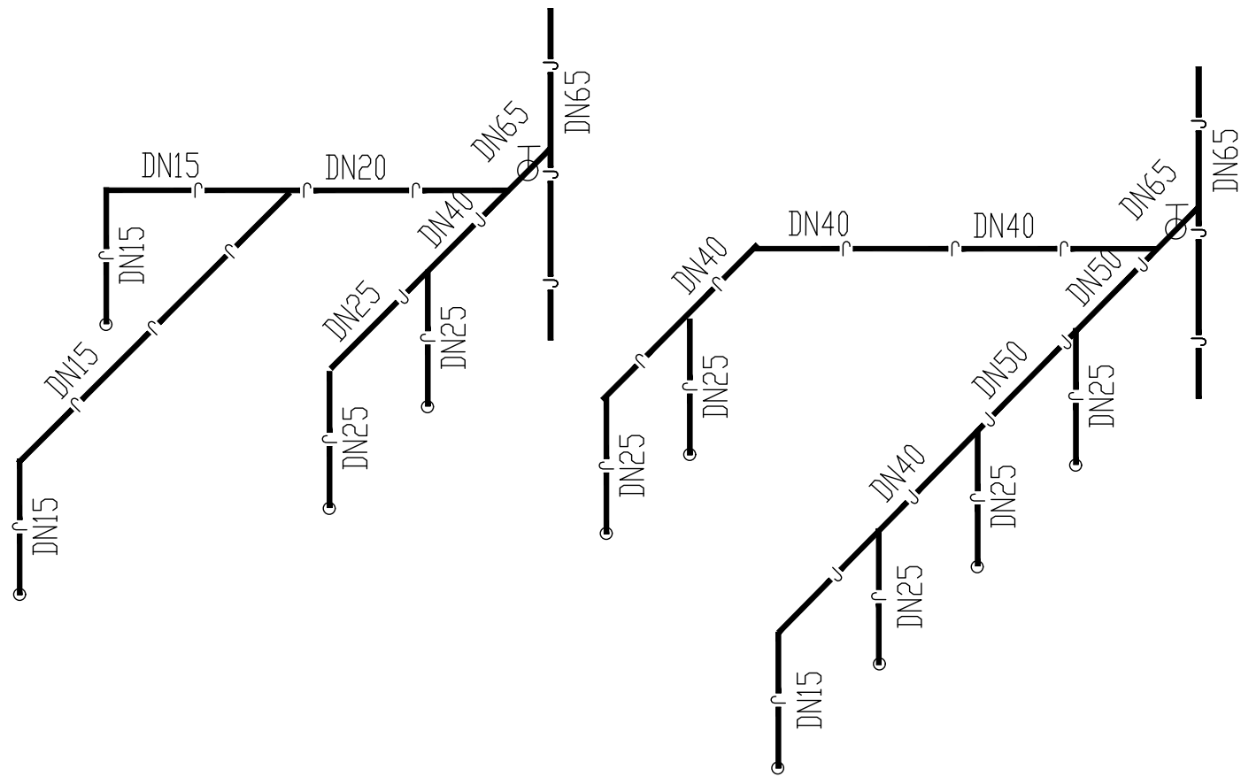
体育馆操场看台给水系统图
