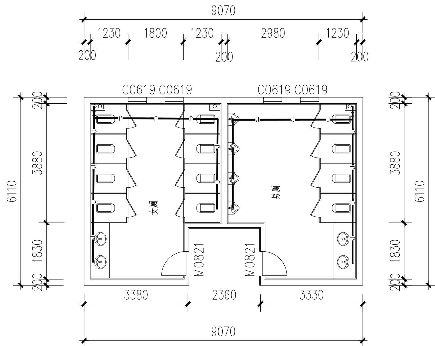
羽毛球馆1-3层给水平面布置图
