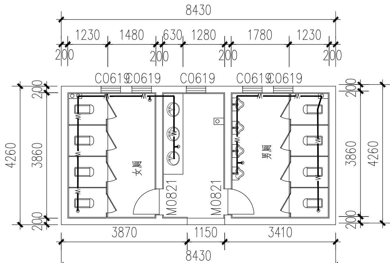
篮球馆1-2层排水平面图布置图
