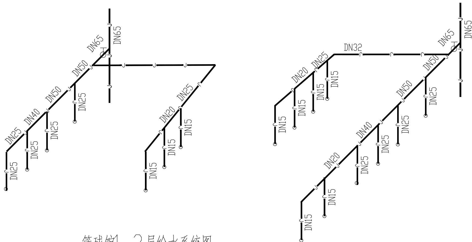
篮球馆1-2层给水系统图
