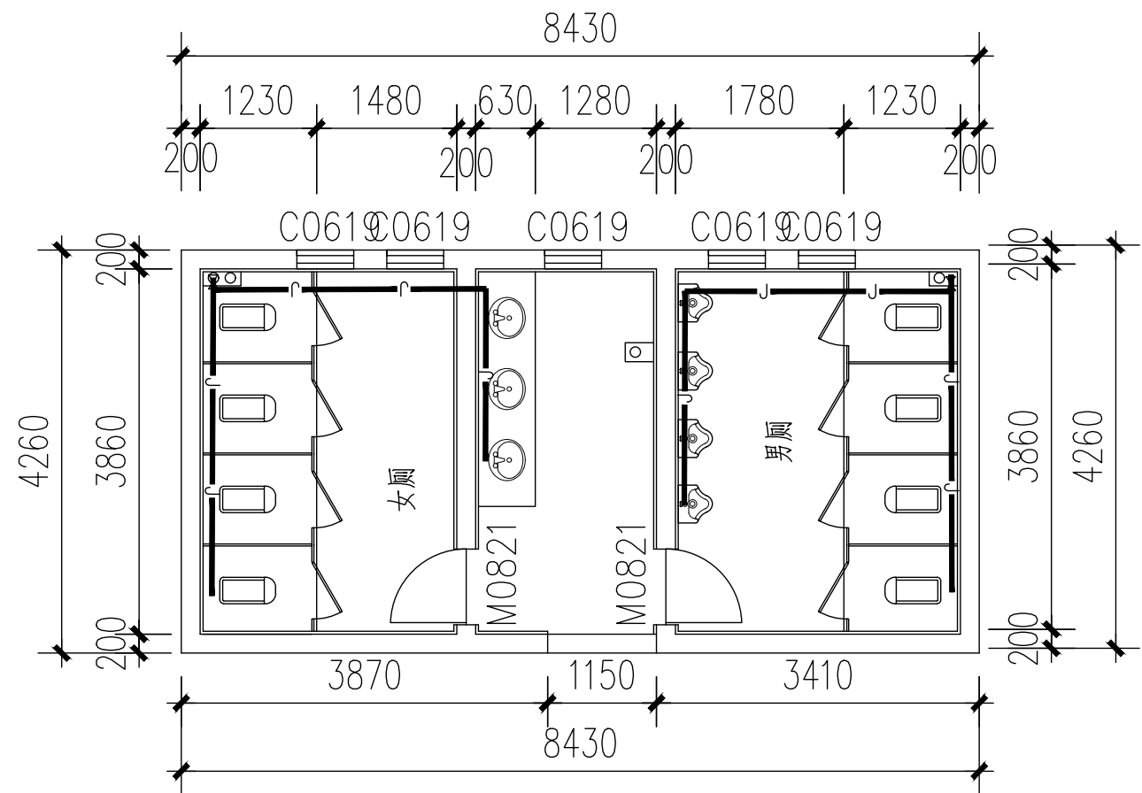
篮球馆1-2层给水平面布置图
