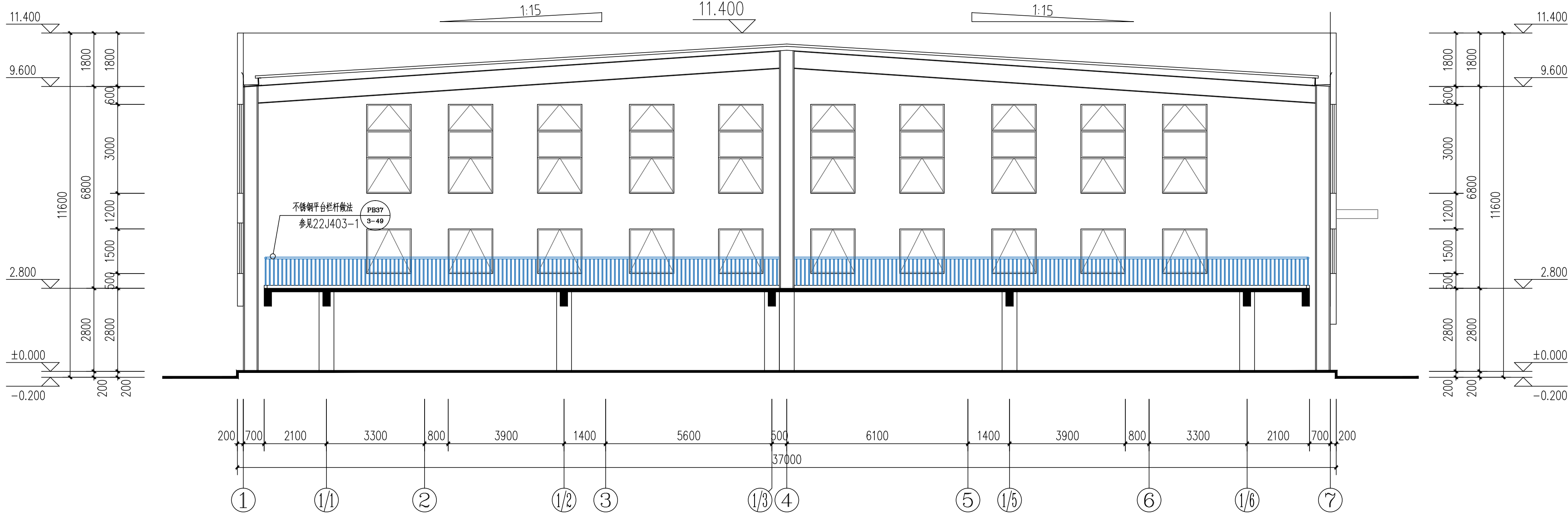
1-1剖面图 1:150
