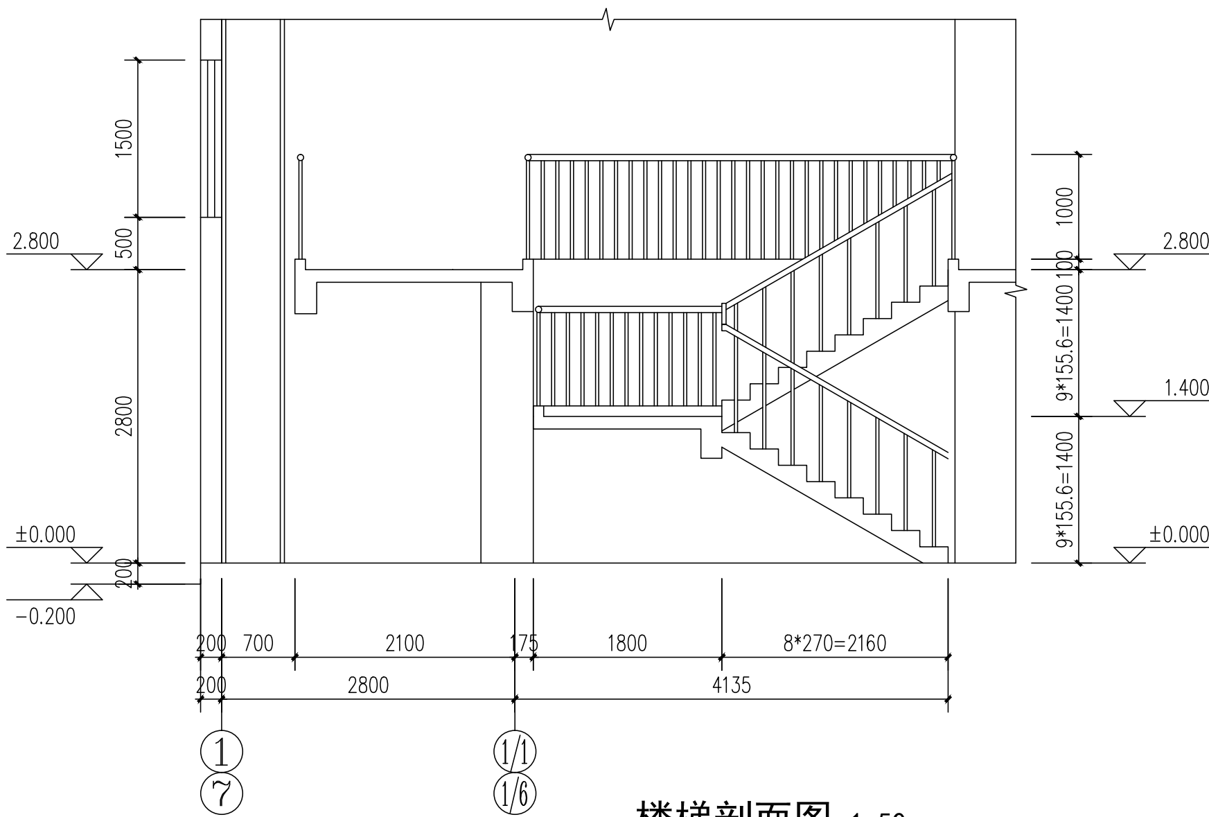
楼梯剖面图 1:50
