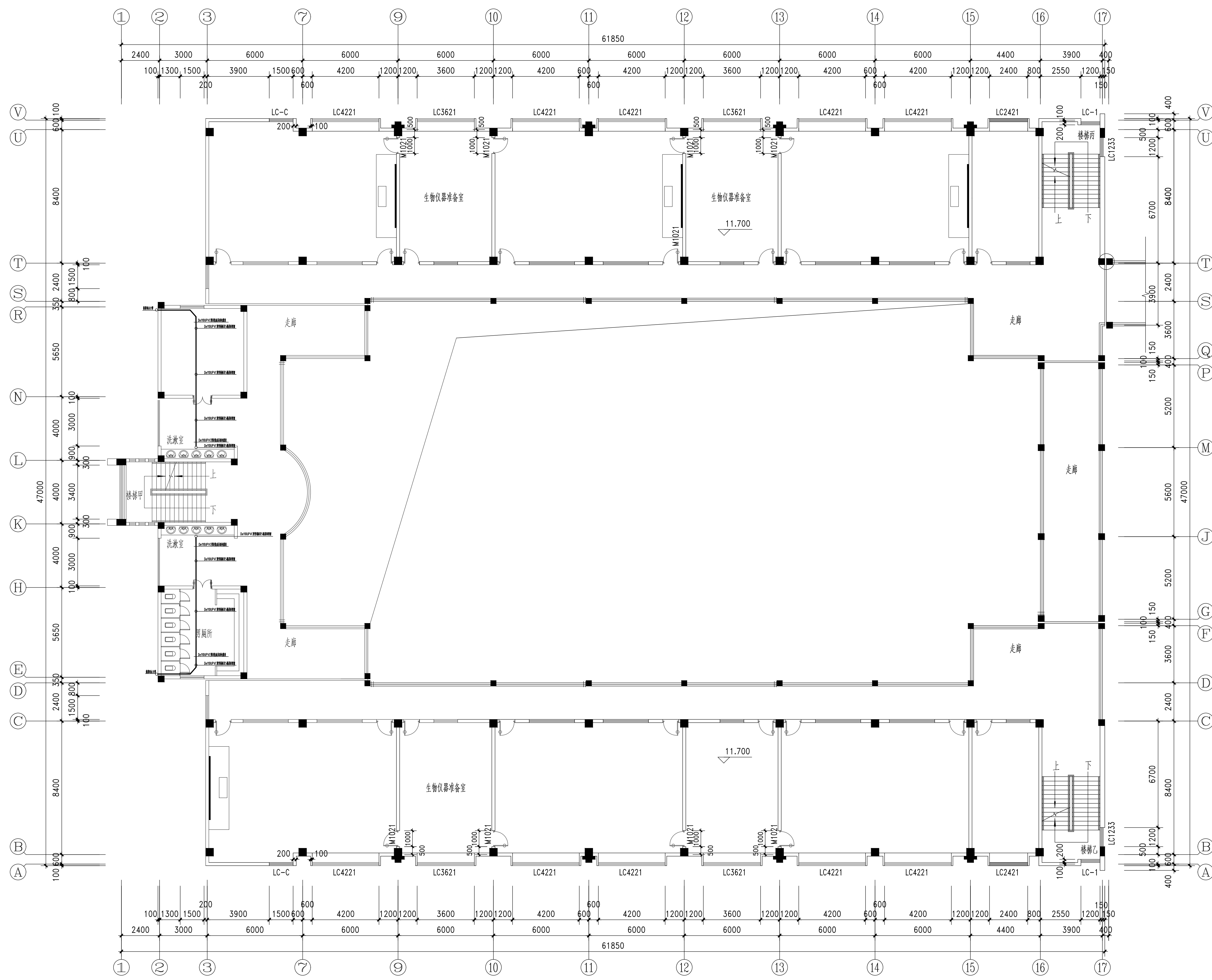
5号楼四楼顶内敷设五楼排水2 1:125
