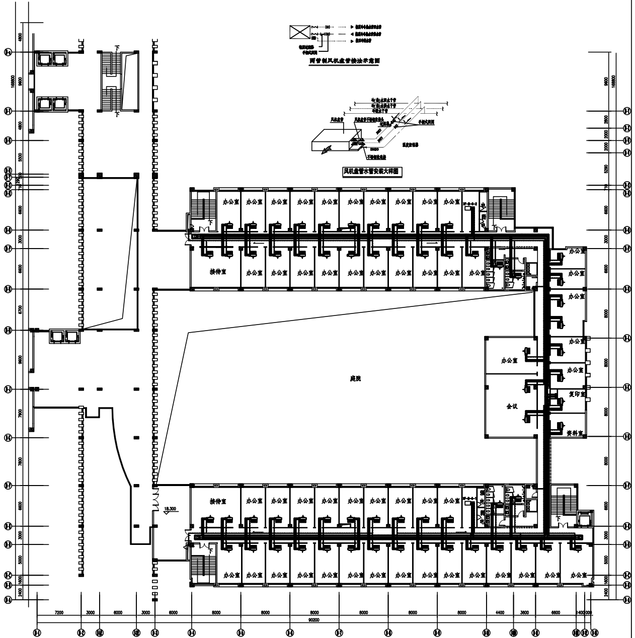
A区、B区六层空调系统平面图
