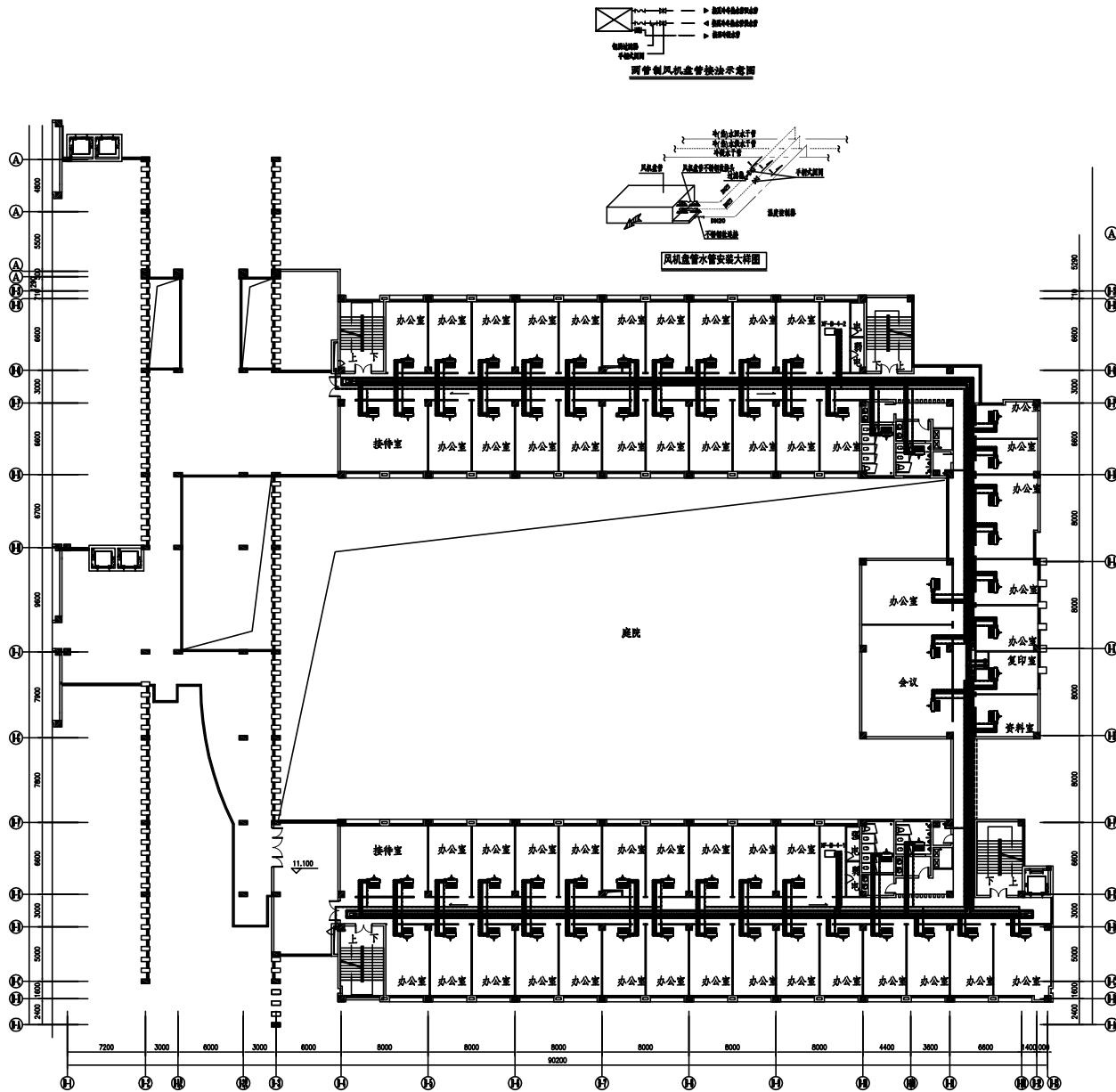
A区、B区四层空调水系统平面图
