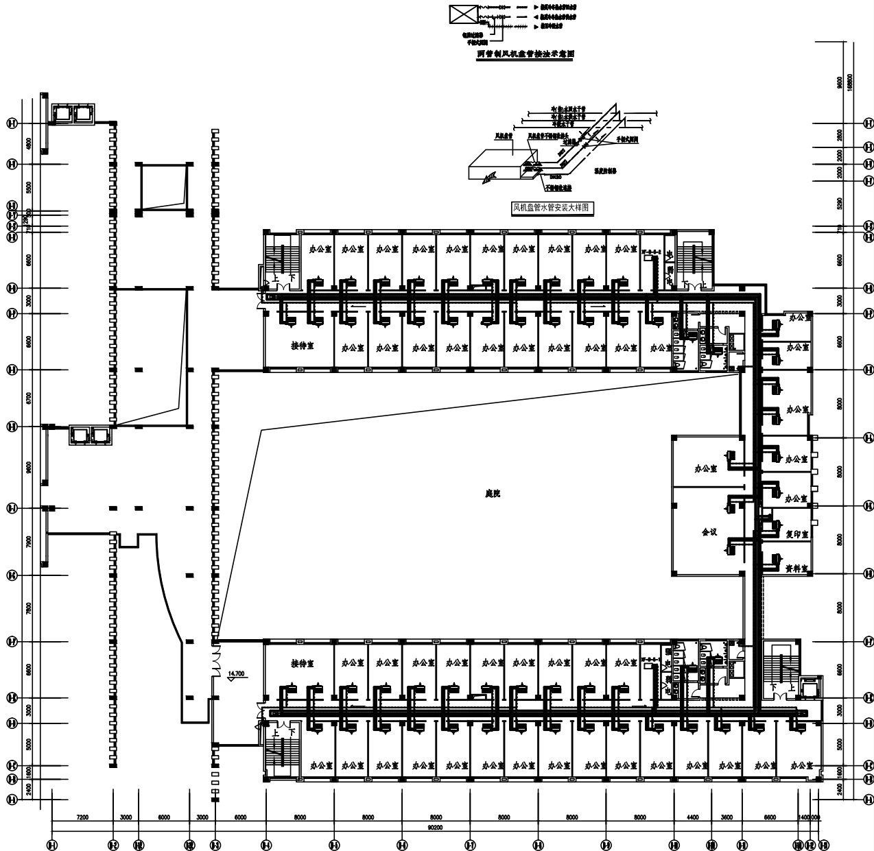
A区、B区五层空调水系统平面图
