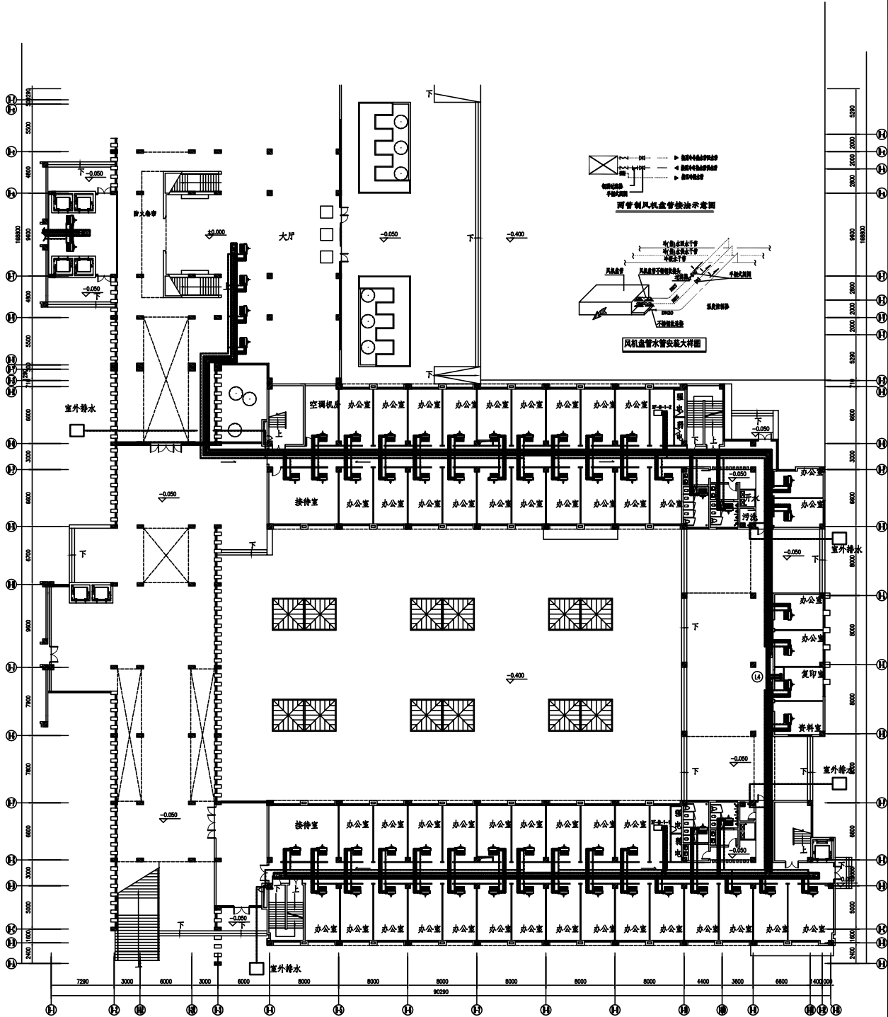
A区、B区一层空调水系统平面图 1:150 注：未标注的水支管管径均为DN25
