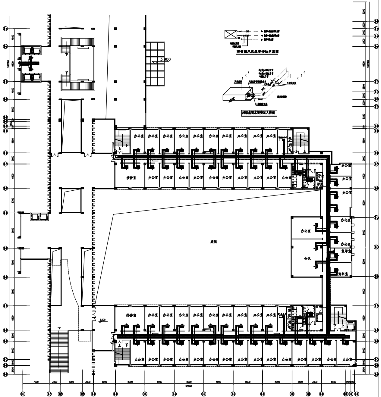
A区、B区二层空调水系统平面图
