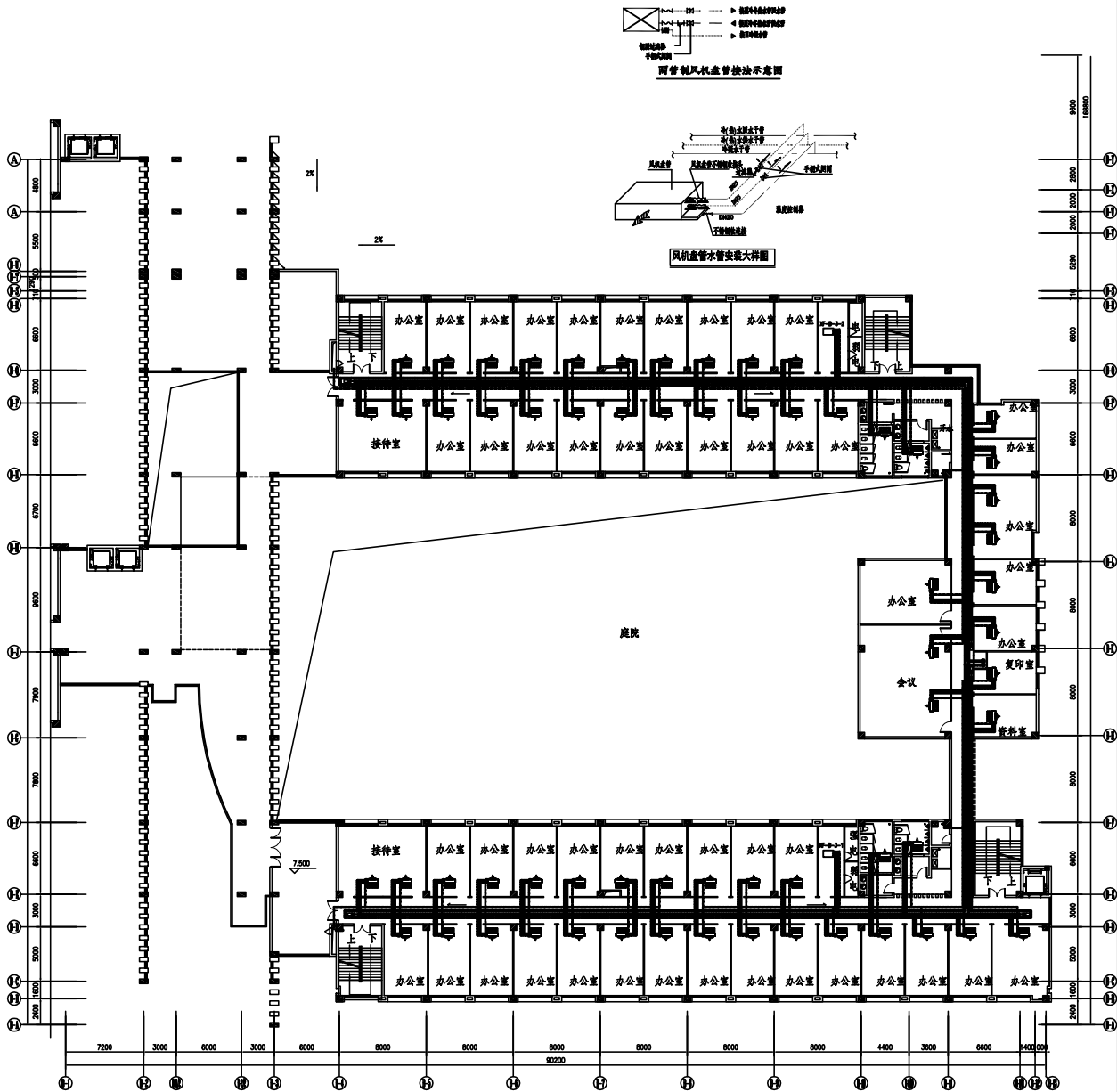
A区、B区三层空调水系统平面图
