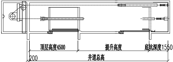
剖面图
