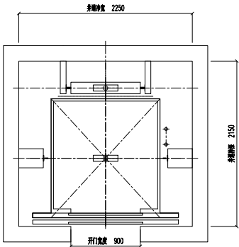
平面图
