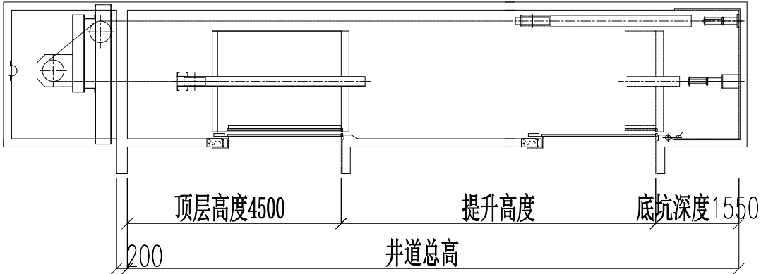
剖面图
