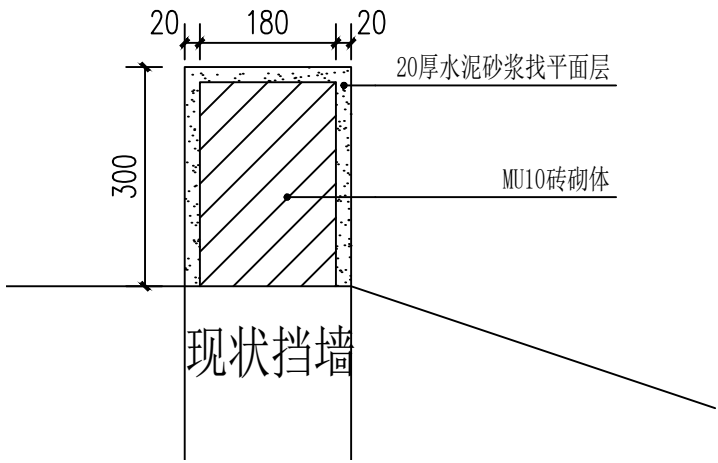
4 现状挡墙出新做法图 1:10
