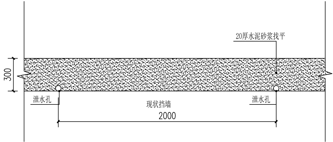
3 现状挡墙出新标准段立面图 1:5
