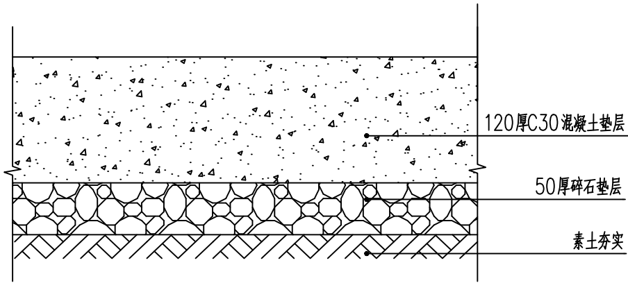
2 新建2.5米宽12公分厚C30混凝土主路 1:5
