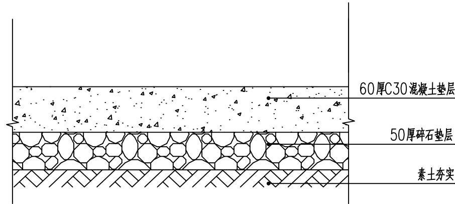
3 新建1.2米宽6公分厚C30混凝土支路 1:5
