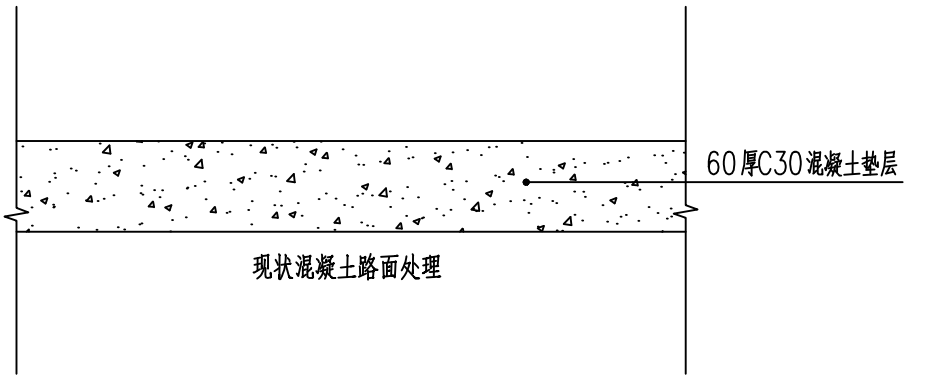
1 加铺6公分C30混凝土 1:5
