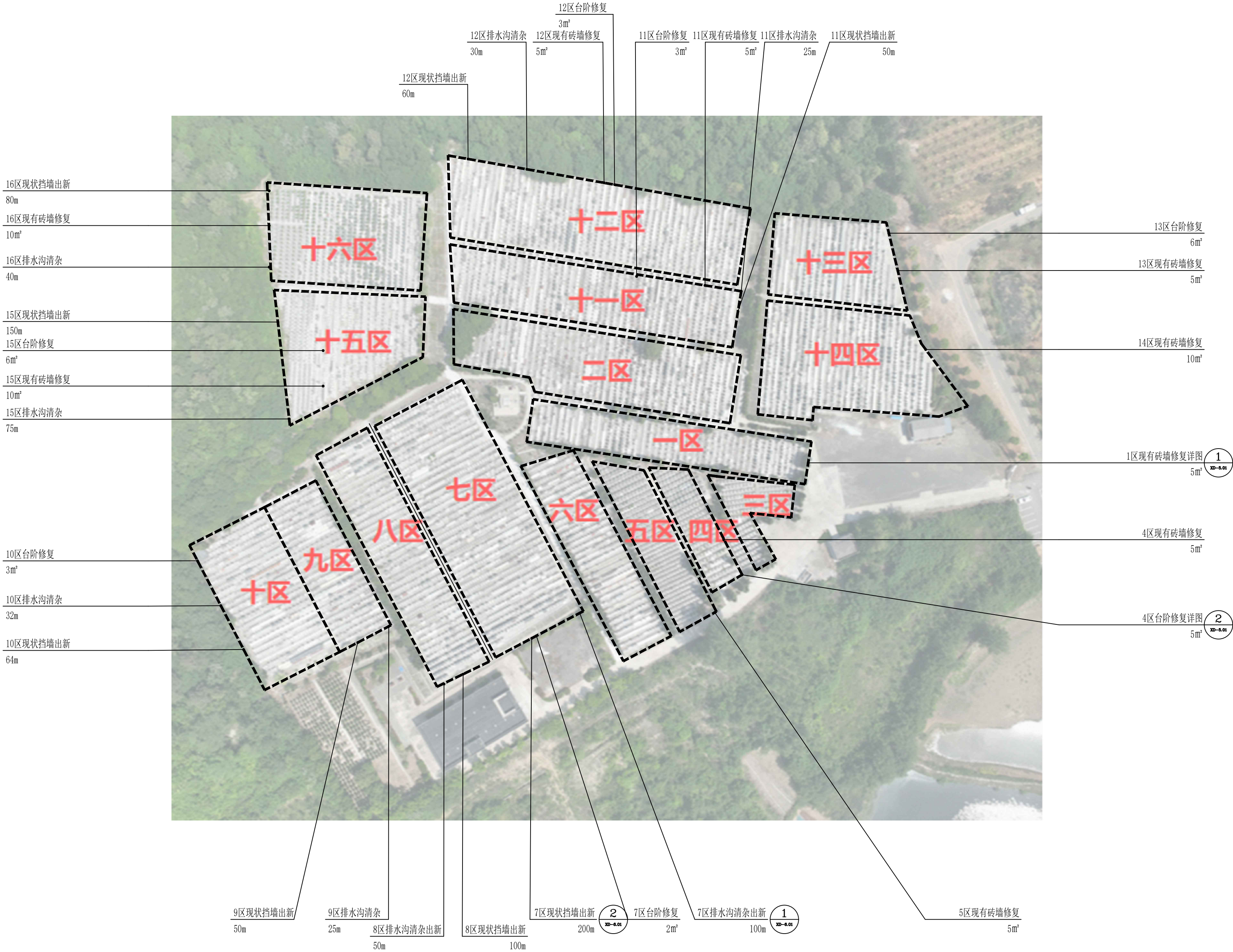
1 修复平面索引总图 1:1000 修复准确位置现场确定，经甲方同意后方可施工。
