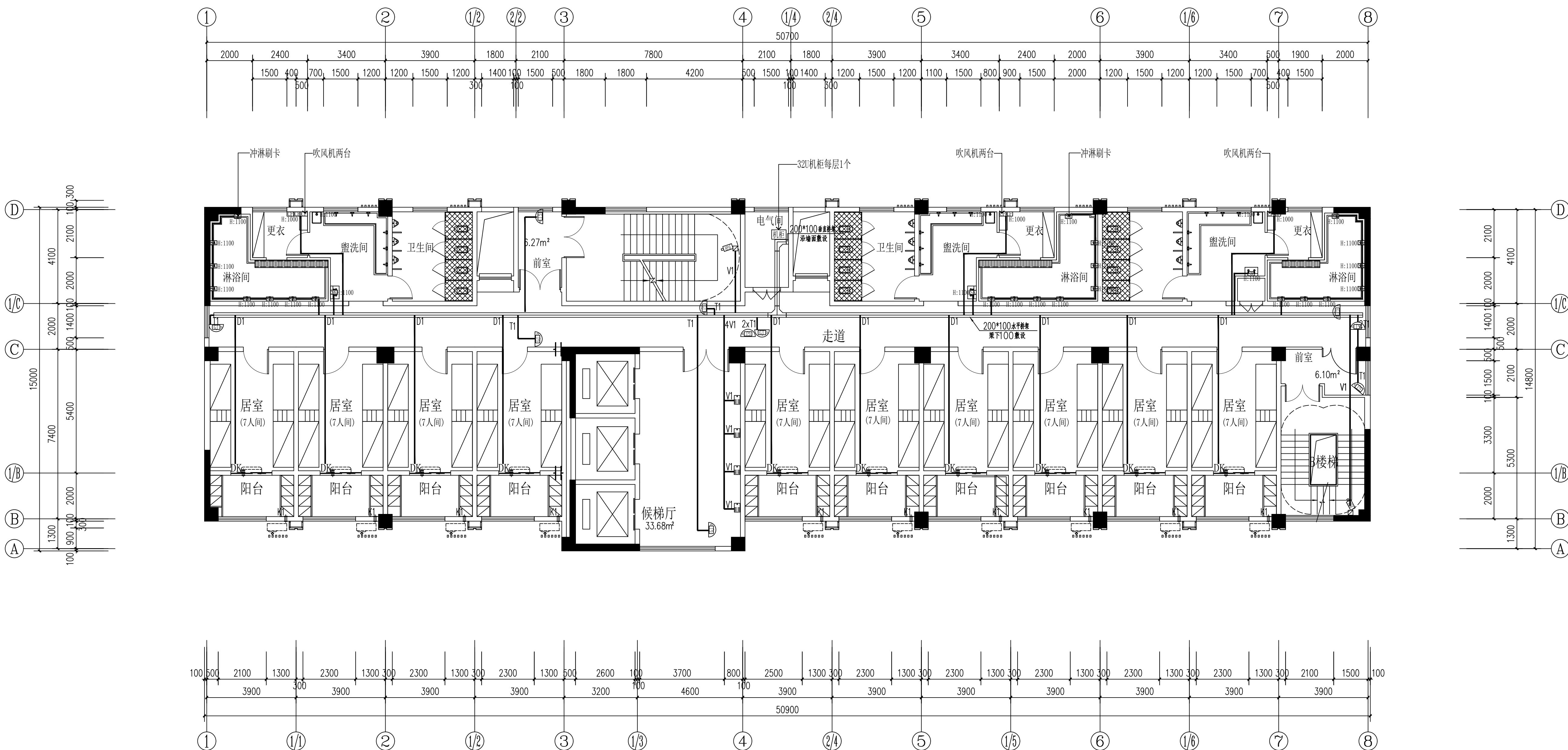
三、五、七、九、十一层监控平面图 1:100
