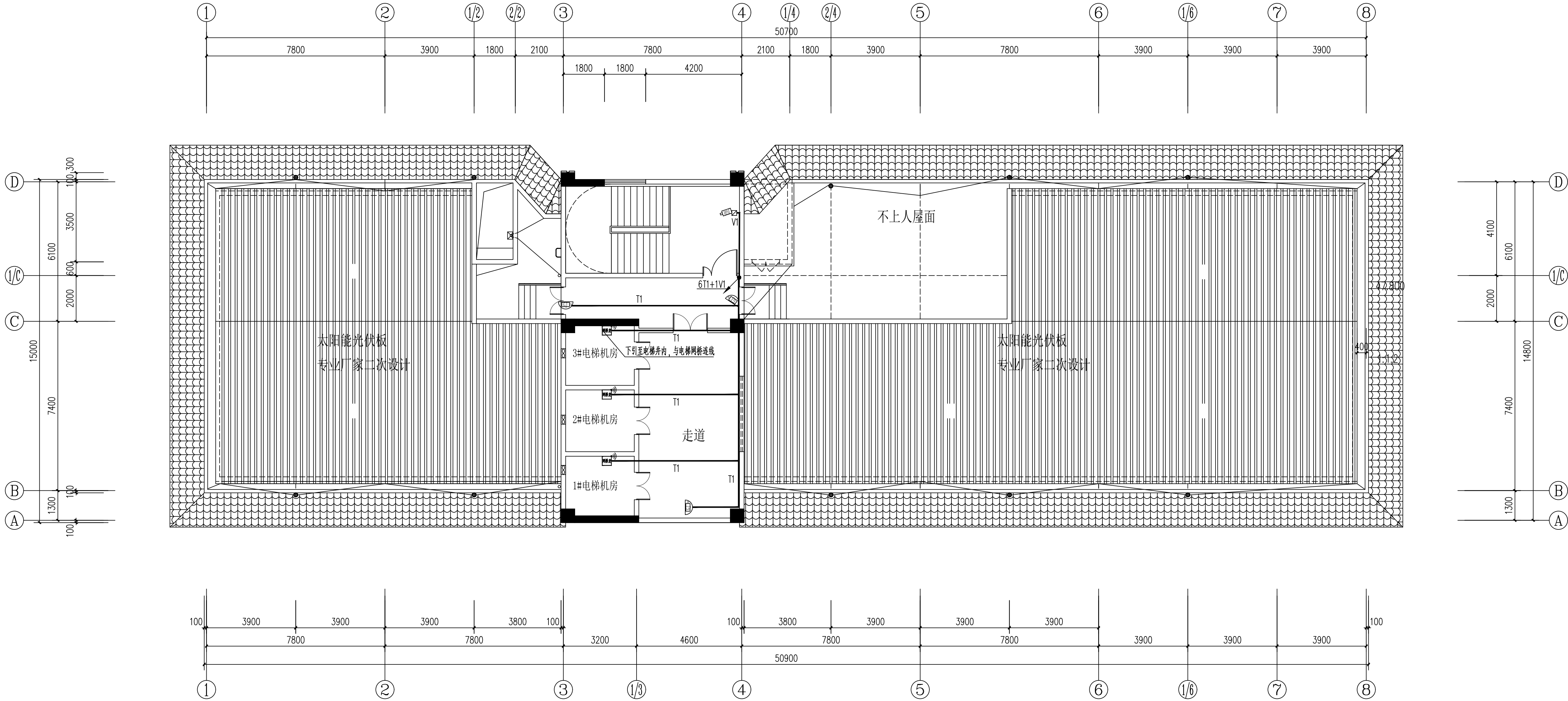
机房层监控平面图 1:100
