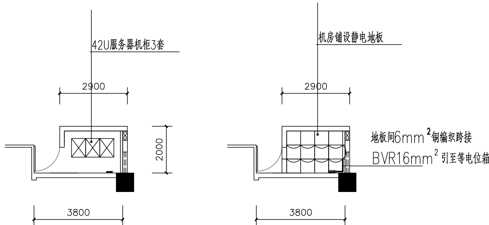
一层机房布置图
