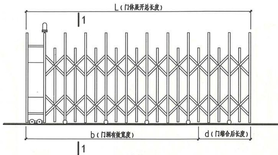
A型立面图
