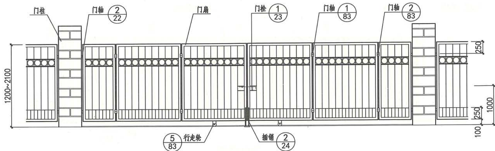
内立面图
