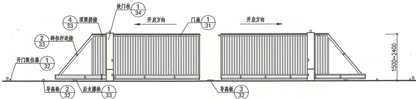
内立面图
