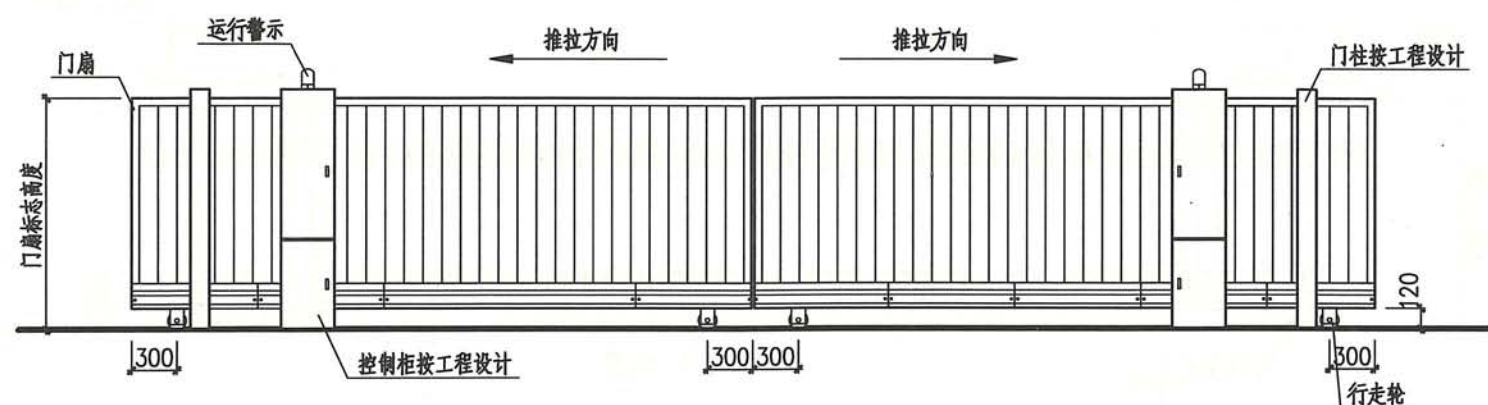
内立面图
