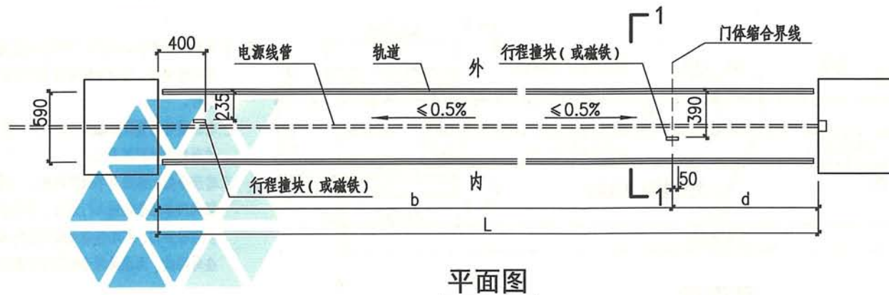
单向伸缩围墙大门明装式导轨、电源线管安装图
