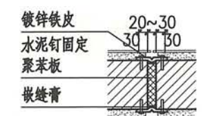
b 变形缝二
