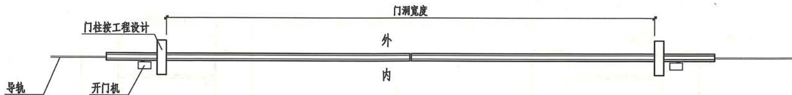
平面图
