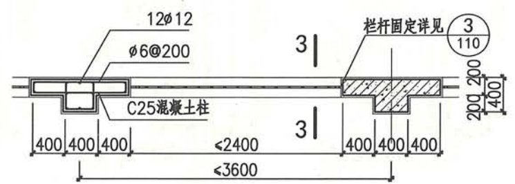
钢筋混凝土围墙平面
