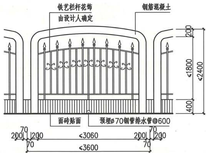
外立面图
