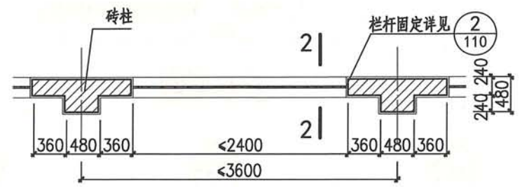
砖围墙平面
