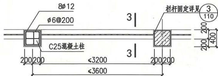
钢筋混凝土围墙平面
