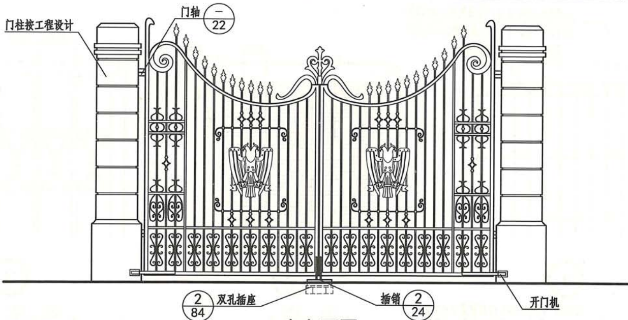
内立面图
