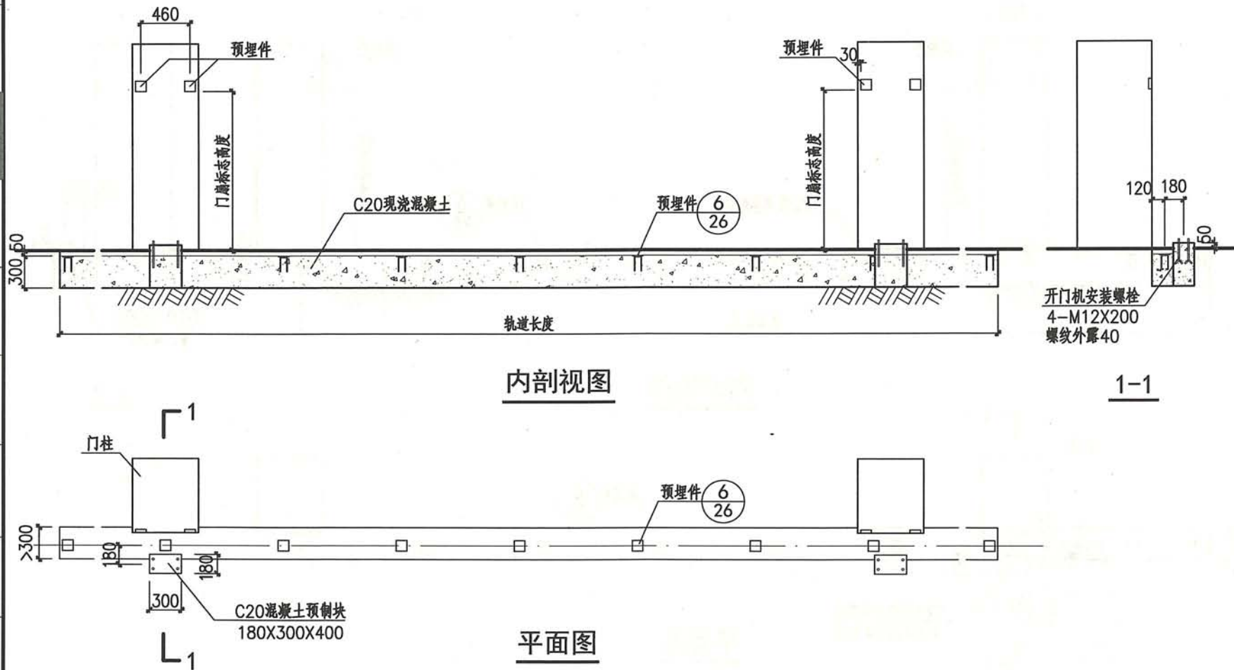
电动双向推拉围墙大门预埋件安装图
