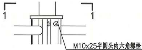
② 控制器连接件 与旋转门翼连接
