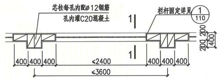
混凝土砌块围墙平面
