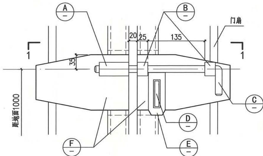
①大门门栓
