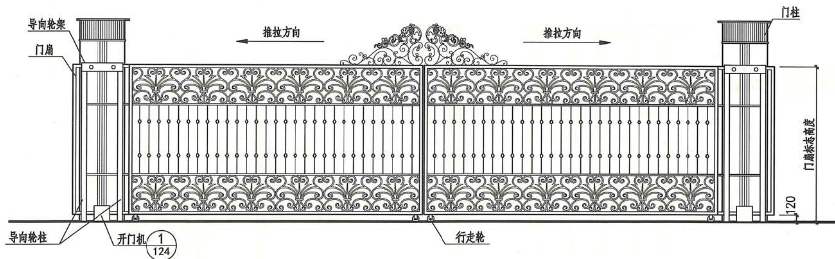
内立面图
