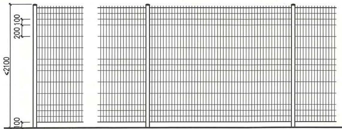
外立面图
