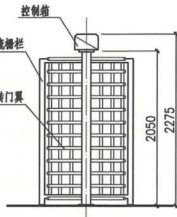
侧立面图
