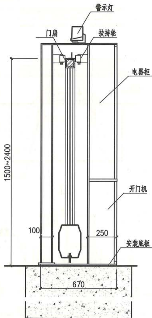
1-1
