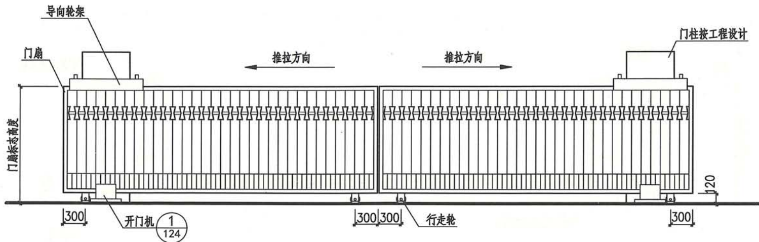
内立面图
