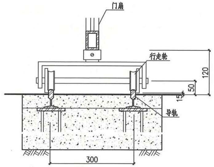
⑤ 行走轮
