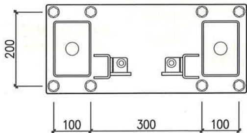
关门柱安装底板
