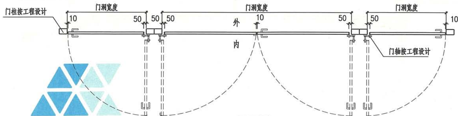
平面图
