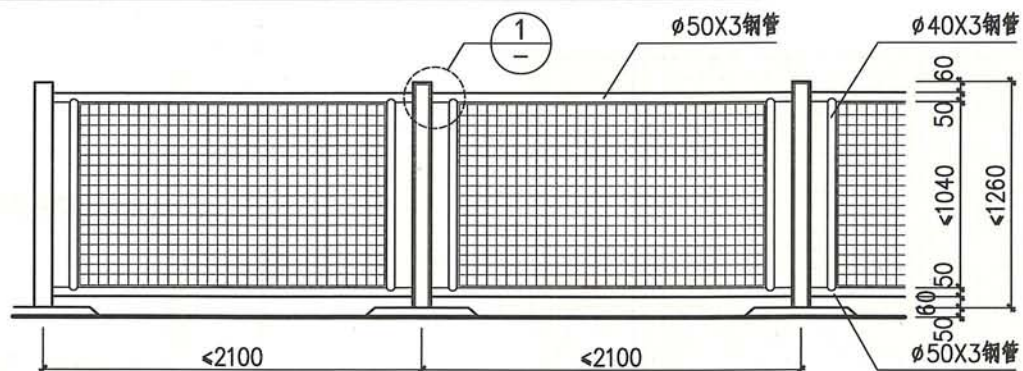
外立面图
