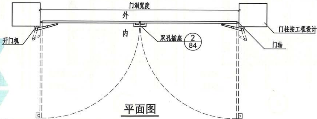
平开围墙大门平、立面图
