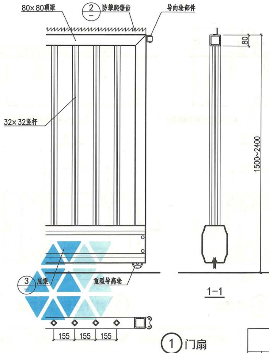
门扇、防攀越锯齿、底梁节点图
