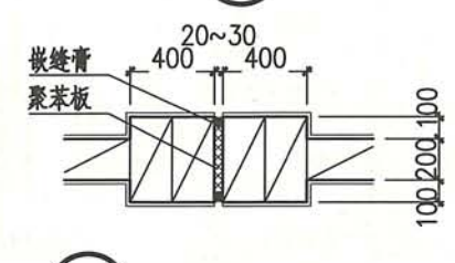
d 混凝土砌块墙变形缝
