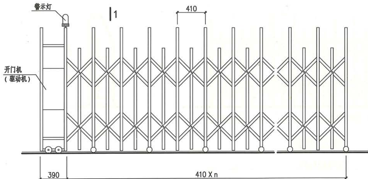
内立面图
