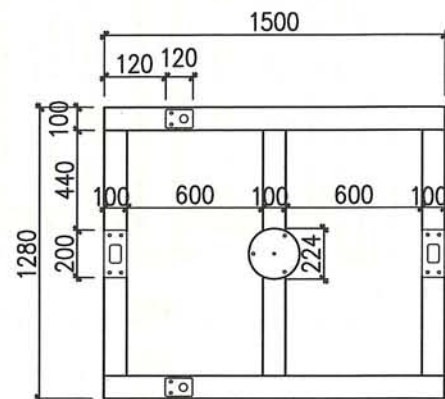
② 单通道旋转门预埋件
