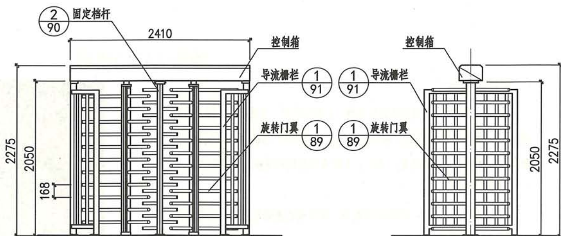
内立面图
