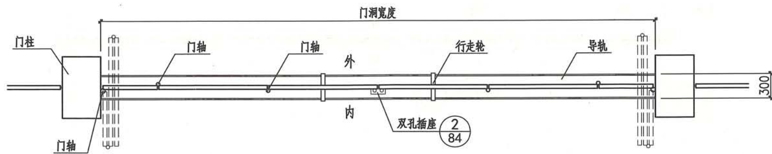
平面图
