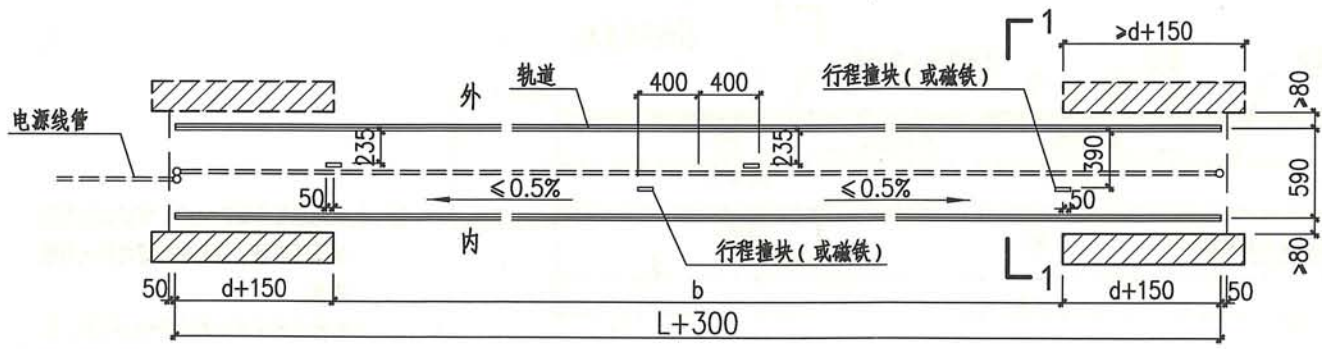
平面图
