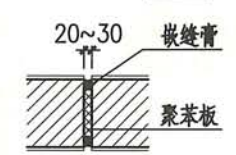
a 变形缝一
