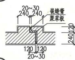
c 砖墙变形缝
