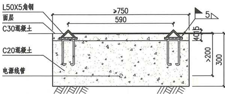
1-1 角钢导轨剖面图
