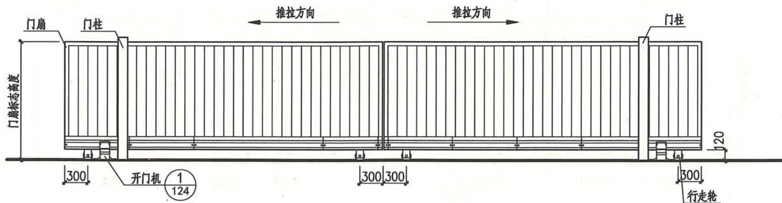
内立面图
