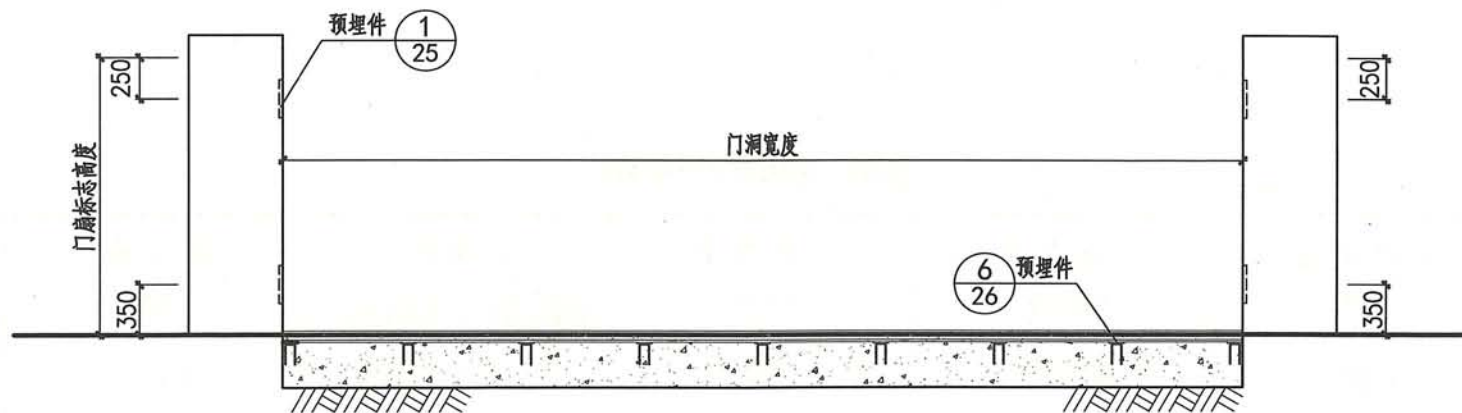
内立面图
