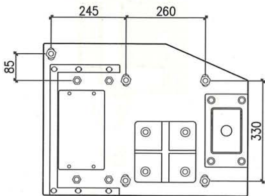
扶门柱安装底板
