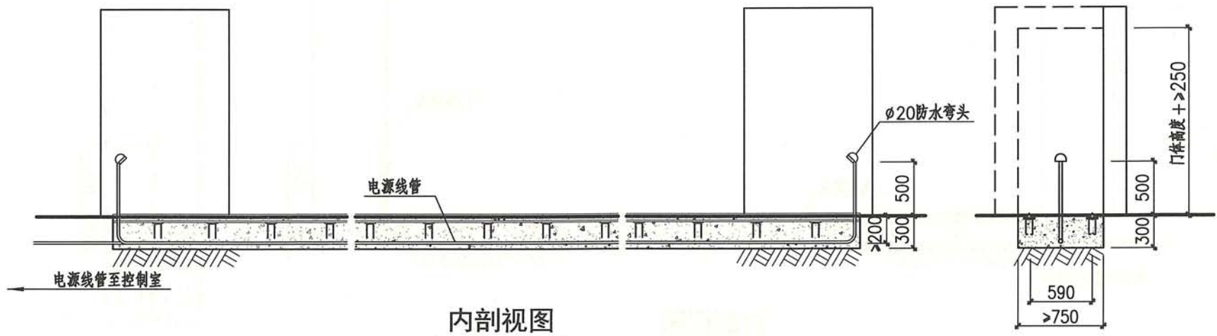
1-1
