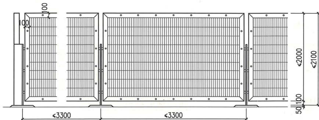
外立面图
