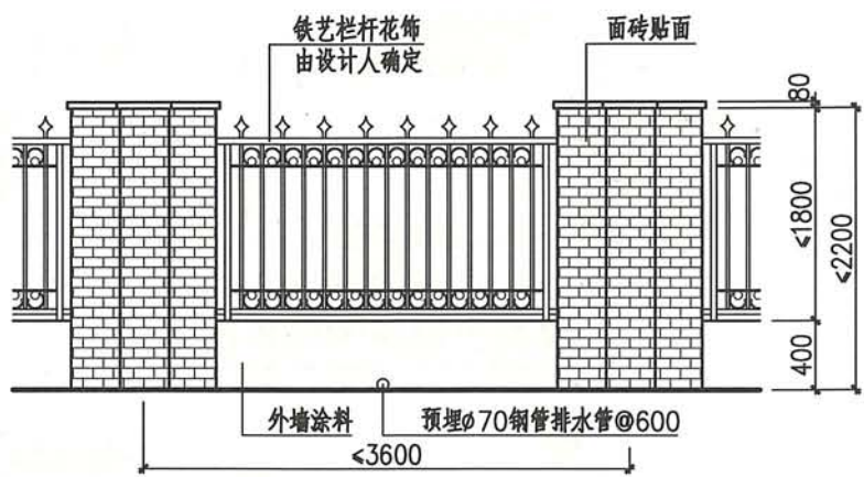
外立面图
