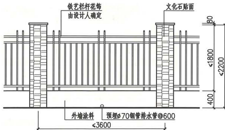
外立面图
