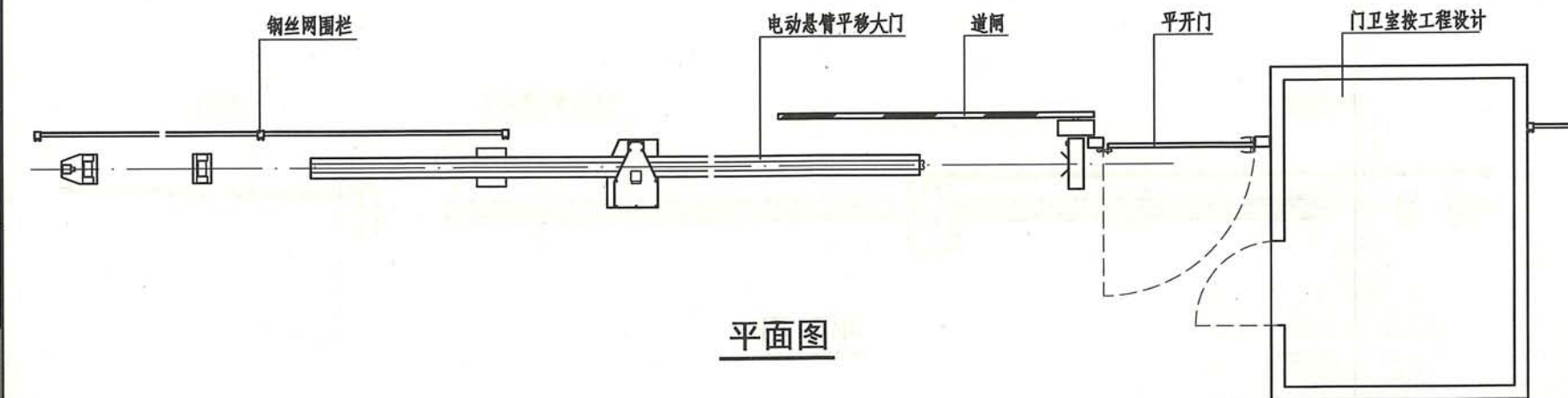
大门组合形式
