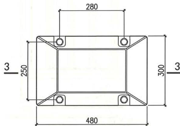
③ 对开悬臂门导高板
