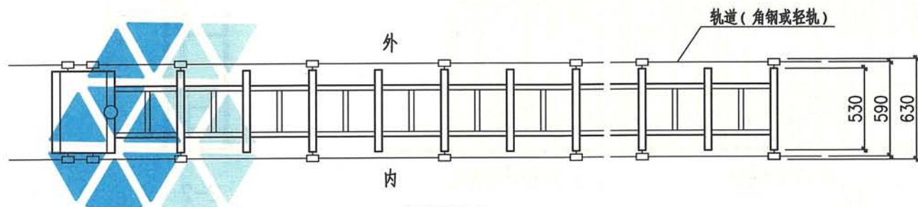
平面图
