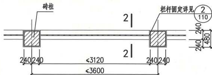
砖围墙平面
