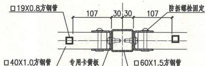
平面图
