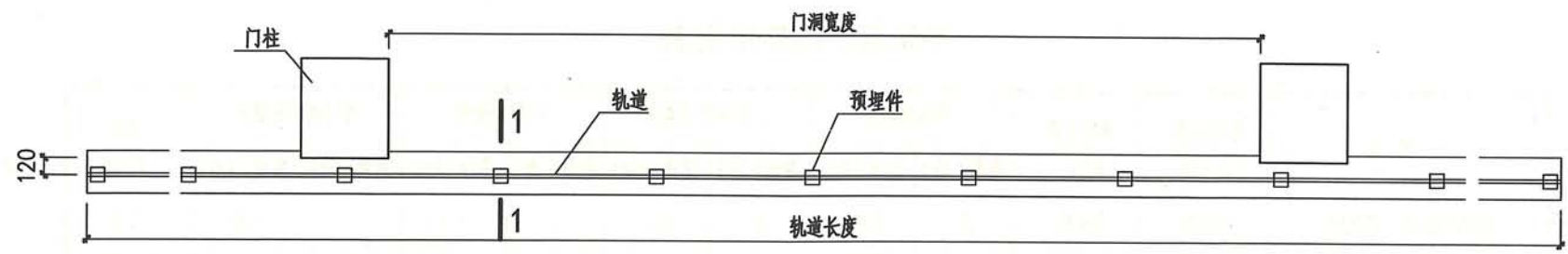
双向推拉轨道平面图
