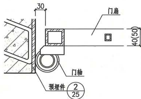
③ 门扇与柱边连接
