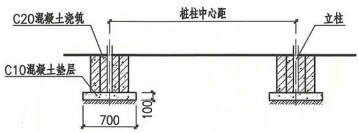
钢筋混凝土独立基础内剖视图
