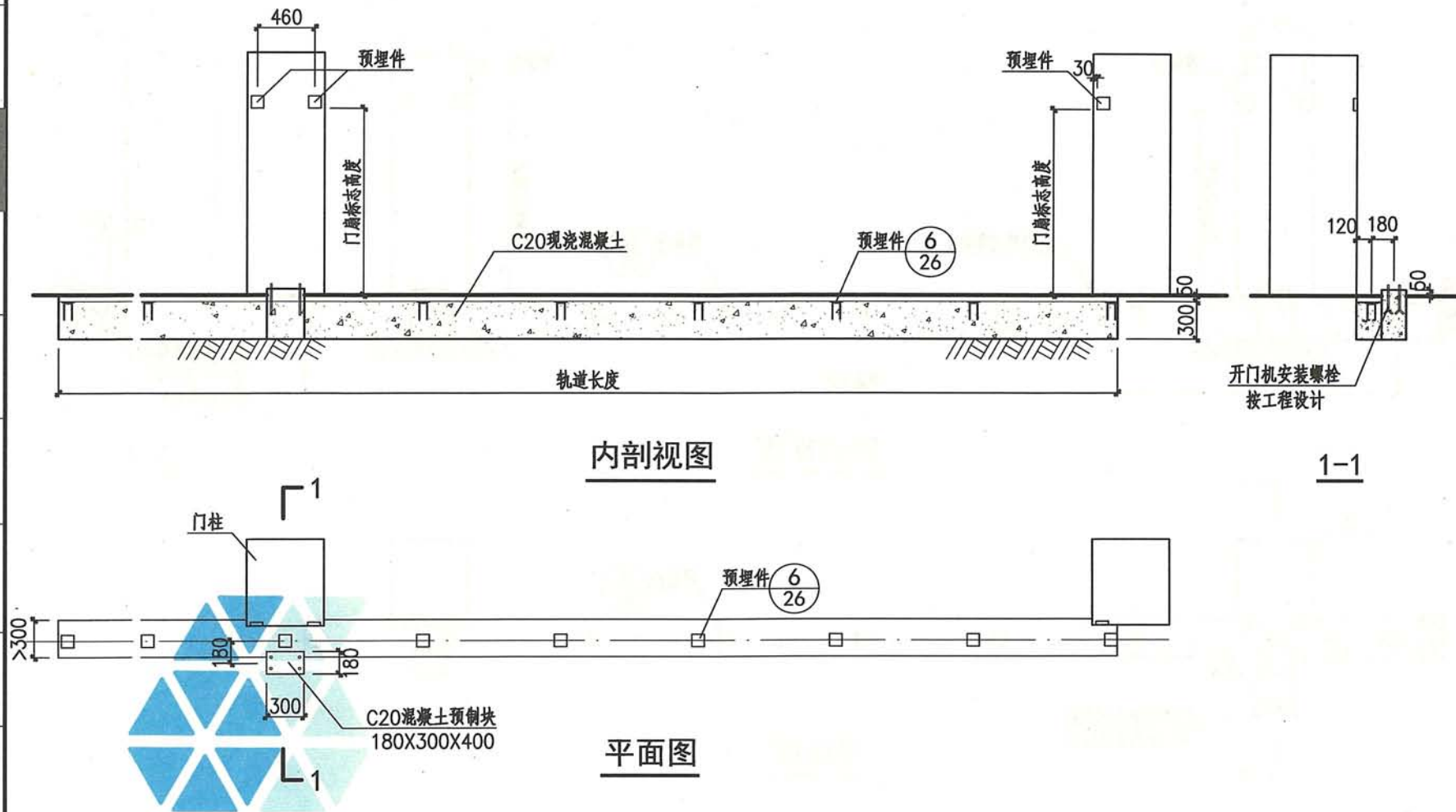
电动单向推拉围墙大门预埋件安装图
