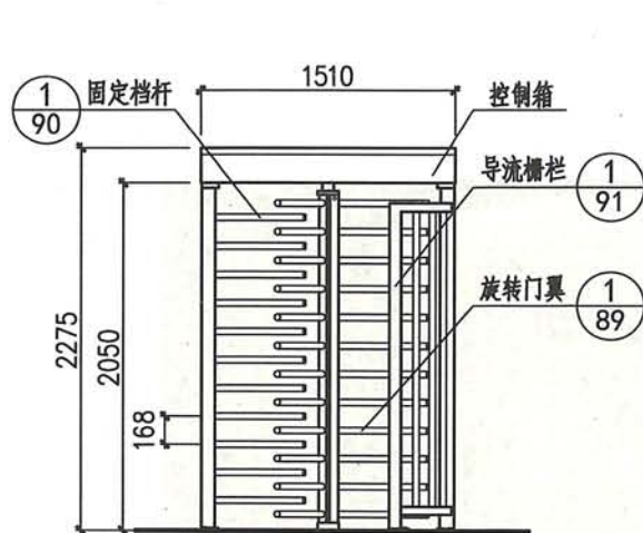
内立面图
