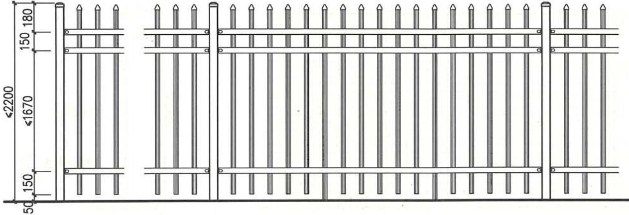
外立面图
