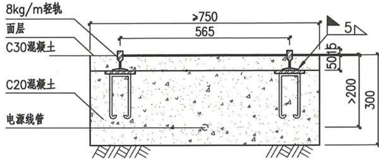
2-2 轻轨导轨剖面图
