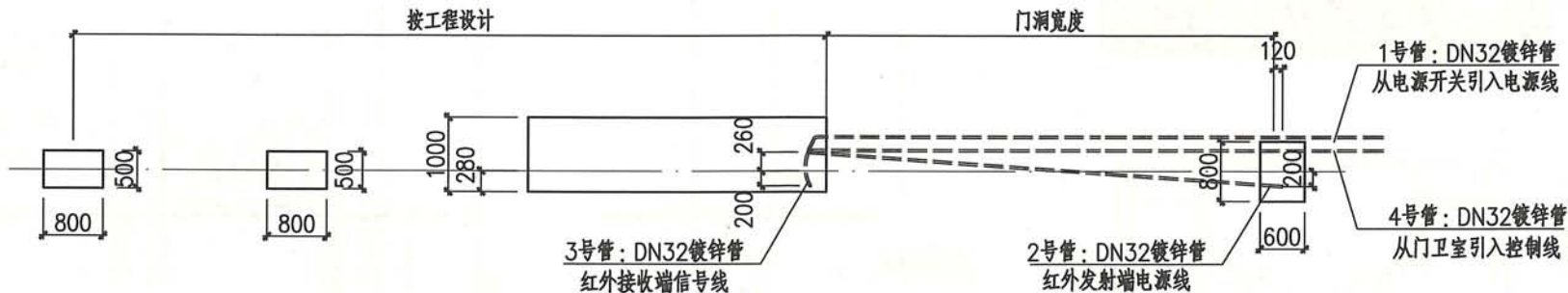
平面图
