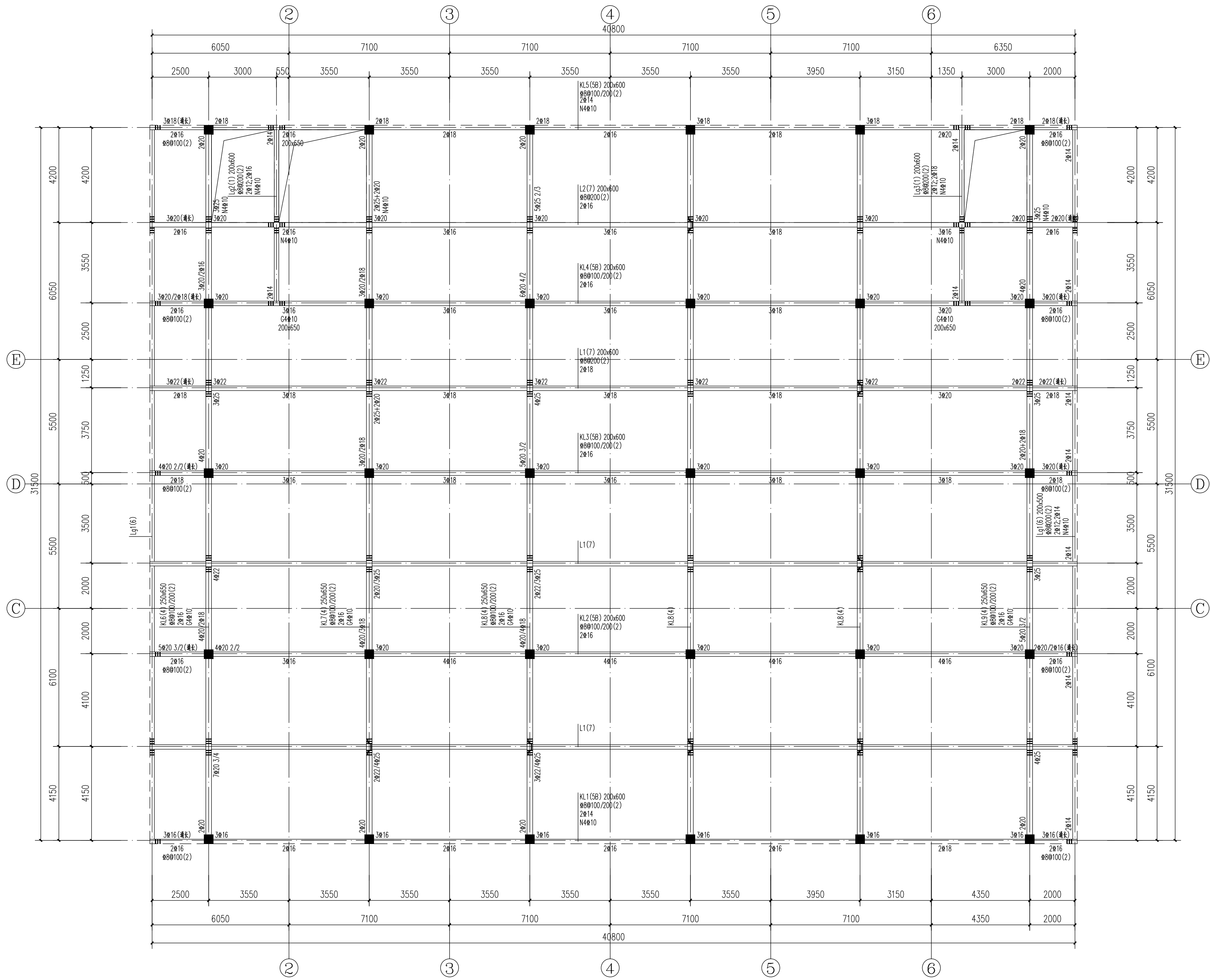
标高2.770楼面梁配筋图
