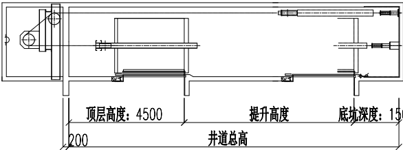
剖面图
