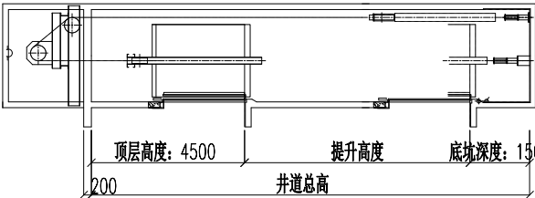
剖面图
