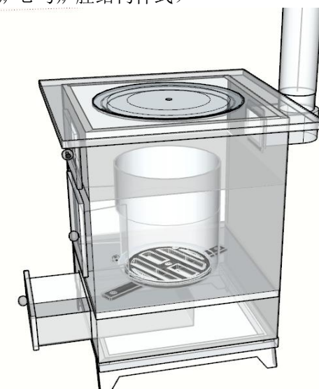
(图2 炉芯与炉膛结构样式)
