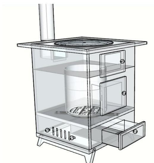
(图3 炉芯内部结构)
