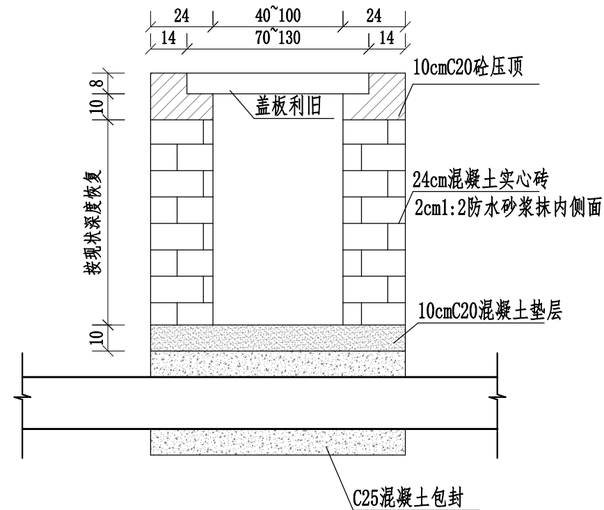
B-B剖面图
