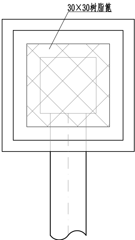
砖砌方井平面图
