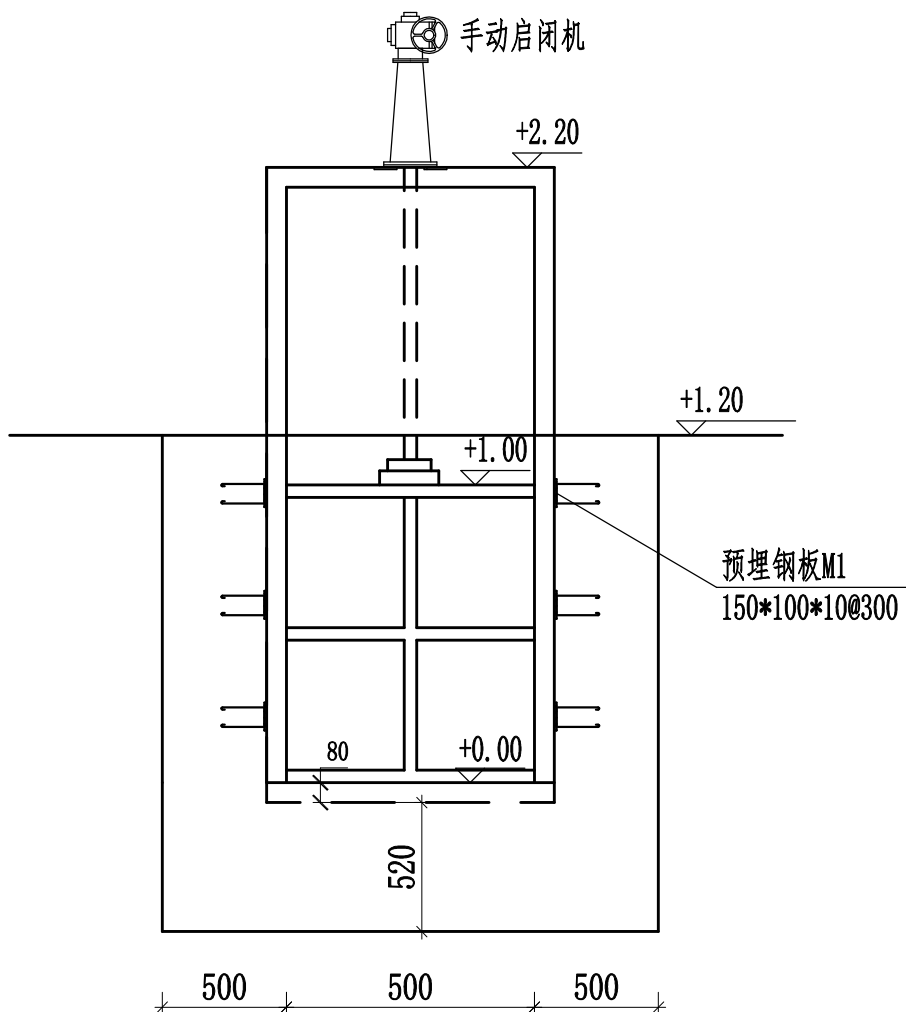
沟渠闸门立面图
