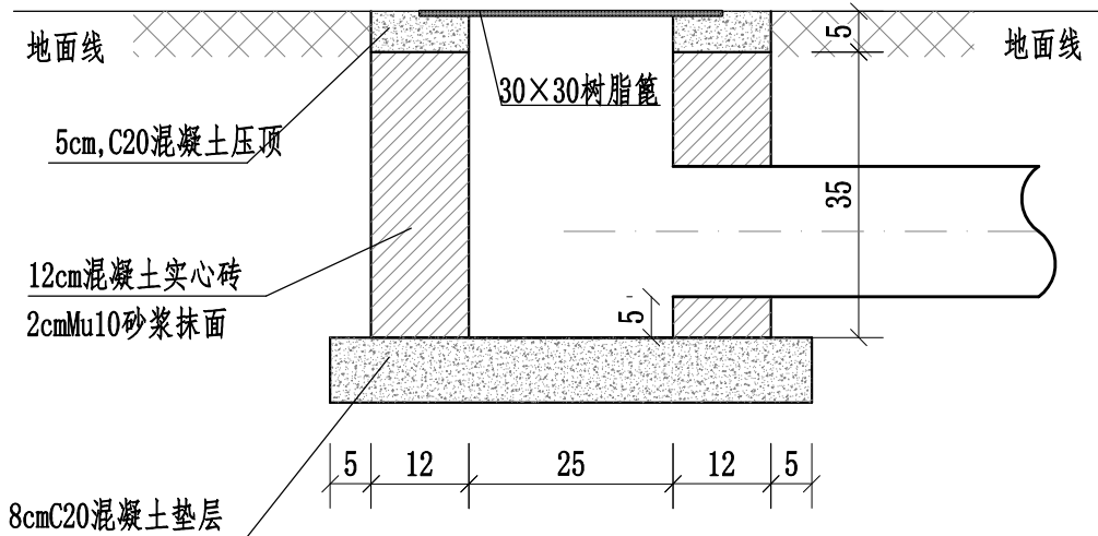
砖砌方井立面图
