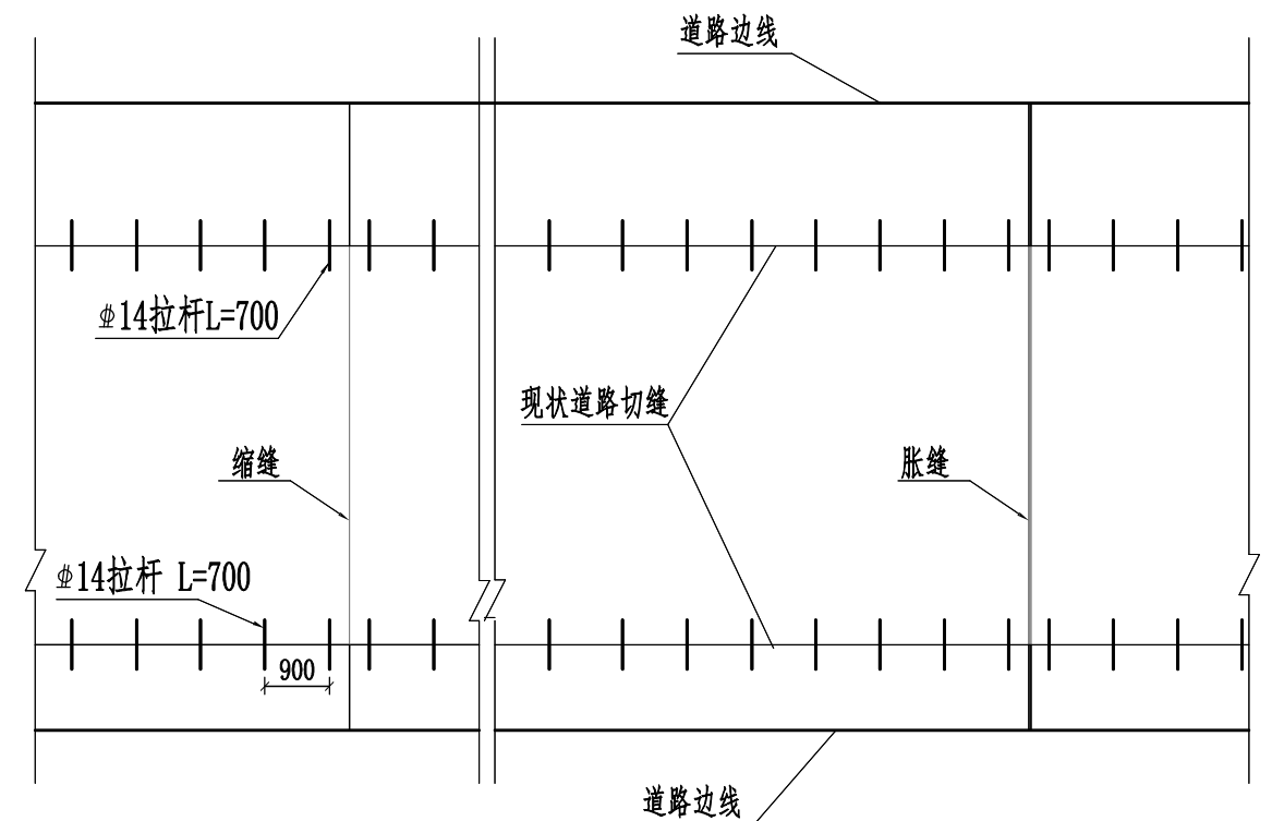
混凝土板块接缝平面示意图
