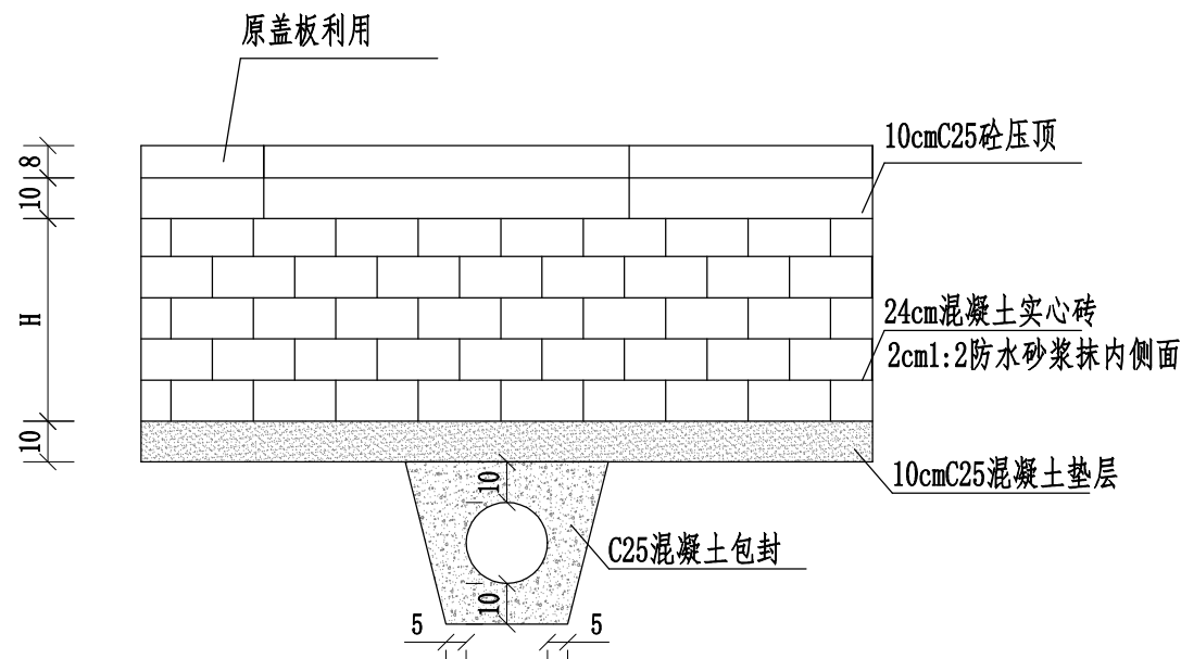
A-A剖面图
