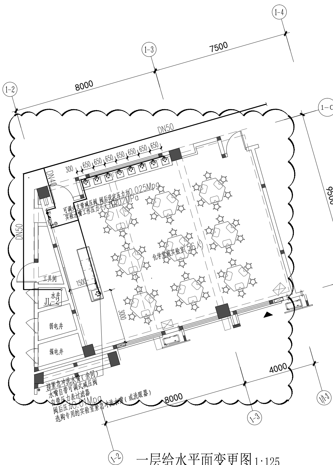
一层给水水平面变更图 1:125
