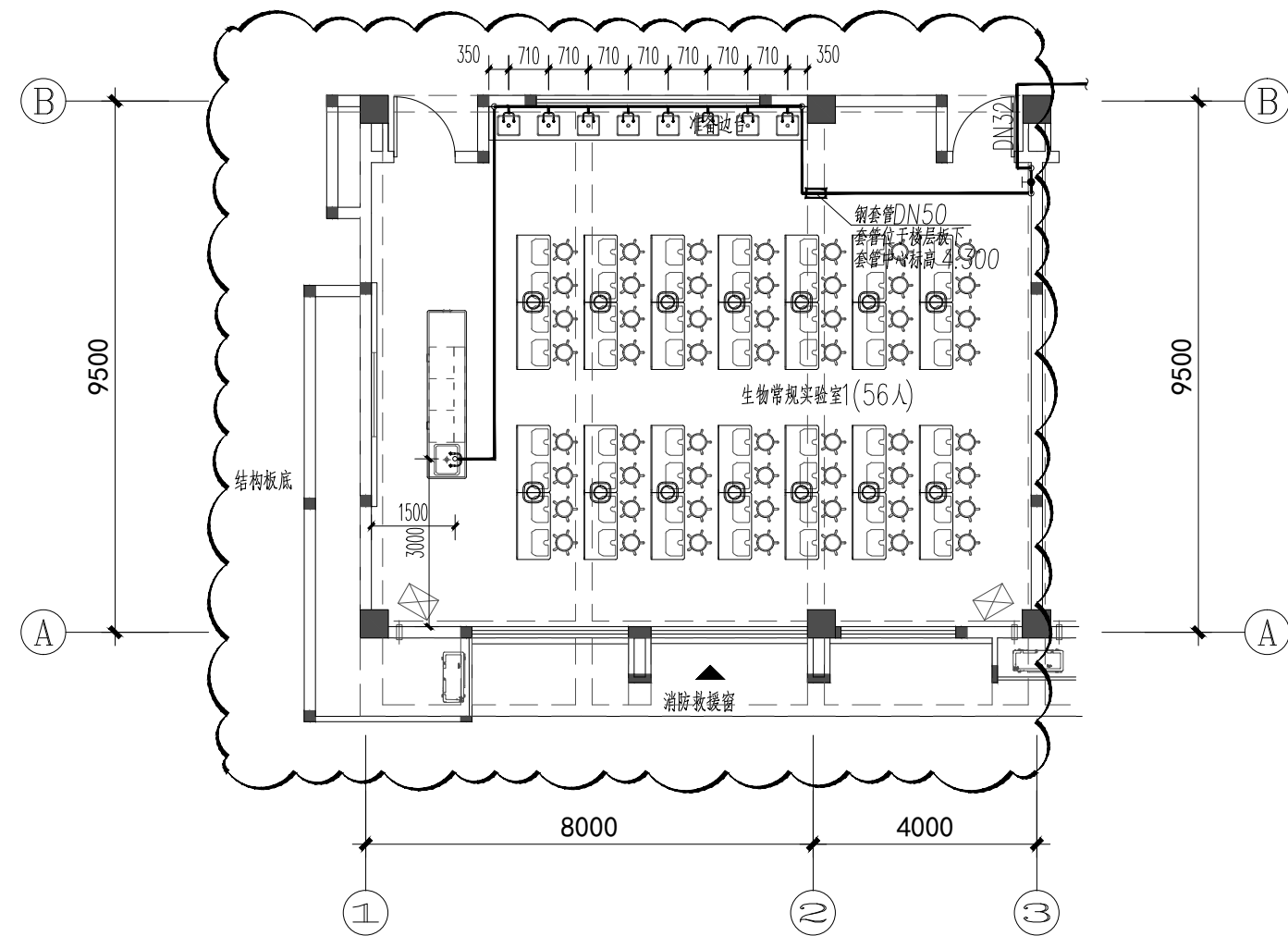
二层给水水平面变更图 1:125
