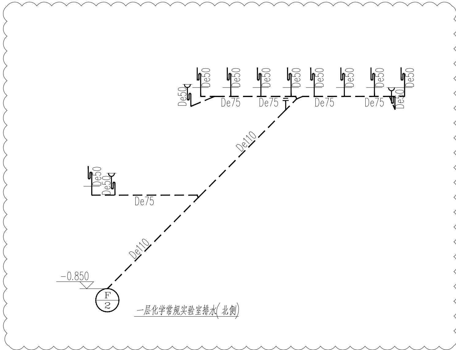
排水系统变更图
