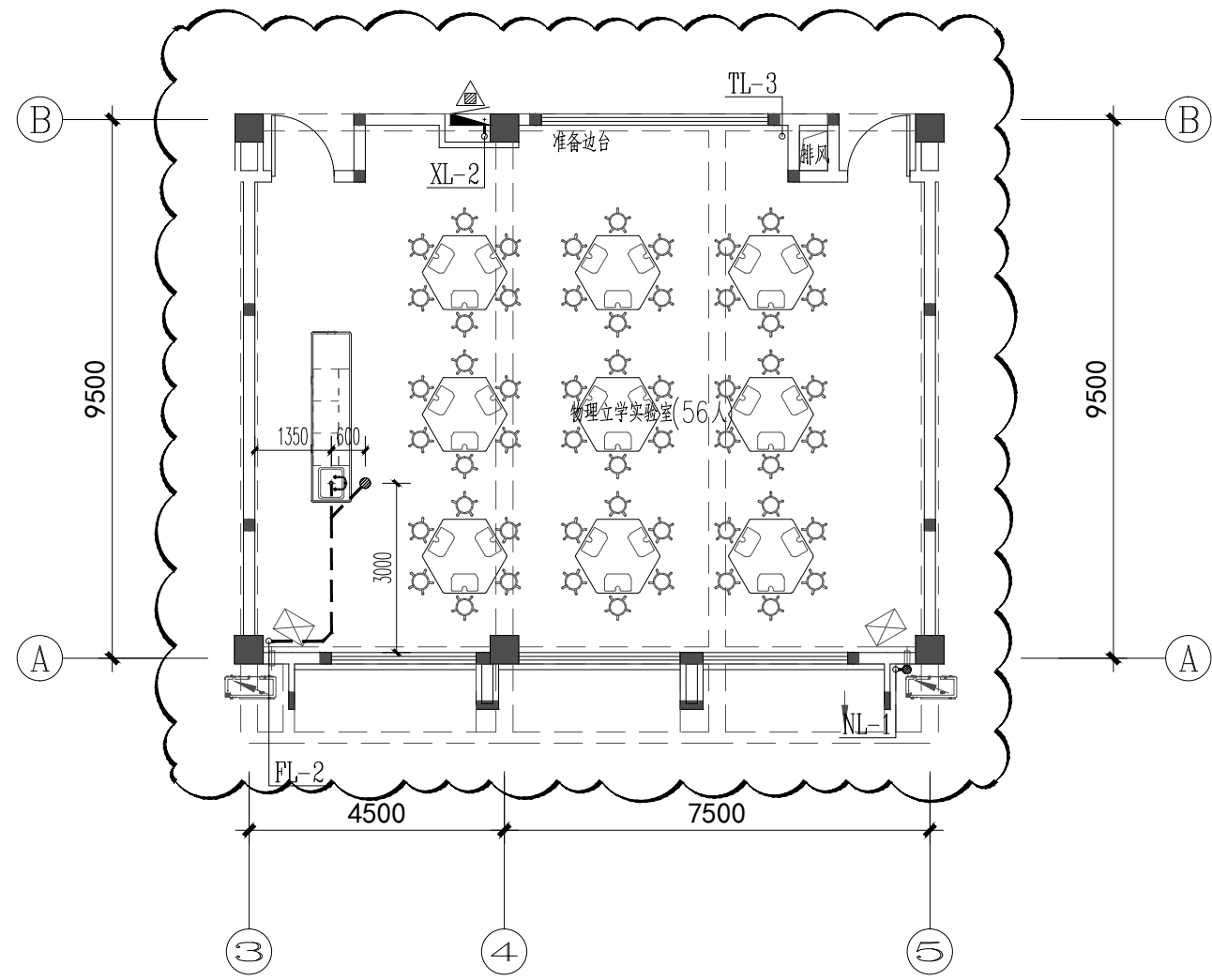
三层给排水、消防平面变更图 1:125
