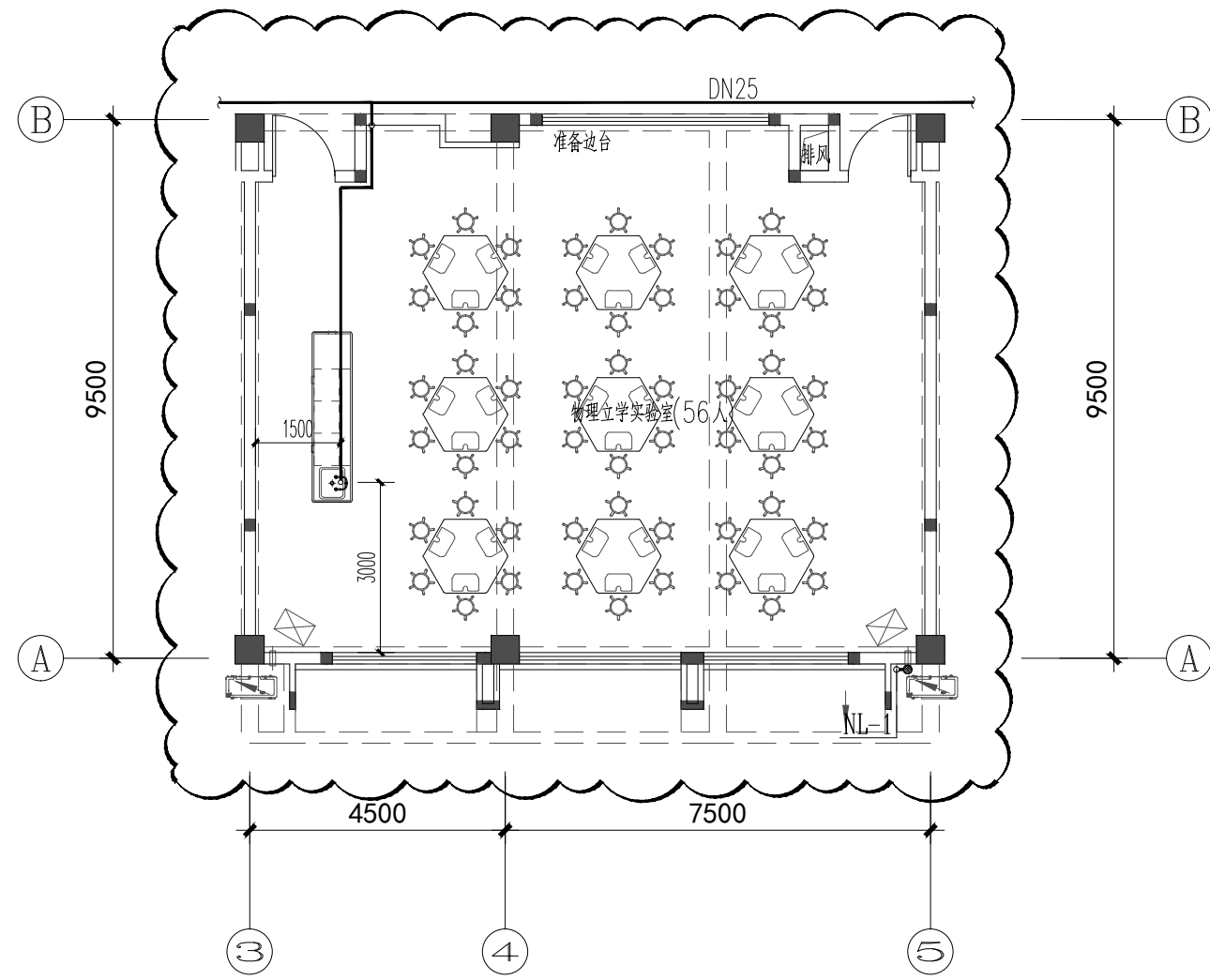
三层给水平面变更图 1:125
