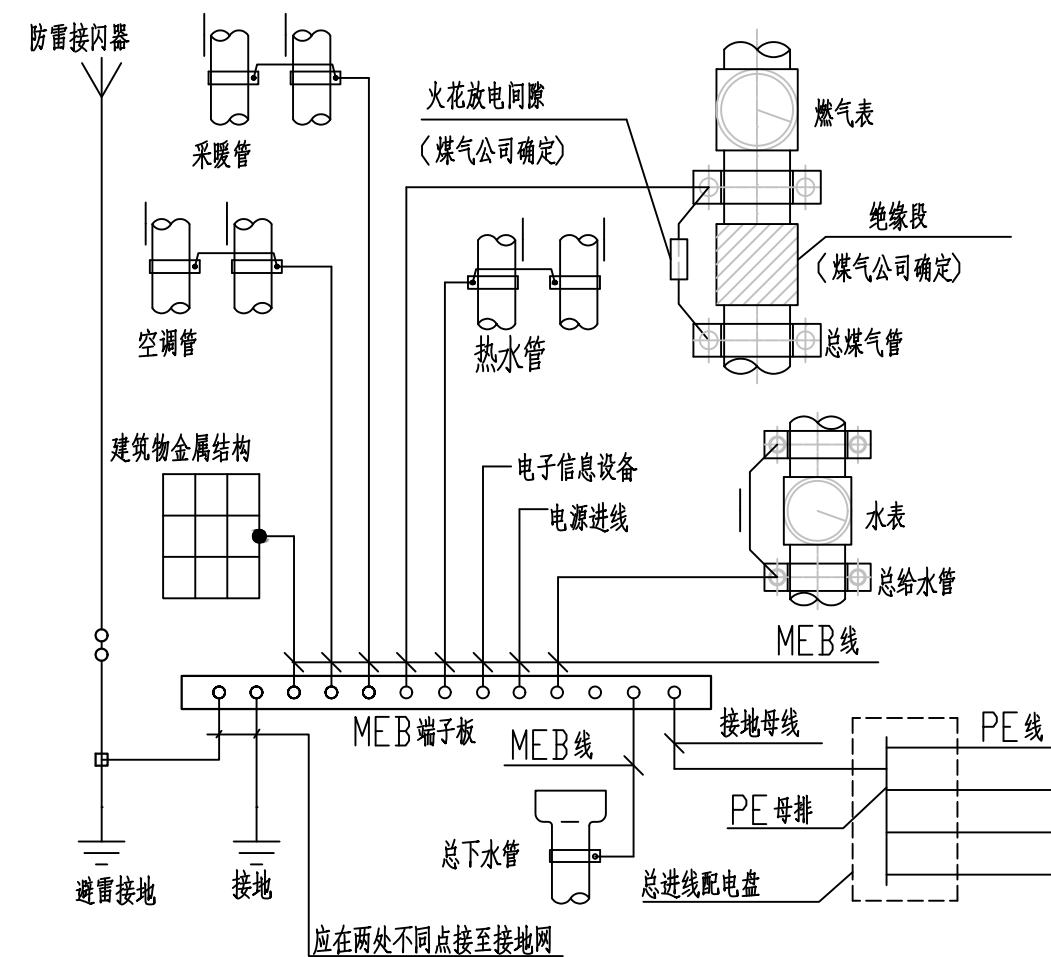
LEB 局部等电位联结示意图
