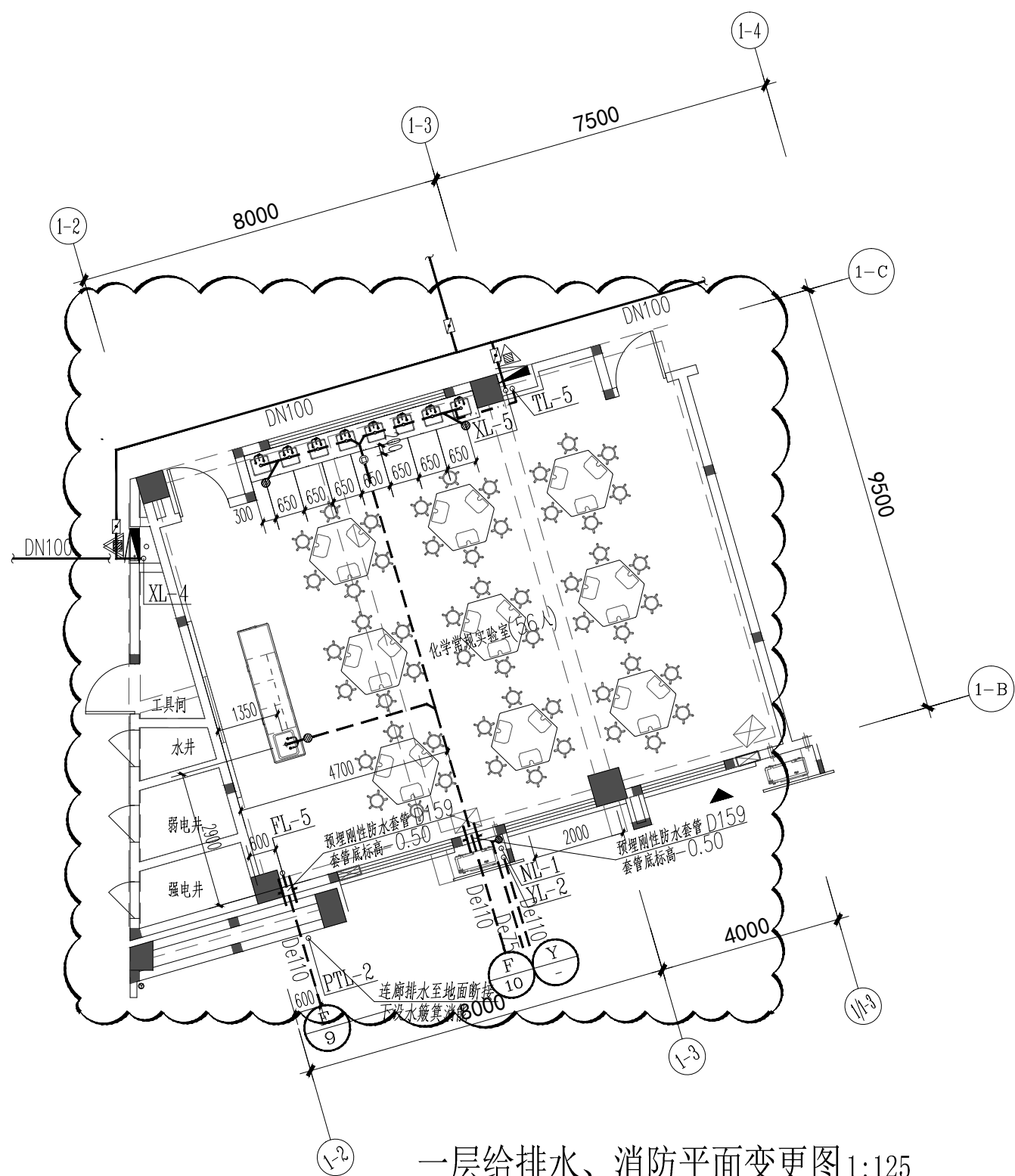
一层给排水、消防平面变更图 1:125
