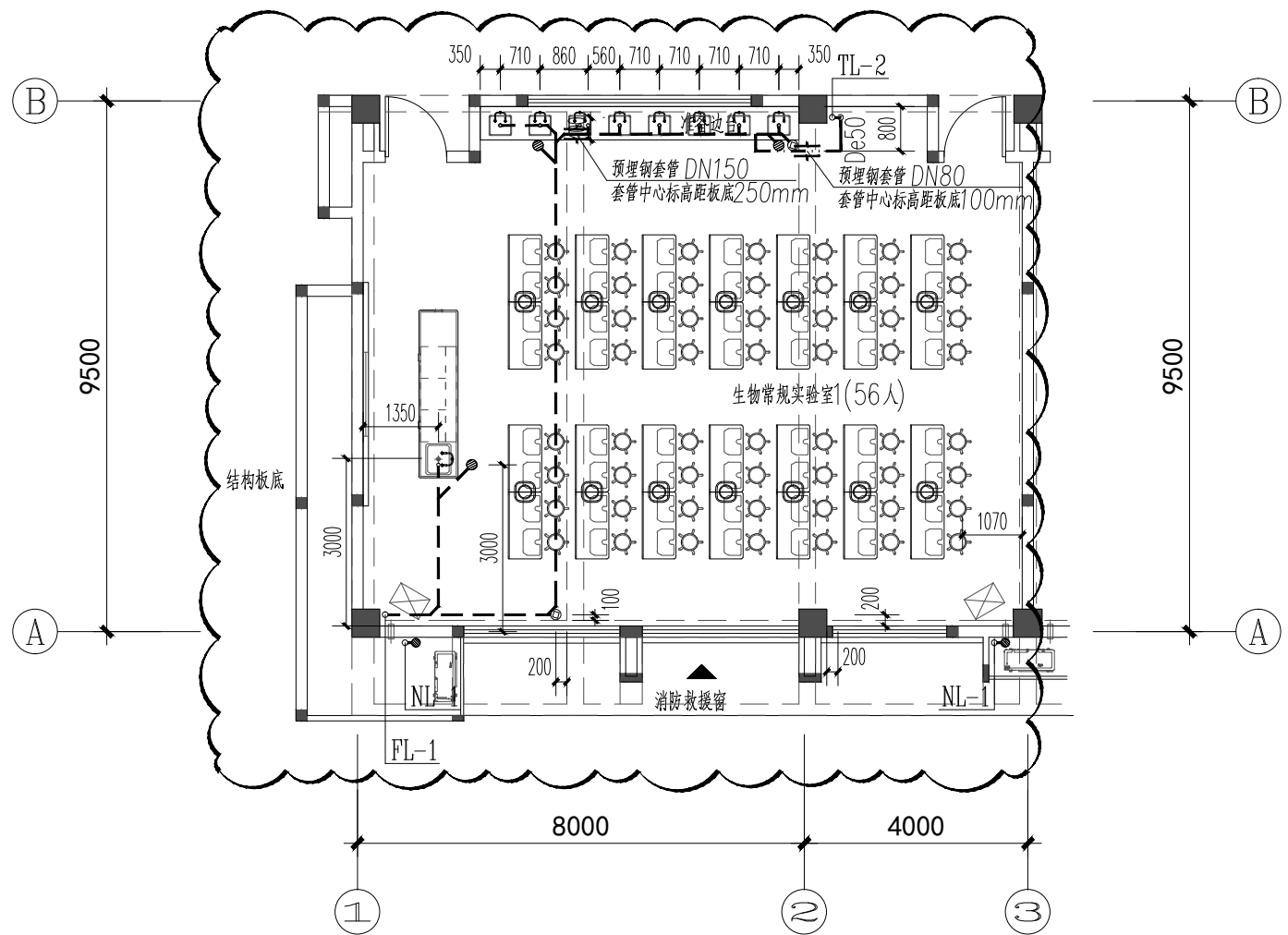
二层给排水、消防平面变更图 1:125
