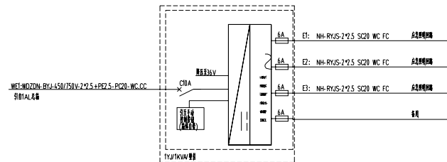
ALE 应急照明配电箱系统图
