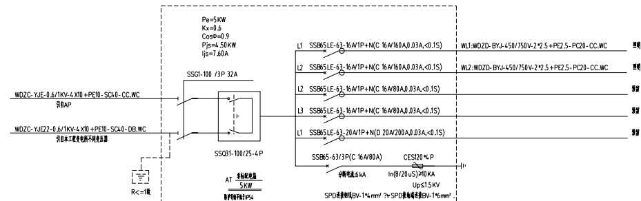
AT配电箱系统图
