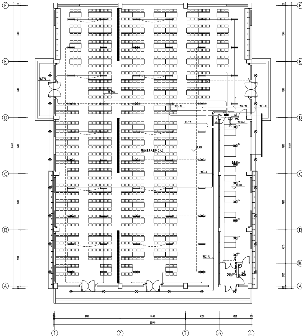
照明平面图 1:100
