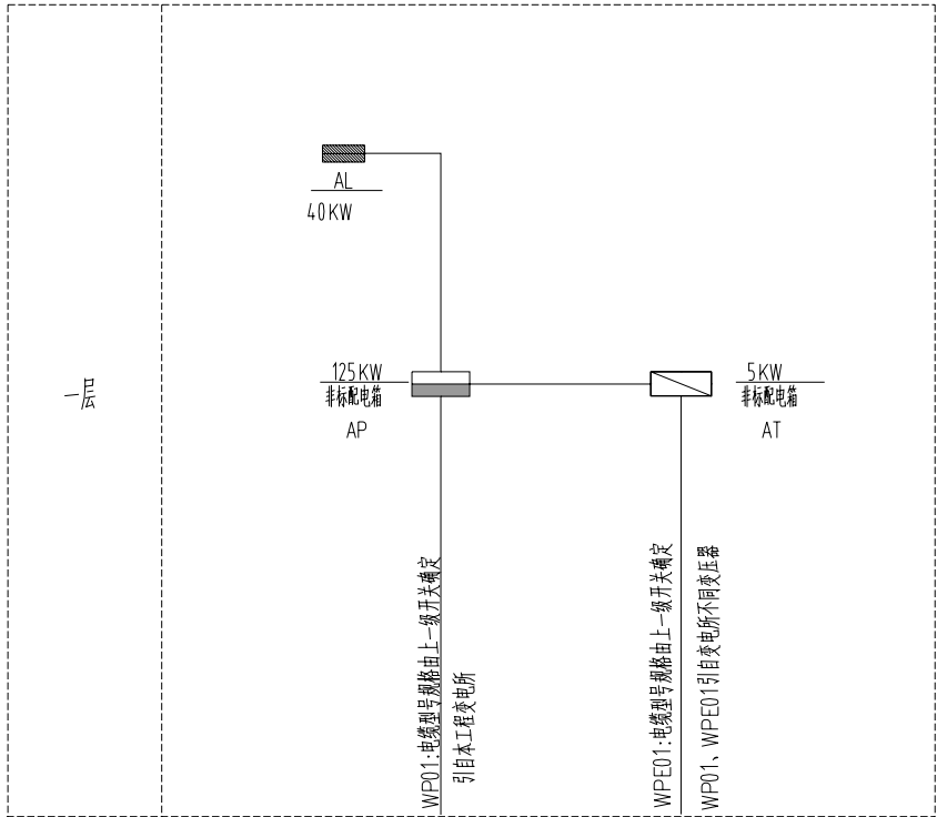
竖向配电干线系统图
