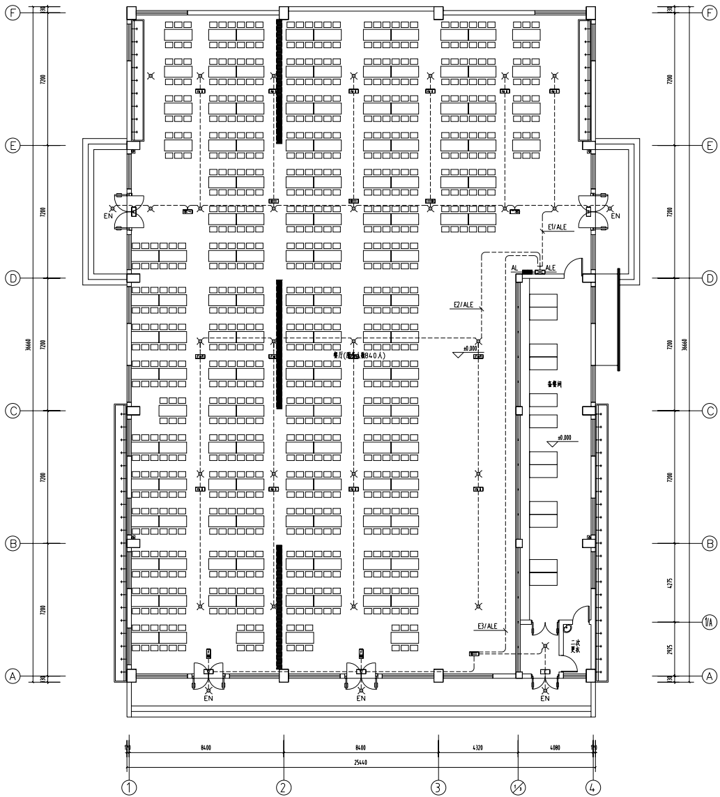
应急照明平面图:100
