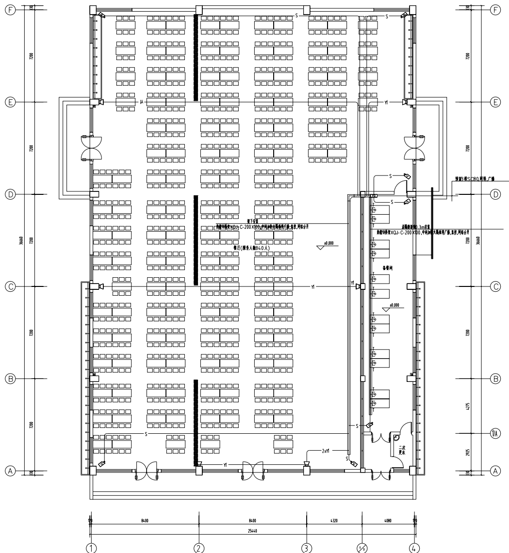
弱电平面图 1:100
