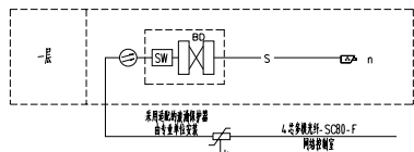
视频监控系統圖
