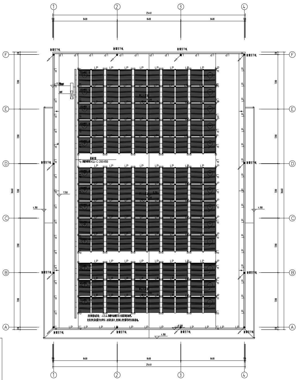
屋面防雷平面图 1:100
