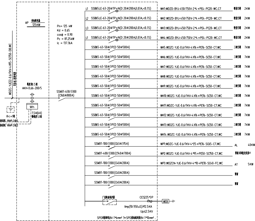
配电箱AP系统图
