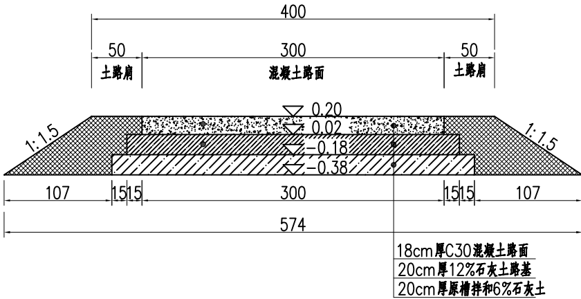
道路设计结构层图
