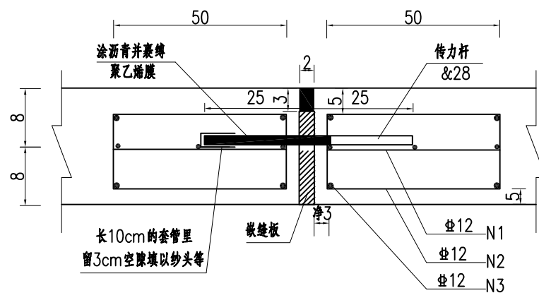
胀缝构造图
