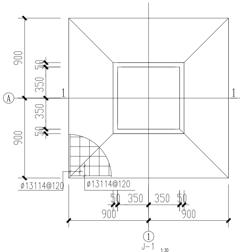
10米高杆灯基础平面图
