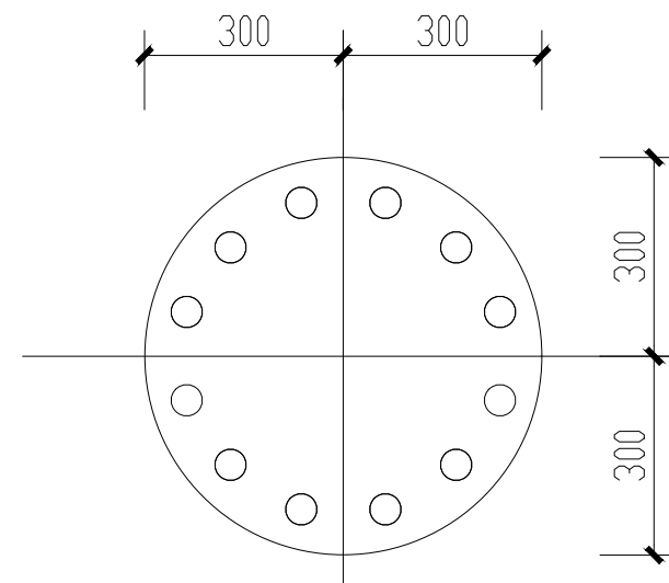
10米高杆灯杆底座平面图
