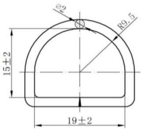
图 C.3 半圆环结构及主要尺寸
