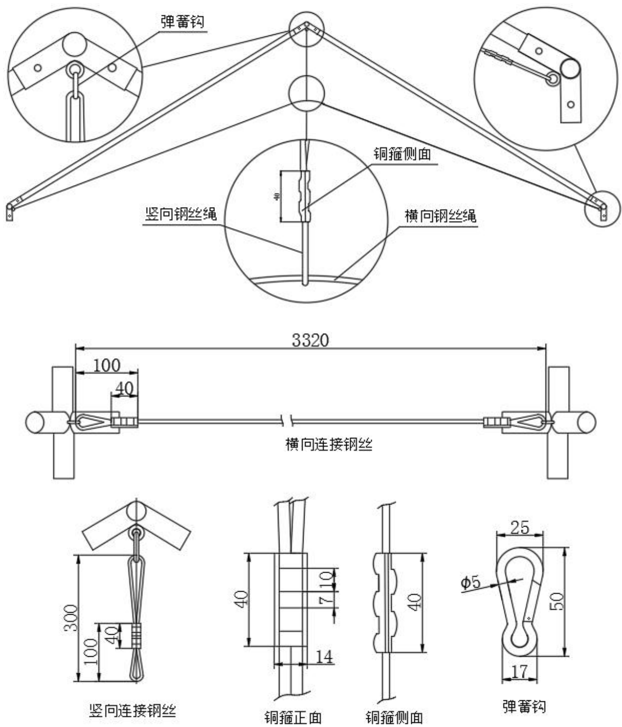
图 B.8 钢丝拉绳结构及主要尺寸
