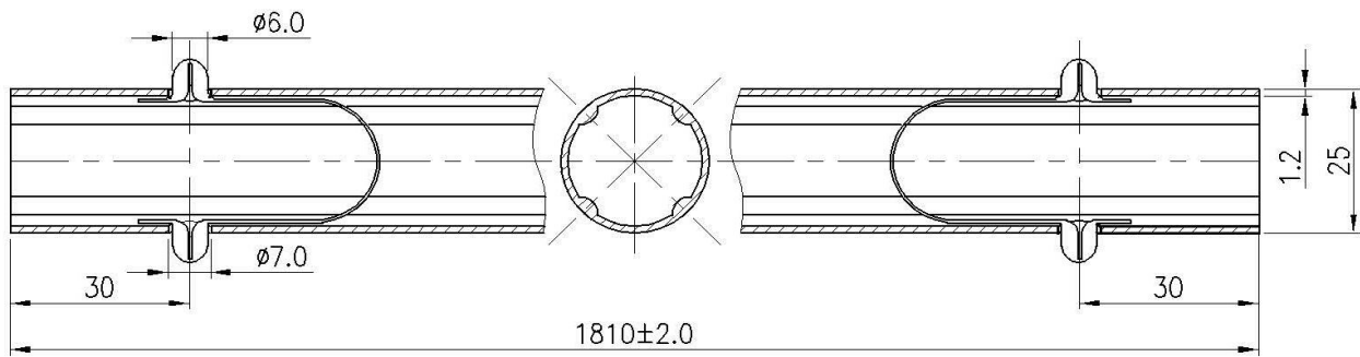
图 B. 1 通用杆结构及主要尺寸
