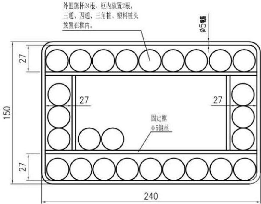
图 C. 5 框架内包装及固定框主要尺寸
