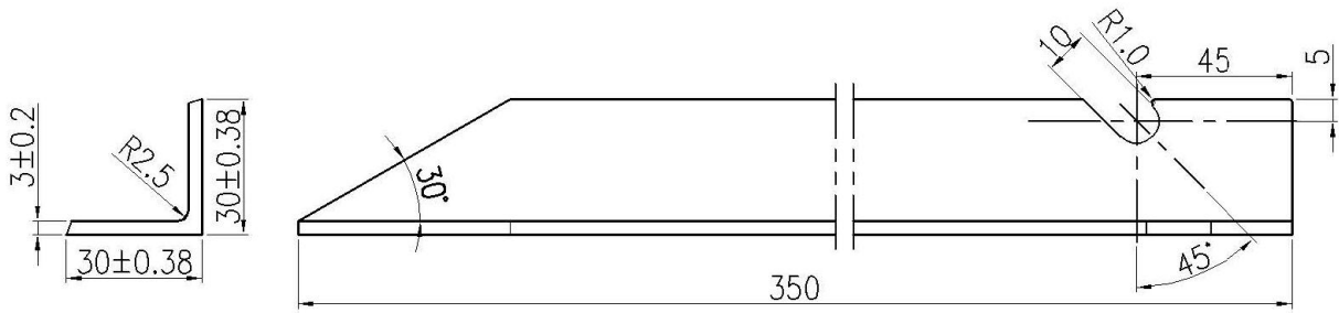
图 C.1 三角桩结构及主要尺寸
