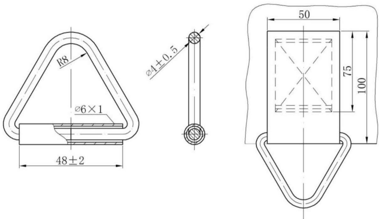
图 C.2 带管三角环结构及主要尺寸
