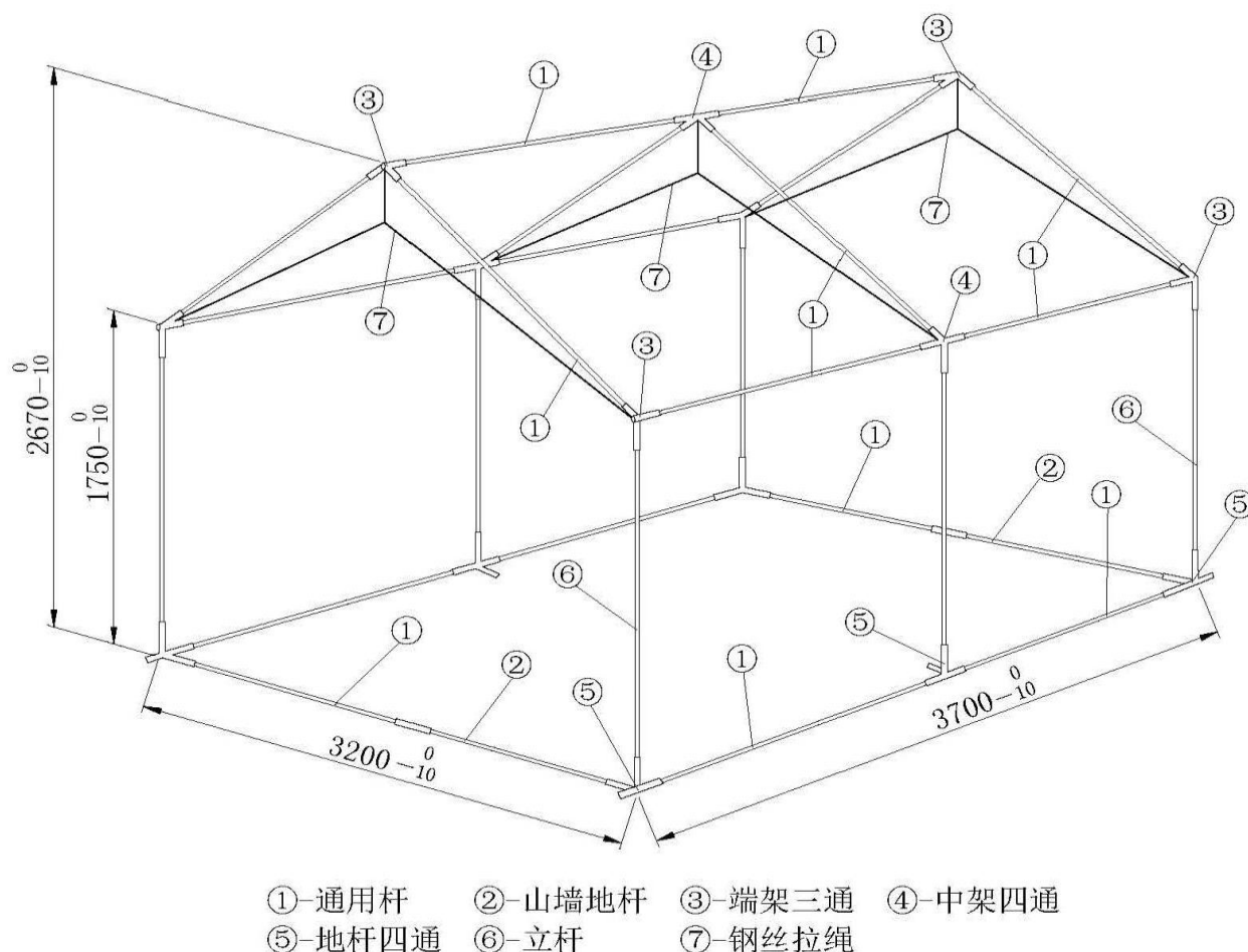
图 2 框架各部件名称、结构及主要尺寸
