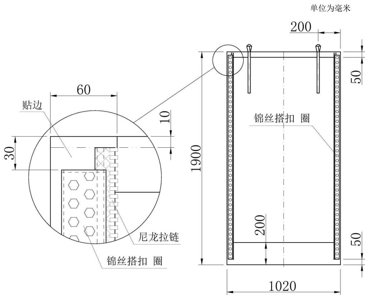
图 A.10 门帘结构及主要尺寸
