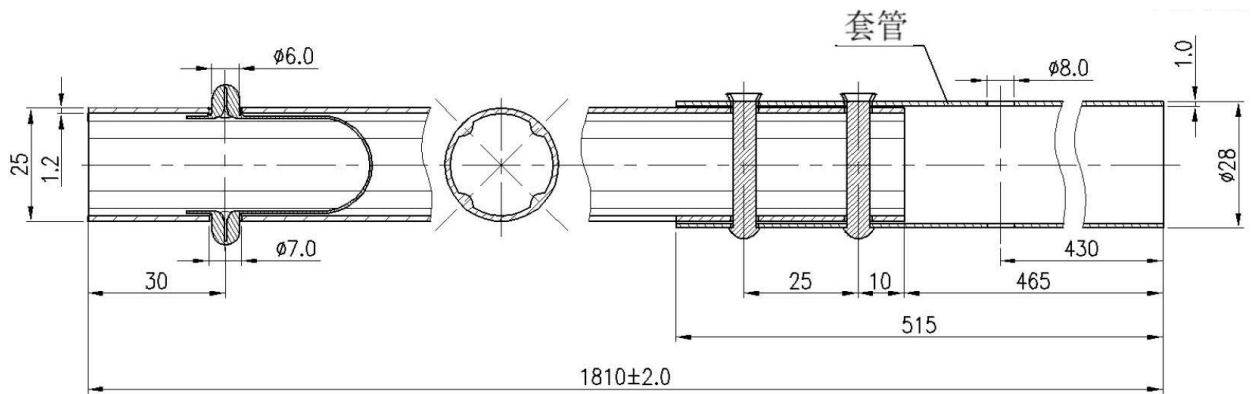
图 B. 3 三墙地杆结构及主要尺寸
