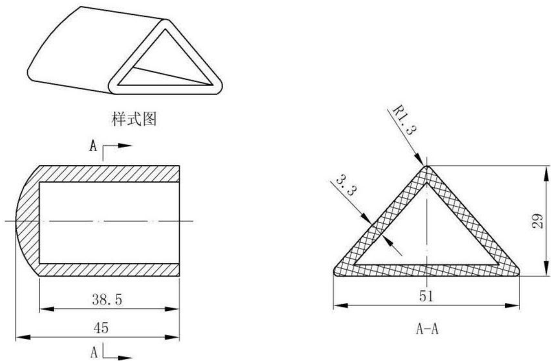
图 C. 4 橡胶桩头结构及主要尺寸
