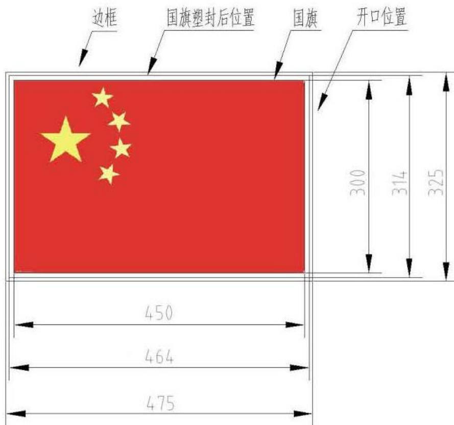
图 E.1 国旗标志主要尺寸
