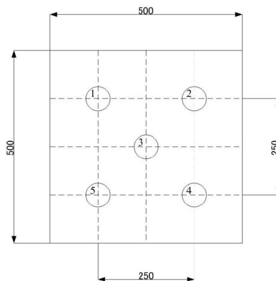
图 I.2 试样静水压测点位置
