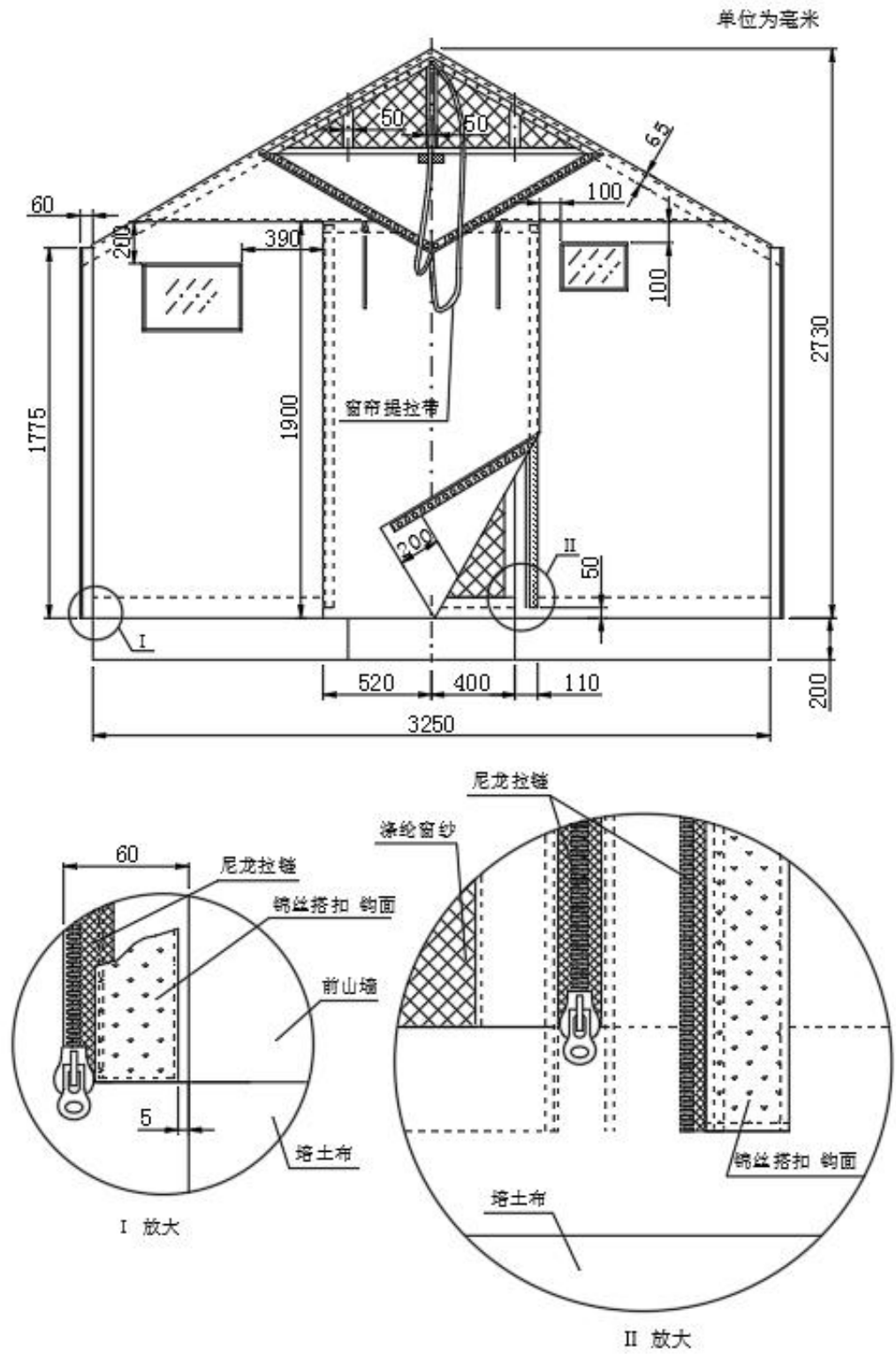
图 A.5 开门山墙面结构及主要尺寸
