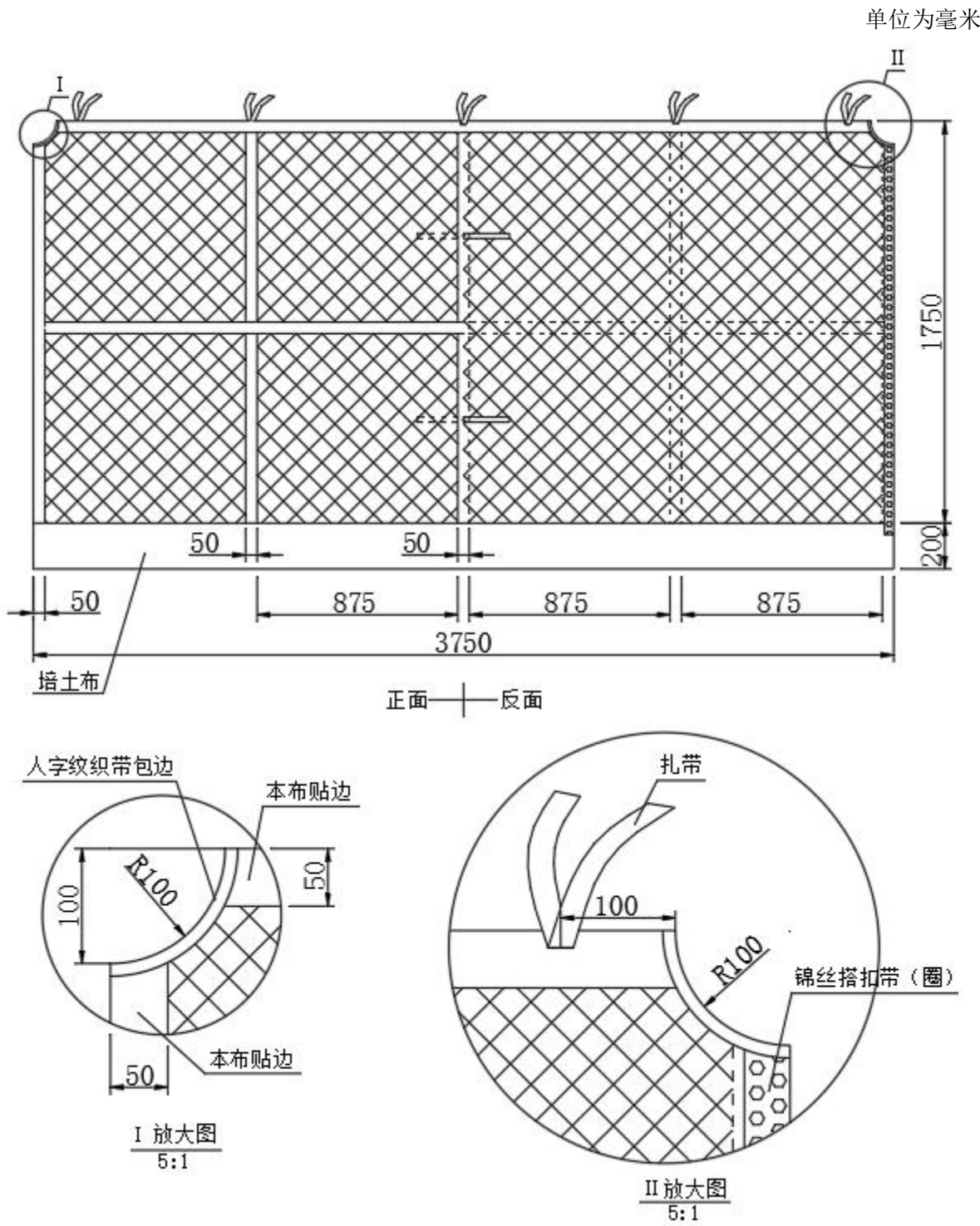
图 A. 12 纱围结构及主要尺寸
