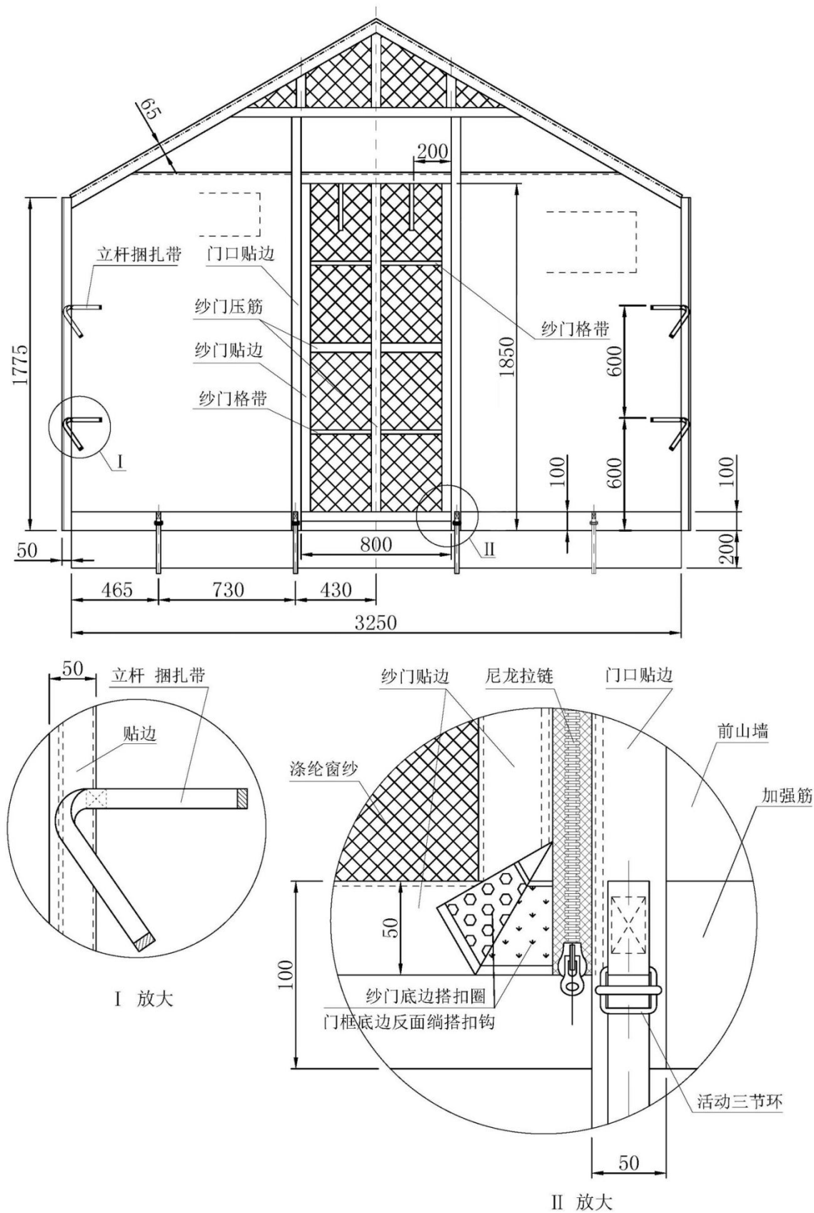
图 A. 6 开门山墙里结构及主要尺寸
