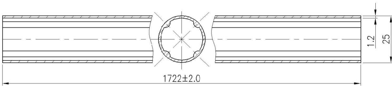
图 B. 2 立杆结构及主要尺寸
