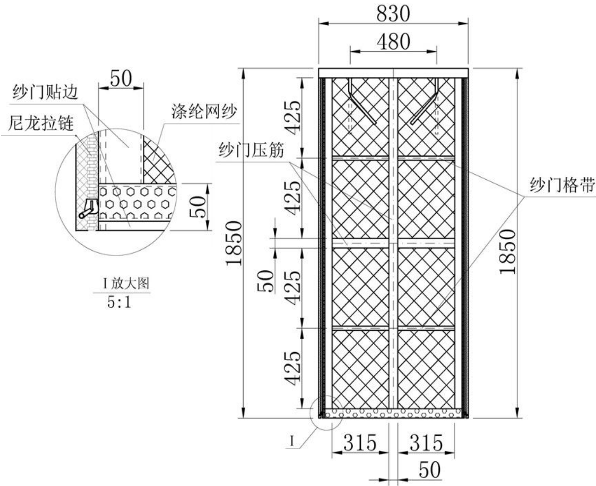
图 A. 11 纱门结构及主要尺寸
