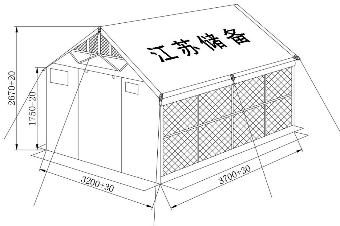
图1 样式、结构及主要尺寸
