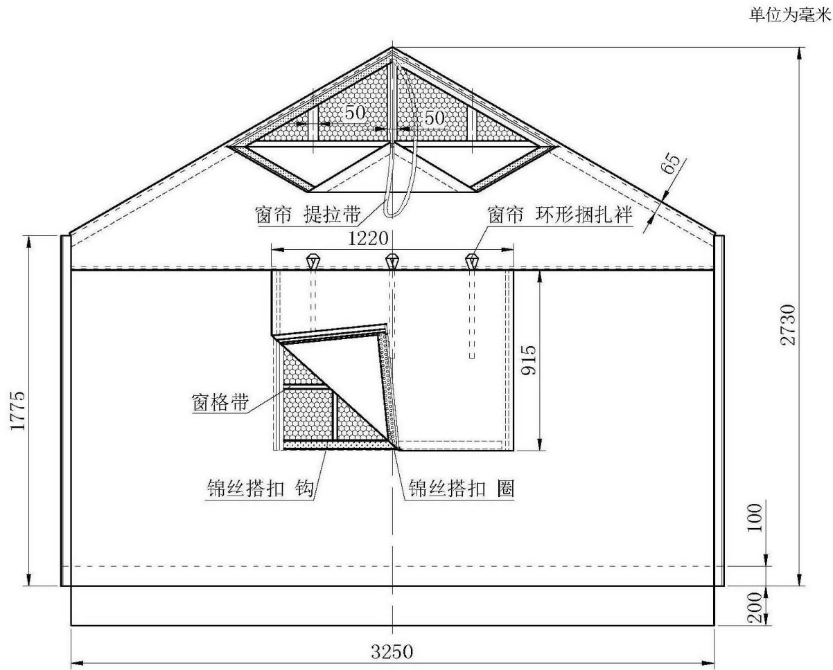
图 A. 7 开窗山墙里结构及主要尺寸
