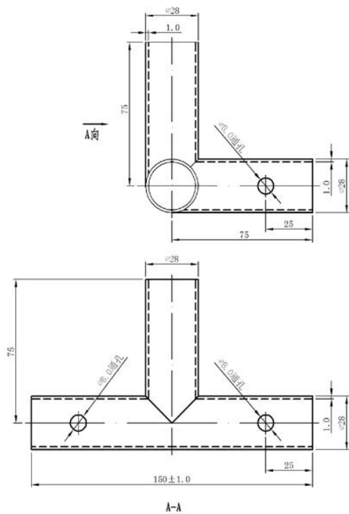
图 B. 6 地杆四通结构及主要尺寸
