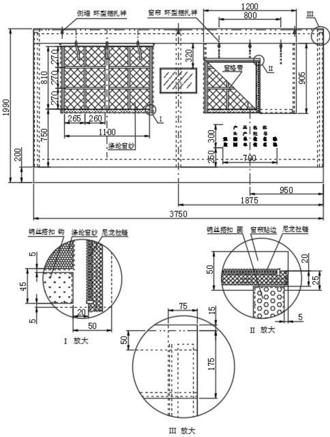
图 A.3 侧墙面与窗户结构及主要尺寸
