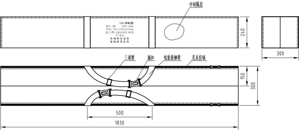
图 A.13 包装袋结构及主要尺寸
