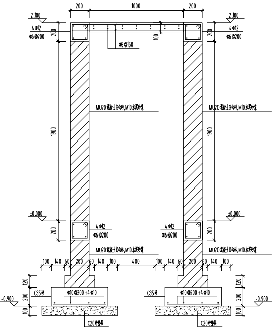
G-A 1、未注明混凝土强度等级均为C30 2、砖墙基础下土层均应压实,压实系数0.97。
