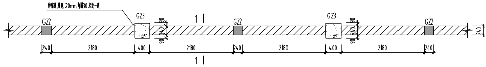
围墙平面布置图 1:100
