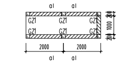
铭牌平面布置图 1:100
