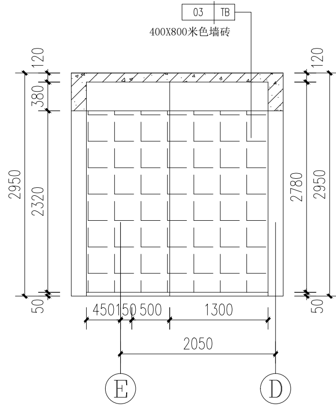
③ 厨房立面详图 1:50
