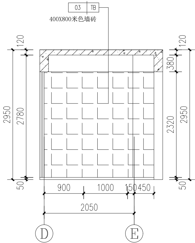
① 厨房立面详图 1:50
