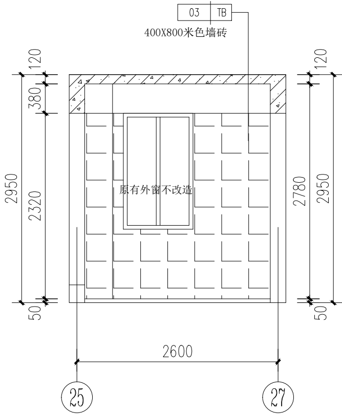
② 厨房立面详图 1:50
