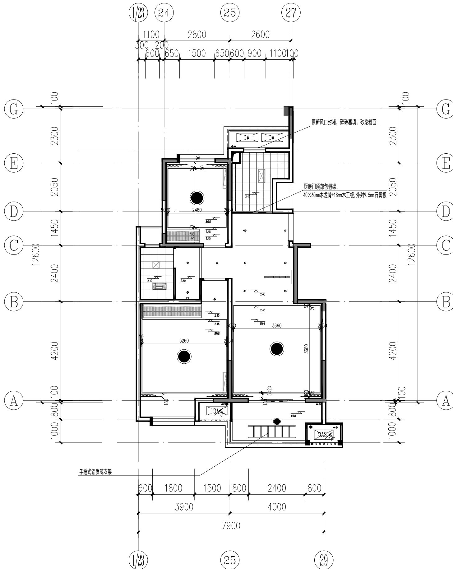
顶面布置图 1:100
