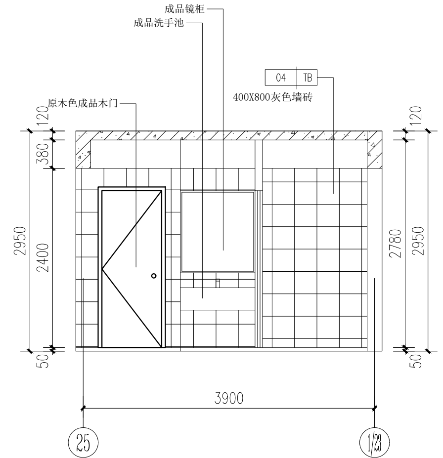
③ 卫生间立面详图 1:50
