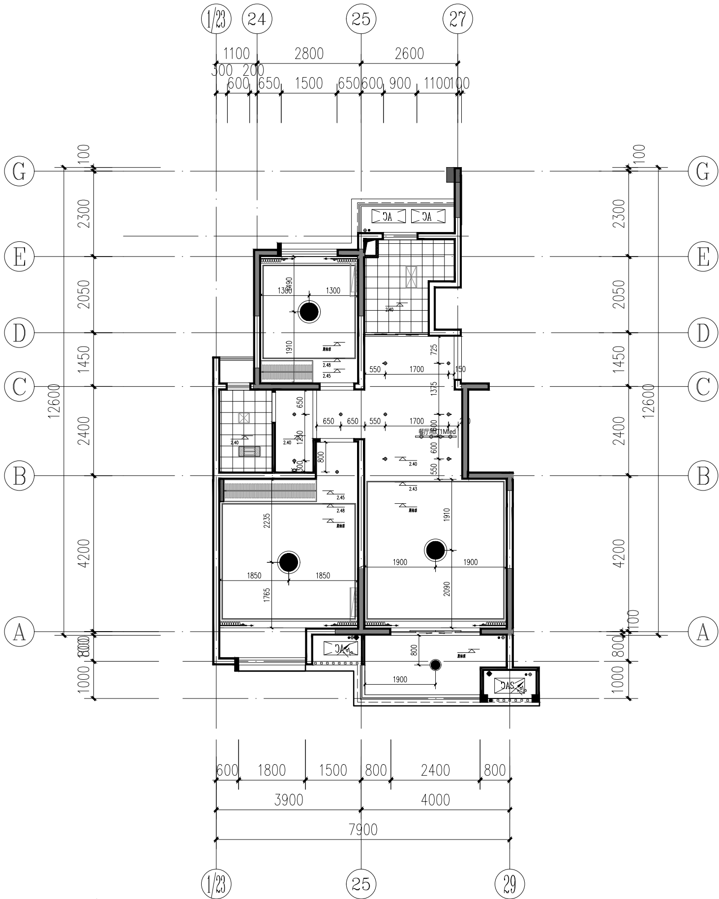
灯具定位图 1:100
