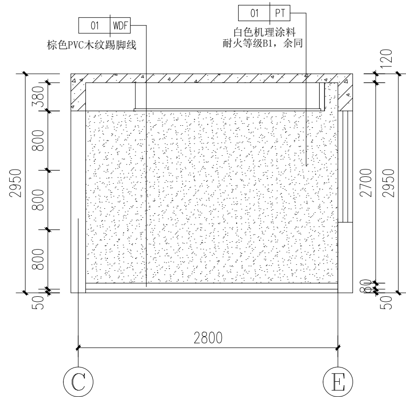
① 次卧室立面详图 1:50
