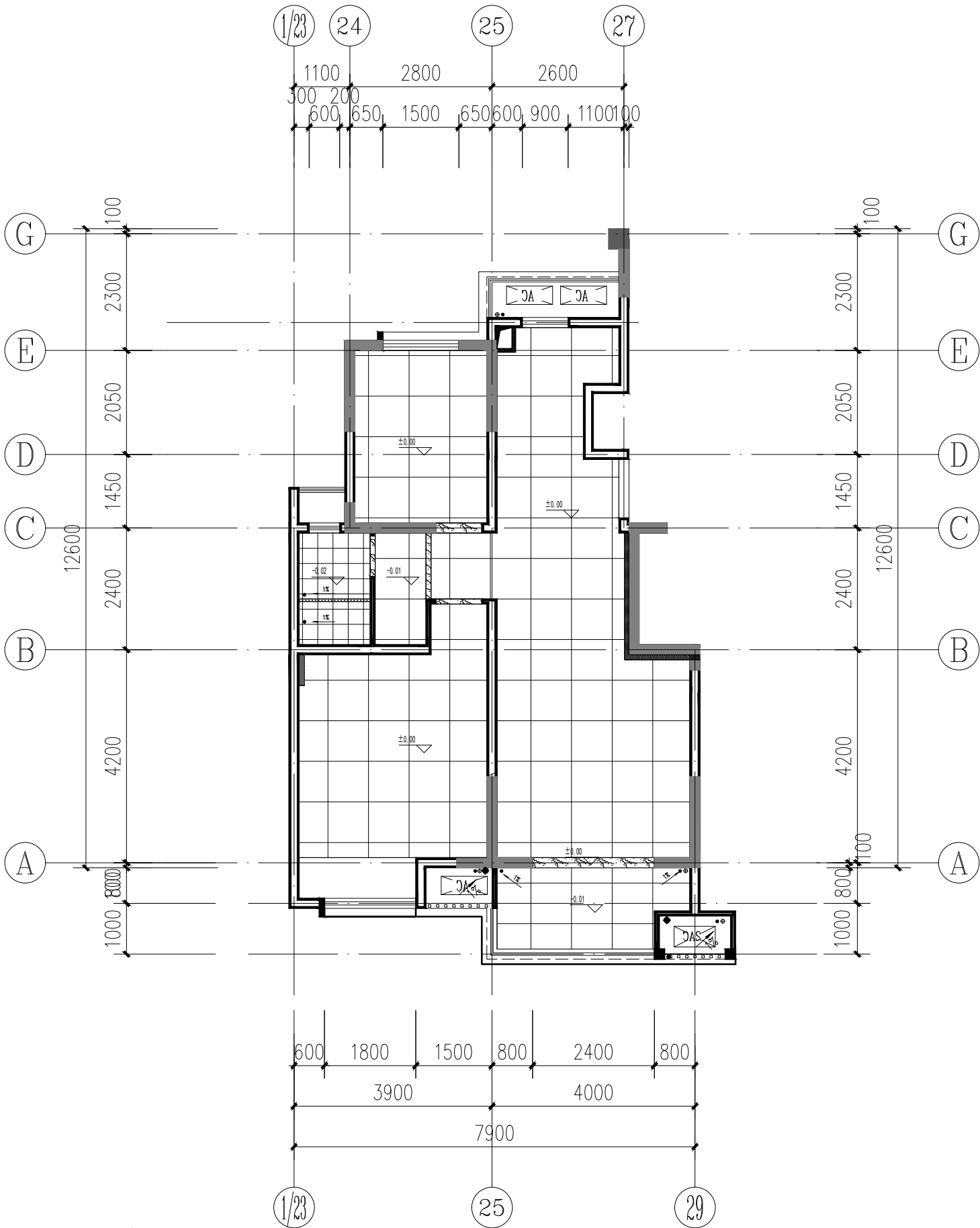
地坪布置图 1:100
