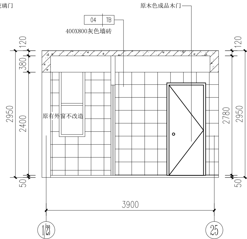
② 卫生间立面详图 1:50
