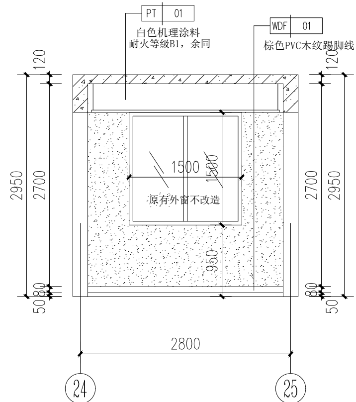
②次卧室立面详图 1:50
