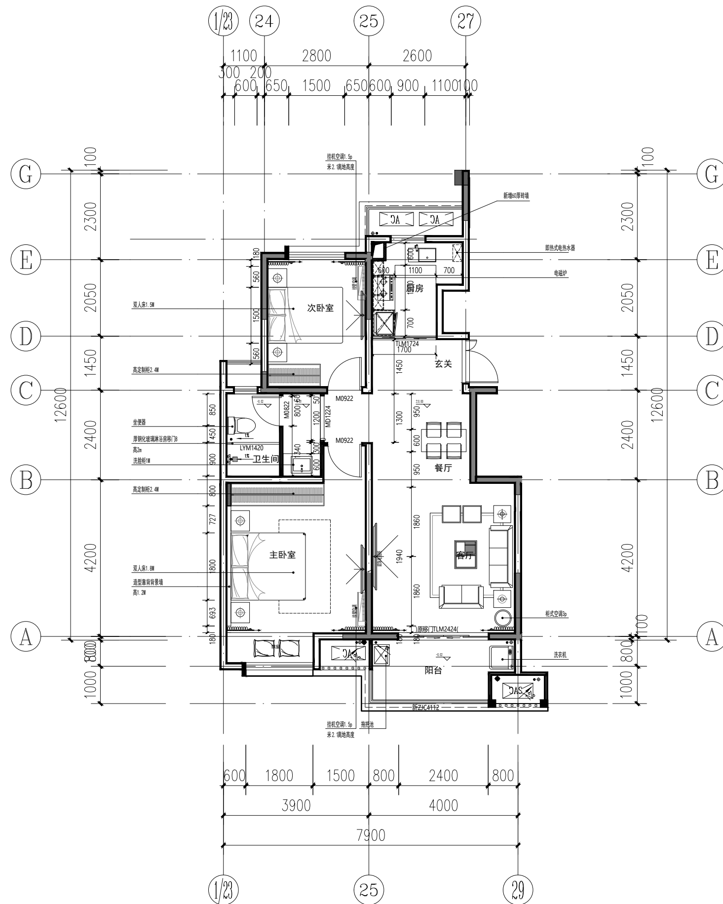
平面尺寸图 1:100
