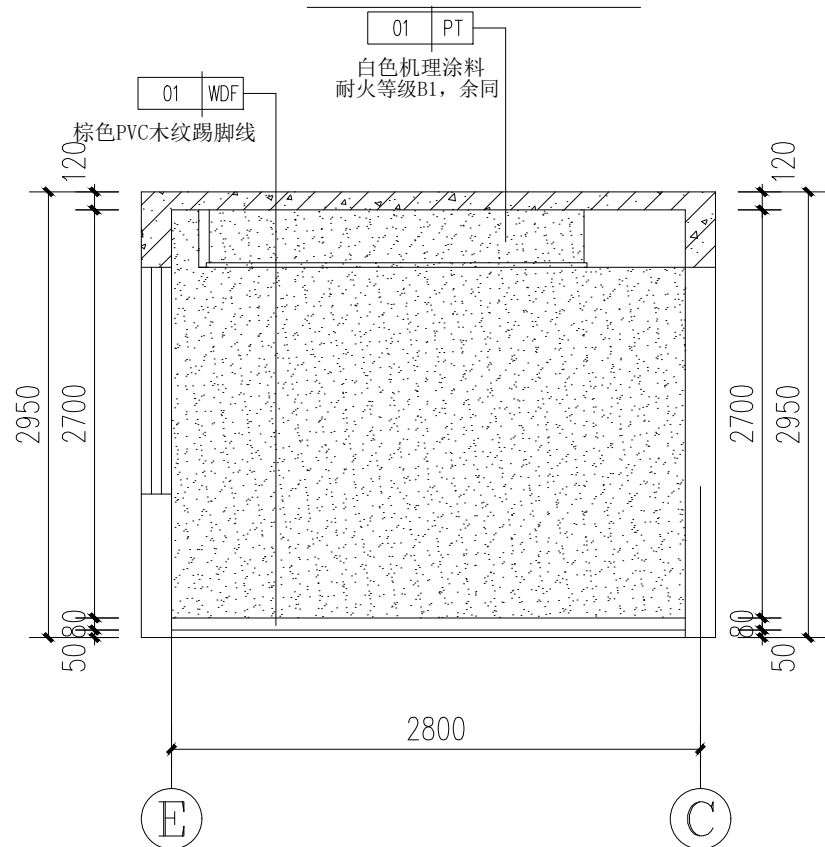
③次卧室立面详图 1:50
