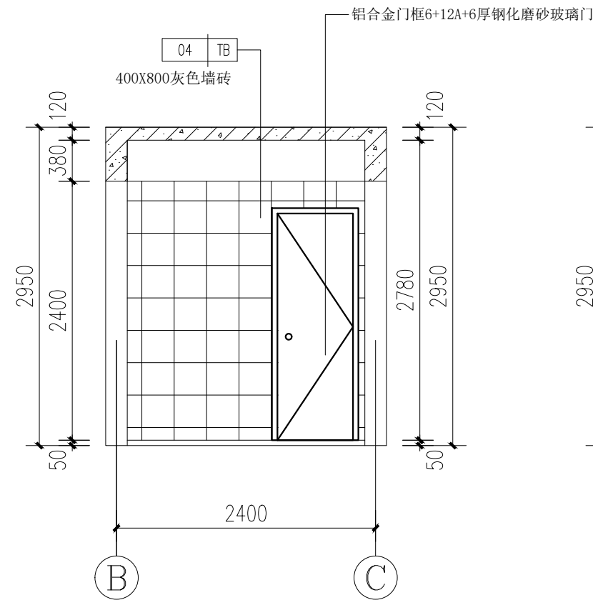
① 卫生间立面详图 1:50
