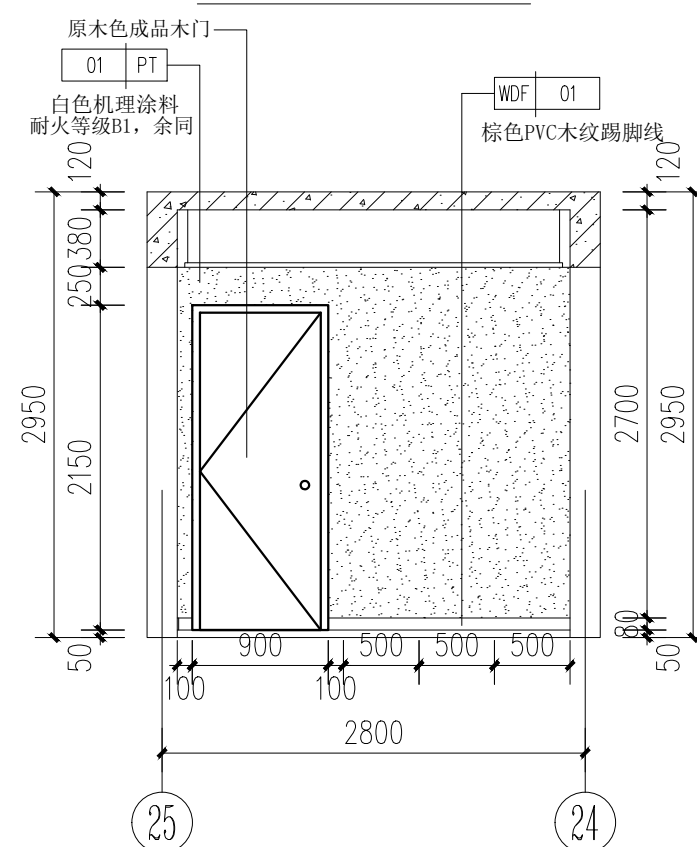
④次卧室立面详图 1:50
