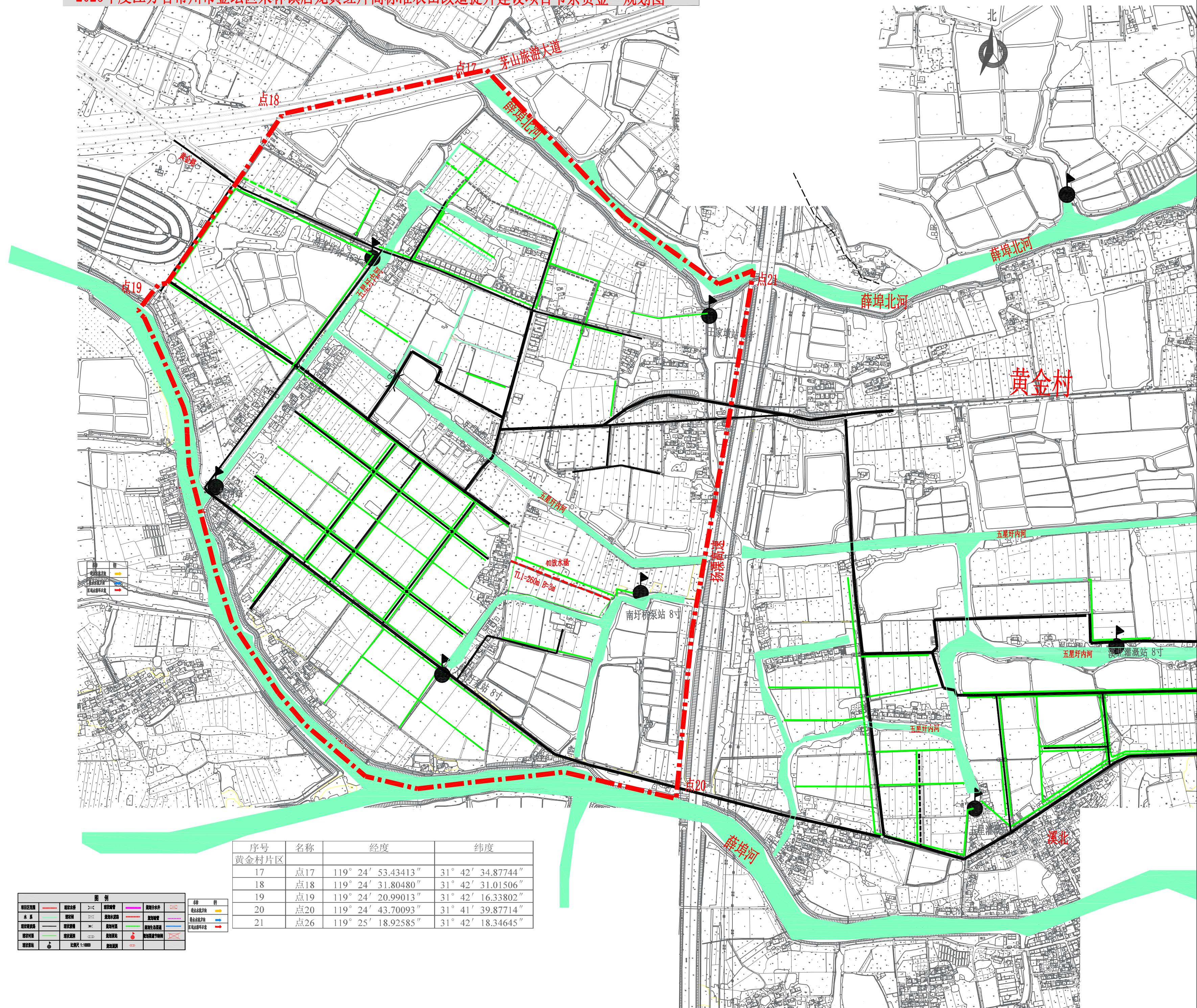
2025年度江苏省常州市金坛区朱林镇唐龙黄红片高标准农田改造提升建设项目节余资金 规划图
