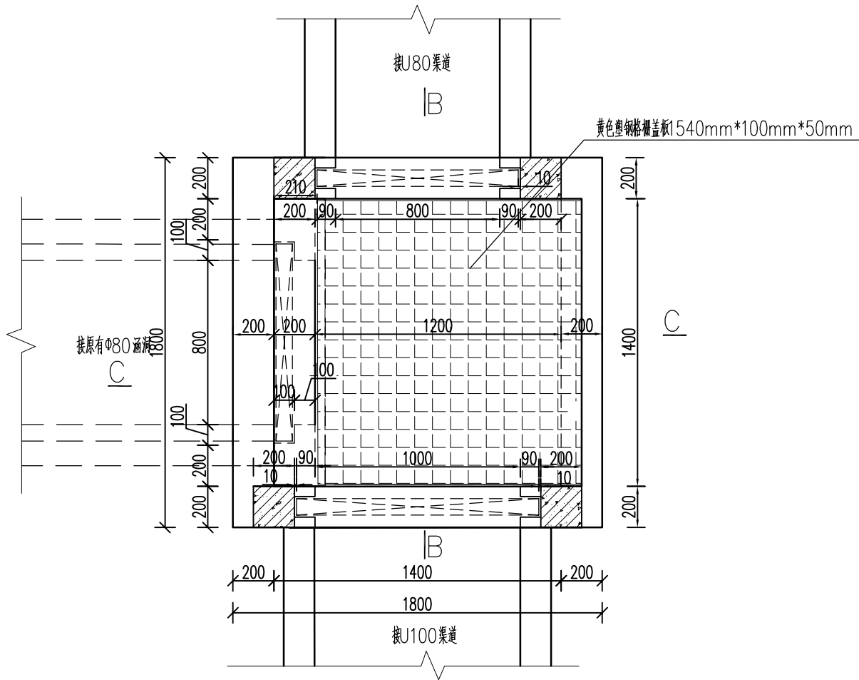
分水井平面图 1:25
