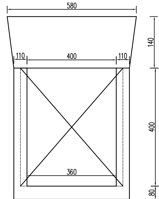
预制放水口大洋图
