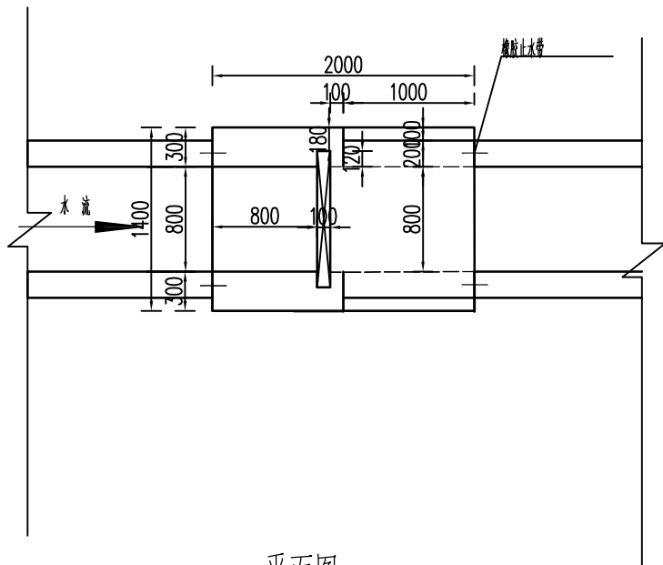
平面图 1:50
