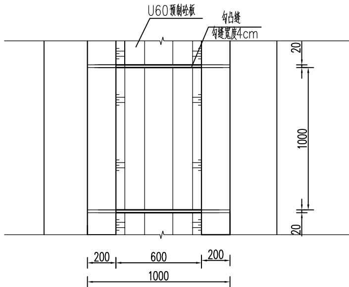
U60渠道平面图 1:25
