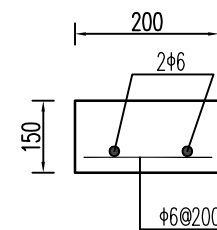
压顶配筋图 1:10
