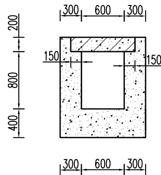
进水端视图 1:50
