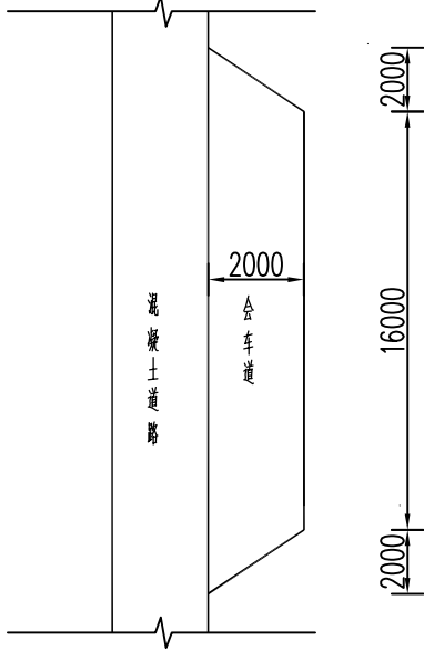
会车道平面图
