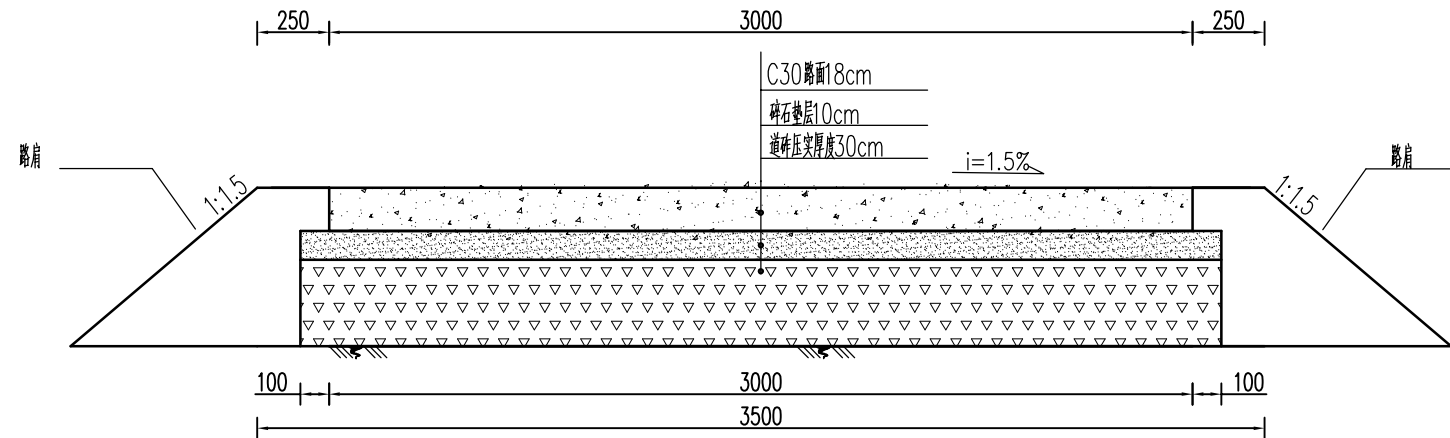
新建3.0m宽混凝土路横断面图 1:25 无路基
