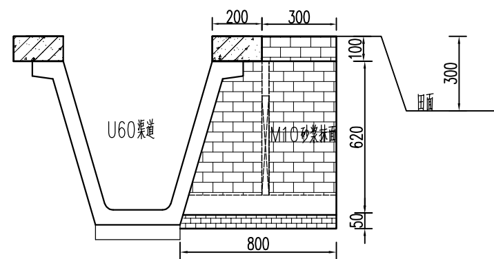
U60放水口纵剖视图 1:20
