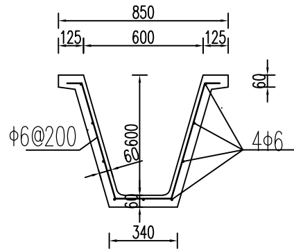
U60渠道板断面尺寸 1:25
