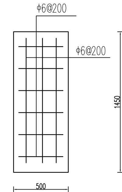
渠道板断面图 1:20
