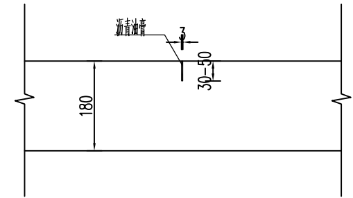
横向缩缝 1:10
