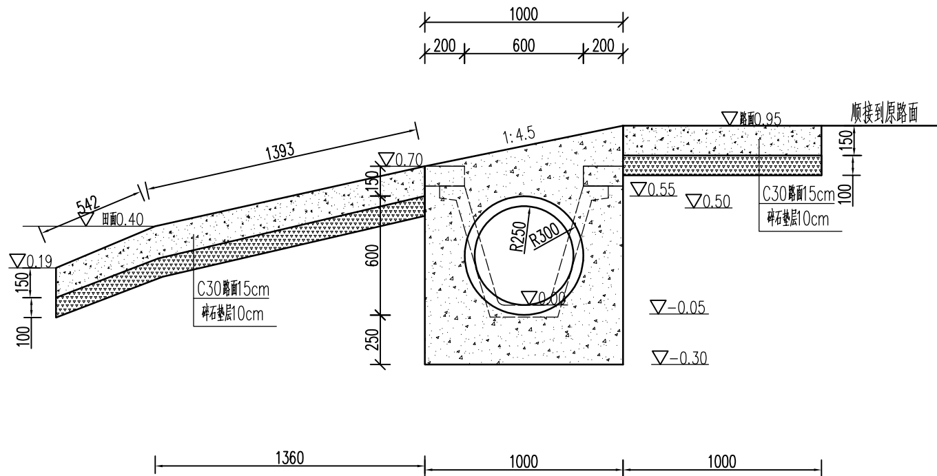
A-A 1:25
