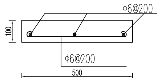
渠道板断面图 1:10
