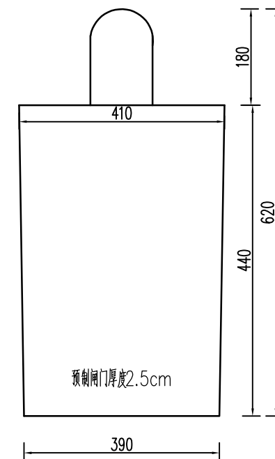
预制闸门大洋图
