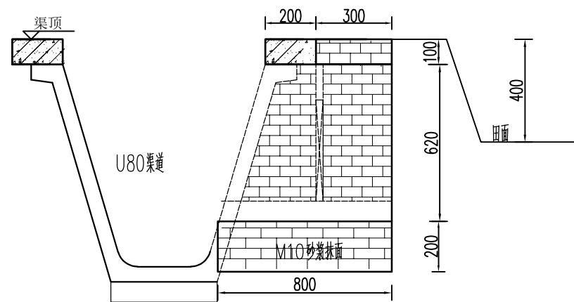
U80放水口纵剖视图 1:20
