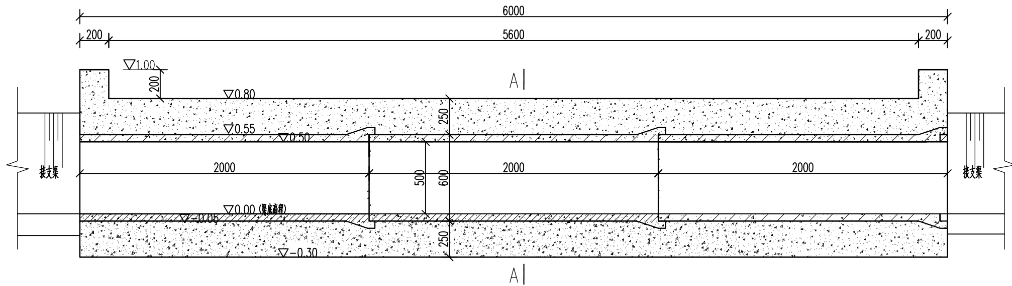
Φ0.5*6m 穿路涵洞剖面图 1:25
