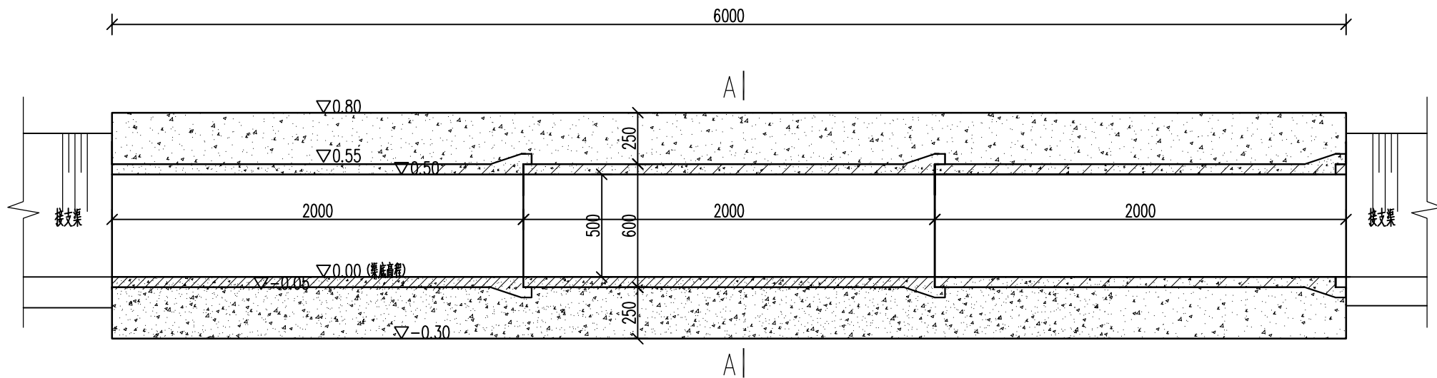
Φ0.5*6m 下田涵洞剖面图 1:25
