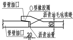
承插式涵管接头 1:25
