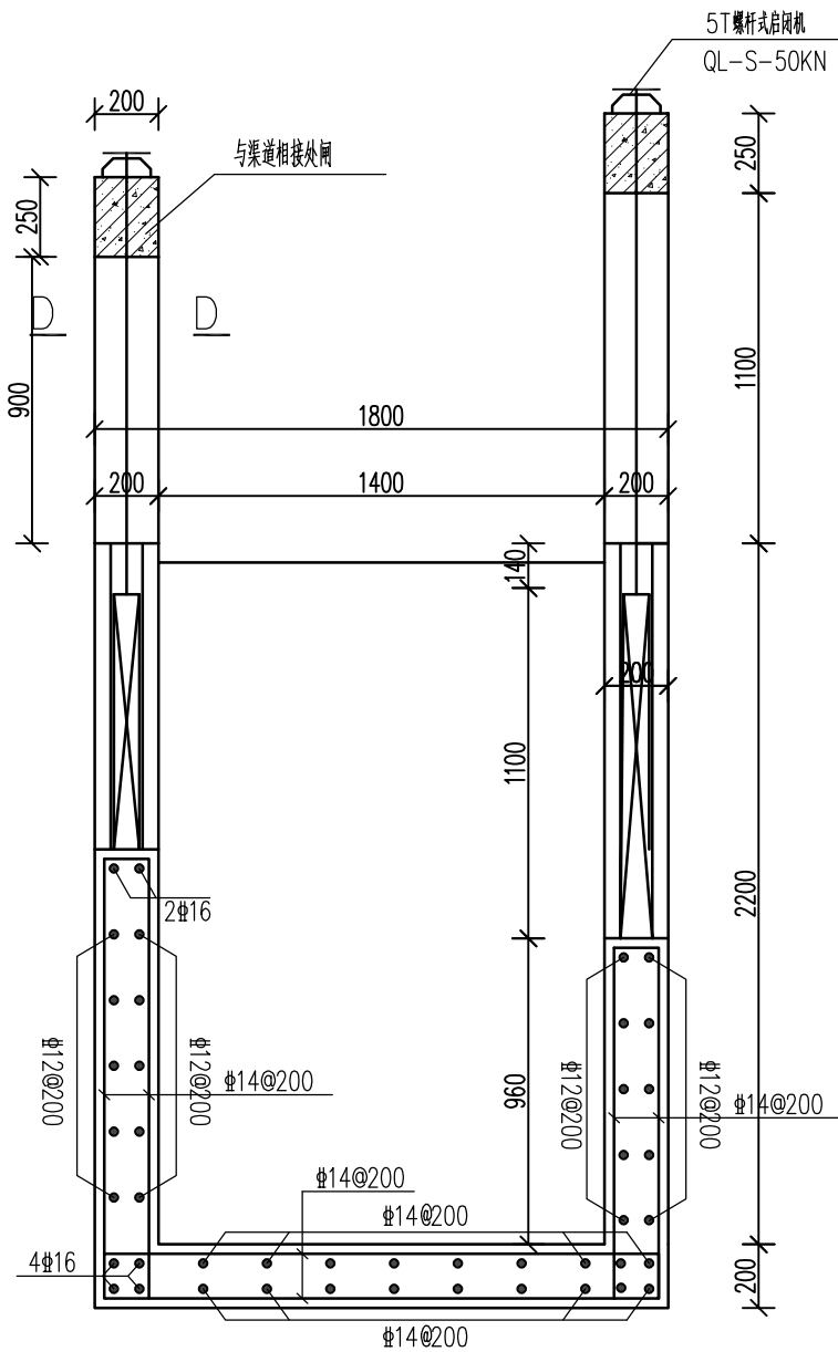
B--B钢筋图 1:25
