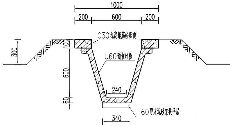
U60渠道断面图 1:25
