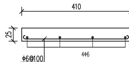
预制闸门配筋图 1:5
