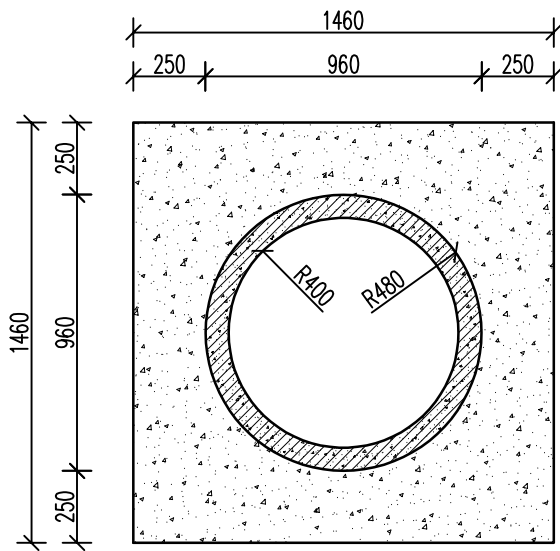
A-A 1:25
