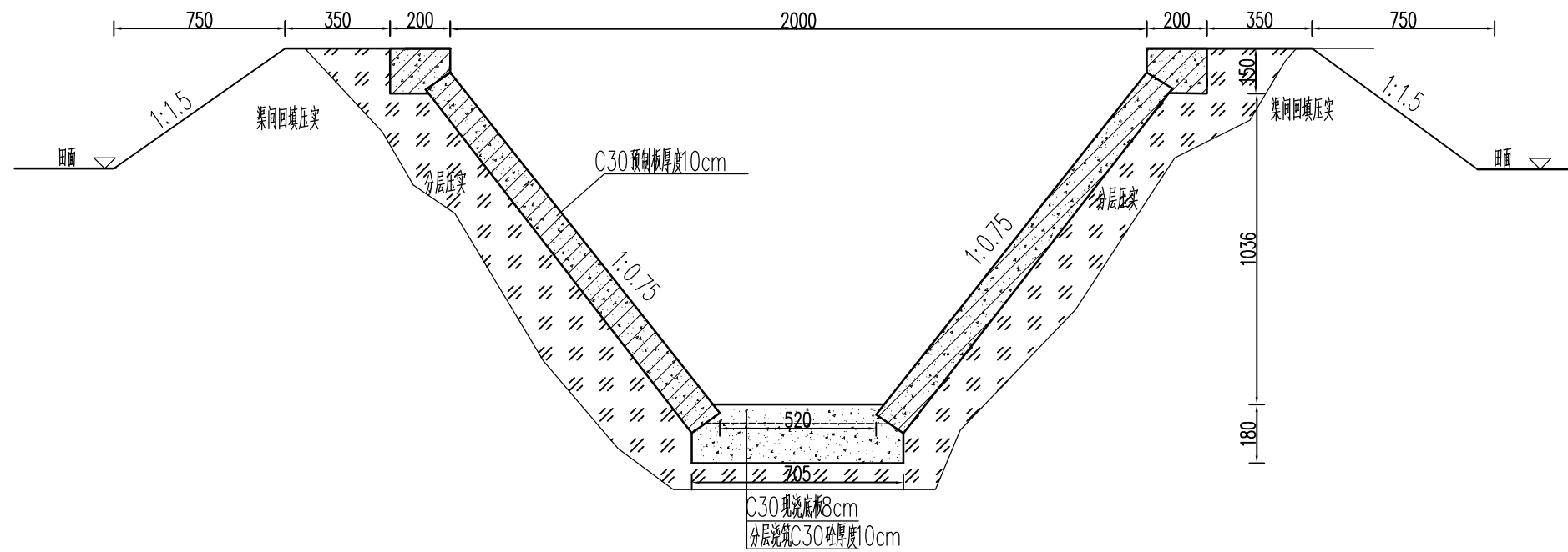
T200渠道断面图 1:25
