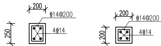
闸门排架剖面钢筋图 1:25
