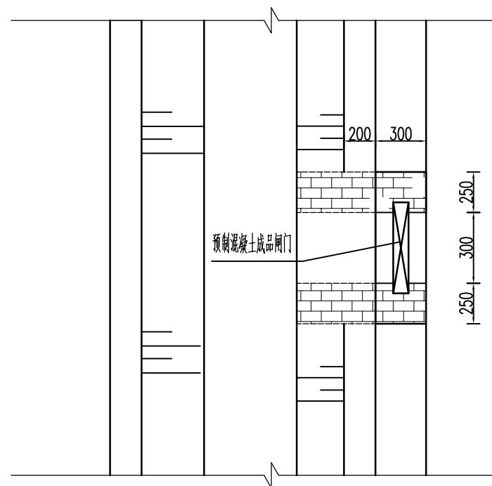
放水口平面图 1:20
