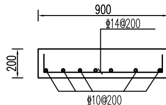
盖板配筋图 1:25
