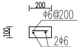
压顶配筋图 1:20
