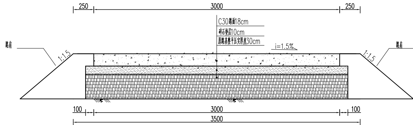
新建3.0m宽混凝土路横断面图 1:25 有路基
