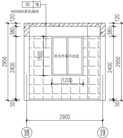
② 厨房立面详图 1:50
