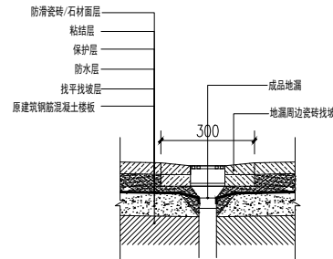
④ 地漏做法节点详图
