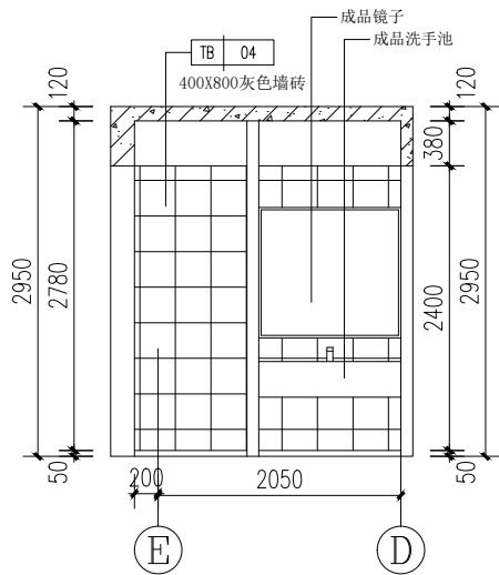
① 卫生间立面详图 1:50
