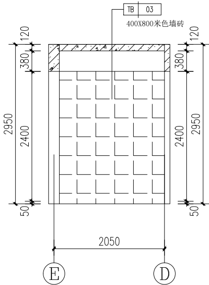
① 厨房立面详图 1:50
