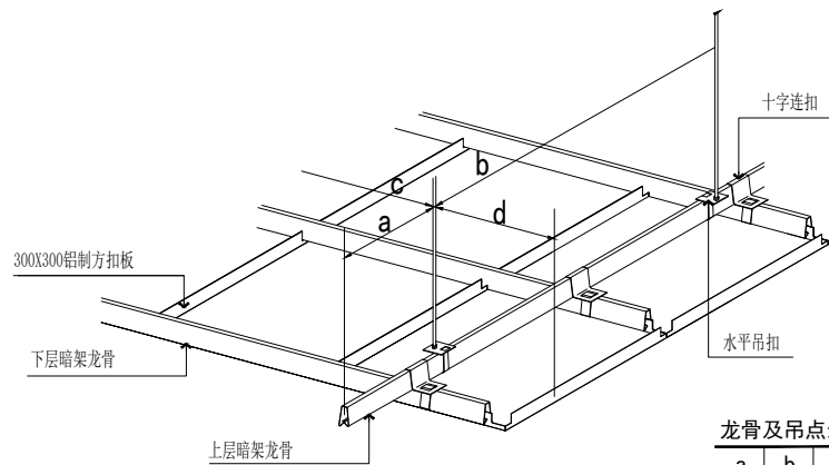
安装示意图
