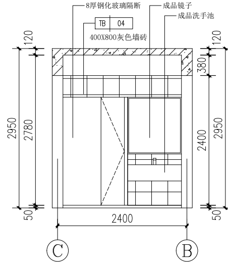
② 卫生间立面详图 1:50
