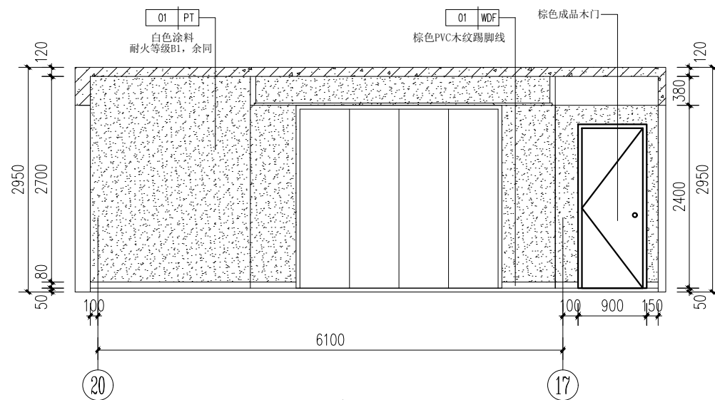
④ 客餐厅立面详图 1:50
