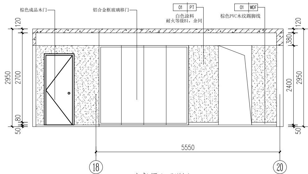
② 客餐厅立面详图 1:50
