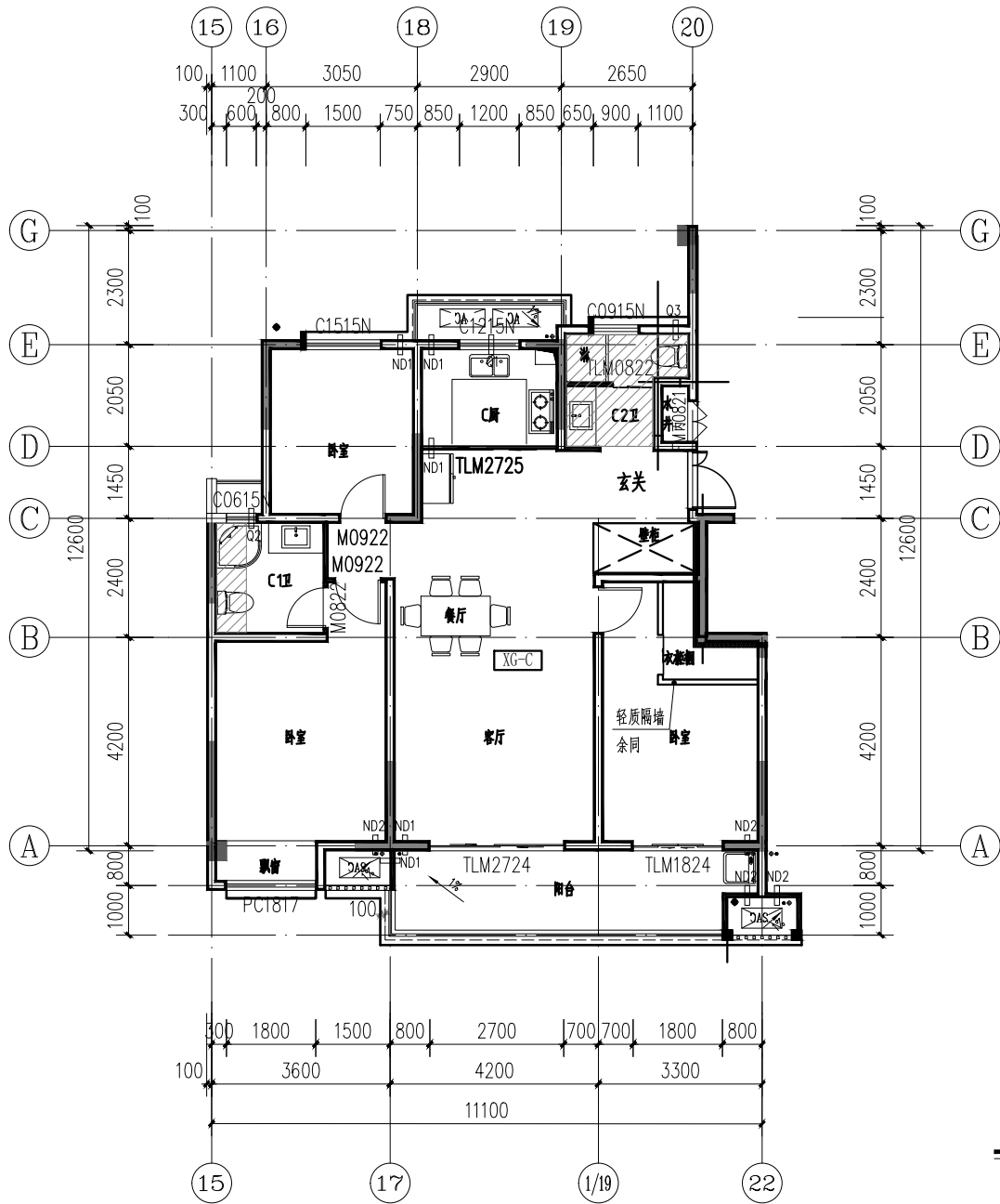
原始平面图 1:100
