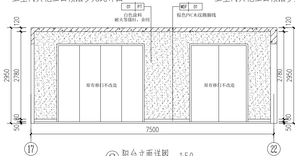
③ 阳台立面详图 1:50
