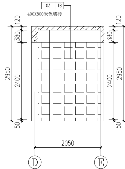
③ 厨房立面详图 1:50
