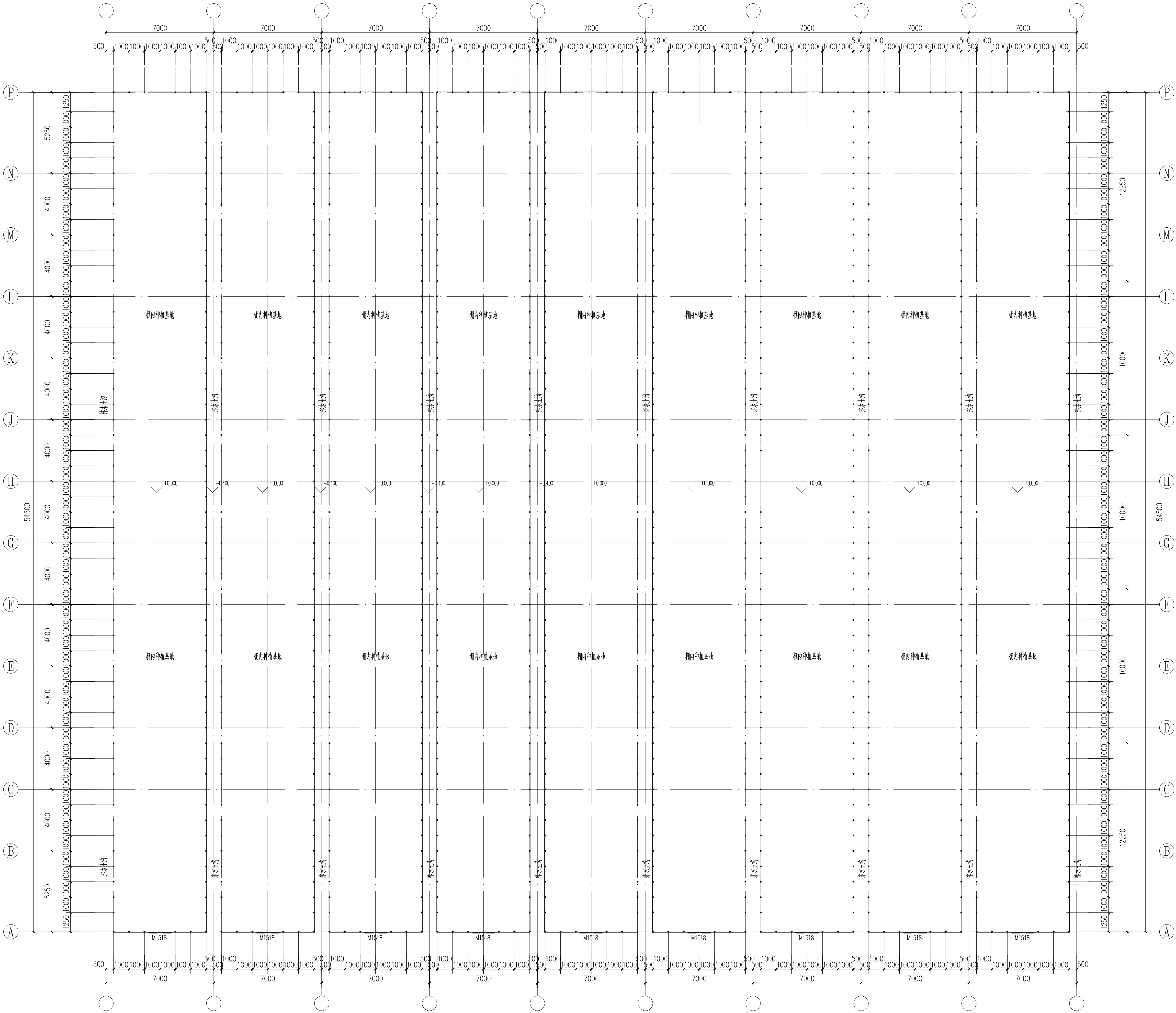
单棚局部平面图 1:120
