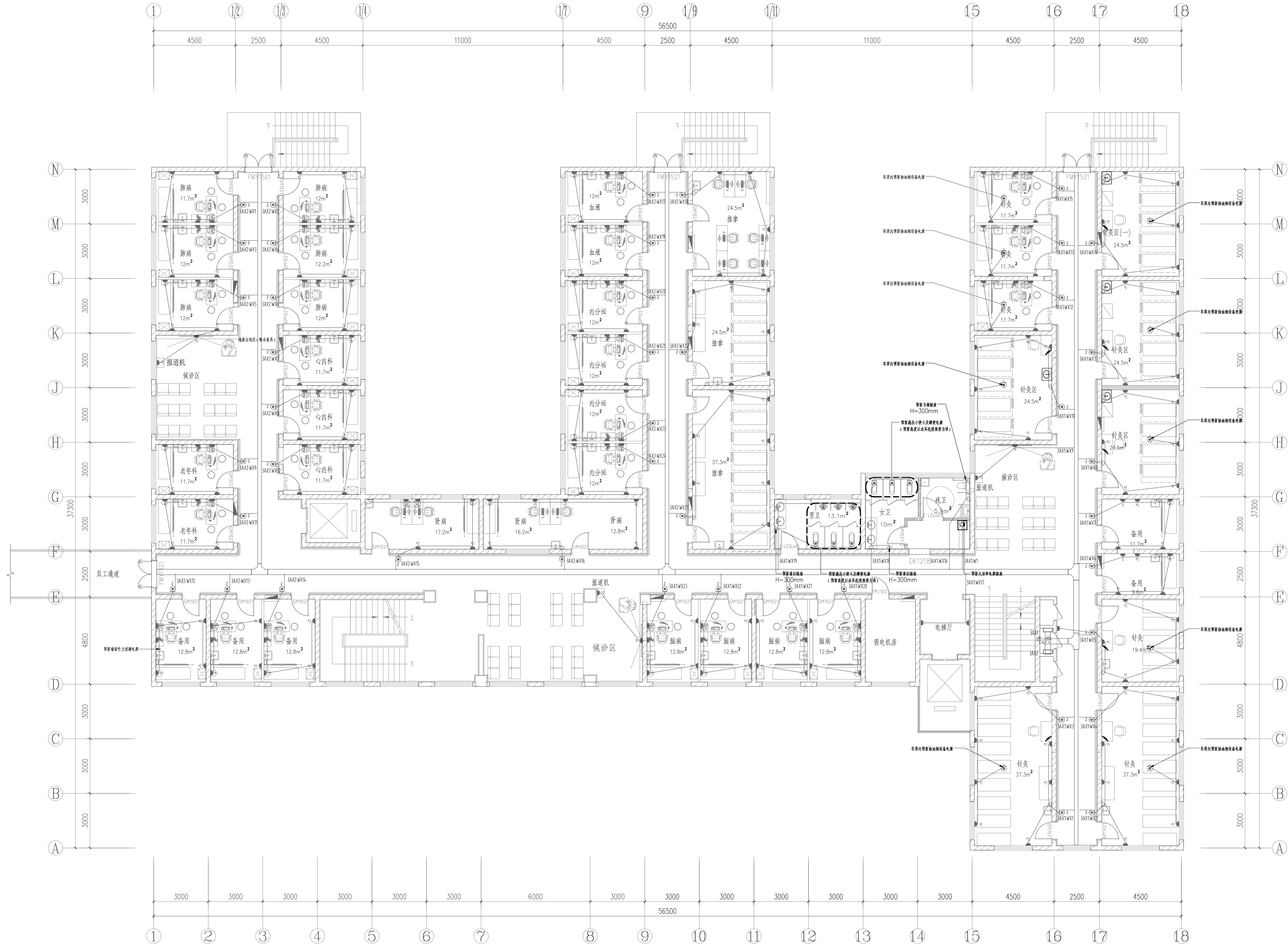
三层平面图 1:100
