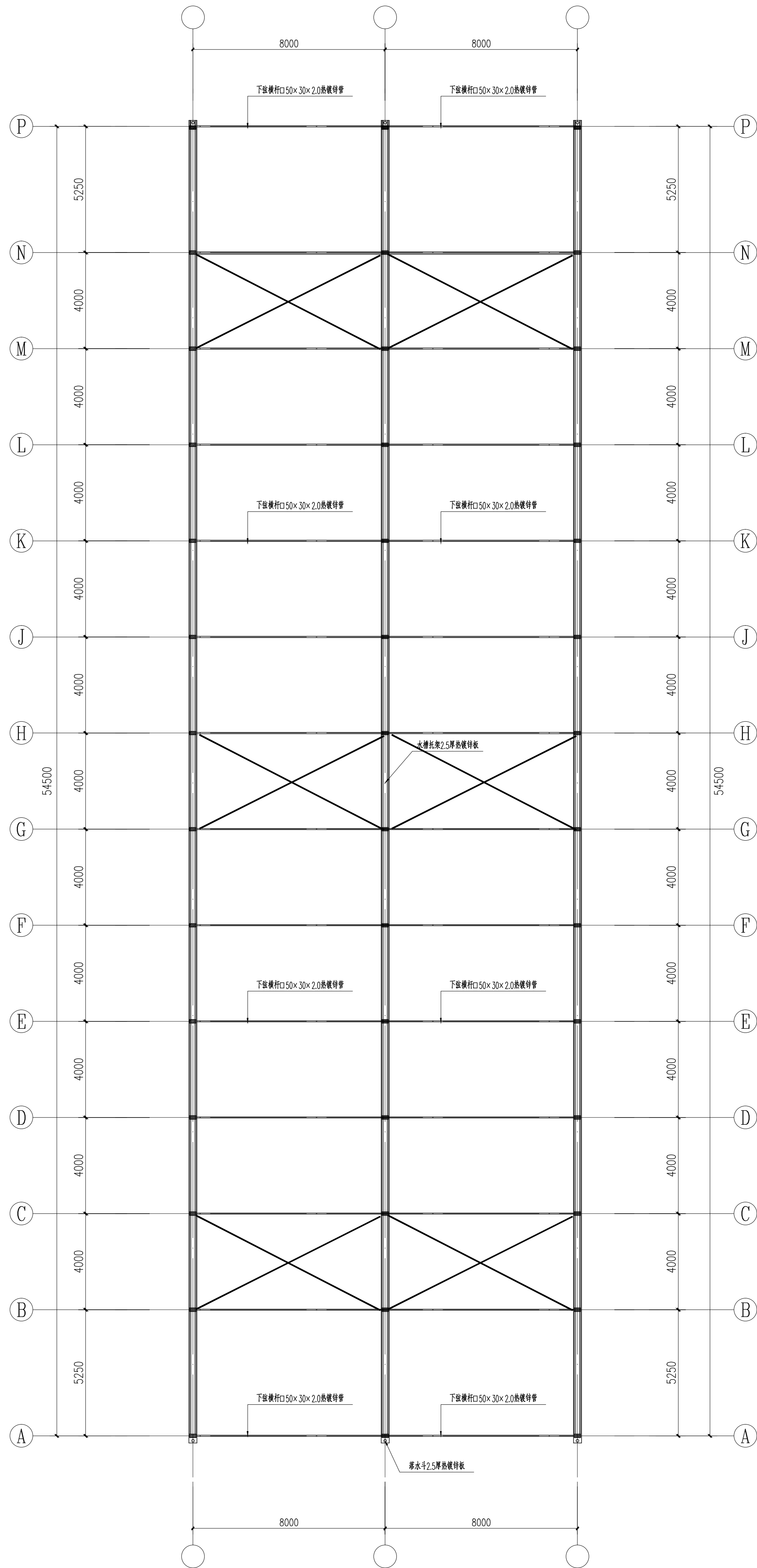
顶层平面布置图 1:120
