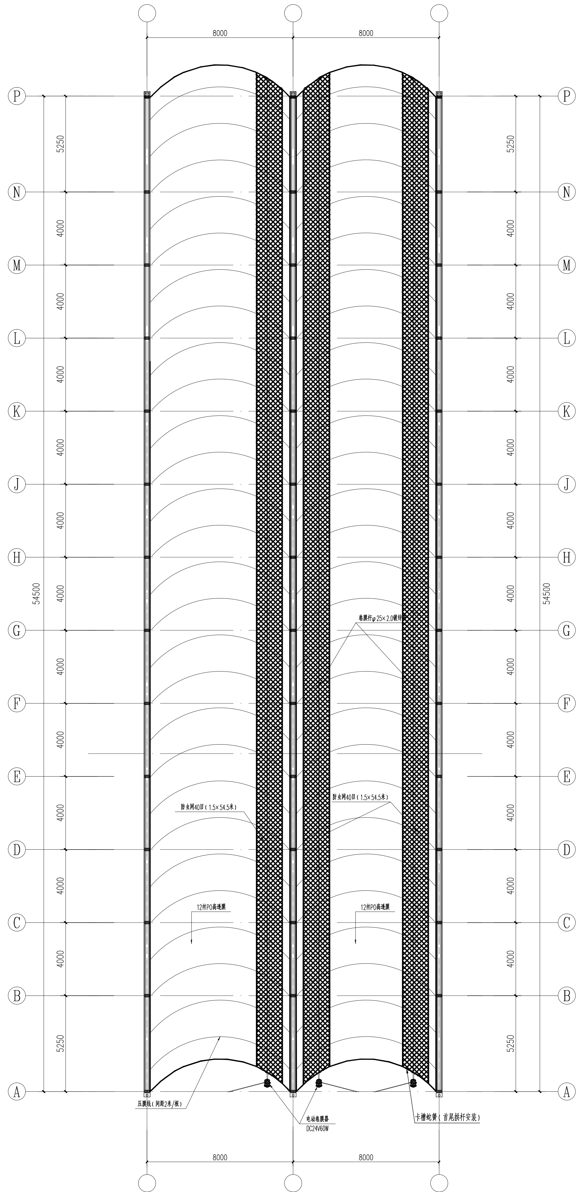
顶面布置图 1:120
