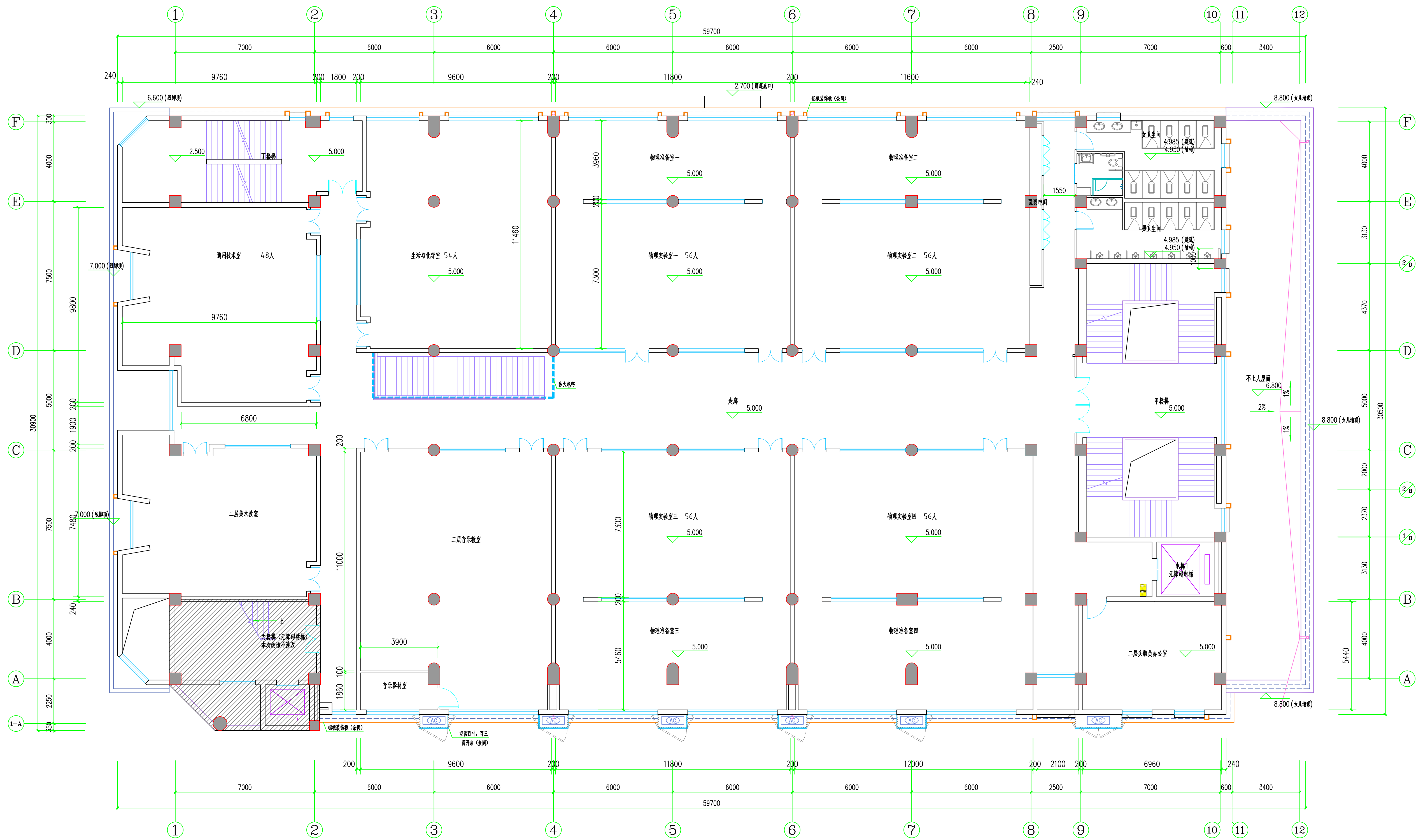
二层平面图 1:100 本层建筑面积1655.24m 2
