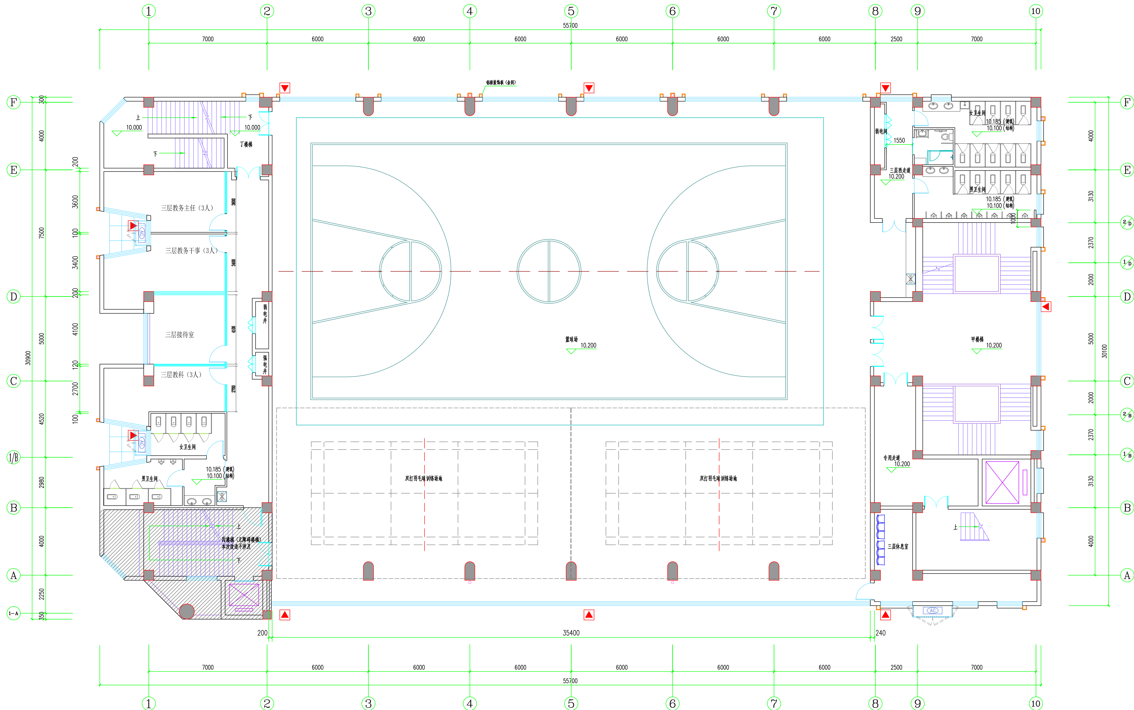
三层平面图 1:100 本层建筑面积1646.21m² ▲ 楼梯间入口
