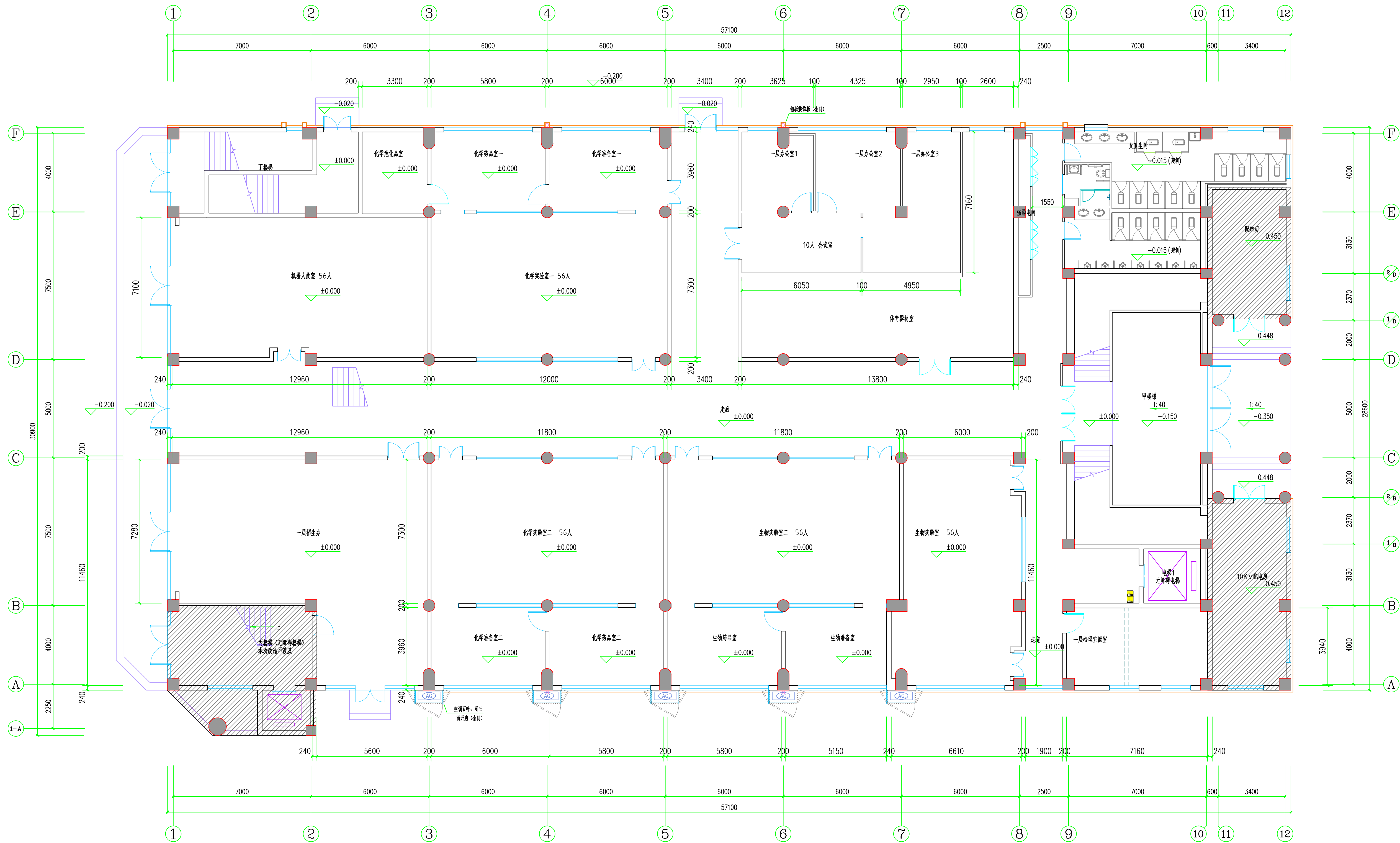
一层平面图 1:100 本层建筑面积1639.89m²
