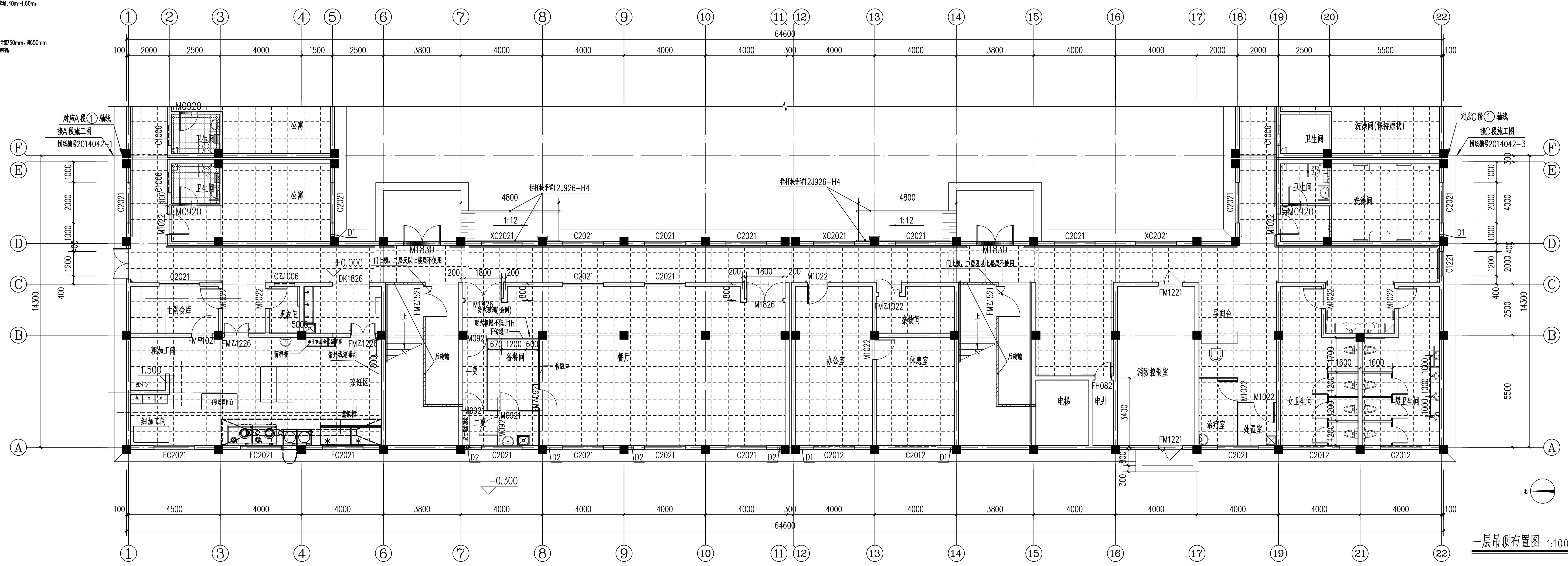
一层地面铺装图 1:100
