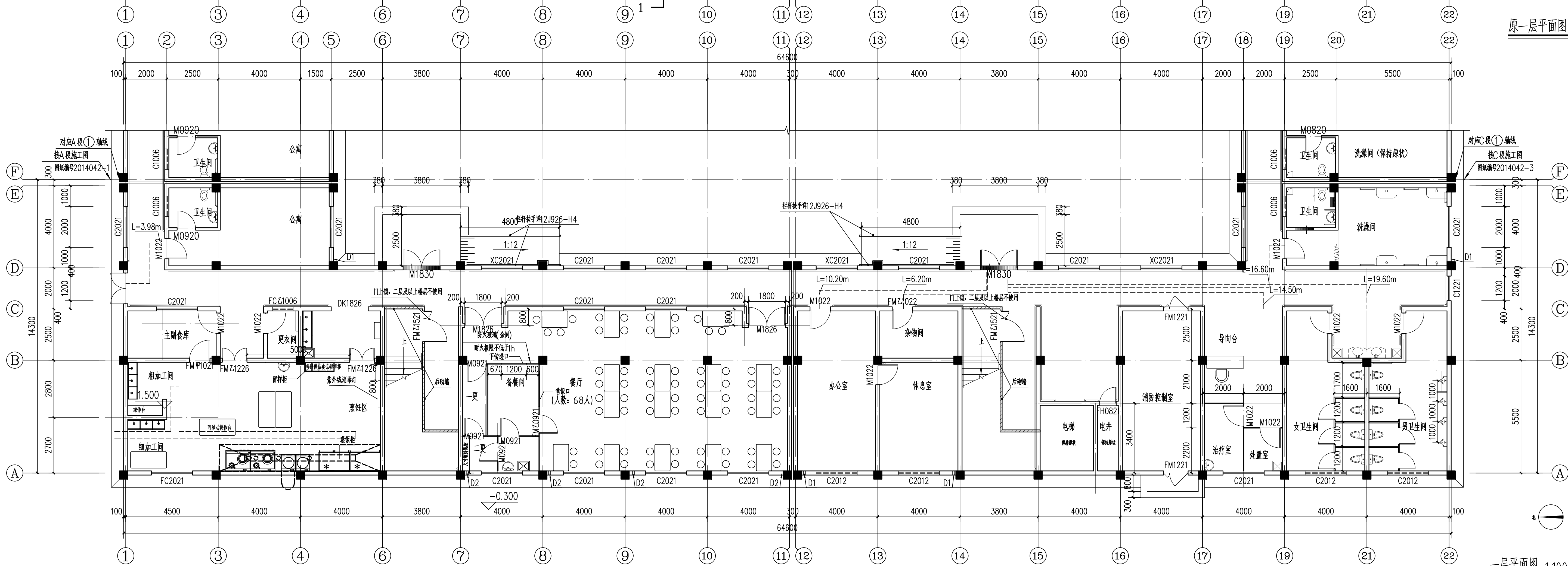
一层平面图 1:100
