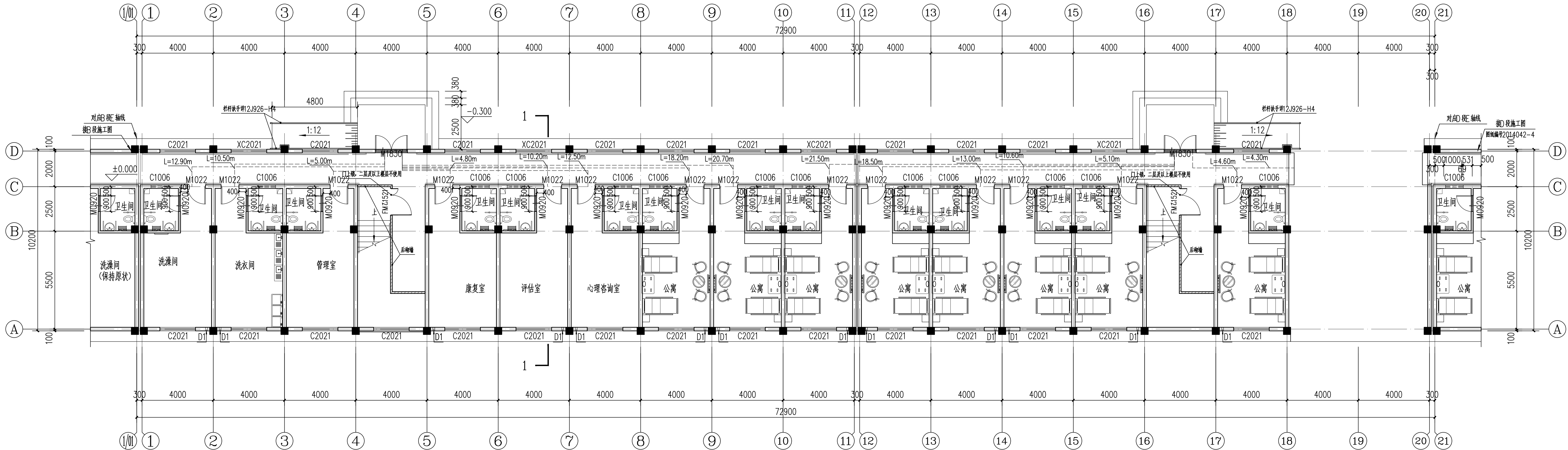
一层平面图 1:120
