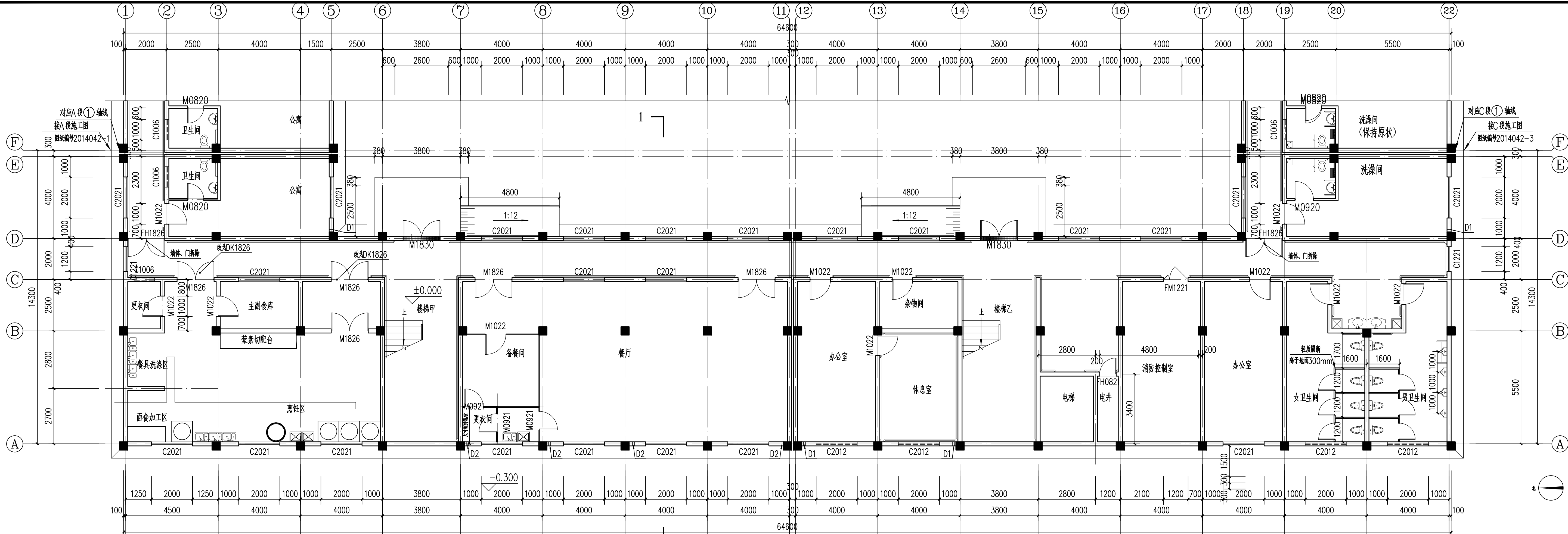
原一层平面图 1:100
