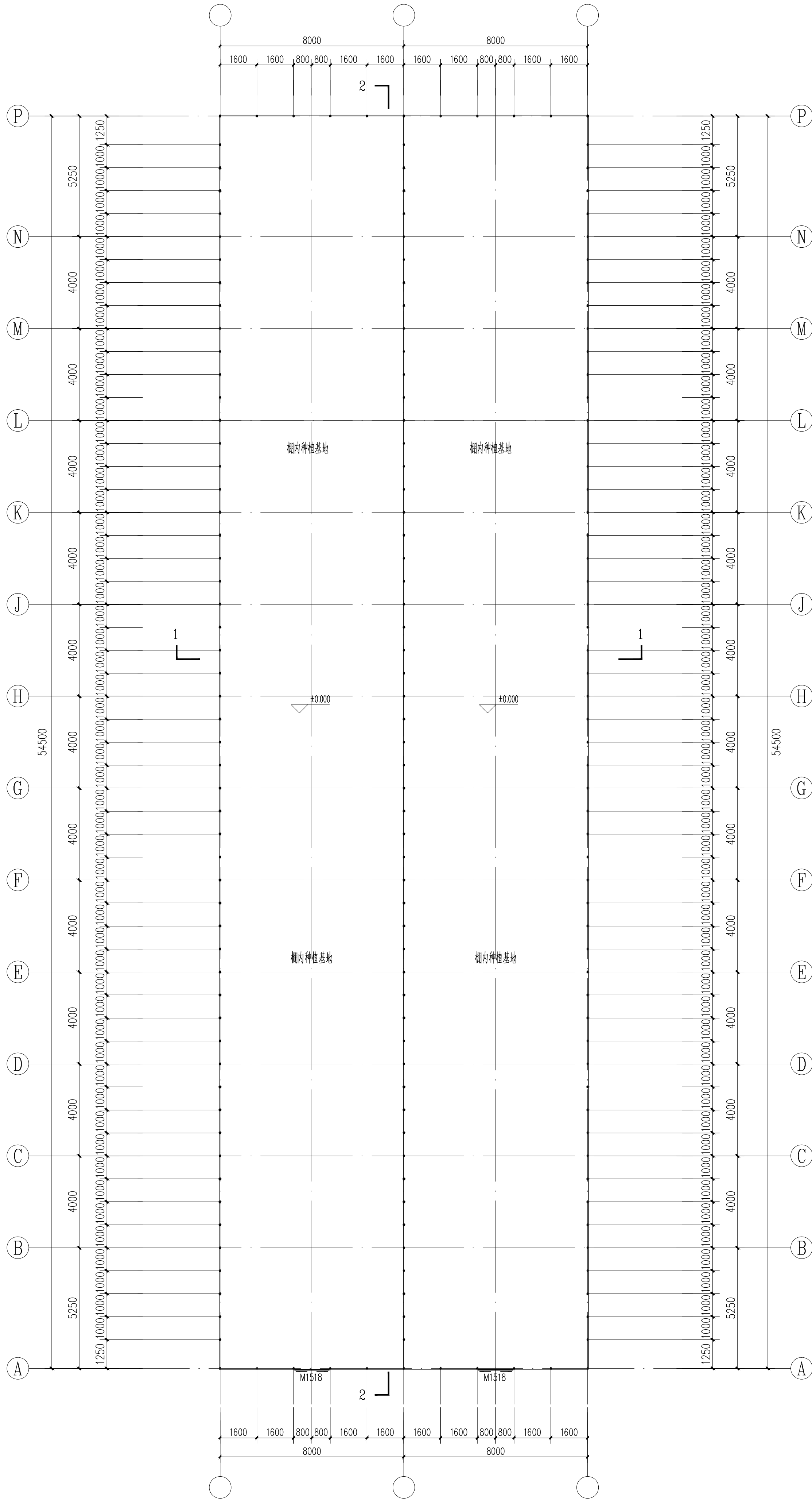
连栋棚局部平面图 1:120
