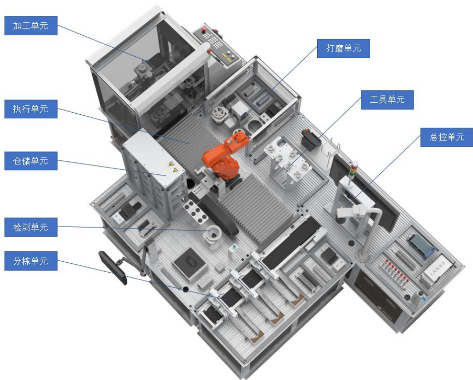
图 6 单元构成
