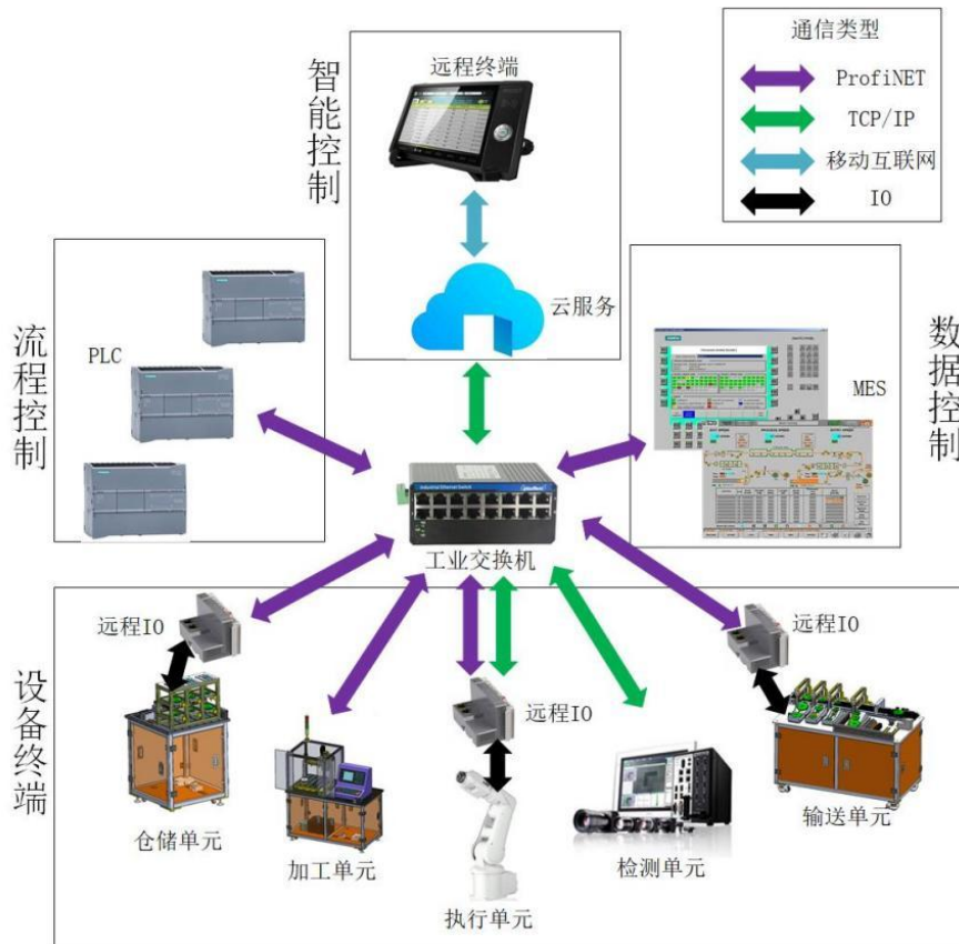
图 5 控制逻辑结构
